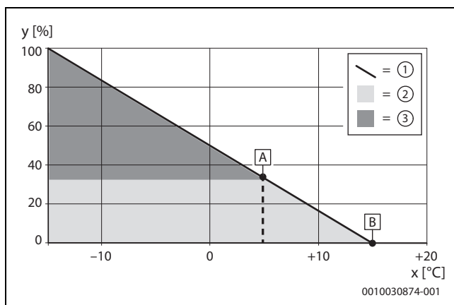
Afb. 1 Buitentemperatuur parallel
