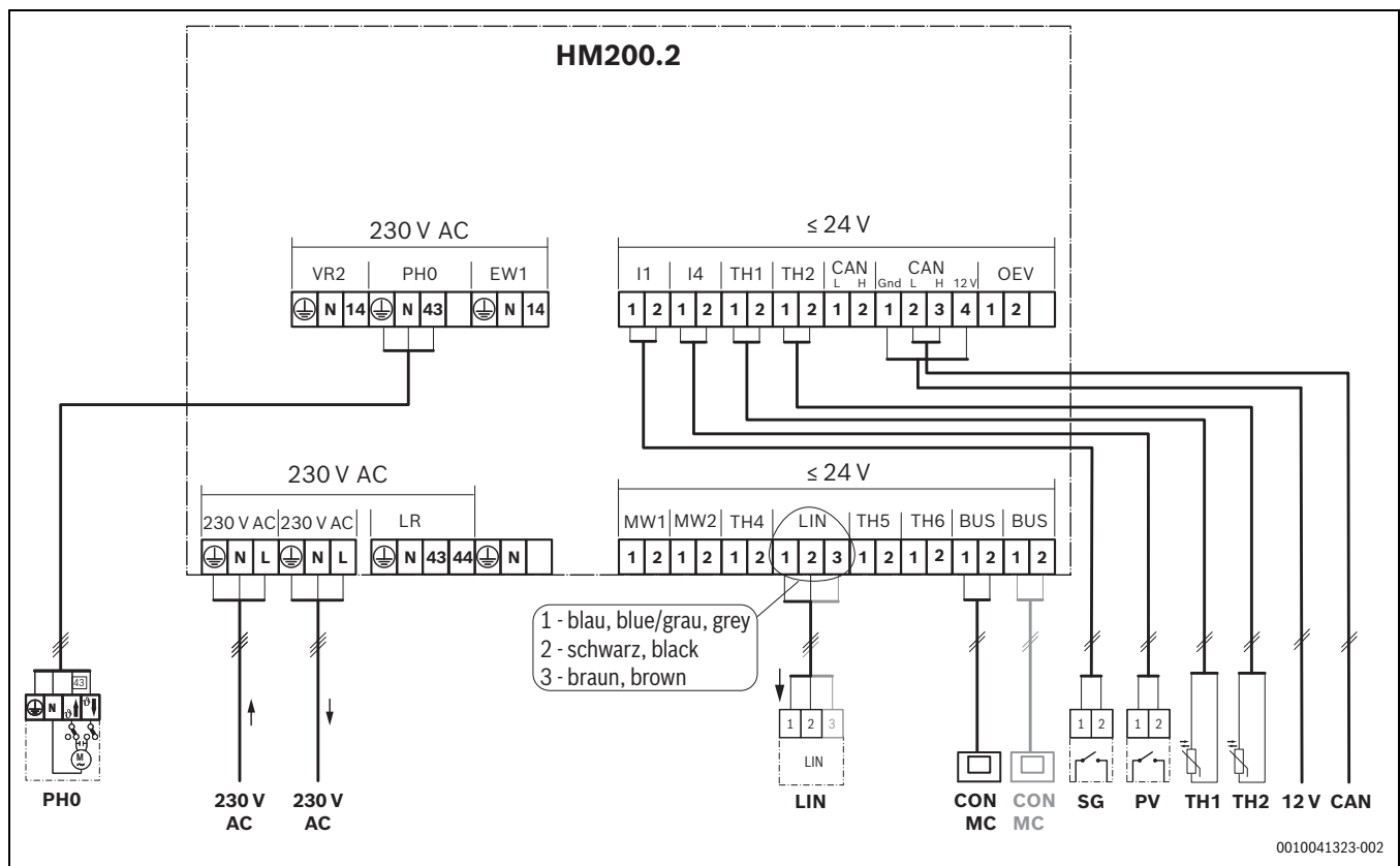
Bild 4 Überblick Anschlussklemmenbelegung
