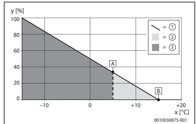
Afb. 2 Buitentemperatuur alternatief
