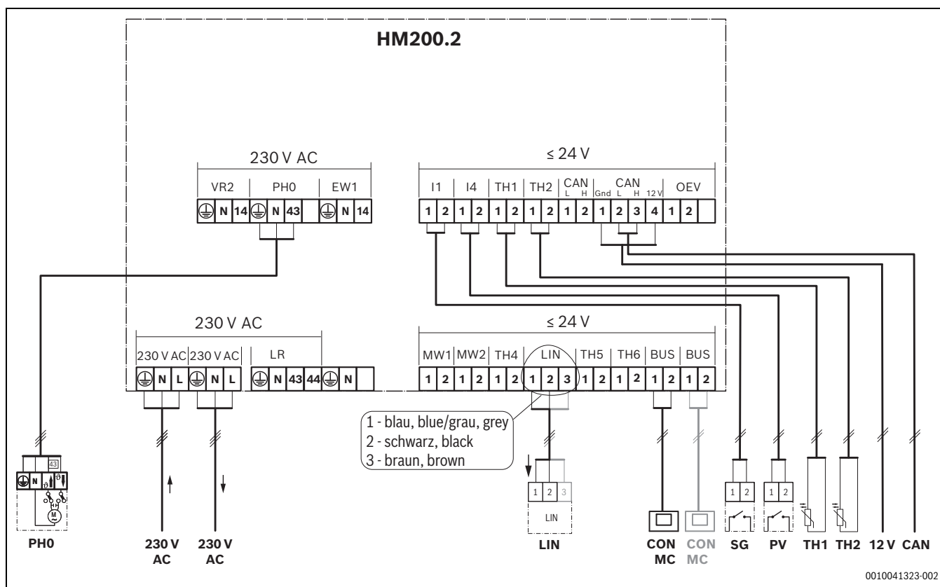
Afb. 4 Overzicht bezetting aansluitklemmen
