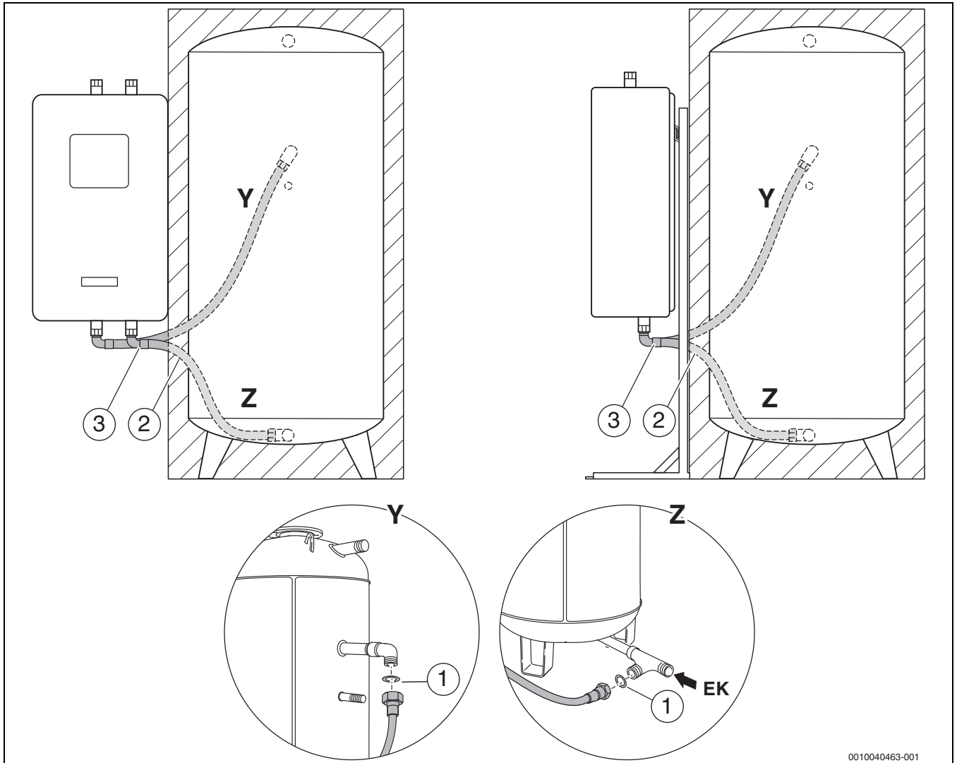
Bild 30 Links: Wandinstallation der Station; rechts: Station an Bodenständer montiert
