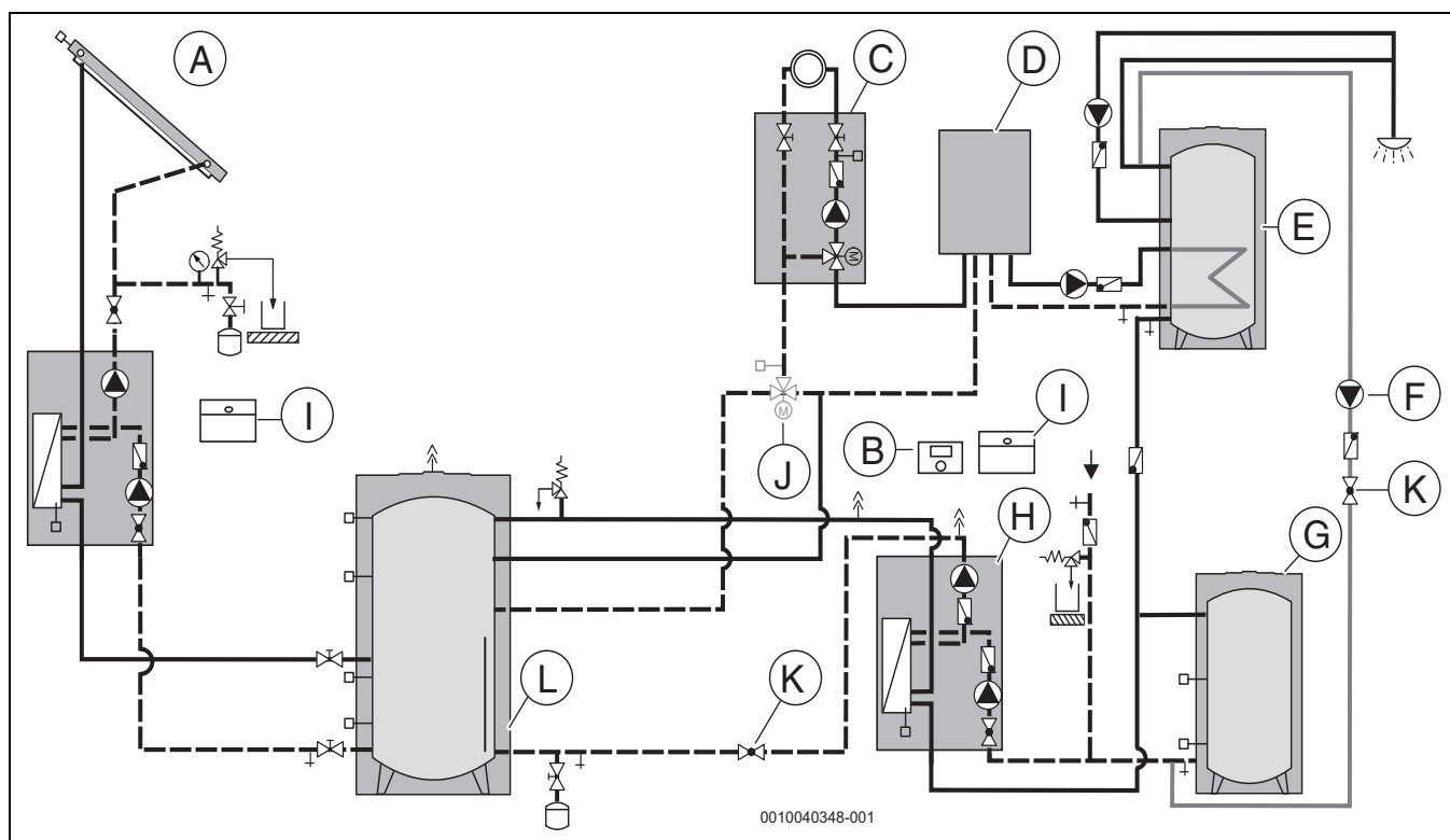
Bild 10 Anlagenbeispiel mit Optionen: Vorwärmstufe mit Umladebetrieb von Pufferspeicher auf Vorwärmpeicher (diese schematische Darstellung gibt keinen Hinweis auf eine mögliche Ausführung vor Ort)
