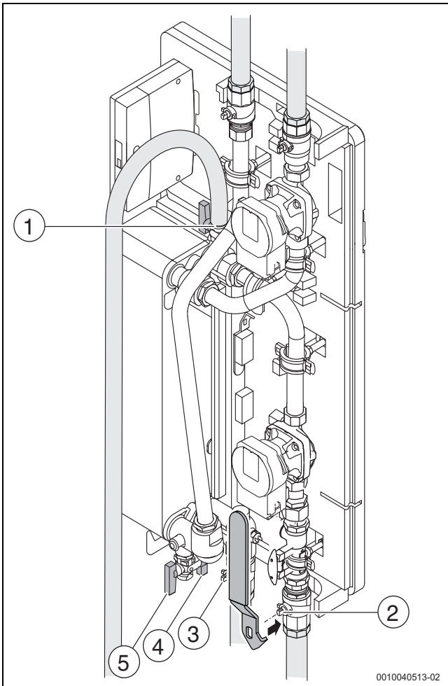
Bild 37 Wärmetauscher reinigen
