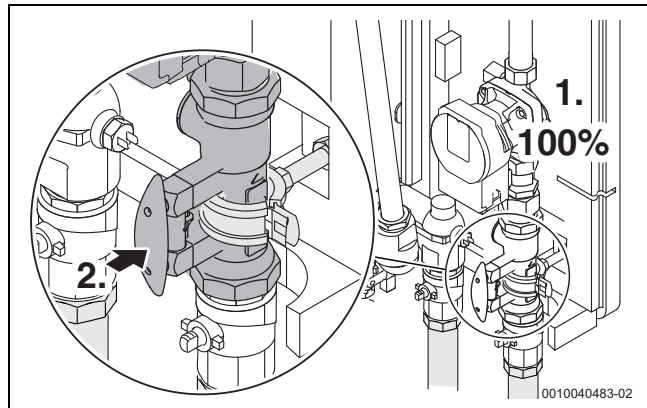
Bild 35 Durchflussbegrenzer Sekundärseite
