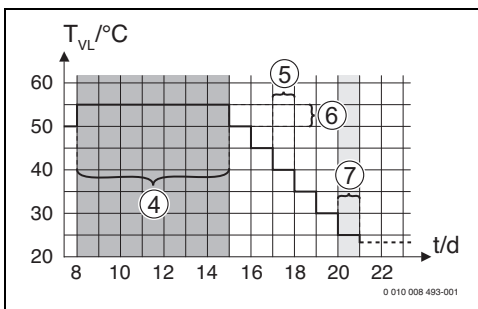
Bild 17 Ablauf der Estrichrocknung mit den Grundeinstellungen in der Abkühlphase
