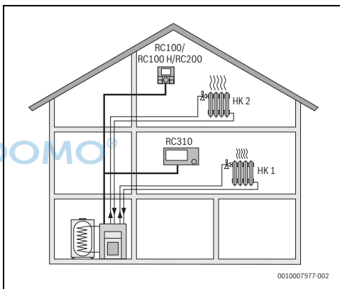
Bild 2 RC100/RC100 H/RC200 als Fernbedienung für den zweiten Heizkreis (HK 2) und RC310 als Regler für den ersten Heizkreis (HK 1)
