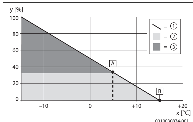
Fig. 1 Temperatura esterna parallela
