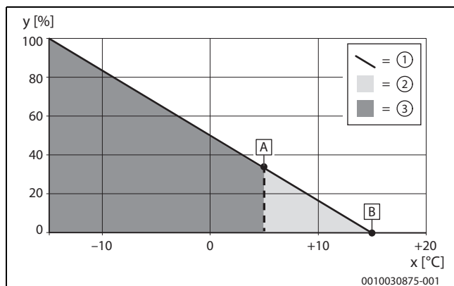
Fig. 2 Température extérieure alternative
