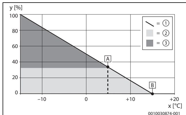
Afb. 1 Buitentemperatuur parallel
