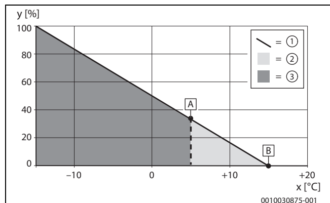
Afb. 2 Buitentemperatuur alternatief
