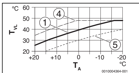
Bild 11 Einstellung der Heizkurve für Fußbodenheizung Parallelverschiebung über gewünschte Raumtemperatur
