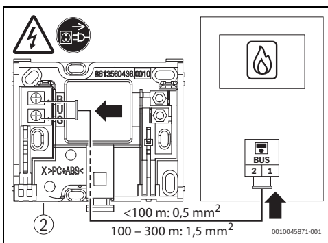
Bild 6 Anschluss der Bedieneinheit an einem Wärmeerzeuger
