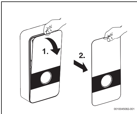
Bild 10 Frontblende abnehmen
