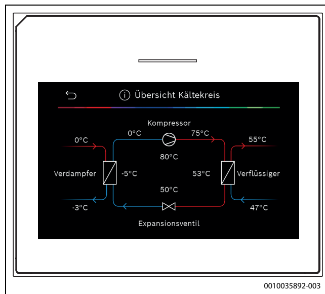
Bild 10 Übersicht Kältekreis
