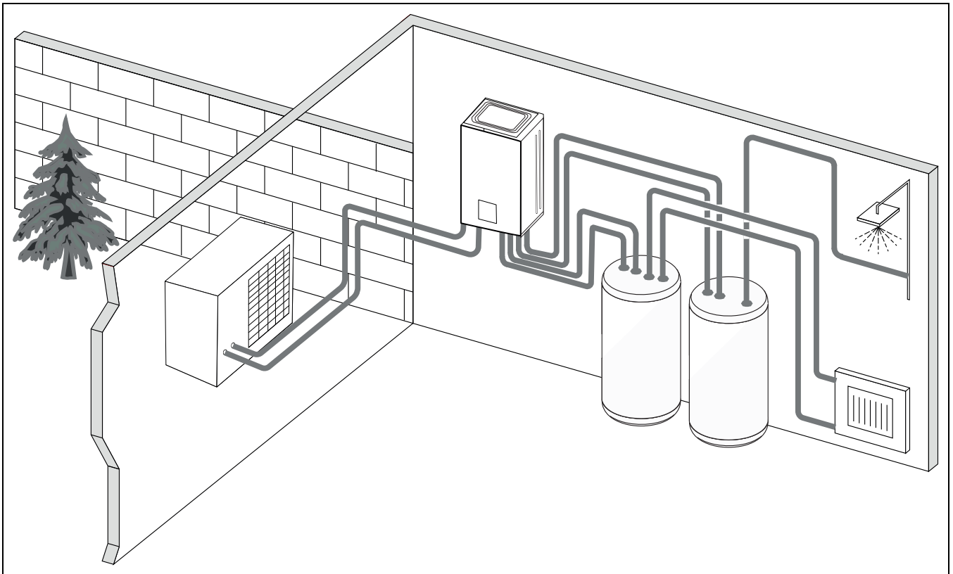
Bild 7 Wärmepumpe Logatherm WLW MB AR, Inneneinheit Logatherm WLW176i/186i E mit elektrischem Zuheizer und externem Warmwasserspeicher
