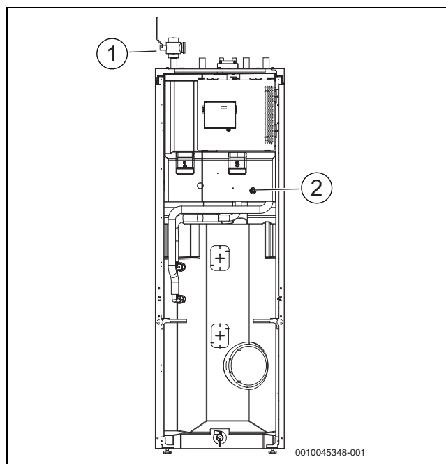
Bild 13 Logatherm WLW176i/186i T
