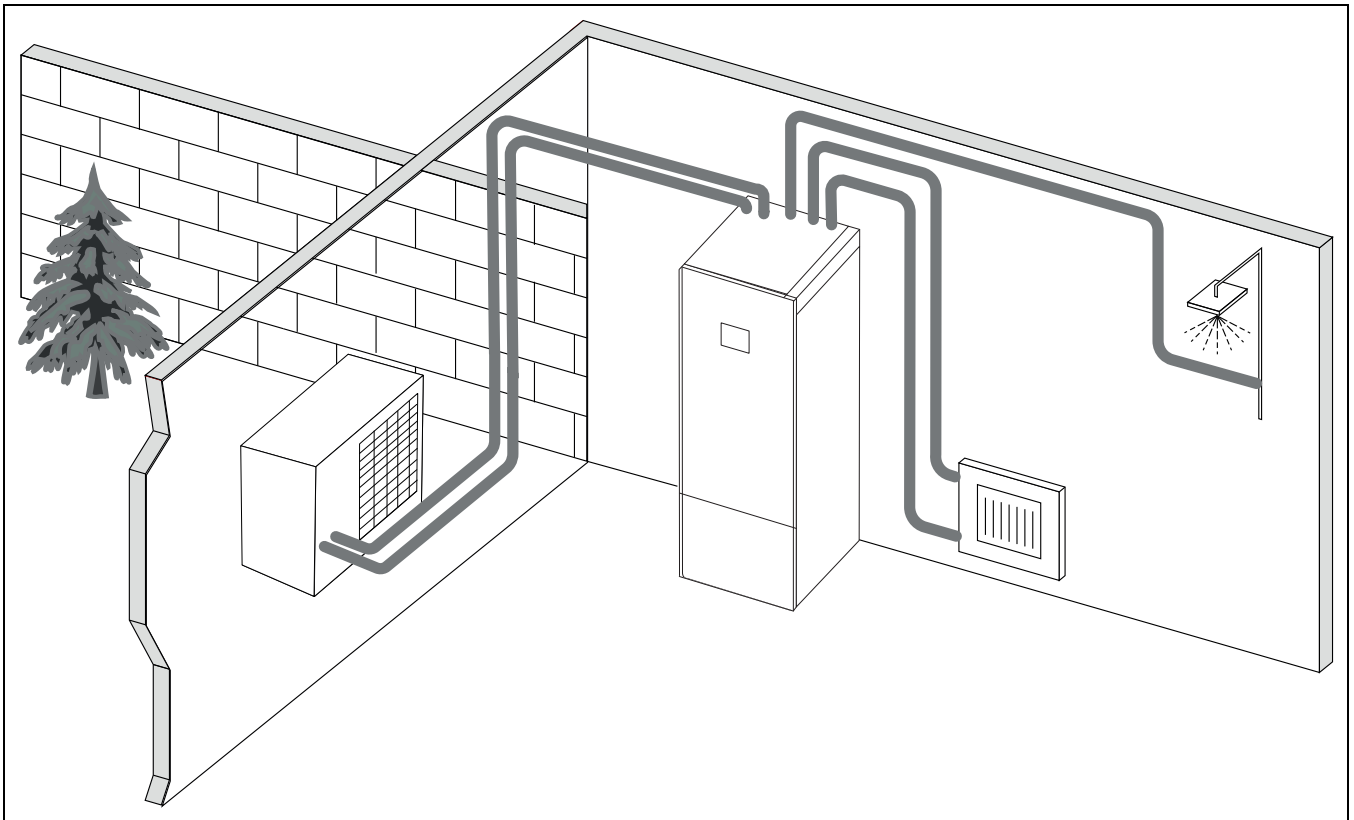
Bild 7 Wärmepumpe Logatherm WLW MB AR, Inneneinheit Logatherm WLW176i/186i T mit integriertem Warmwasserspeicher und elektrischem Zuleiter
