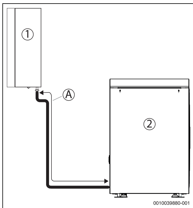
Bild 15 Rohrlänge A
