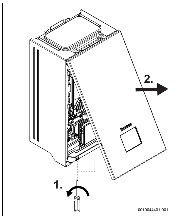
Bild 10 Frontplatten abnehmen
