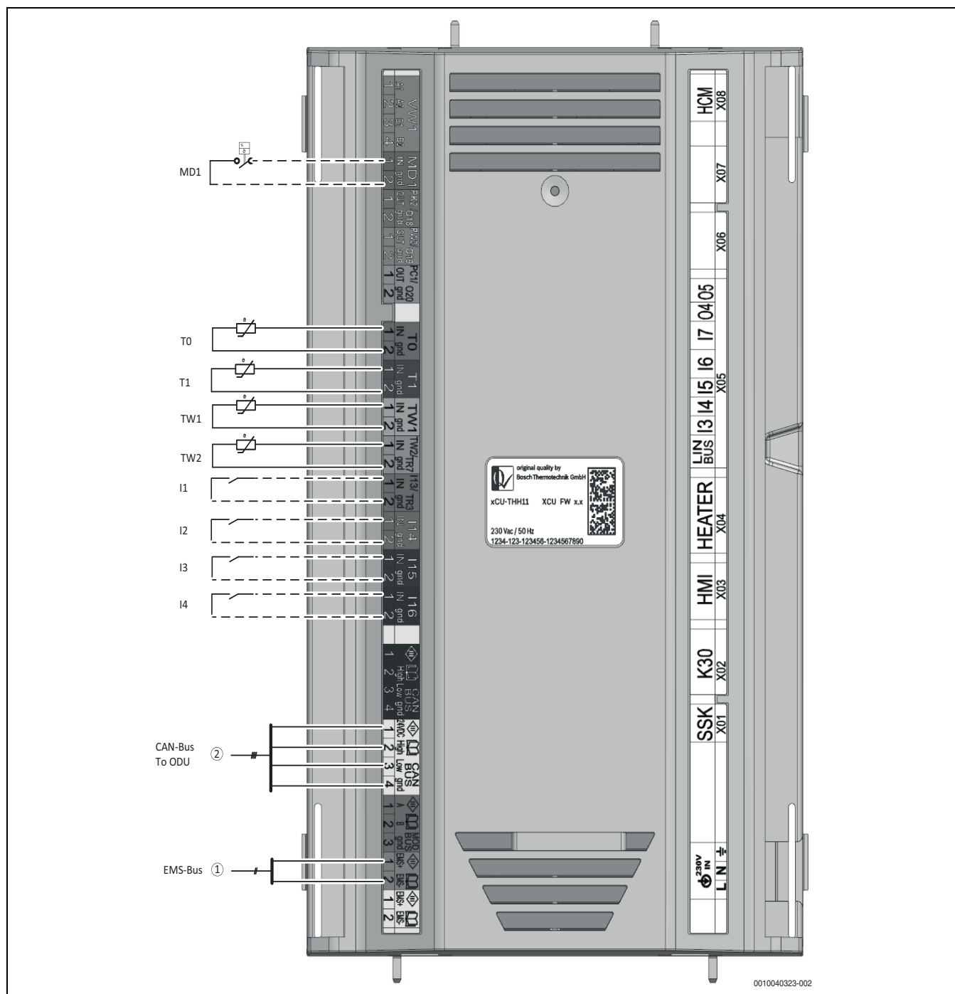
Bild 34 Anschlüsse
