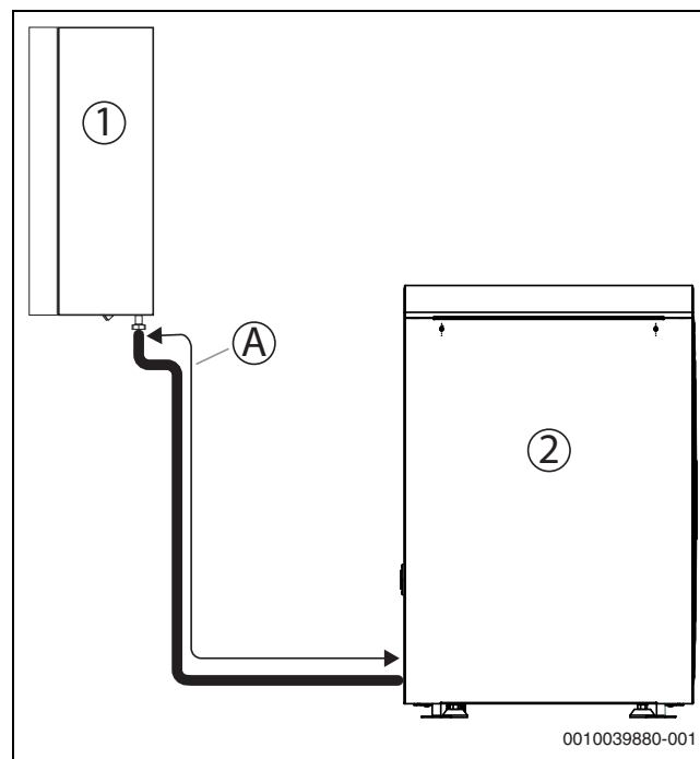
Bild 15 Rohrlänge A
