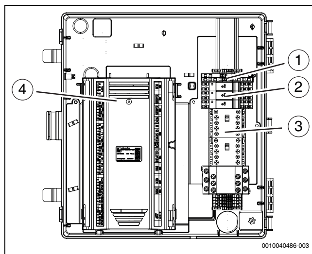
Bild 28 Anordnung der Bauteile im Klemmenkasten
