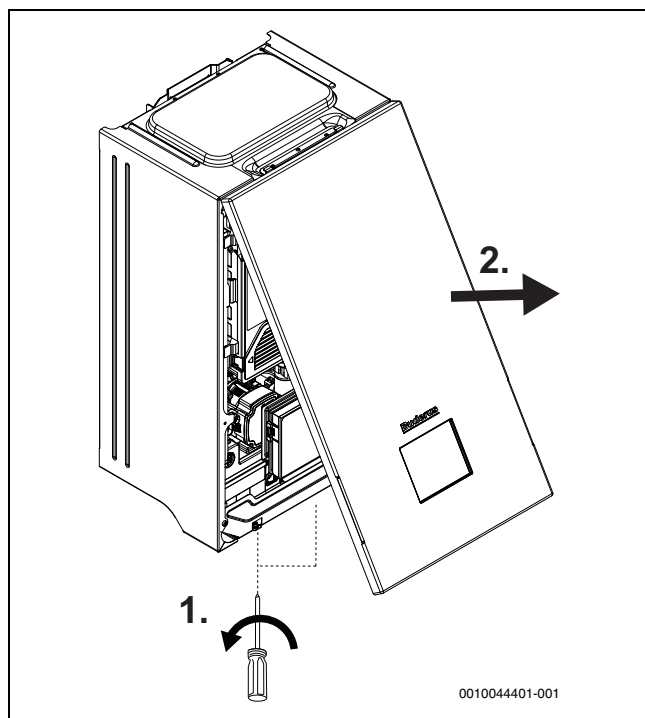
Bild 10 Frontplatten abnehmen
