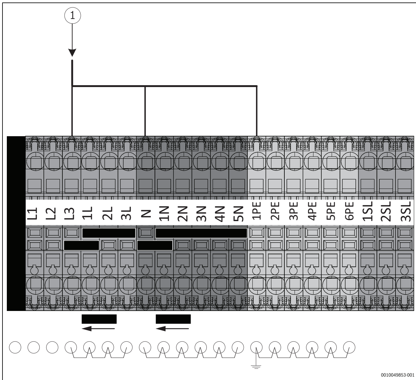
Bild 31 Elektrischer Anschluss, einphasig, nur 3 kW
