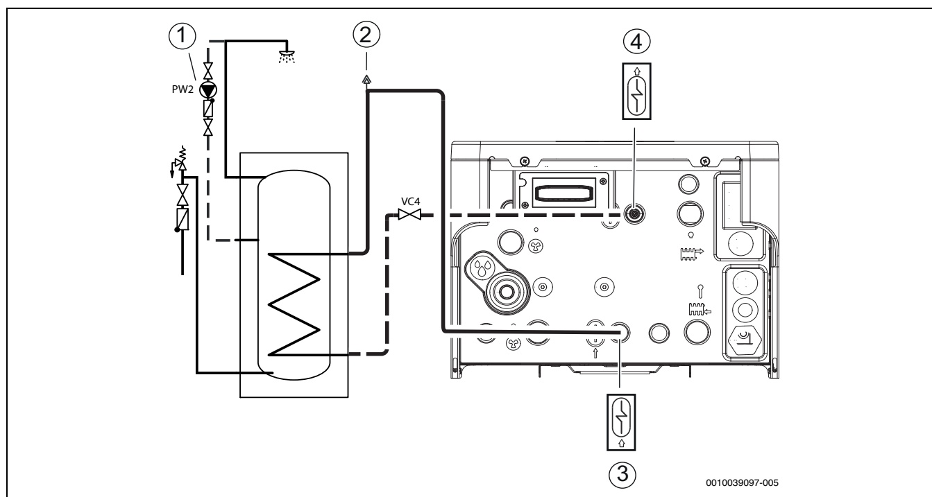
Bild 18 Trinkwasseranschlüsse Inneneinheit
