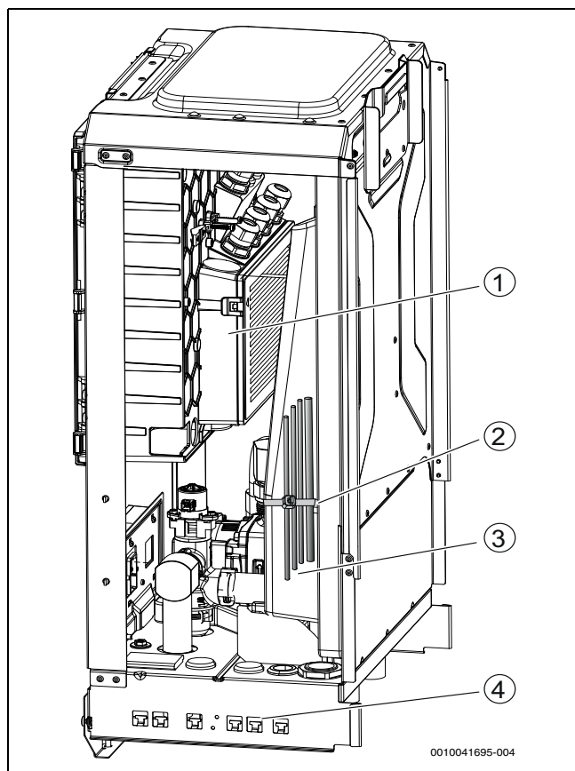
Bild 26 Kabelführung
