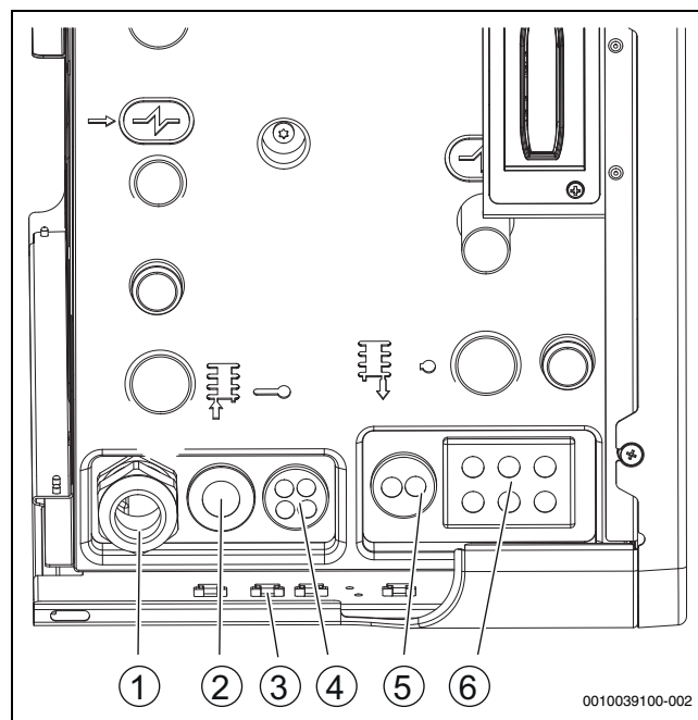
Bild 25 Kabeleinführungen der Inneneinheit
