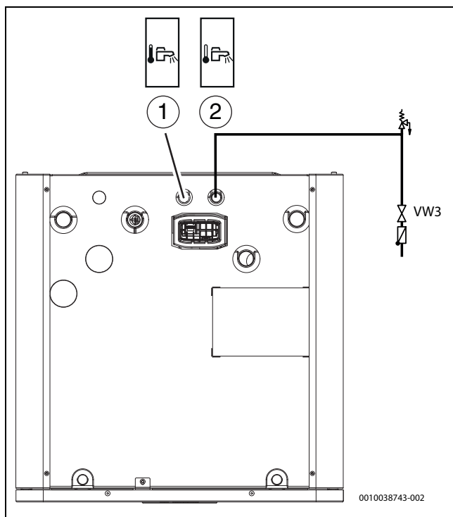
Bild 23 Wärmepumpenanschlüsse Trinkwasser
