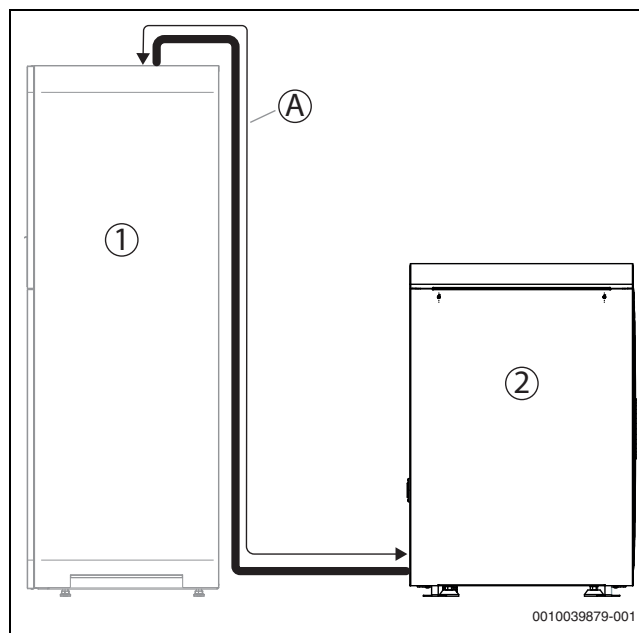
Bild 19 Rohrlänge A
