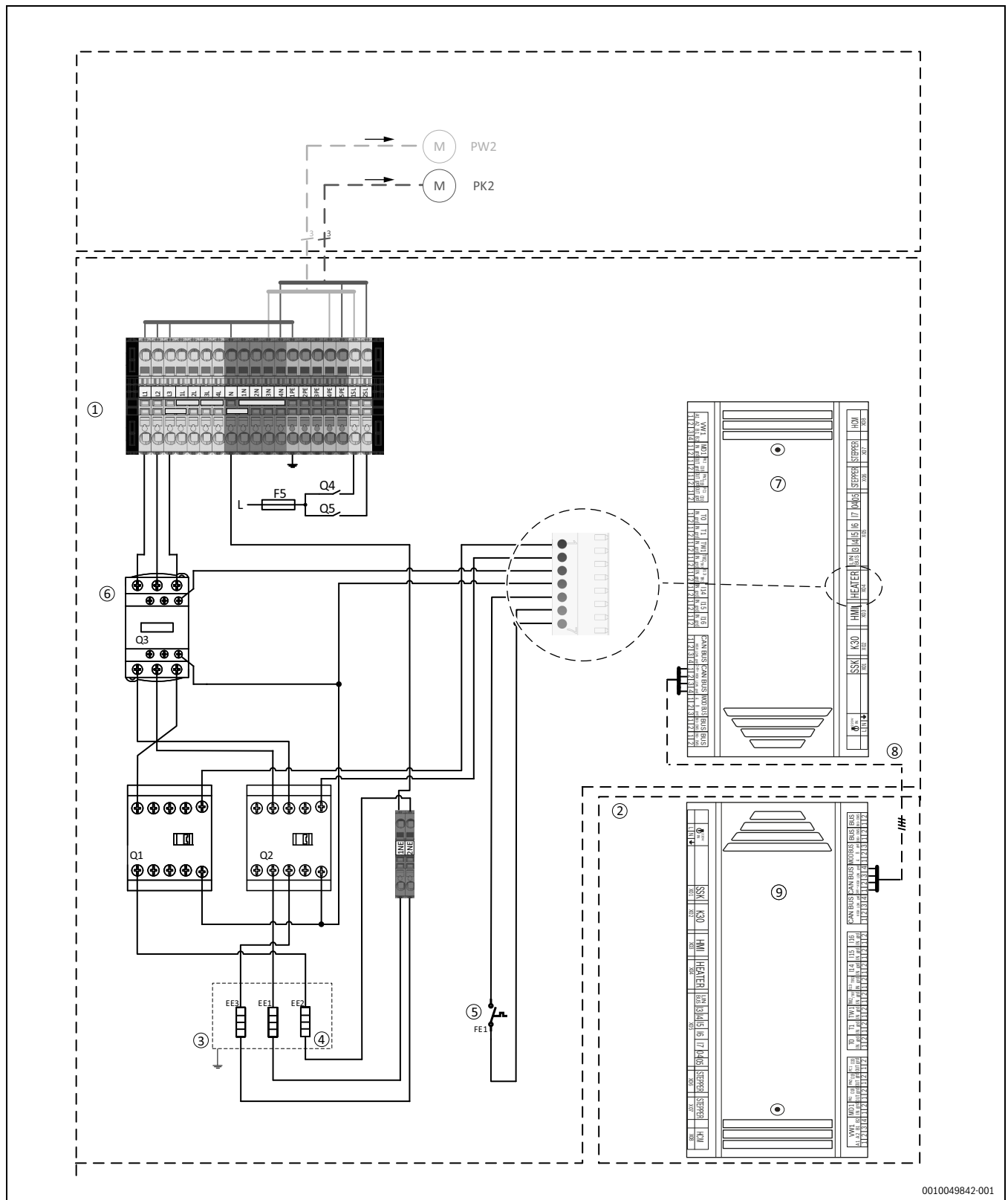
Bild 52 Spannungsversorgung Inneneinheit
