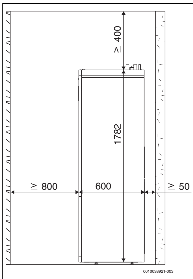
Bild 2 Mindestabstand (mm)
