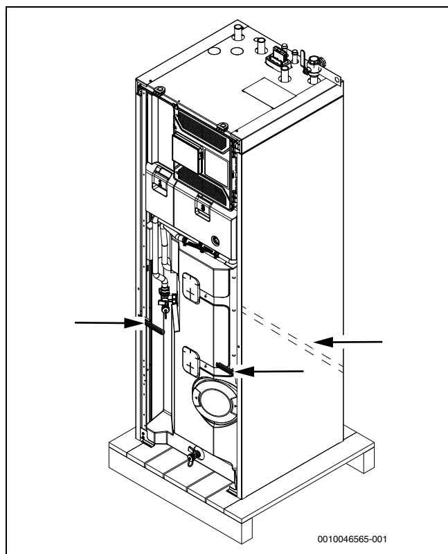
Bild 10 Transportbügel
