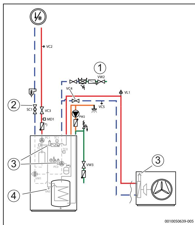
Bild 24 Inneneinheit, Wärmepumpe und Heizungsanlage (nur für Polen)
