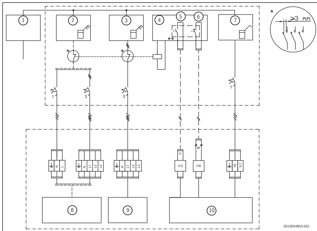
Bild 42 Alternative Lösung
