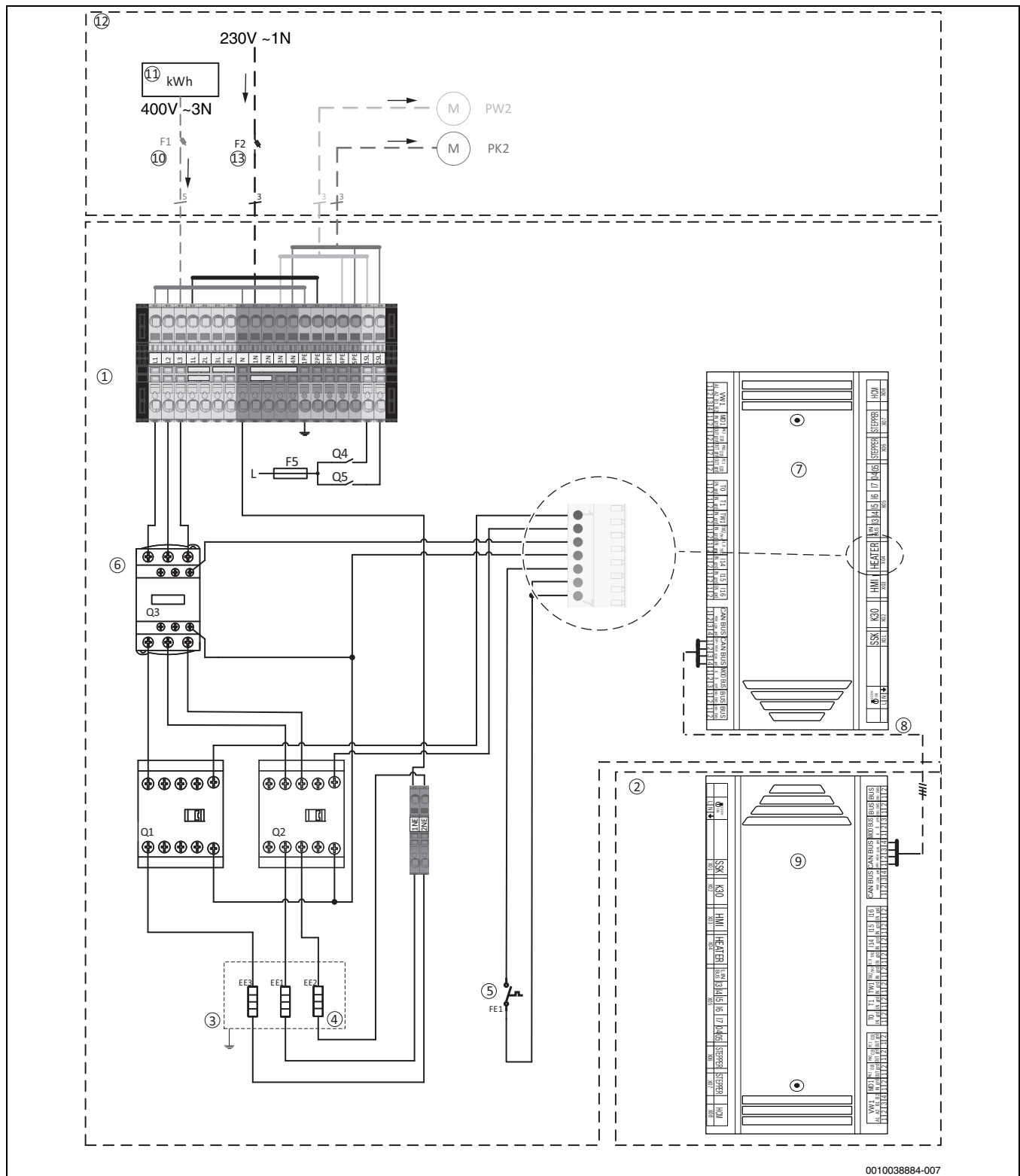
Bild 51 Spannungsversorgung Inneneinheit
