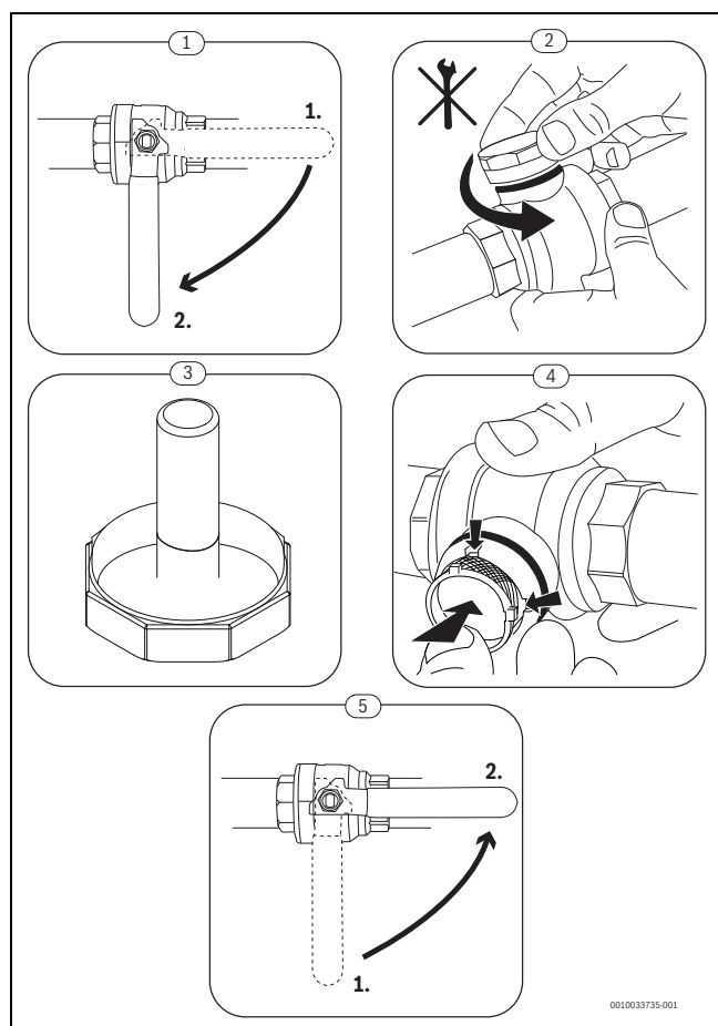
Bild 44 Siebreinigung
