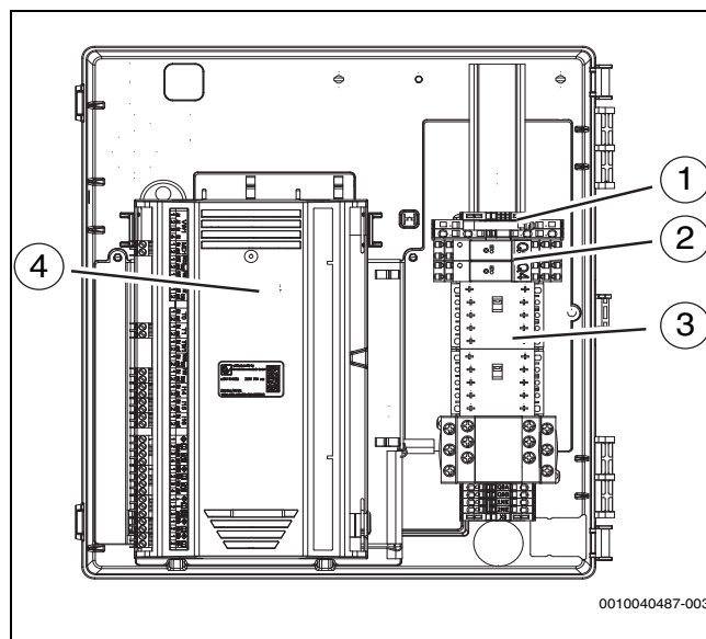
Bild 33 Anordnung der Komponenten im Klemmenkasten
