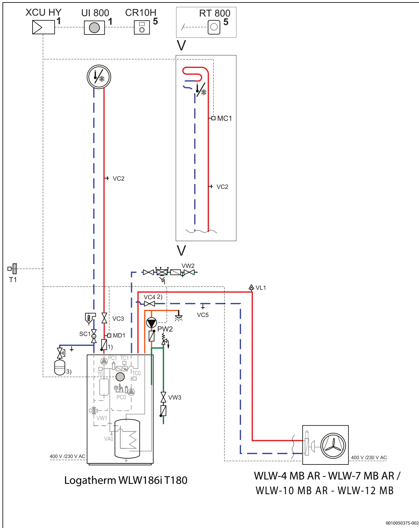
Bild 48 Tower Inneneinheit, Wärmepumpe (ODU) und ein ungemischter Heizkreis (für Deutschland, Österreich, Schweiz)
