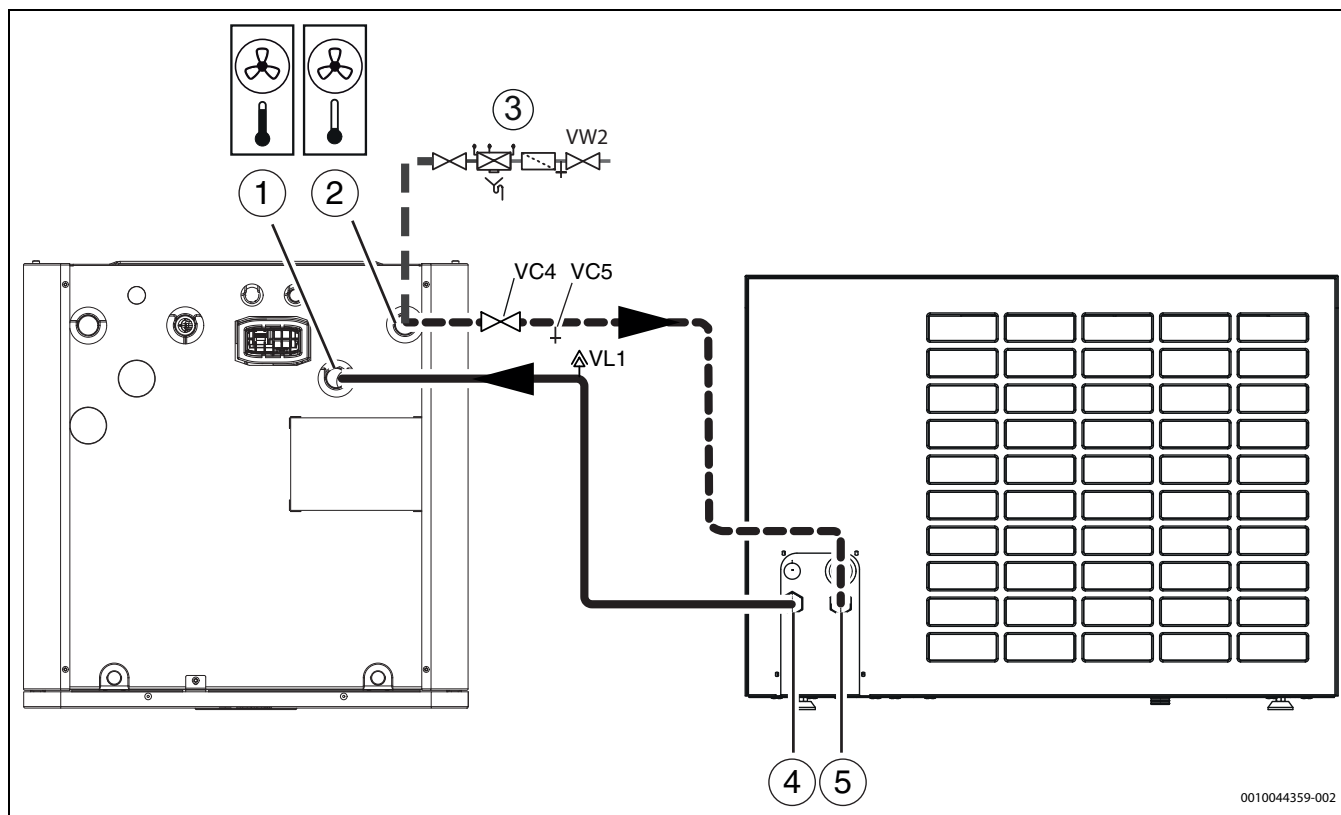
Bild 20 Inneneinheit an die Wärmepumpe anschließen
