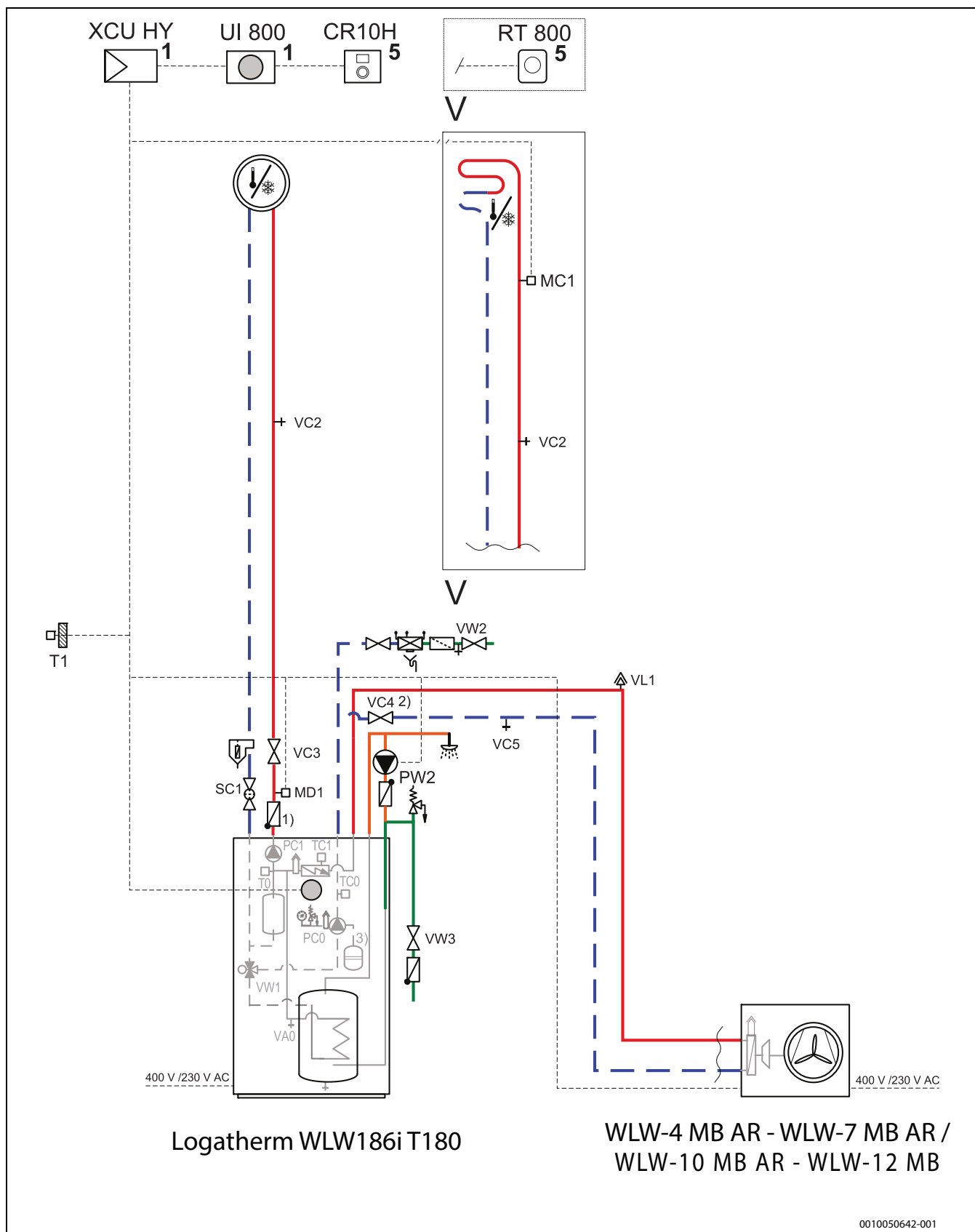
Bild 47 Tower Inneneinheit, Wärmepumpe (ODU), ein ungemischter Heizkreis (nur für Polen)
