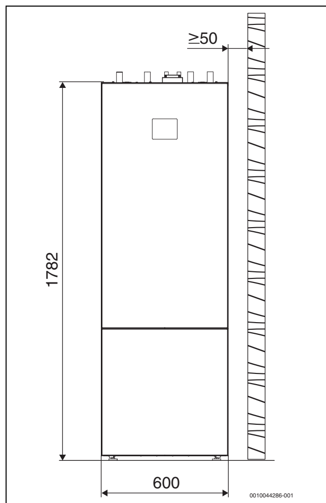
Bild 3 Abmessungen (mm)
