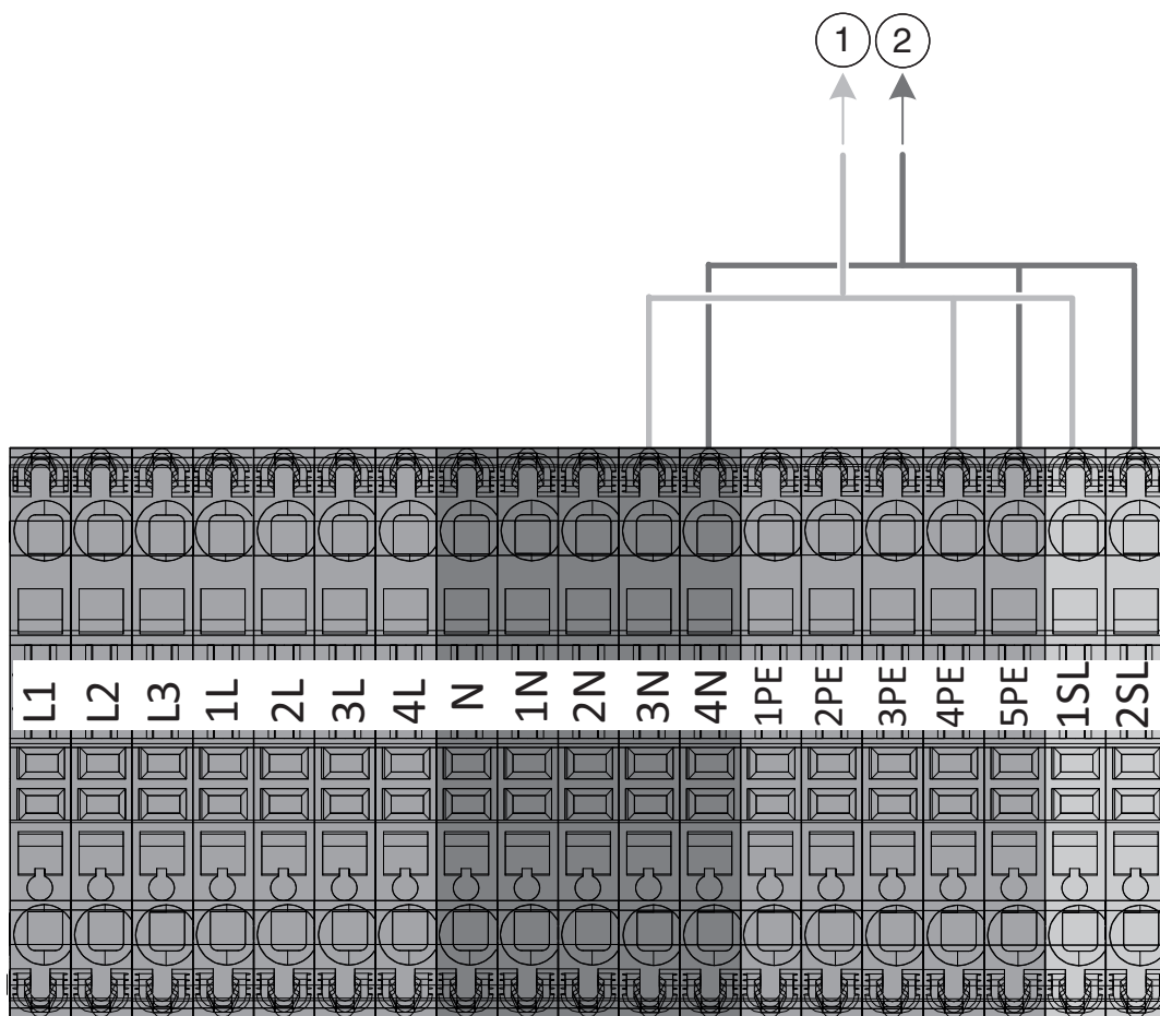
Bild 36 Elektrische Anschlüsse für Zubehör
