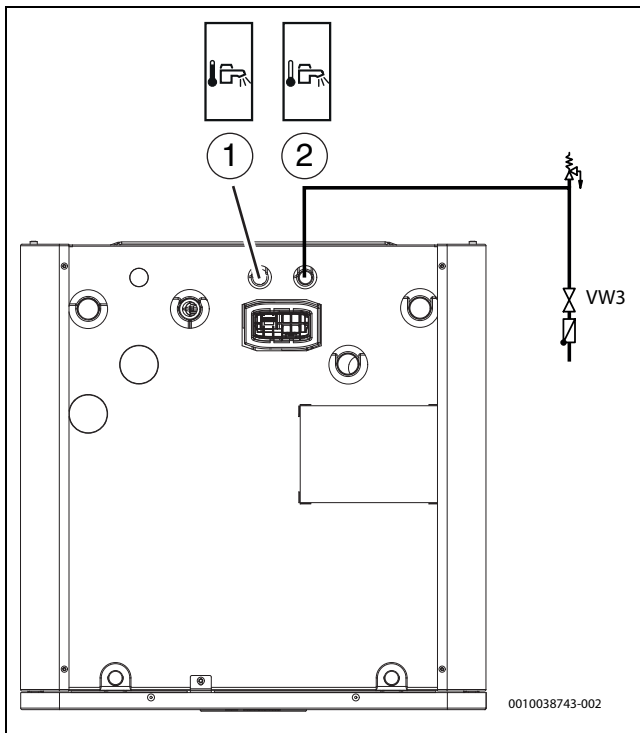
Bild 23 Warmepumpenanschlüsse Trinkwasser
