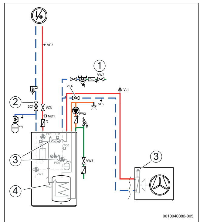
Bild 24 Inneneinheit, Wärmepumpe und Heizungsanlage
