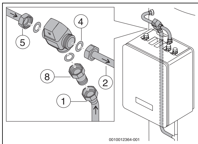
Bild 20 Anschlussrohr handfest verschrauben
