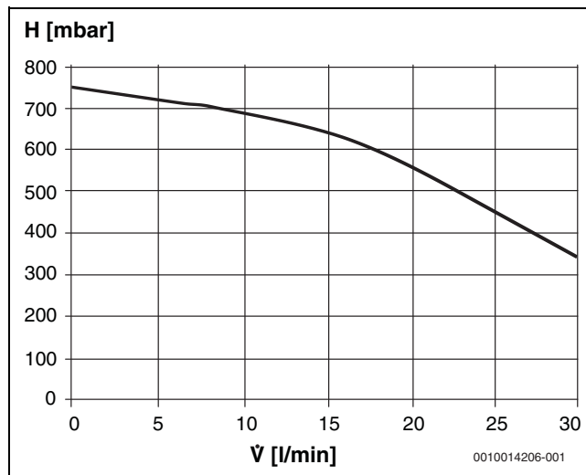
Bild 6 Restförderhöhe Primärkreispumpe
