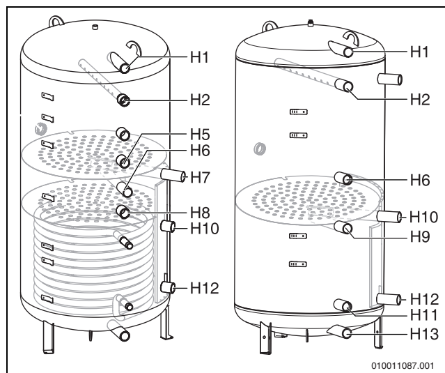
Bild 27 Pufferspeicher mit Trennblechen
