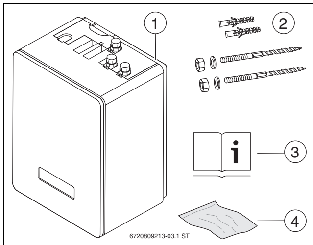
Bild 2 Lieferumfang Frischwasserstation
