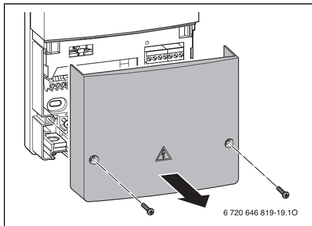
Bild 32 Modul öffnen
