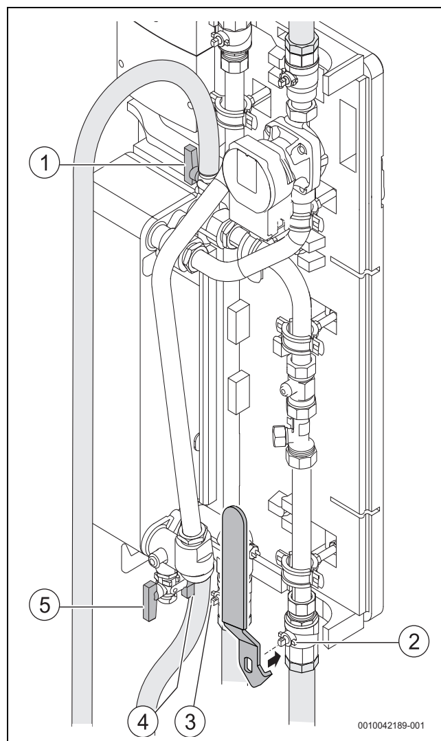
Bild 66 Wartung Frischwasserstation
