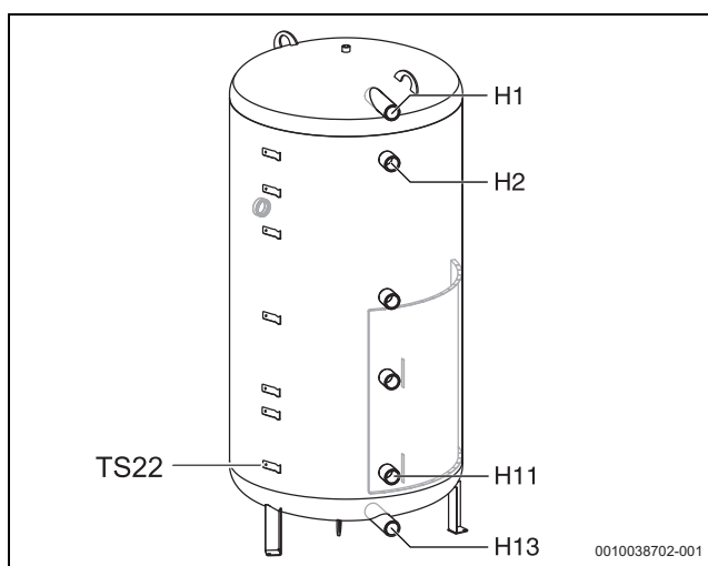
Bild 35 Pufferspeicher als Bereitschaftsspeicher (getrenntes Volumen), Hydraulik (→ Bild 6, Seite 6)
