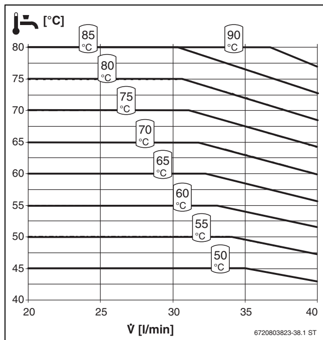
Bild 60 Temperaturverhalten Einzelstation FS40/3E
