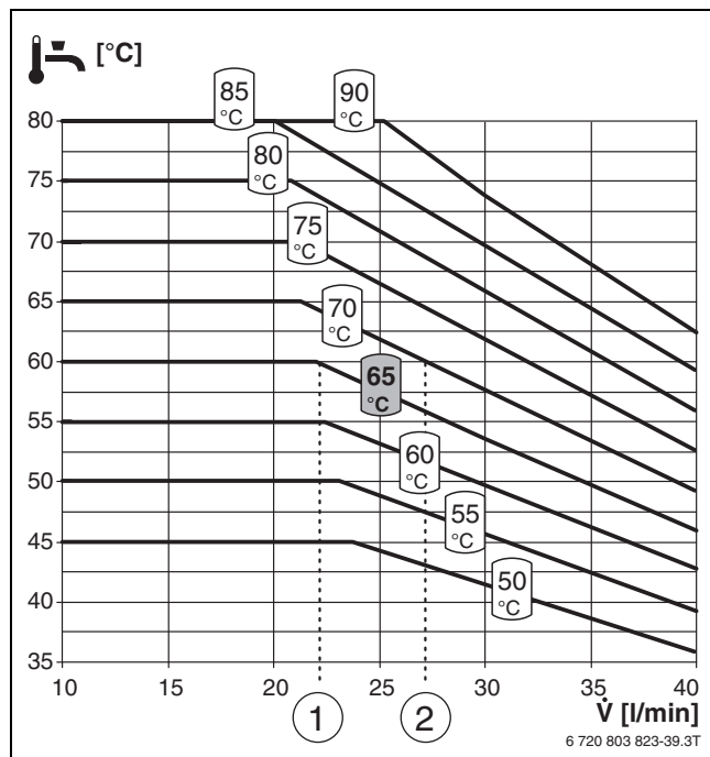
Bild 59 Temperaturverhalten Einzelstation FS27/3E
