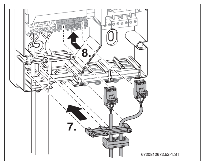
Bild 53 Anschlussklemmen in Modul montieren
