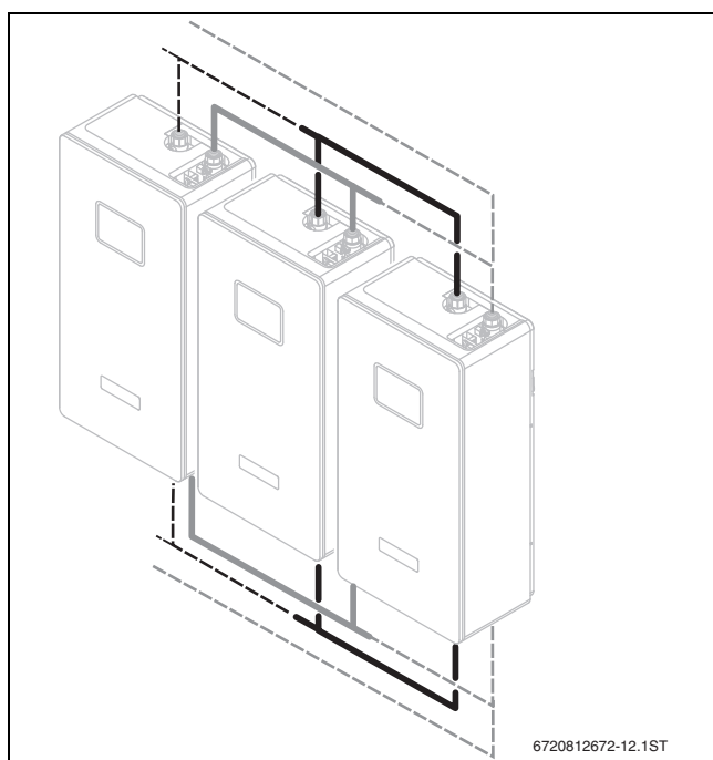
Bild 27 Beispiel: FS120/3E mit Verrohrungssatz (Tichelmann-Prinzip)
