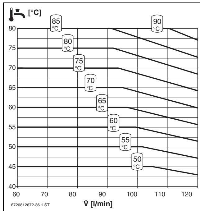
Bild 63 Temperaturverhalten Kaskade FS120/3E
