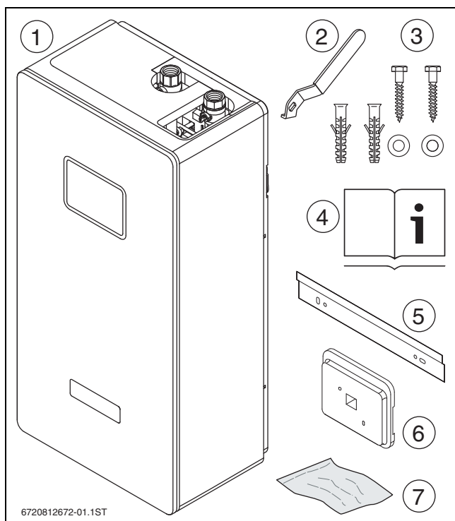
Bild 2 Lieferumfang Einzelstation
