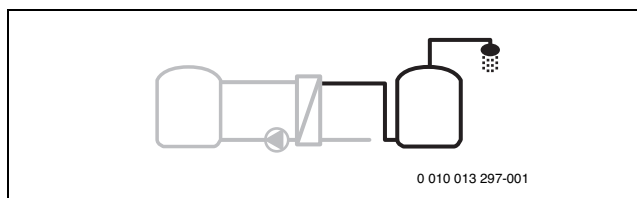
Bild 43 Vorwärm Frischwasserstation
