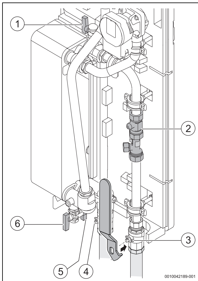
Bild 67 Volumenstromfühler wechseln
