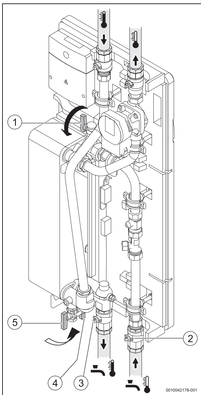
Bild 56 Spül- /Befüllvorrichtungen an der Einzelstation
