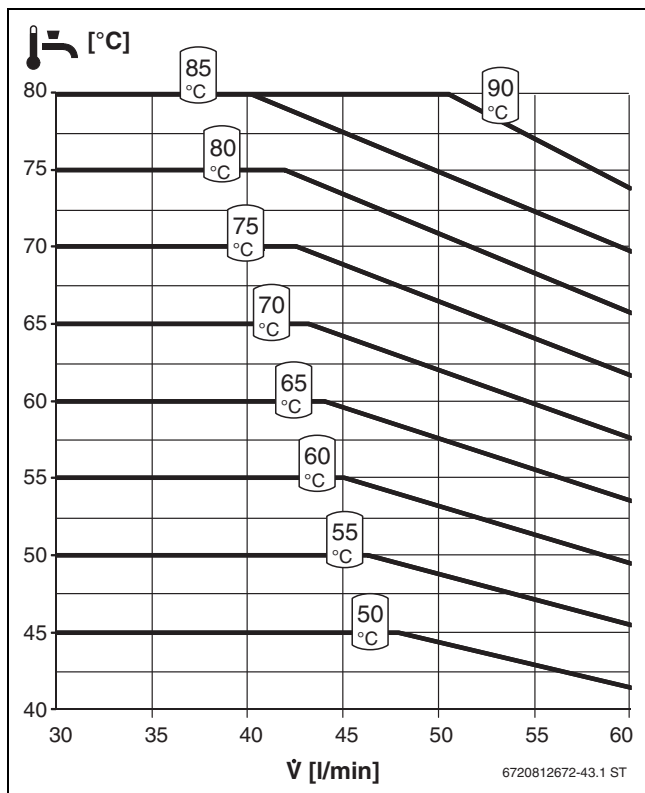
Bild 61 Temperaturverhalten Kaskade FS54/3E
