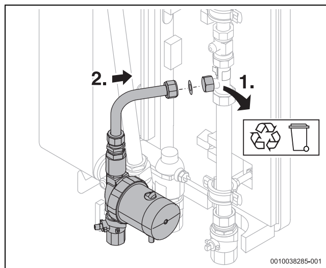
Bild 22 Zirkulationsstrang montieren
