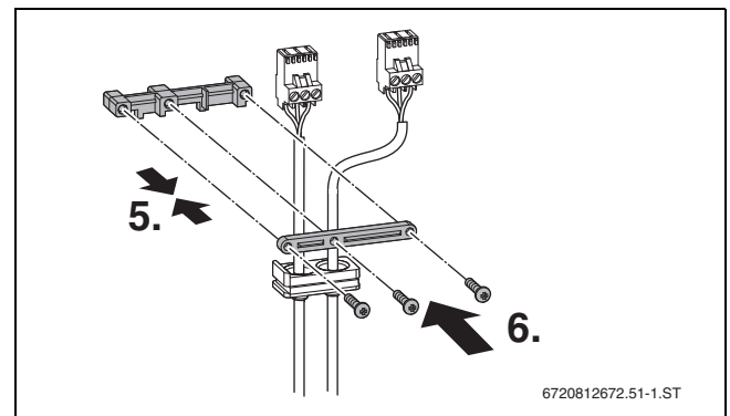
Bild 52 Zugentlastung montieren
