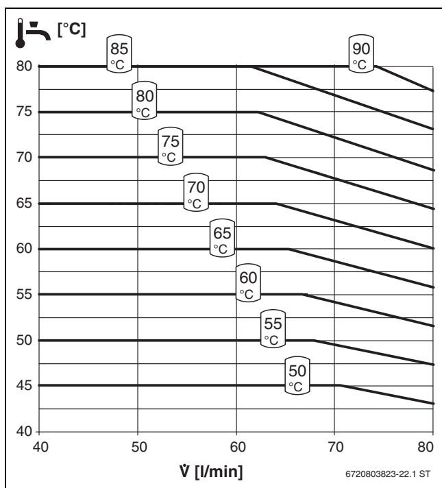
Bild 62 Temperaturverhalten Kaskade FS80/3E
