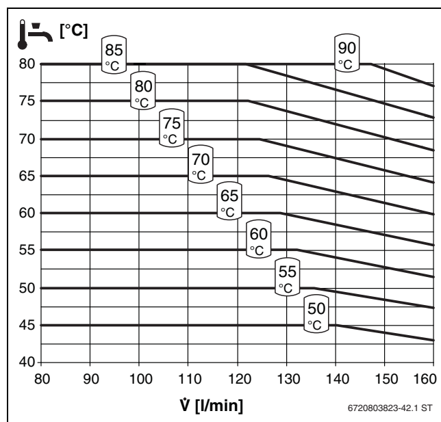
Bild 64 Temperaturverhalten Kaskade FS160S/3E
