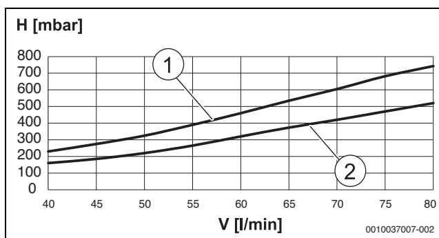
Bild 11 Druckverlust Sekundärseite Kaskade inkl. Verrohrungssatz und Kaskadenventil
