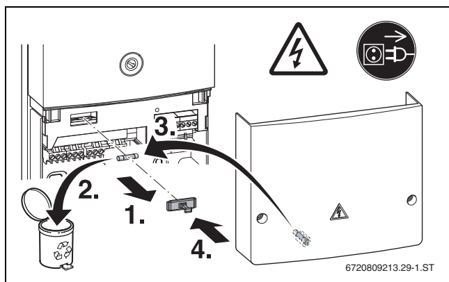
Bild 68 Sicherung tauschen
