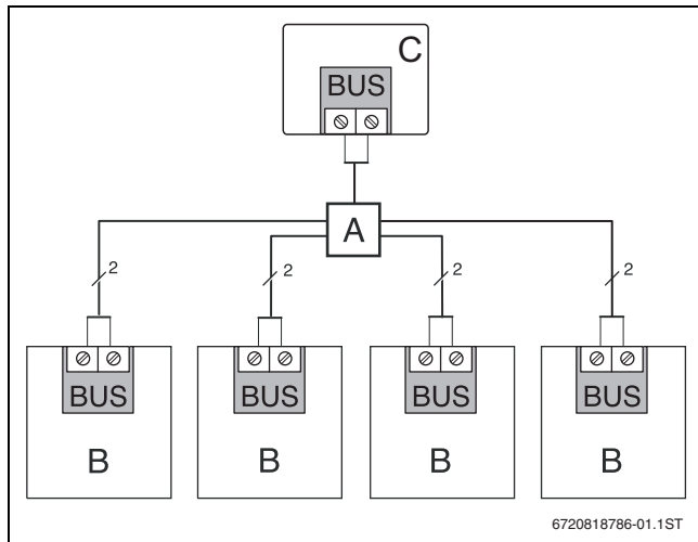
Bild 54 BUS-Leitungen anschließen
