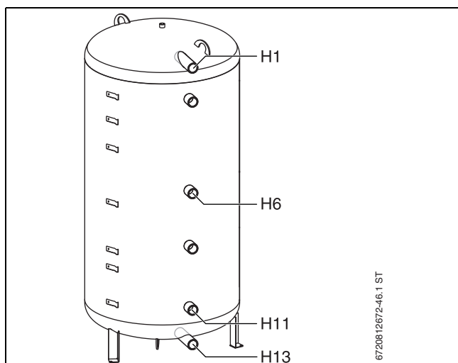
Bild 37 Pufferspeicher als Solarspeicher für Vorwärmesystem (auch mit internem Wärmetauscher möglich), Hydraulik (→ Bild 7, Seite 7)
