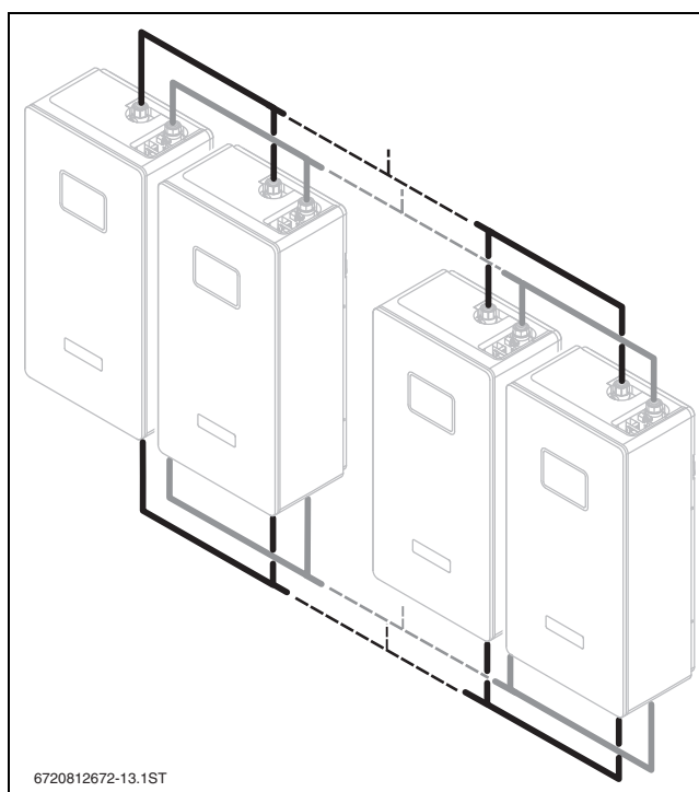
Bild 28 Beispiel: FS160S/3E mit 2 Verrohrungssätzen
