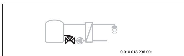
Bild 42 Ventil Rücklauf
