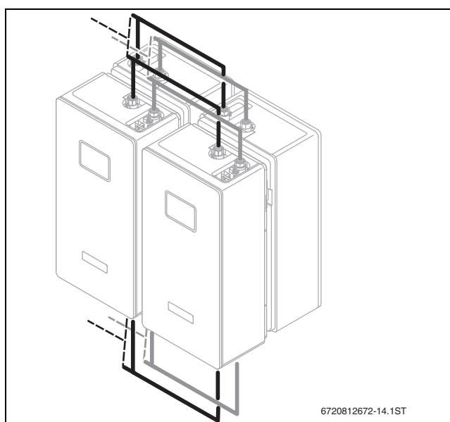
Bild 29 Beispiel: FS160S/3E mit 2 Verrohrungssätzen (alternativ: 4 Stationen bauseits in einer Reihe verbinden)
