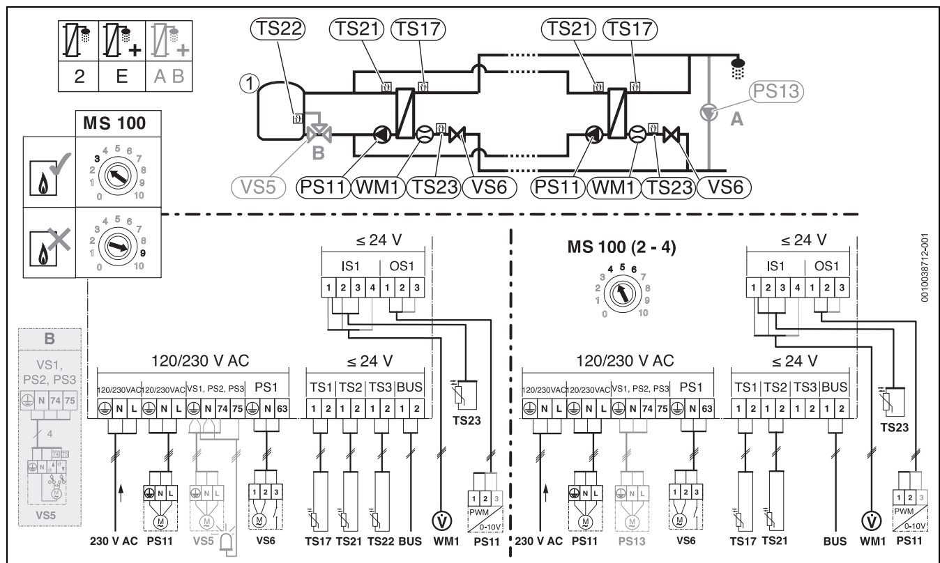
Bild 49 Anschlussklemmen bei Frischwasserstation Kaskade
