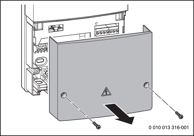
Bild 46 Modul öffnen
