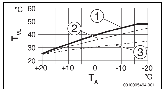
Bild 9 Einstellung der Heizkurve für Fußbodenheizung Steigung über Auslegungstemperatur T_{\text{AL}} und minimale Außentemperatur T_{\text{A,min}}
