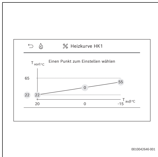
Bild 5 Startmenü Heizkurve
