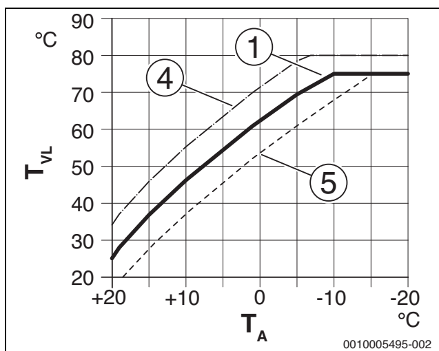
Bild 12 Einstellung der Heizkurve für Heizkörper Parallelverschiebung über Raumtemperatur-Offset oder gewünschte Raumtemperatur
