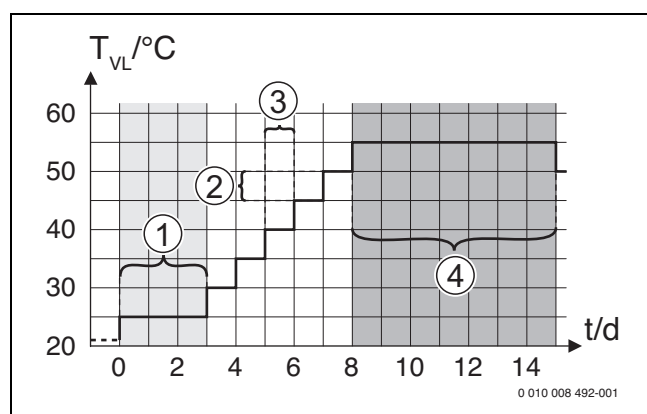
Bild 13 Ablauf der Estrich Trocknung mit den Grundeinstellungen in der Aufheizphase
