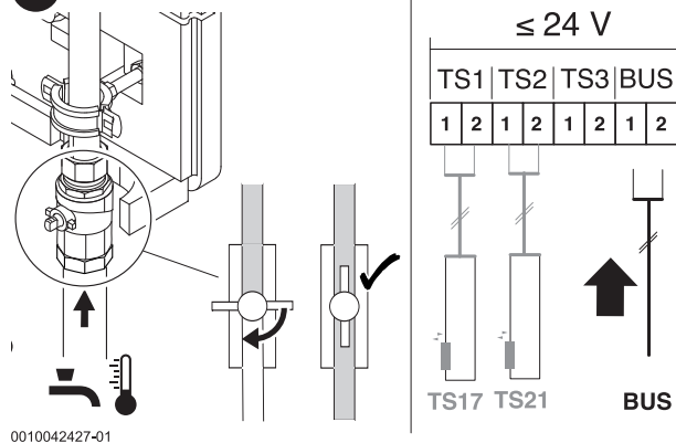
Rys. 13 Otworzyć wszystkie zawory odcinające wody zimnej i podłączyć wszystkie przewody magistrali BUS. Dźwignię zaworów kaskady z powrotem przesunąć w lewo.
