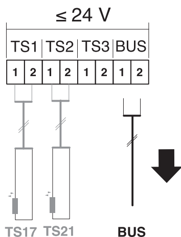
Rys. 8 Ponowne odłączanie przewodu magistrali BUS
