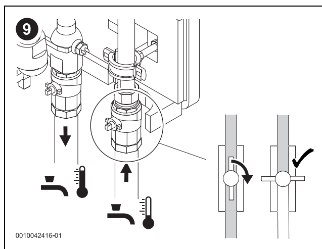
Afb. 9 Sluit de afsluiting koud water
