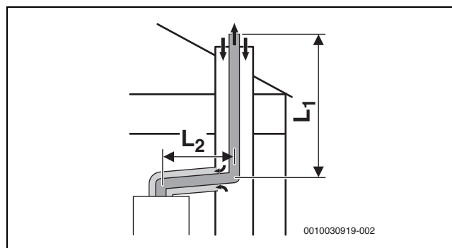
Bild 44 Starre Abgasführung nach C 93x im Schacht und konzentrische Luft-Abgas-Führung im Aufstellraum
