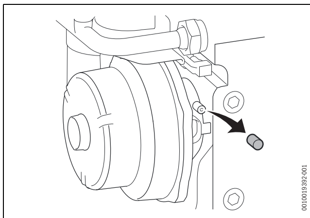
Bild 81 Messstutzen an der Mischeinrichtung
