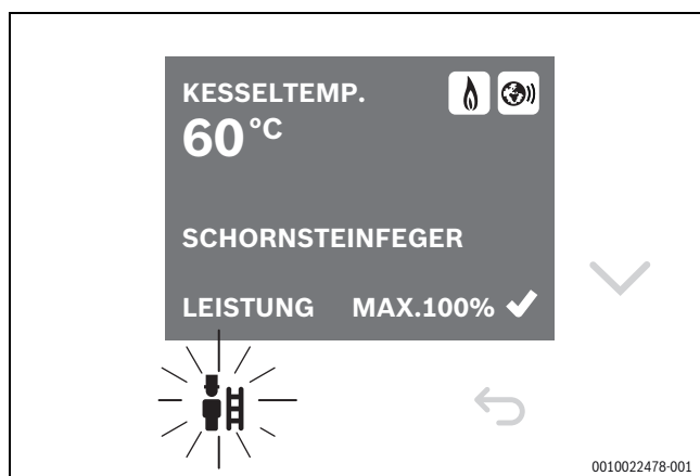
Bild 68 Menü Schornsteinfegerbetrieb
