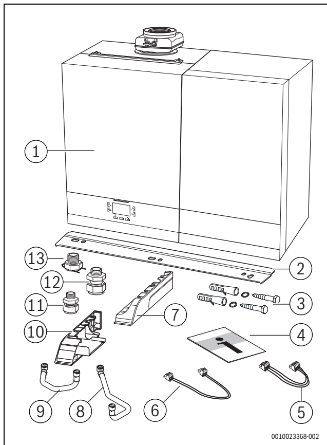
Bild 2 Lieferumfang
