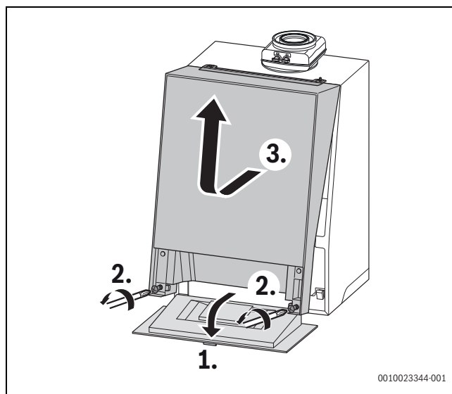
Bild 17 Verkleidung Gerät demontieren
