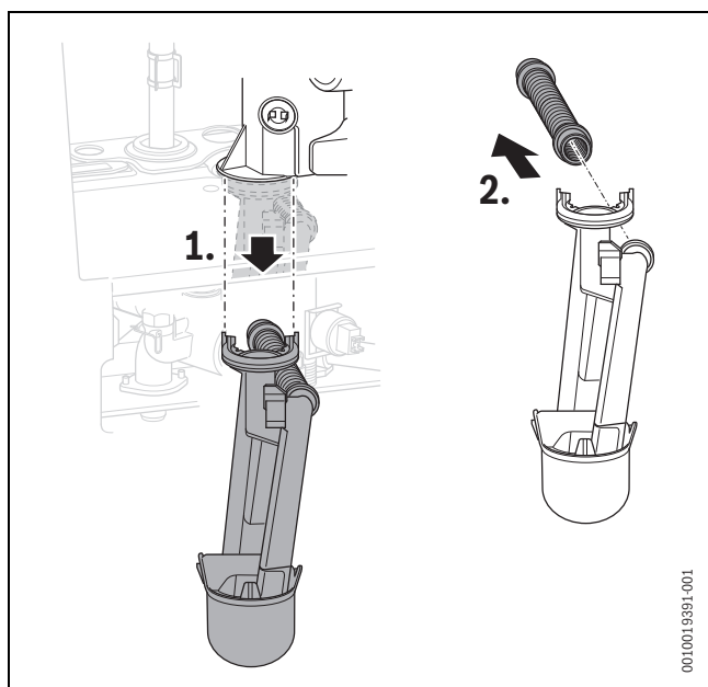
Bild 80 Kondensatsiphon
