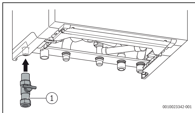
Bild 16 Gasanschluss herstellen
