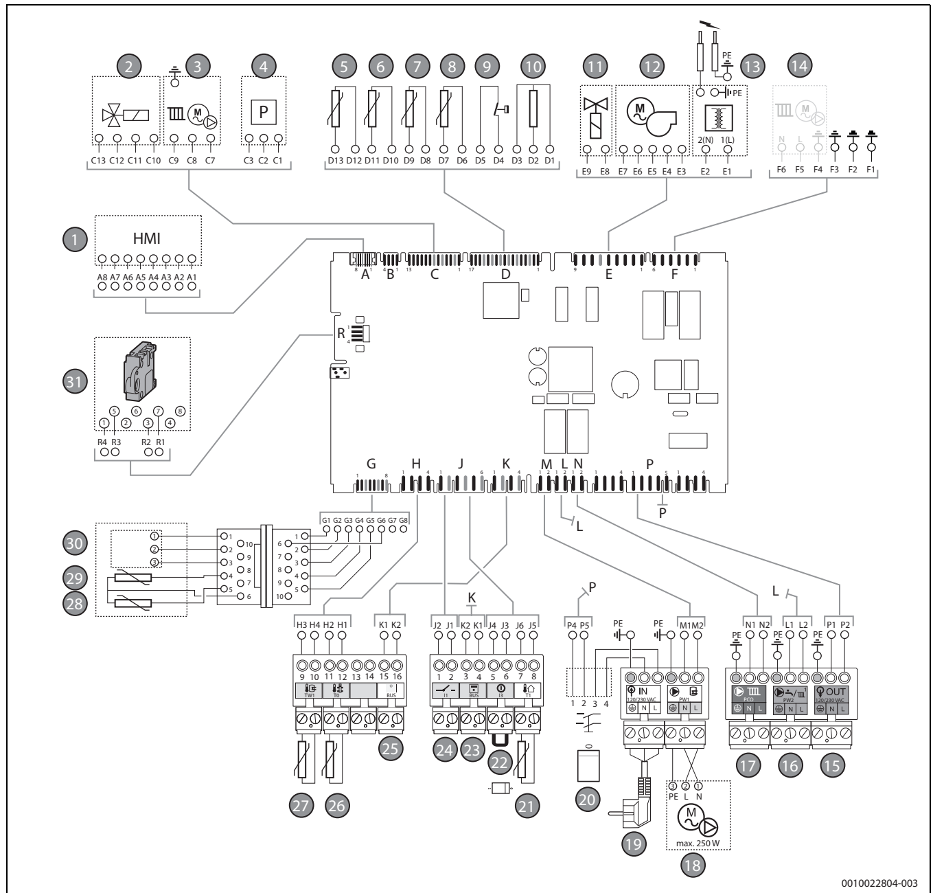
Bild 6 Anschlussplan
