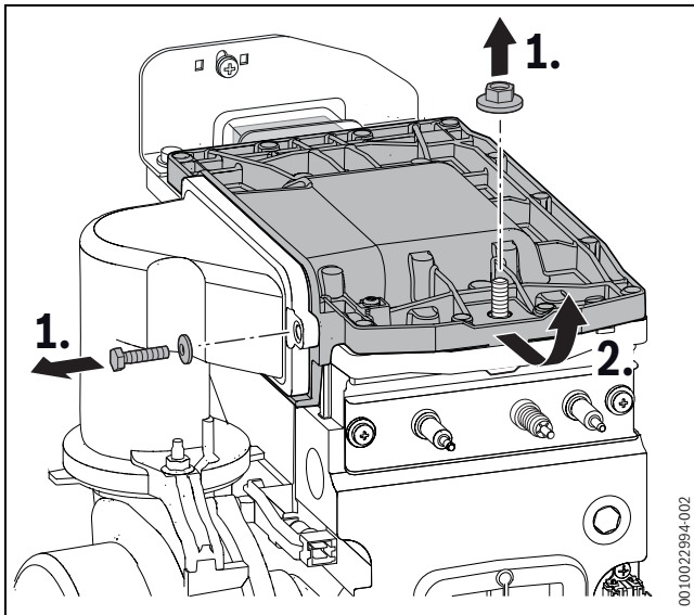
Bild 76 Brennerdeckel ausbauen
