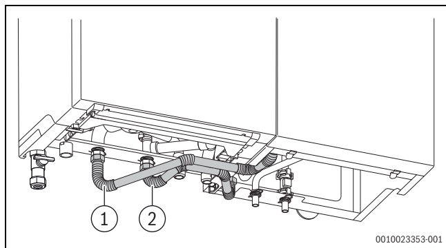
Bild 20 Warmwasserspeicher und Gerät verbinden
