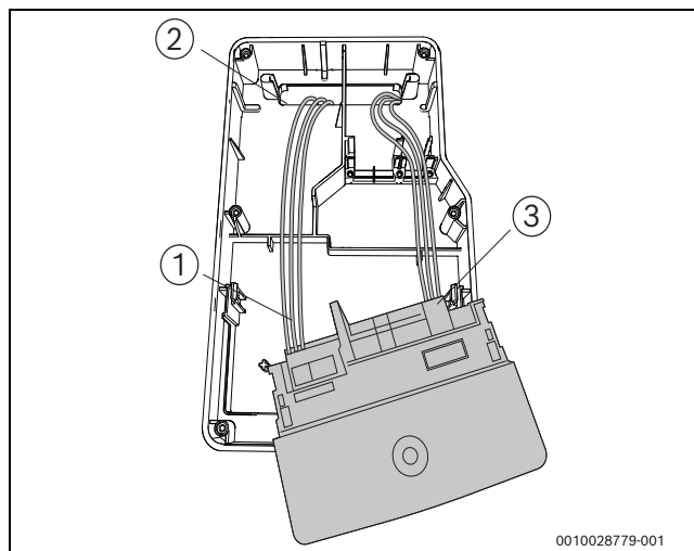
Bild 56 Funktionsmodul anschließen
