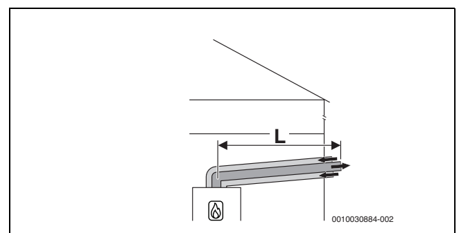
Bild 37 Horizontale konzentrische Luft-Abgas-Führung nach C 13x durch die Außenwand
