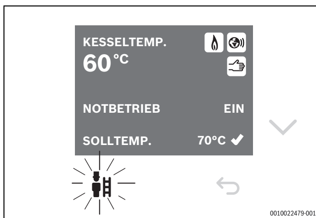
Bild 69 Menü Notbetrieb
