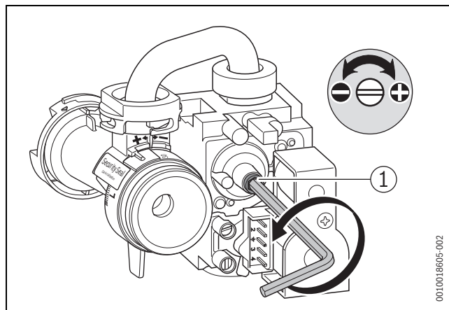
Bild 64 Plombe entfernen
