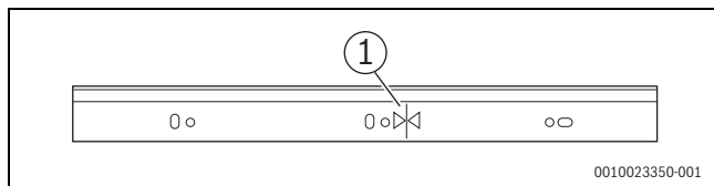
Bild 15 Markierung zum Positionieren des Warmwasserspeichers
