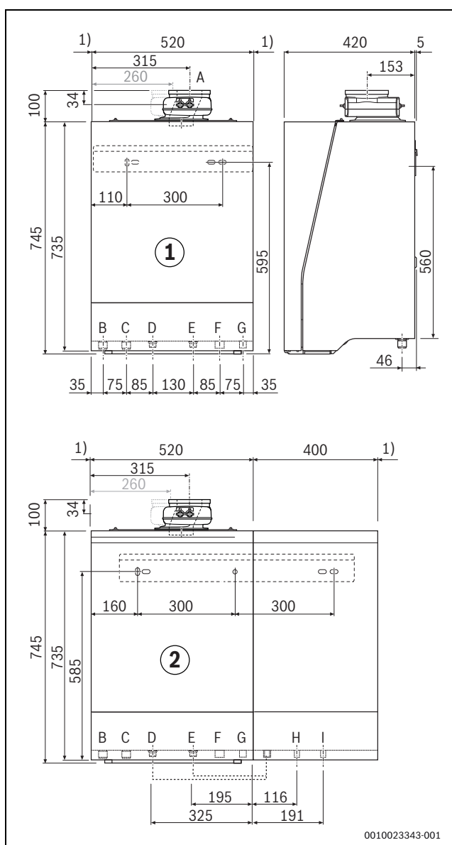
Bild 5 Abmessungen und Anschlüsse [mm]
