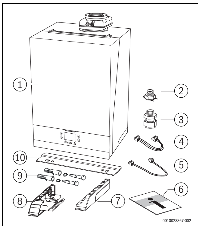
Bild 1 Lieferumfang
