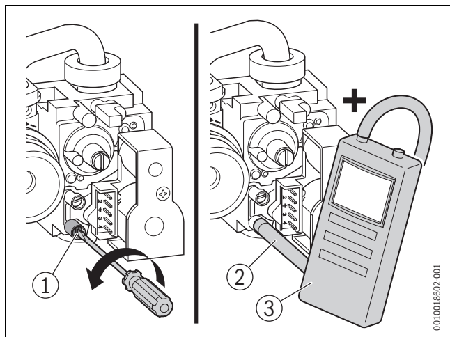
Bild 61 Gas-Anschlussdruck messen
