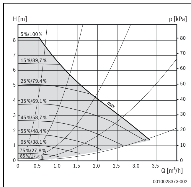
Bild 277 Pumpenkennfelder und Pumpenkennlinien der Solarpumpe Para ST 15/7-50/iPWM 2, Drehzahlbereich 20–100 %, Volumenstrombereich 0–16,5 l/min
