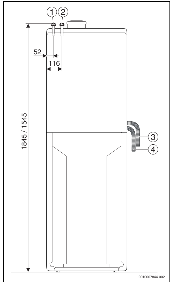
Bild 13 Anschlussmaße des Zubehörs Anschluss-Set Heizungsunterstützung HU (Maße in mm)
