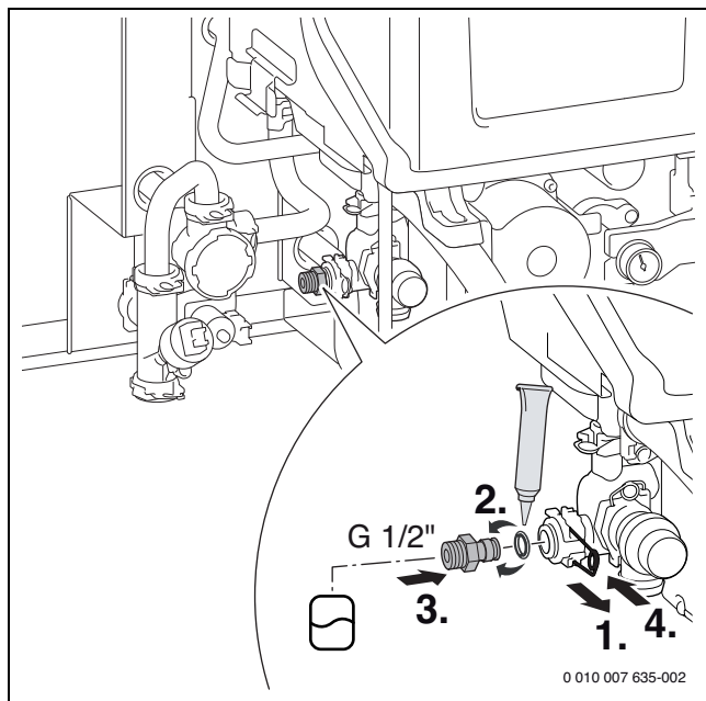
Bild 117 Verbindungsstück für den bauseitigen Anschluss eines externen Ausdehnungsgefäßes montieren
