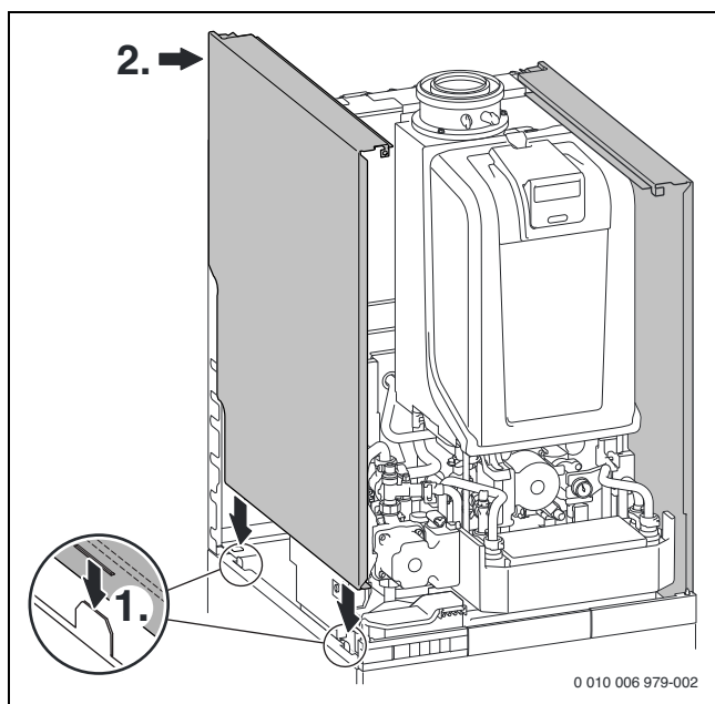
Bild 239 Rechte und linke Verkleidung montieren
