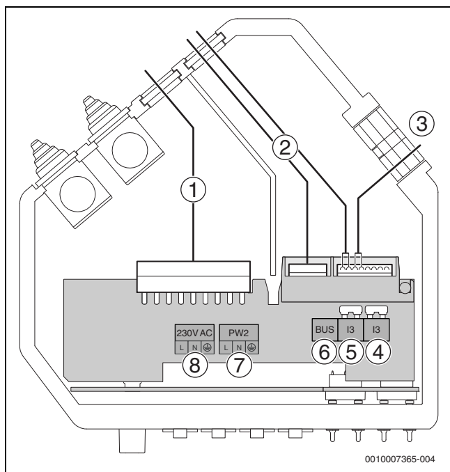
Bild 229 Anschlussbox
