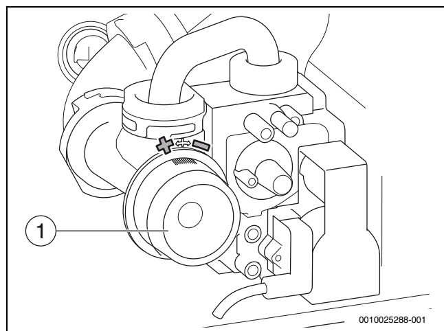
Bild 248 Gas-Luft-Verhältnis einstellen
