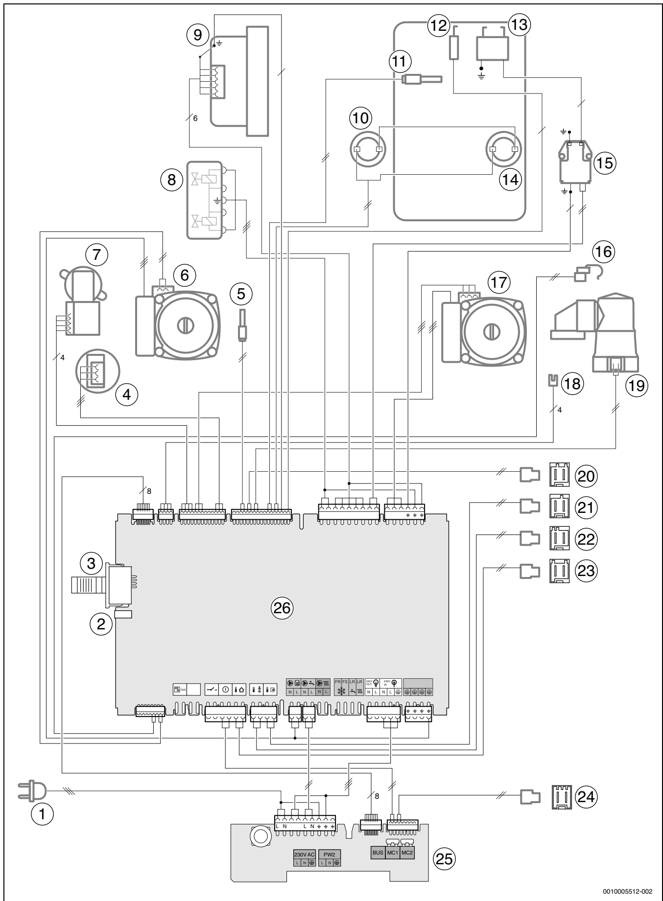
Bild 275 Elektrische Verdrahtung
