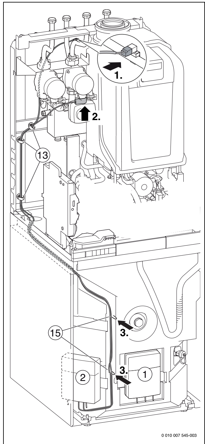
Bild 143 GB.192-..iT100-.-Geräte: Anschluss Heizungspumpe gemischter Heizkreis und Temperaturfühler
