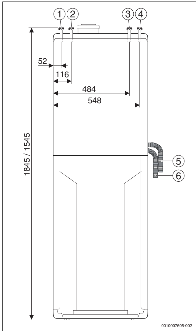
Bild 15 Anschlussmaße des Zubehörs Anschluss-Set solare Heizungsunterstützung SHU (Maße in mm)
