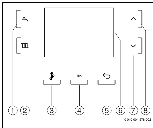
Bild 244 Bedienfeld
