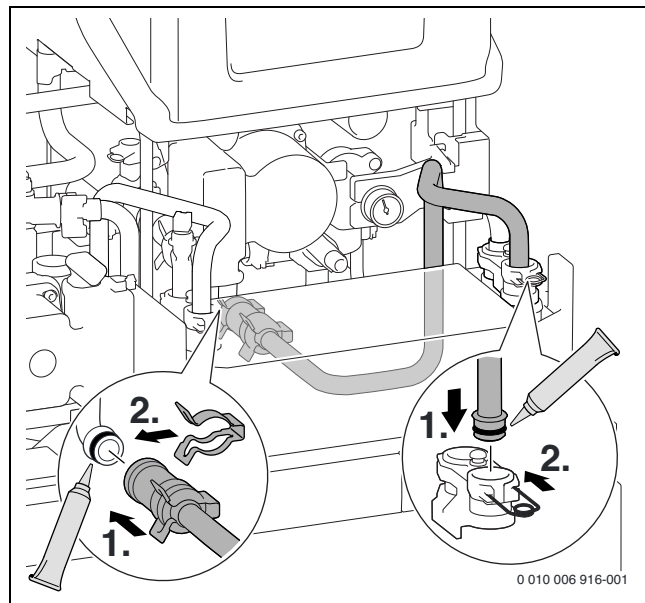
Bild 62 Rohrverbindung zwischen Plattenwärmetauscher und Wärmeblock erstellen (Rücklauf)
