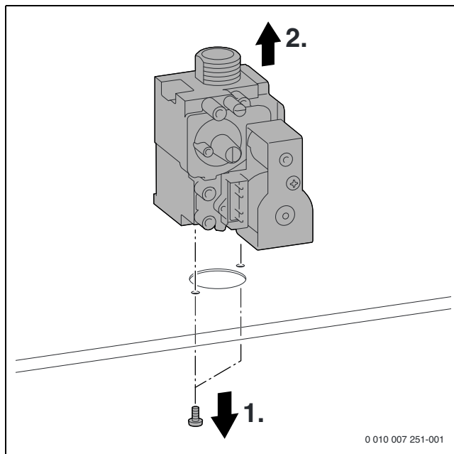
Bild 270 Gasarmatur ausbauen
