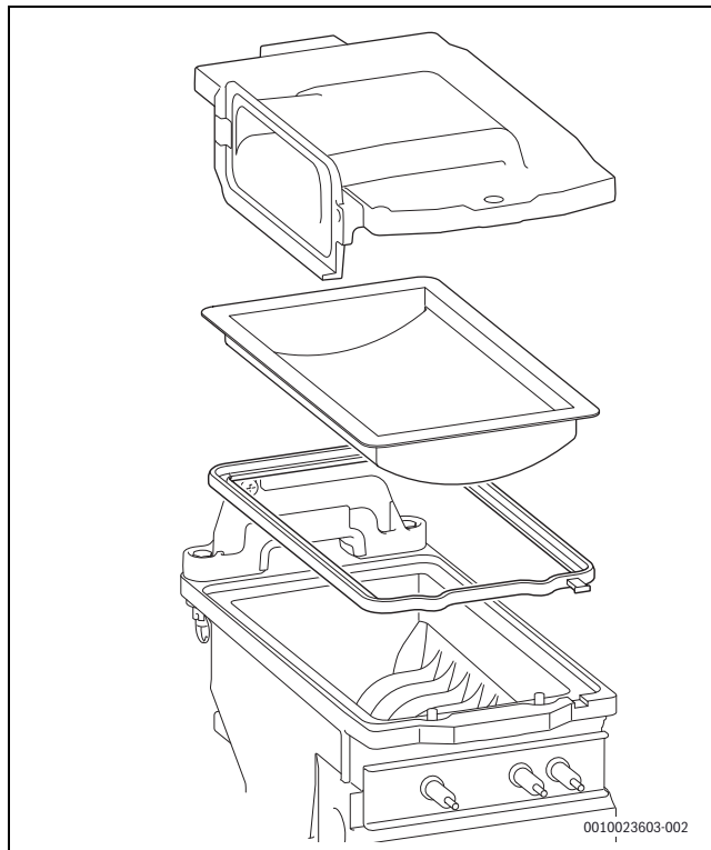
Bild 256 Brenner
