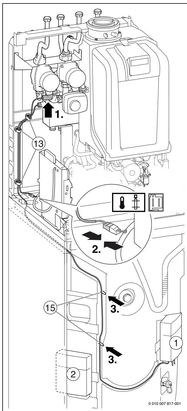
Bild 140 GB.192-..iT150-.-Geräte: Anschluss Heizungspumpe ungemischter Heizkreis und Hydraulische Weiche
