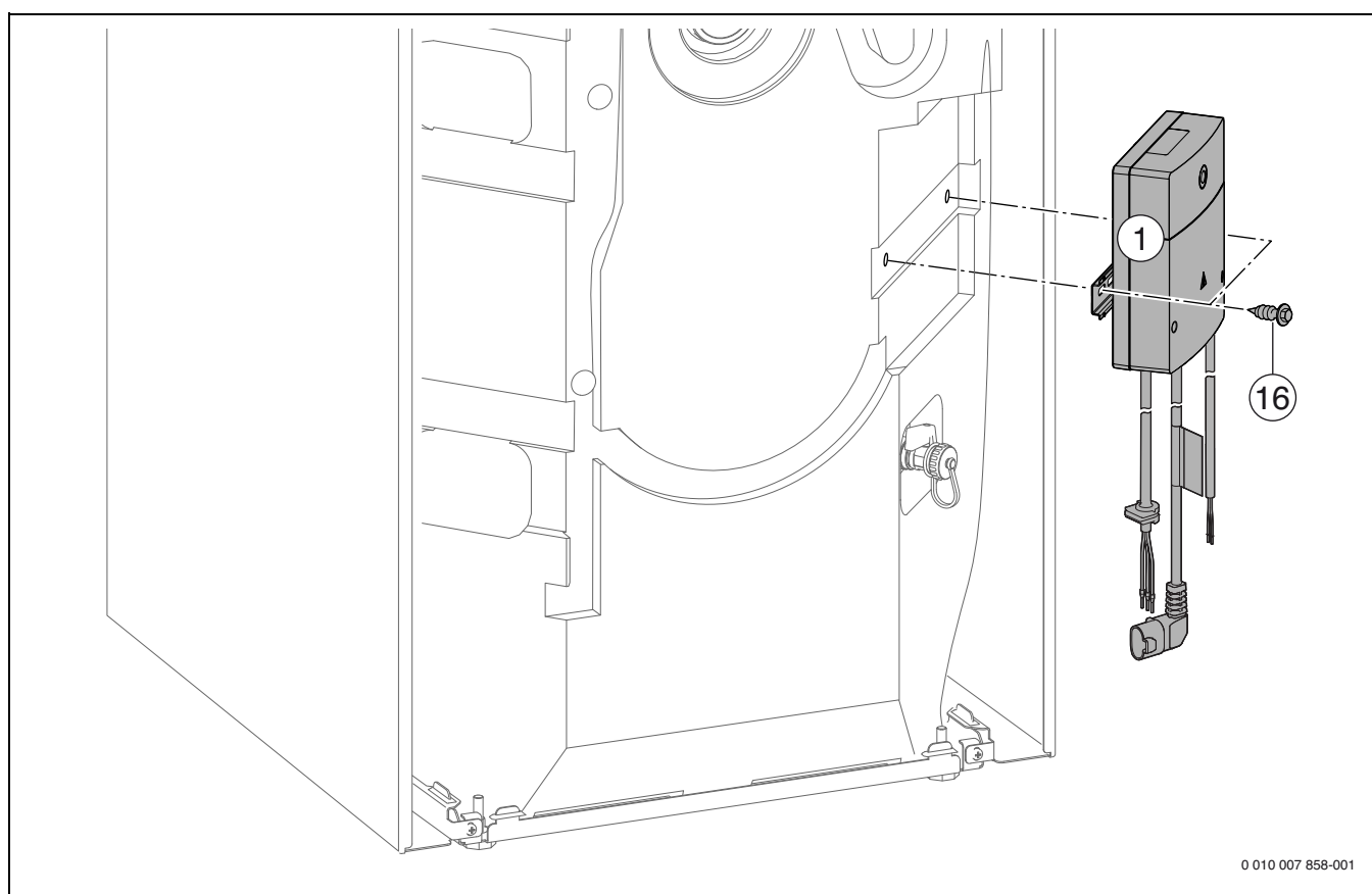
Bild 110 GB.192...iT150...Geräte
