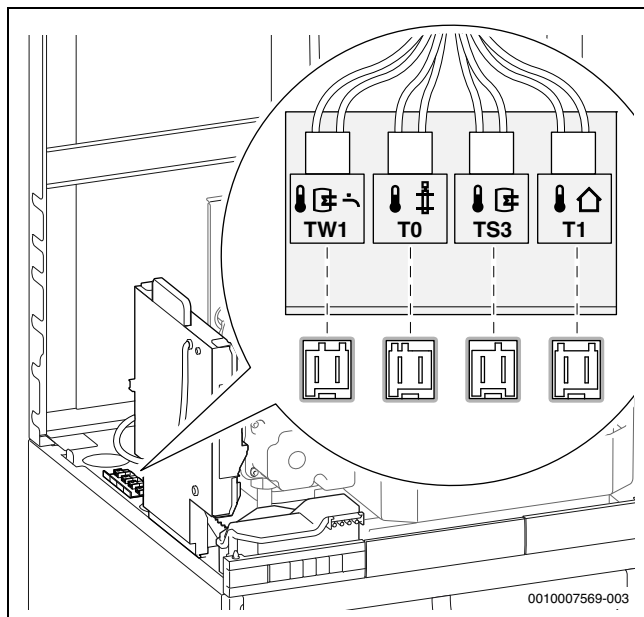
Bild 231 Stecker am Steuergerät
