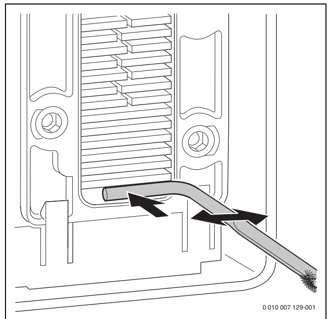
Bild 261 Kondensatwanne reinigen
