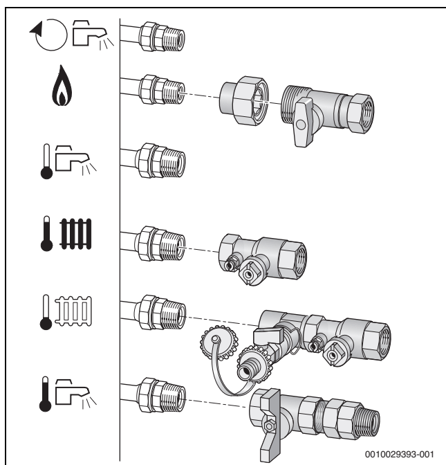
Bild 50 Montage des Armaturen-Sets am Beispiel Anschlüsse nach rechts AS-H1/Horizontales Anschluss-Set
