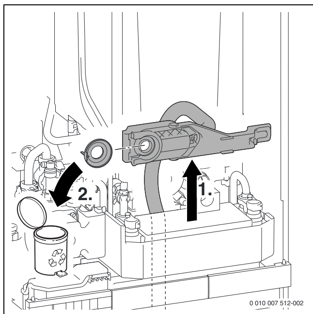
Bild 57 Schmutzfänger aus der Wartungsposition abnehmen und Schutzdeckel abnehmen
