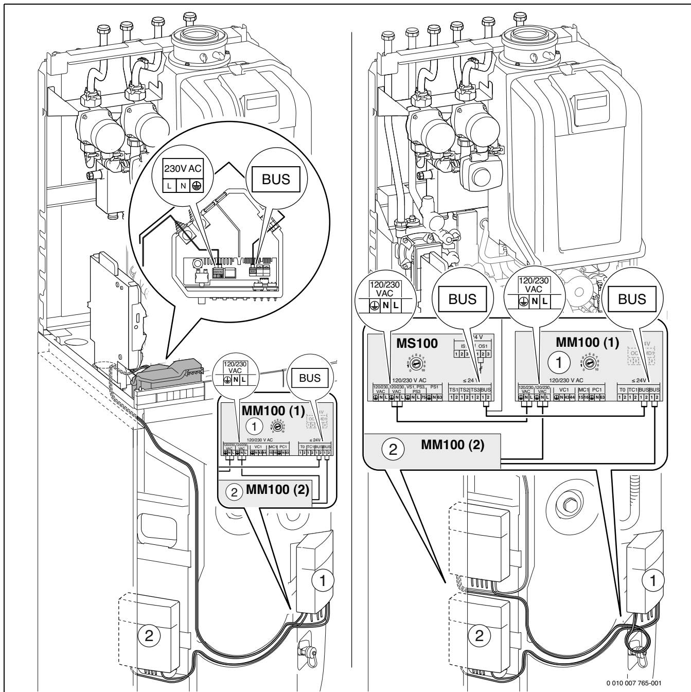
Bild 148 GB.192...iT150...-Geräte: Anschluss ohne Modul MS100 (links) und mit Modul MS100 (rechts) durchschleifen
