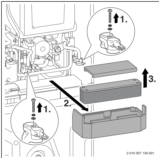
Bild 266 Plattenwärmetauscher ausbauen
