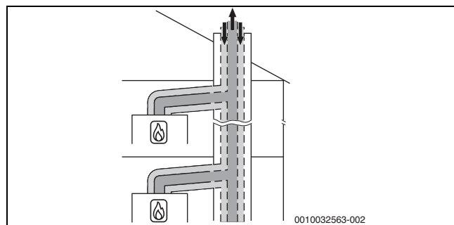
Bild 39 Mehrfachbelegung nach C_{(10)3x} mit konzentrischer Luft-Abgas-Führung im Aufstellraum
