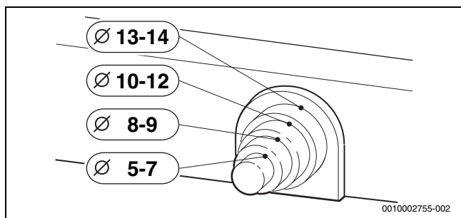
Bild 228 Zugentlastung an Kabeldurchmesser anpassen
