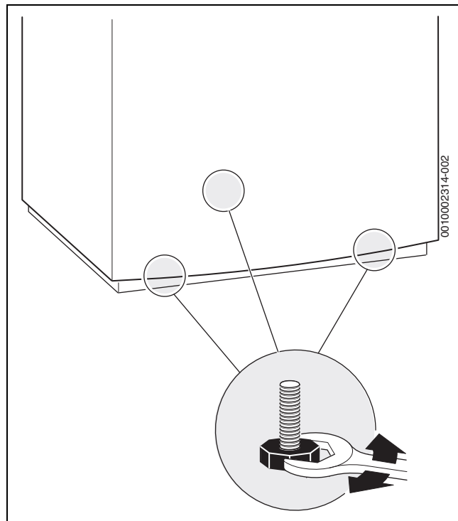
Bild 54 Speicher ausrichten
