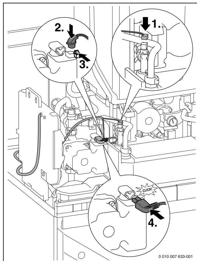
Bild 66 Speicherladepumpe und Warmwasser-Temperaturfühler anschließen
