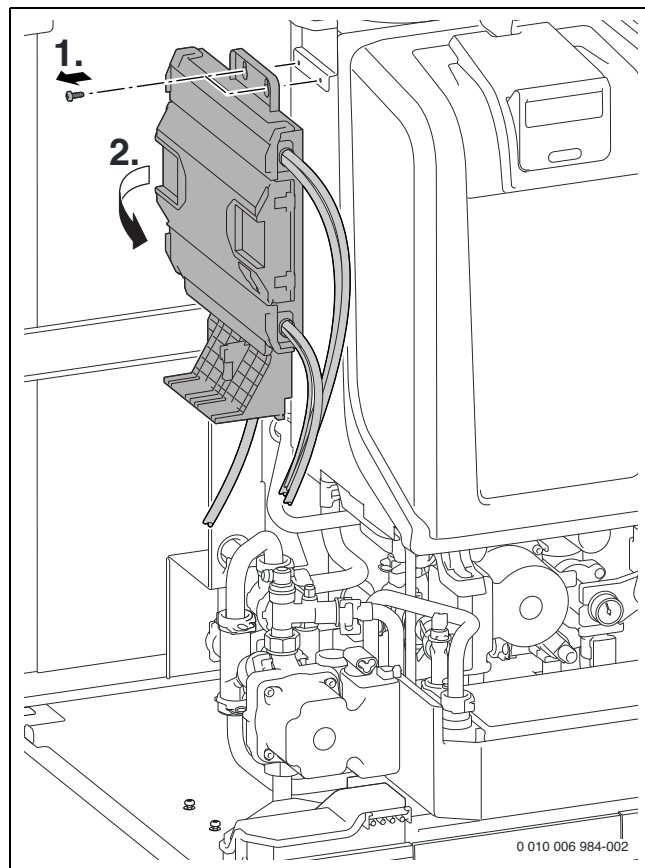
Bild 63 Steuergerät abnehmen
