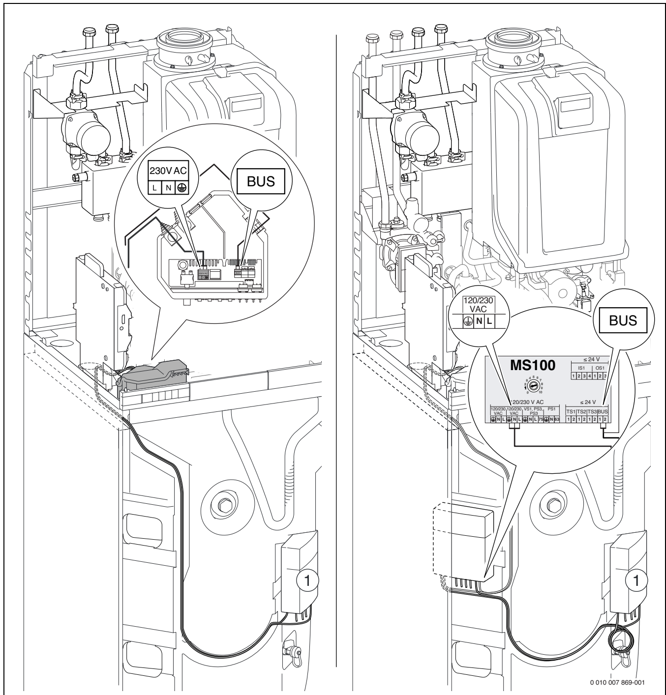
Bild 114 GB.192-..iT150-.-Geräte: Anschluss ohne Modul MS100 (links) und mit Modul MS100 (rechts)
