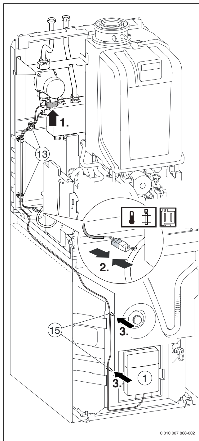
Bild 113 GB.192-..iT100-.-Geräte: Anschluss Heizungspumpe ungemischter Heizkreis und Hydraulische Weiche
