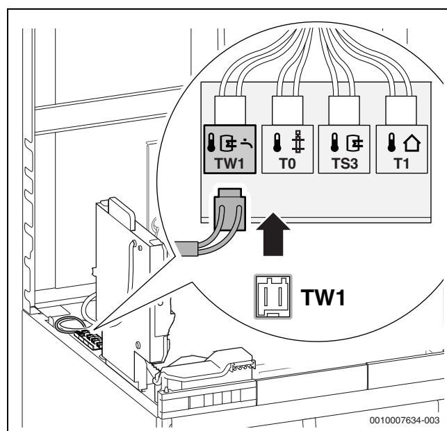
Bild 67 Speichertemperaturfühler anschließen
