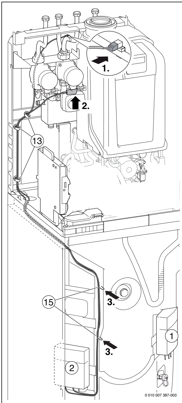
Bild 142 GB.192-..iT150-.-Geräte: Anschluss Heizungspumpe gemischter Heizkreis und Temperaturfühler
