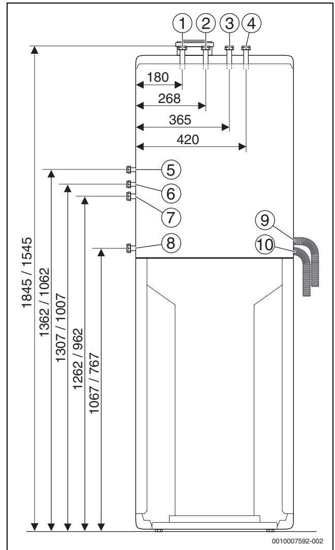
Bild 11 Anschlussmaße des Zubehörs Heizkreiserweiterung 2 (Maße in mm)
