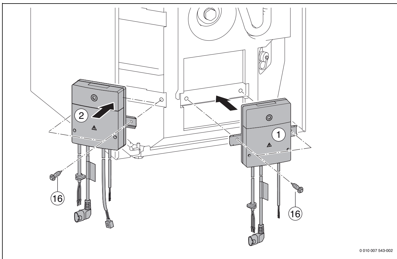
Bild 139 GB.192-..iT100-.-Geräte
