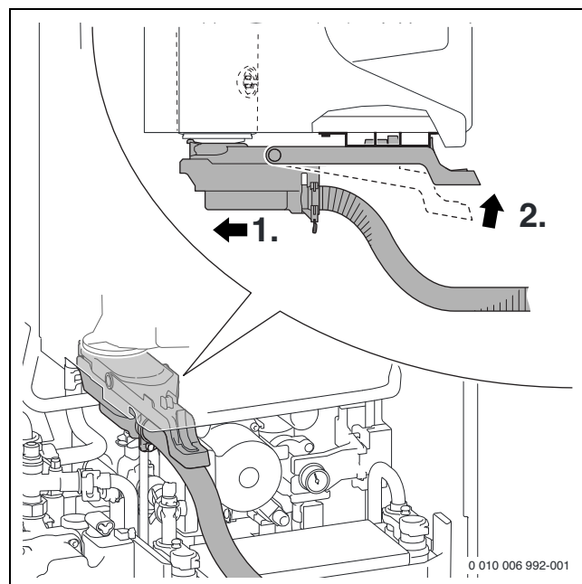
Bild 58 Schmutzfänger montieren
