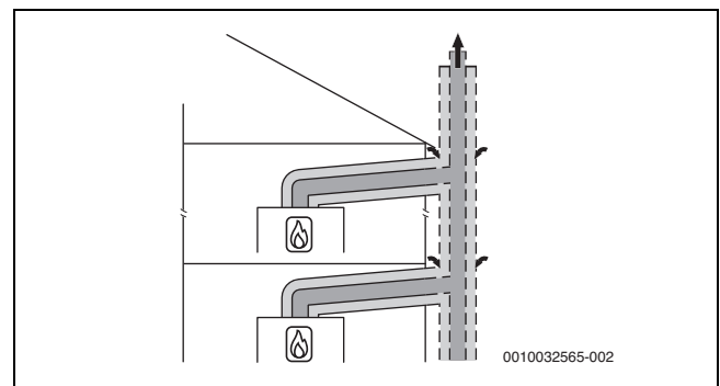
Bild 40 Mehrfachbelegung nach C_{(12)3x} mit konzentrischer Luft-Abgas-Führung im Aufstellraum
