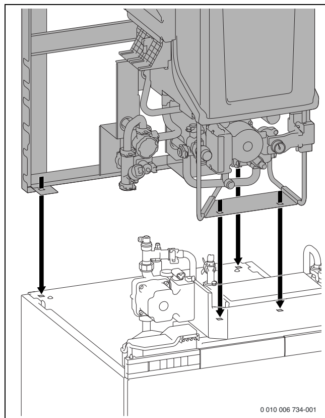
Bild 55 Gerät auf dem Speicher aufsetzen
