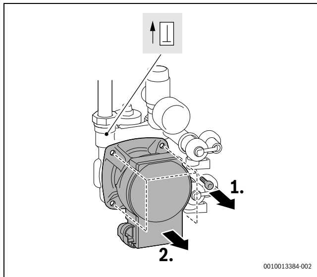
Bild 271 Solarpumpe ausbauen
