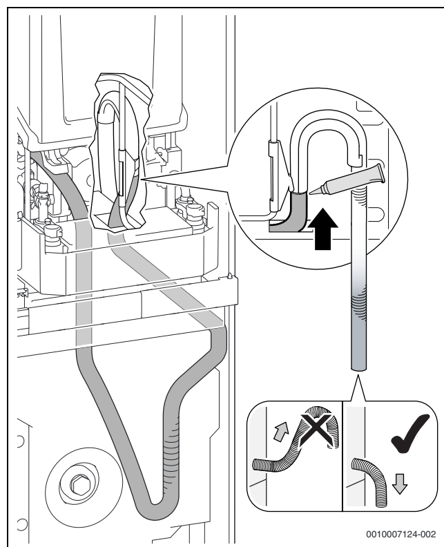
Bild 59 Siphonschlauch am Endstück einstecken
