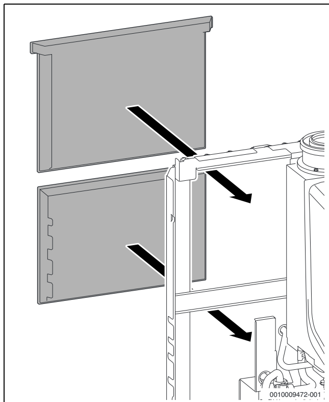
Bild 238 Wärmedämmungen an der Rückseite montieren
