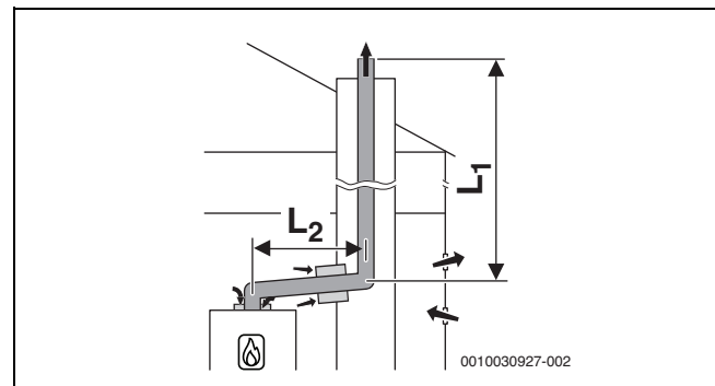
Bild 35 Starre Abgasführung im Schacht nach B 23p /B 53p mit raumluftabhängiger Luftzufuhr am Gerät und konzentrischem Verbindungsstück zwischen Aufstellraum und Schacht
