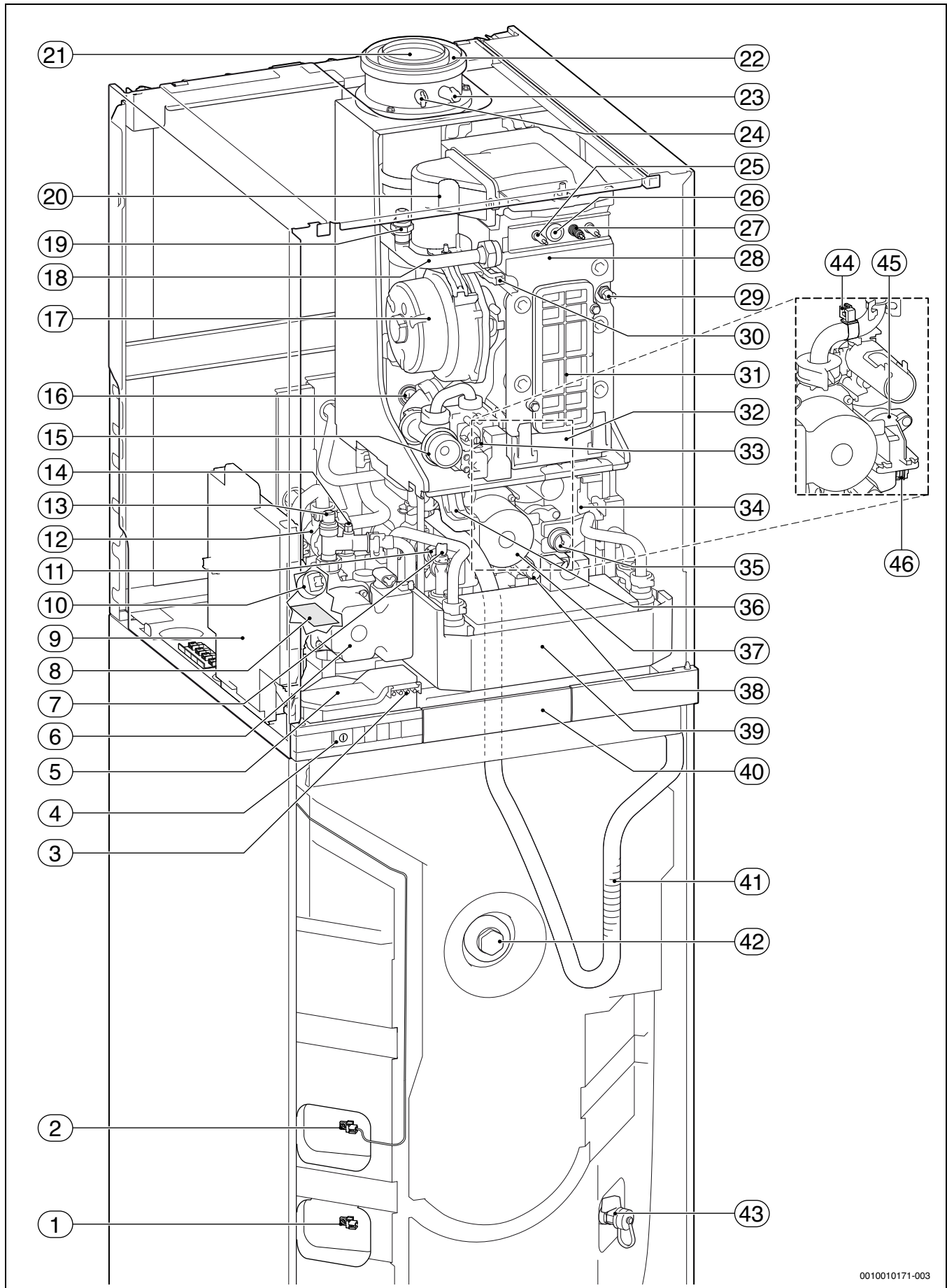
Bild 18 GB.192... iT150...-Geräte
