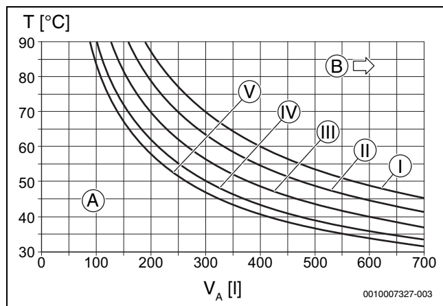
Bild 47 Kennlinien des Ausdehnungsgefäßes 17 I
