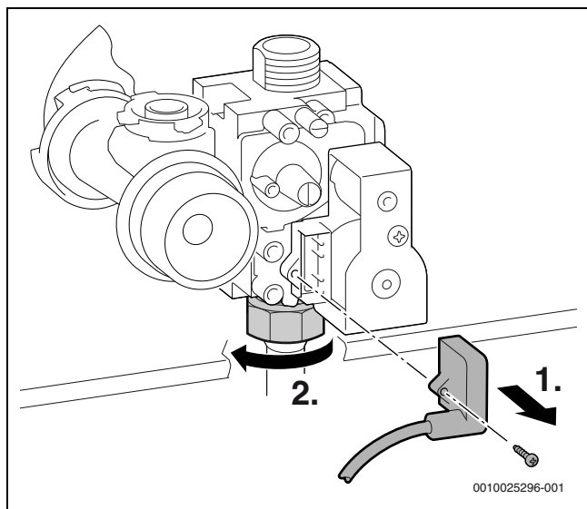
Bild 269 Stecker abziehen und Überwurfmutter lösen
