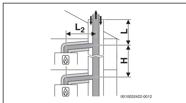
Bild 42 Mehrfachbelegung nach C (14)3x mit kollektiver starrer Abgasführung und konzentrischer Luft-Abgas-Führung im Aufstellraum
