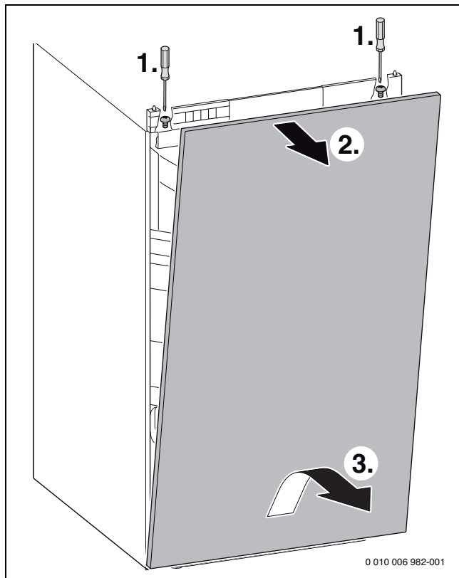
Bild 53 Vordere Verkleidung am Speicher abnehmen
