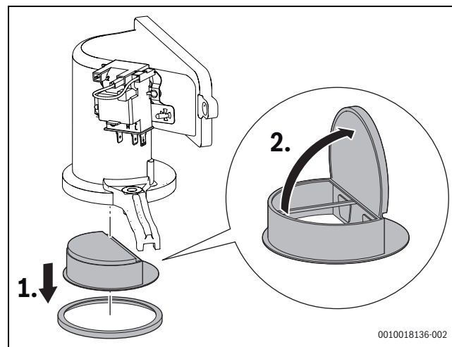
Bild 265 Rückschlagklappe in der Mischeinrichtung
