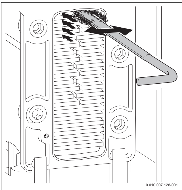
Bild 259 Wärmeblock mit Bürste reinigen
