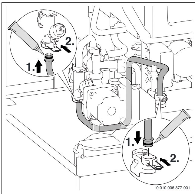
Bild 61 Rohrverbindung zwischen 3-Wege-Ventil und Plattenwärmetauscher erstellen (Vorlauf)
