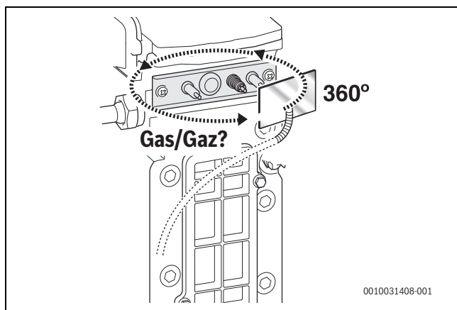
Bild 254 Dichtheit kontrollieren
