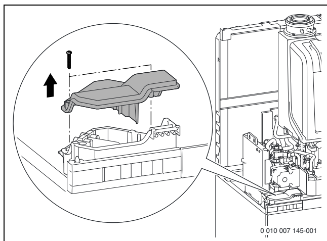
Bild 227 Abdeckung der Anschlussbox entfernen
