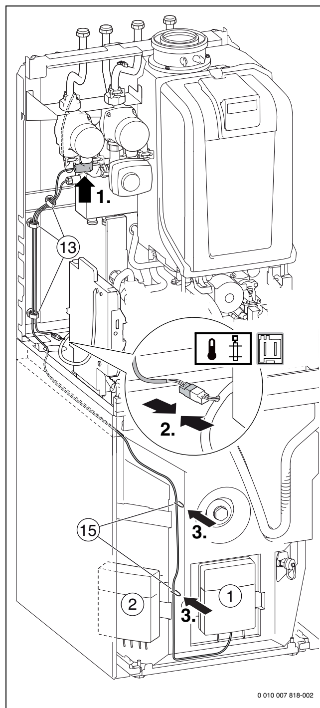
Bild 141 GB.192-..iT100-.-Geräte: Anschluss Heizungspumpe ungemischter Heizkreis und Hydraulische Weiche
