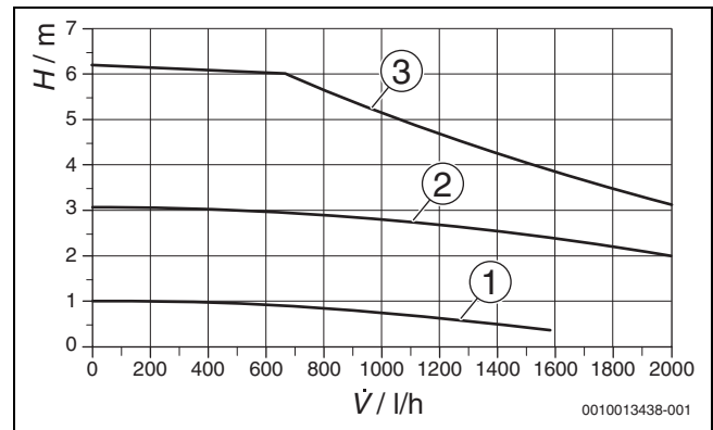
Bild 282 Pumpenkennlinien für die Pumpenstufen I bis III
