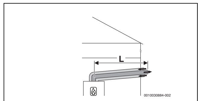
Bild 25 Horizontale konzentrische Luft-Abgas-Führung nach C 13x durch die Außenwand
