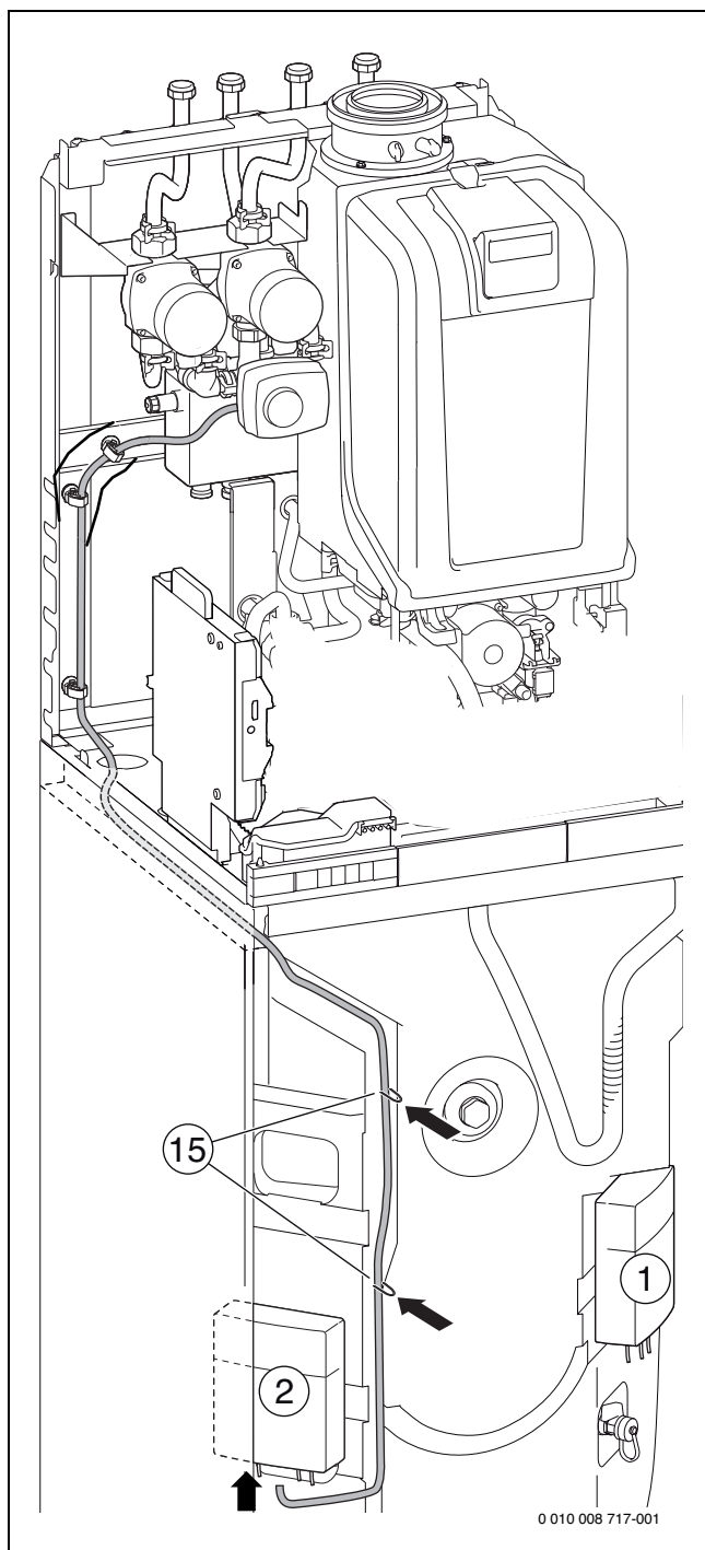
Bild 144 GB.192...iT150...-Geräte: Anschluss Mischermotor
