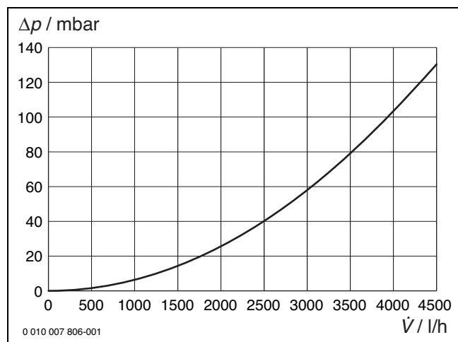
Bild 278 Druckverlust-Diagramm ungemischter Heizkreis (HK1)
