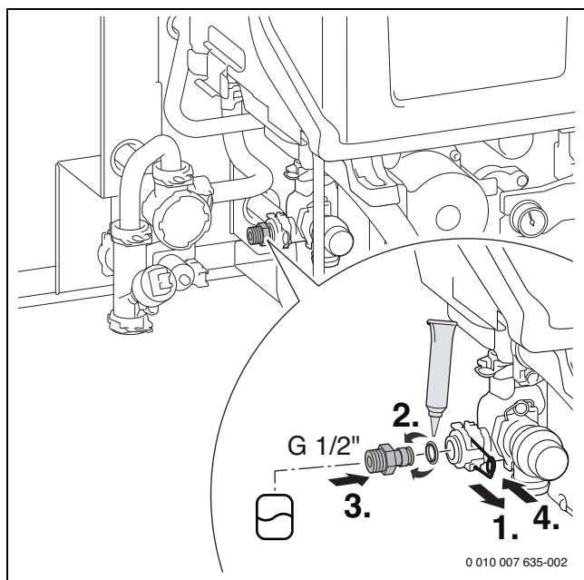
Bild 151 Verbindungsstück für den bauseitigen Anschluss eines externen Ausdehnungsgefäßes montieren
