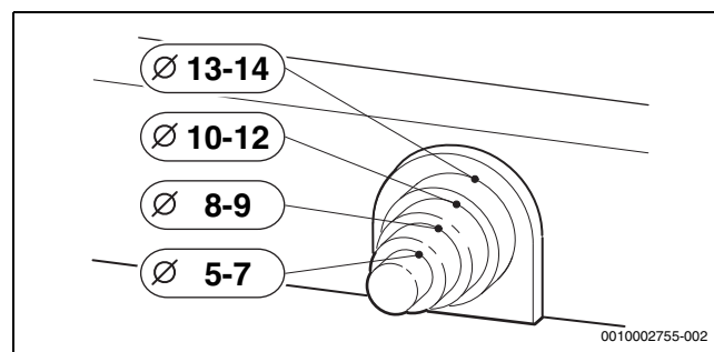
Bild 146 Zugentlastung Kabel Mischermotor anpassen
