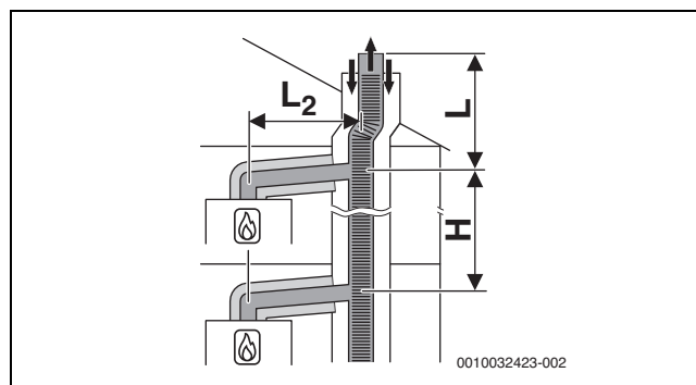
Bild 43 Mehrfachbelegung nach C (14)3x mit kollektiver flexibler Abgasableitung und konzentrischer Luft-Abgas-Führung im Aufstellraum
