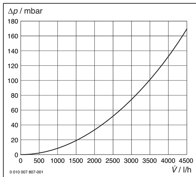
Bild 279 Druckverlust-Diagramm gemischter Heizkreis (HK2)
