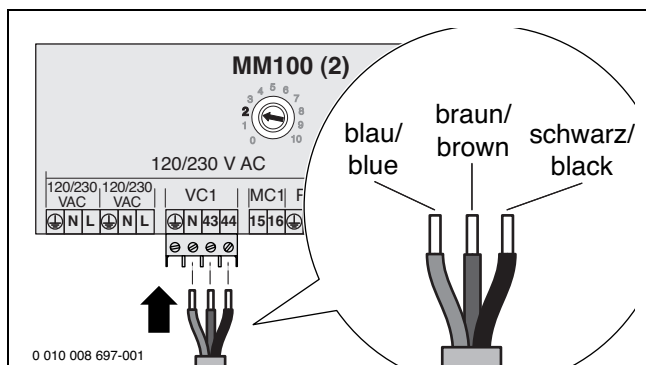
Bild 147 Anschluss Kabel Mischermotor am Modul MM100 [2]
