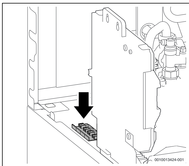
Bild 65 Steckerleiste auf dem Speicher befestigen
