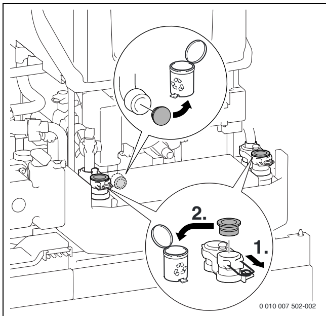
Bild 60 Stopfen am Wärmeblock und am Plattenwärmetauscher entfernen
