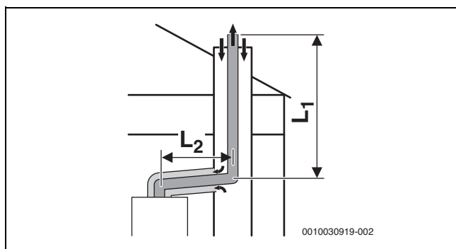
Bild 33 Starre Abgasführung nach C 93x im Schacht und konzentrische Luft-Abgas-Führung im Aufstellraum
