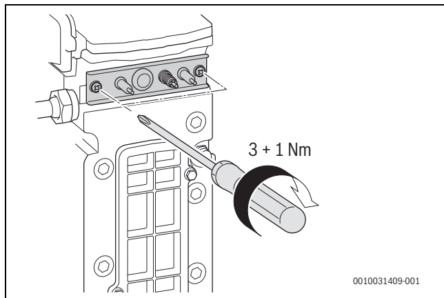
Bild 253 Elektroden-Set wieder einbauen
