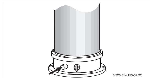
Bild 249 Abgasmessstutzen
