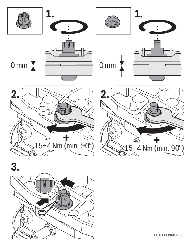
Bild 257 Mutter am Brennerdeckel festziehen
