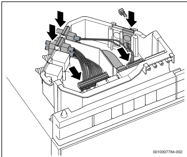
Bild 69 Steuergerät an der Anschlussbox anschließen
