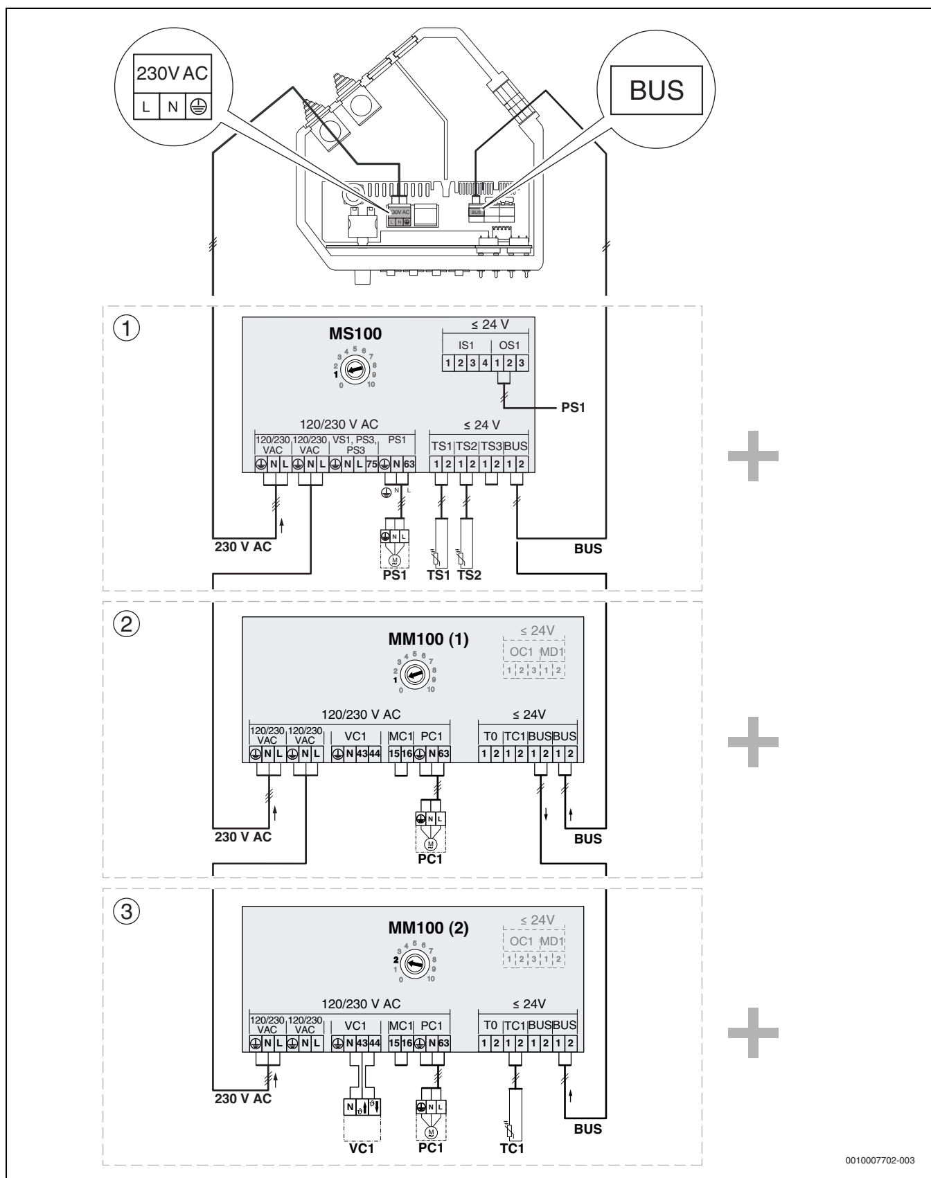
Bild 230 Anschluss der Module MS100 und MM100, wenn vorhanden
