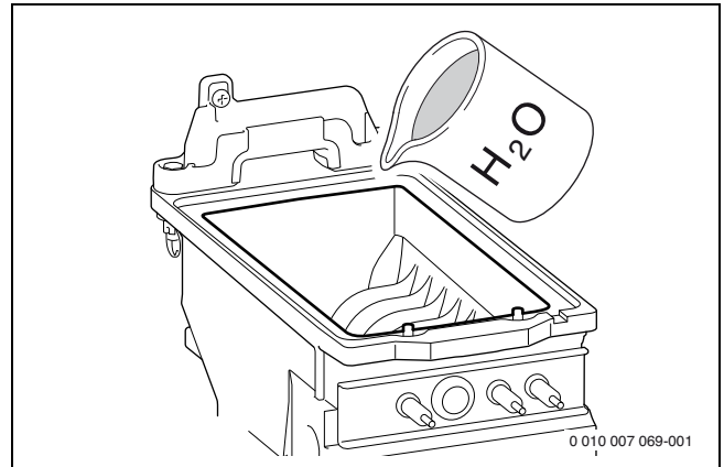
Bild 260 Spülen
