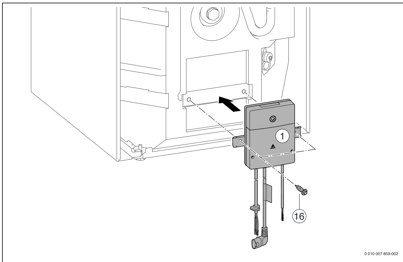
Bild 111 GB.192-..iT100..-Geräte
