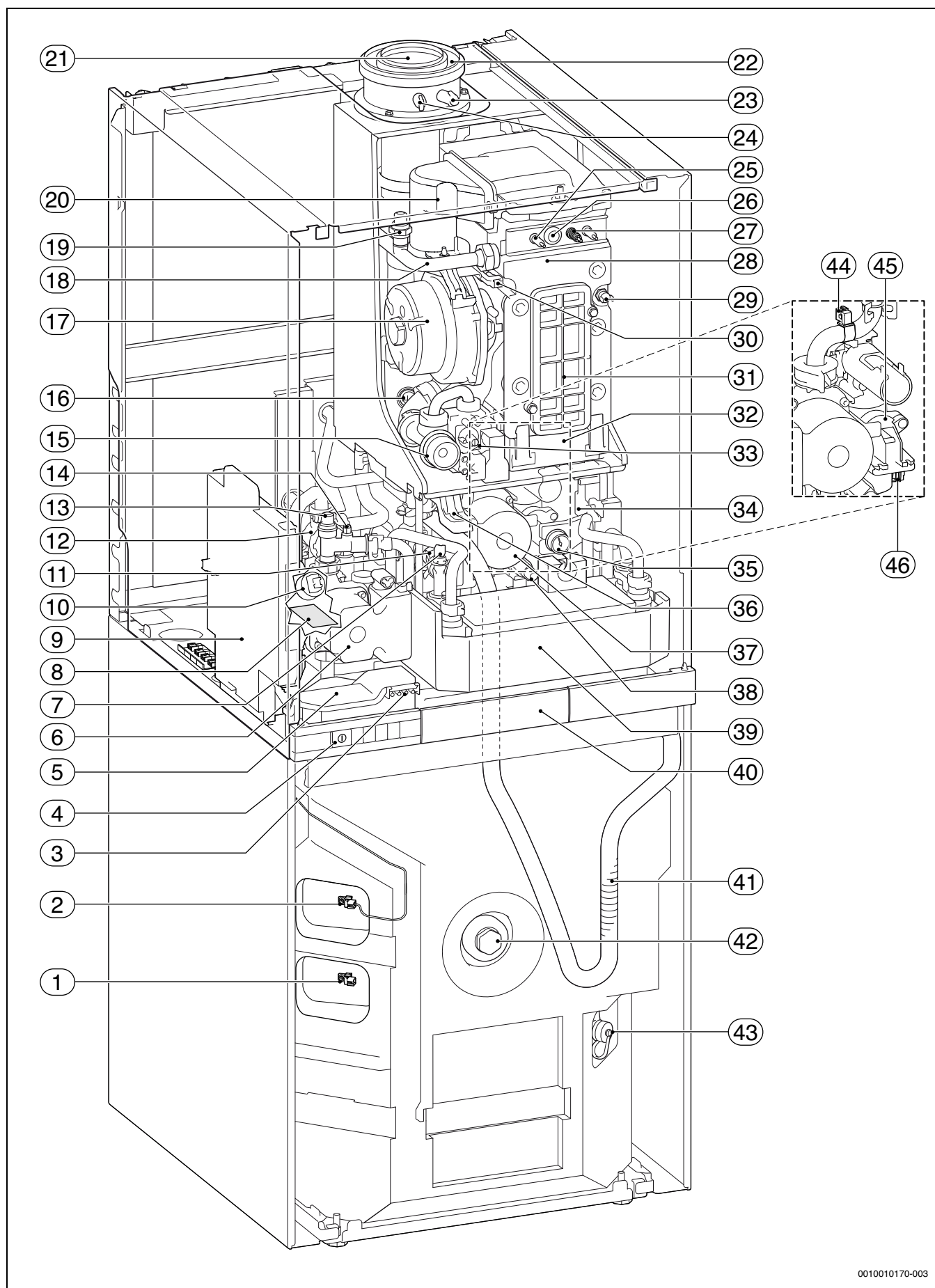
Bild 19 GB.192... iT100...-Geräte
