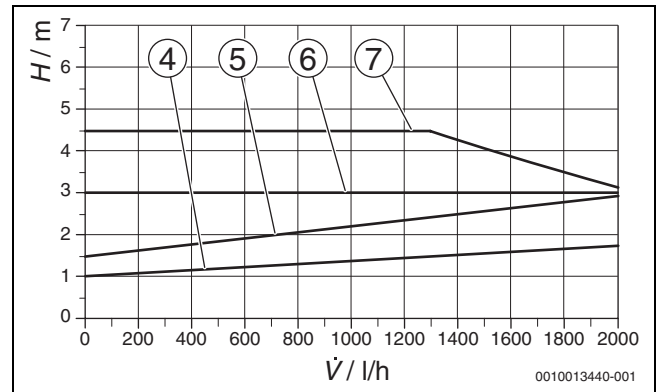
Bild 283 Pumpenkennlinien für Proportionaldruck und Konstantdruck
