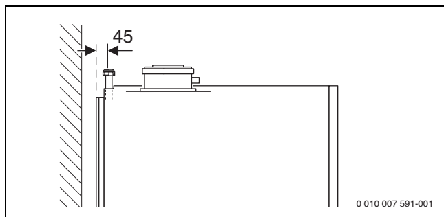
Bild 16 Anschlussmaße des Zubehörs Anschluss-Set solare Heizungsunterstützung SHU (Maße in mm)
