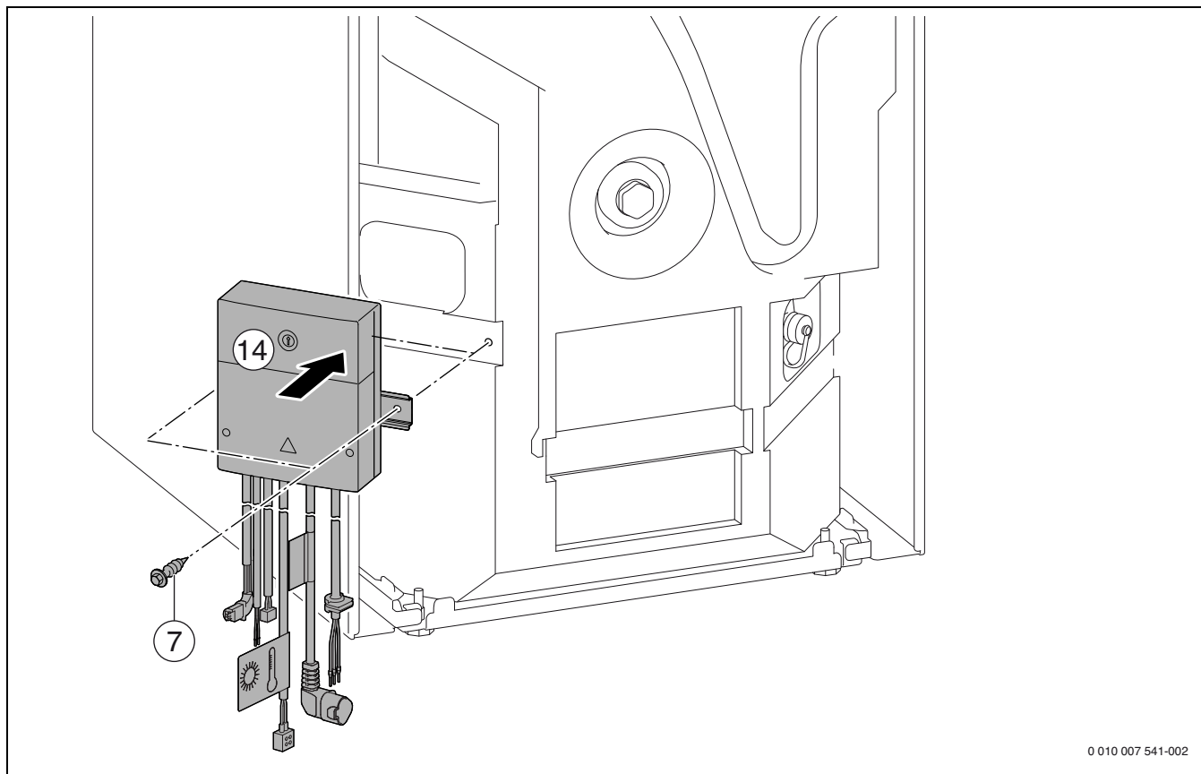
Bild 176 GB.192...iT100...-Geräte
