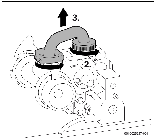
Bild 268 Gasrohr ausbauen
