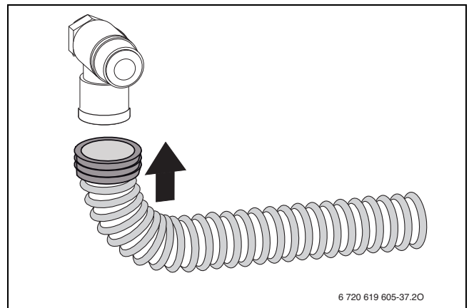
Bild 48 Schlauch am Sicherheitsventil montieren
