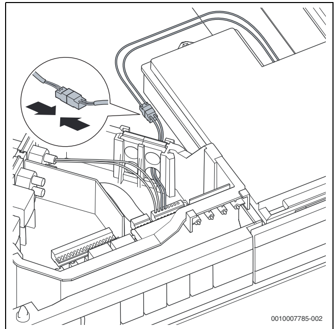
Bild 71 Schublade für den Regler an der Anschlussbox anschließen
