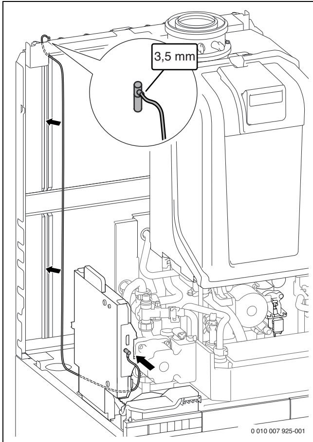
Bild 232 Anschluss und Verlegung des Kabels an Buderus Logamatic web KM100
