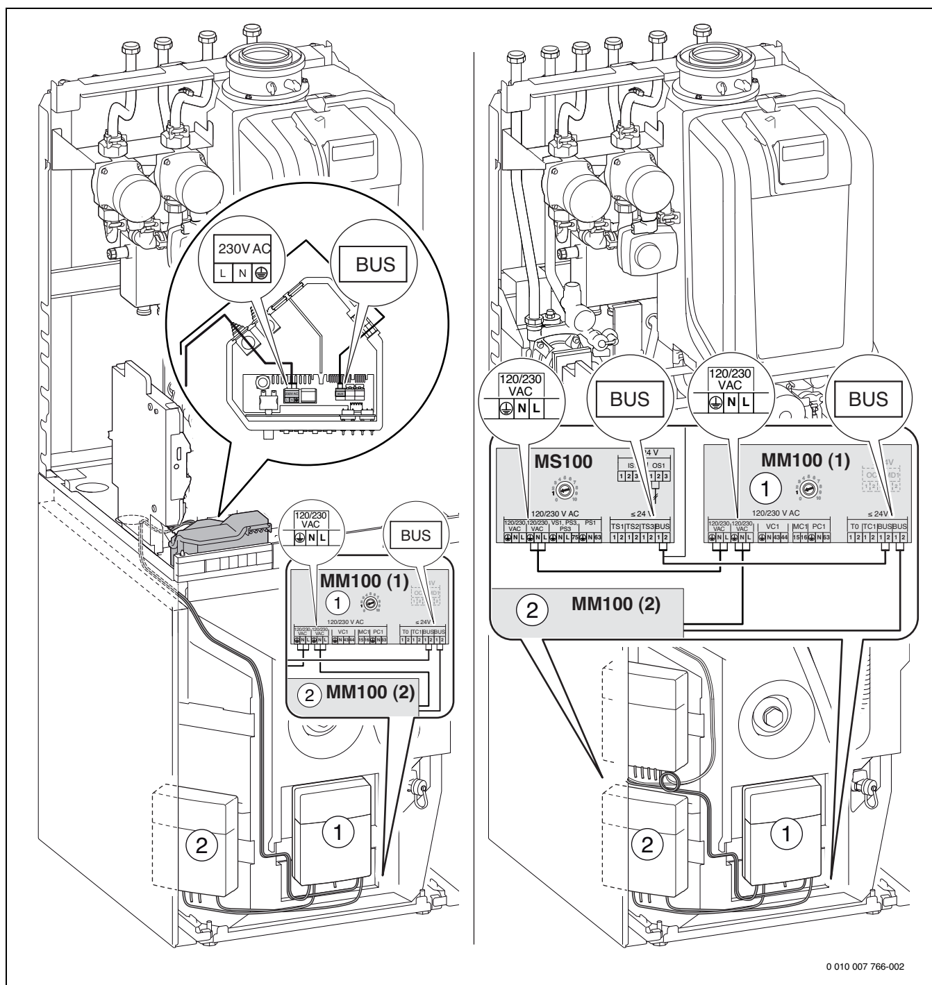
Bild 149 GB.192...iT100...-Geräte: Anschluss ohne Modul MS100 (links) und mit Modul MS100 (rechts) durchschleifen
