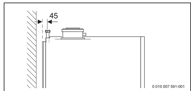
Bild 14 Anschlussmaße des Zubehörs Anschluss-Set Heizungsunterstützung HU (Maße in mm)
