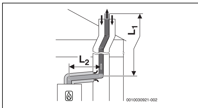
Bild 34 Flexible Abgasführung nach C 93x im Schacht und konzentrische Luft-Abgas-Führung im Aufstellraum
