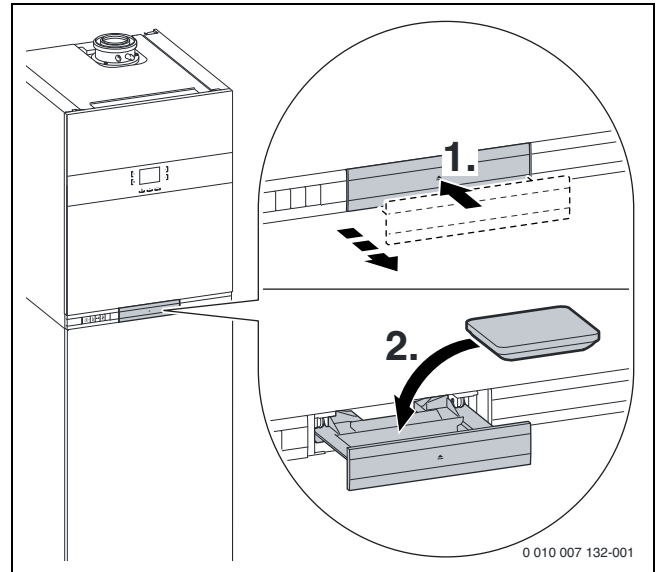
Bild 233 Heizungsregler einstecken
