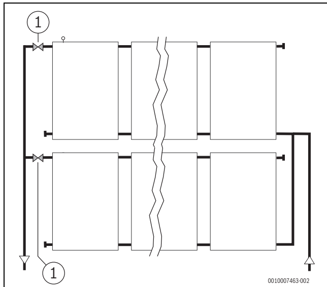
Bild 235 Spülen von parallel geschalteten Kollektorfeldern
