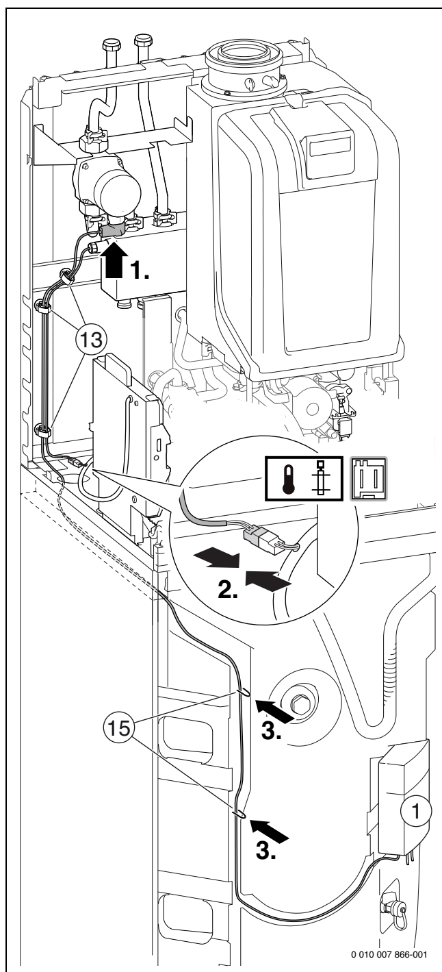
Bild 112 GB.192-..iT150-.-Geräte: Anschluss Heizungspumpe ungemischter Heizkreis und Hydraulische Weiche
