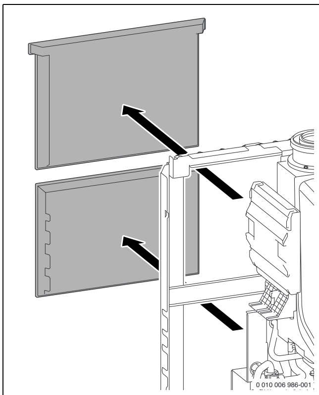
Bild 72 Wärmedämmungen an der Rückseite abnehmen
