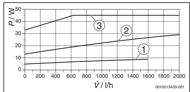
Bild 284 Leistungsaufnahme für die Pumpenstufen I bis III
