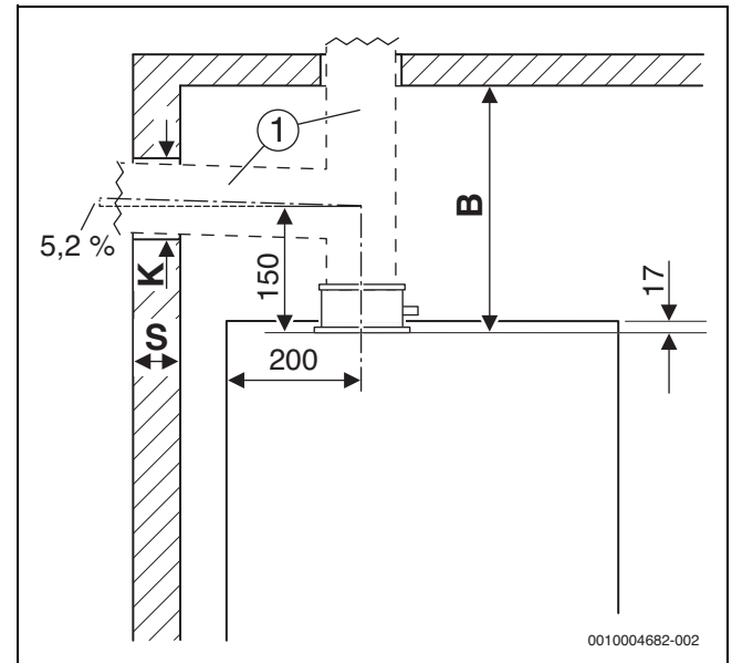
Bild 17 Abmessungen und Mindestabstände
