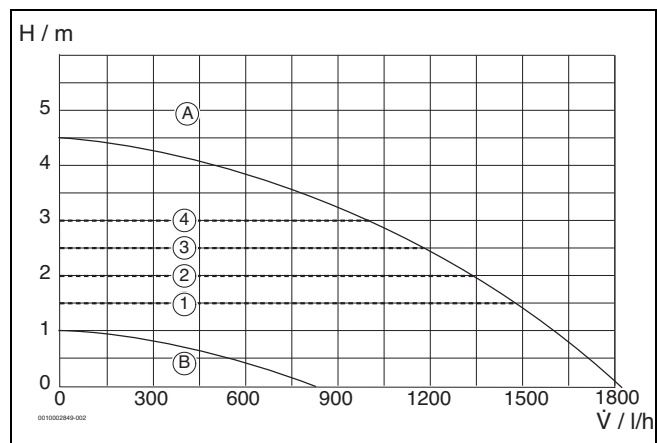
Bild 276 Pumpenkennfelder und Pumpenkennlinien
