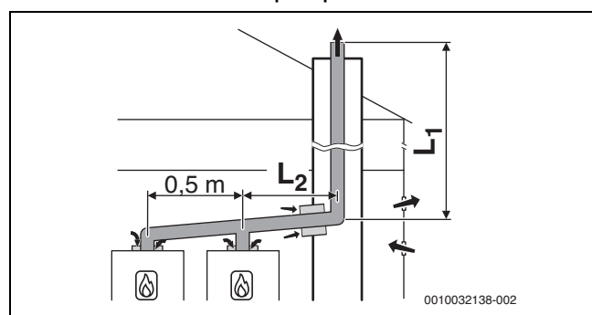
Bild 44 Kaskade mit 2 Geräten: Starre Abgasführung im Schacht nach B 23p /B 53p mit raumluft- abhängiger Luftzufuhr am Gerät
