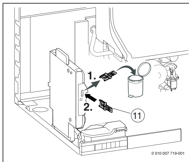
Bild 163 KIM tauschen
