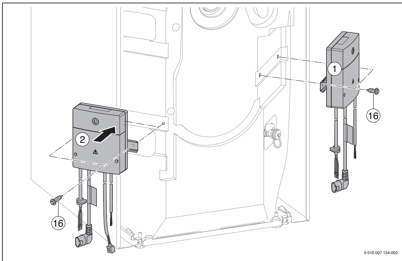
Bild 138 GB.192-..iT150-.-Geräte
