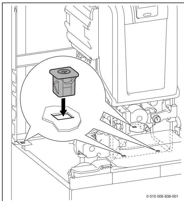
Bild 56 Gerät mit den 4 mitgelieferten Clips auf dem Speicher fixieren
