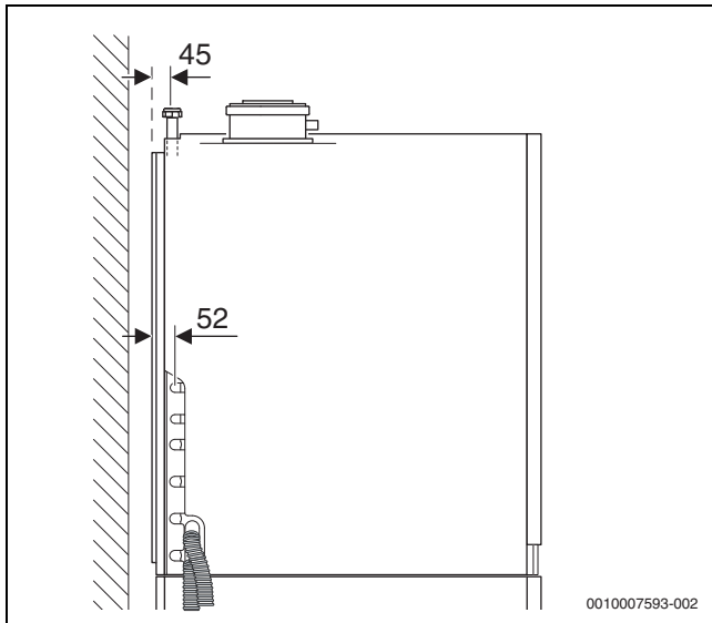
Bild 12 Anschlussmaße des Zubehörs Heizkreiserweiterung 2 (Maße in mm)
