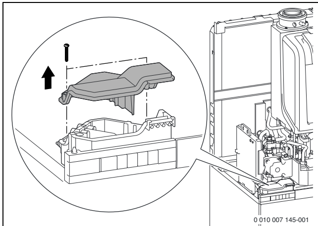
Bild 68 Abdeckung der Anschlussbox entfernen
