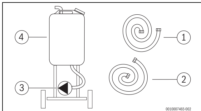
Bild 236 Bestandteile einer Befülleinrichtung
