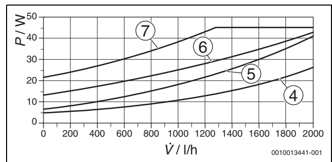
Bild 285 Leistungsaufnahme für Proportionaldruck und Konstantdruck
