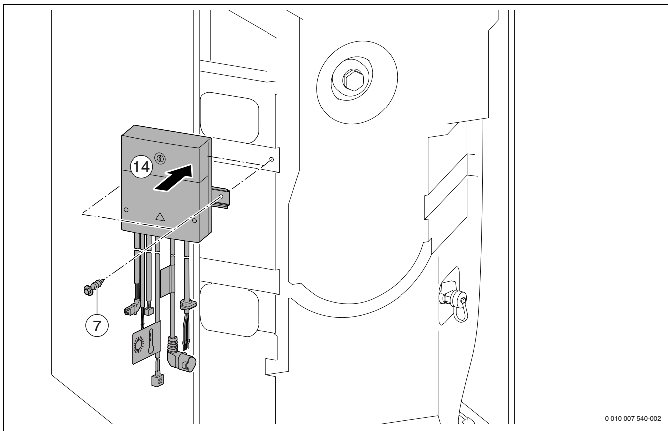
Bild 175 GB.192...iT150...-Geräte
