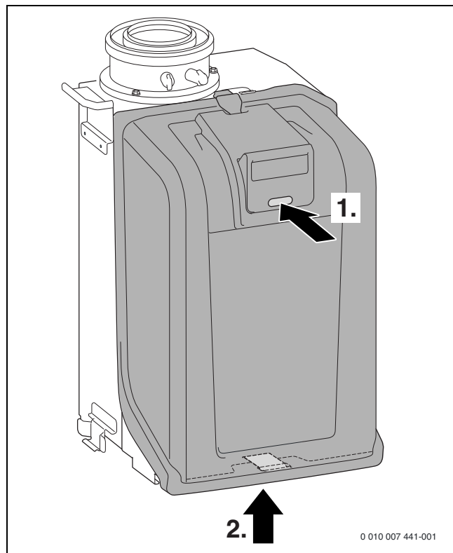
Bild 247 Brennerhaube abnehmen
