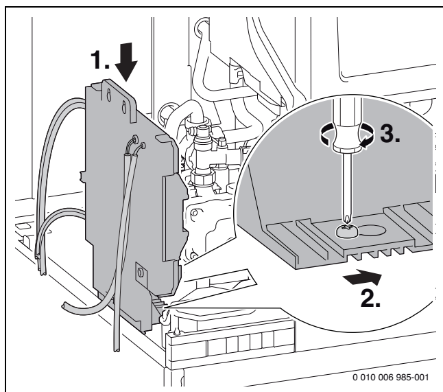
Bild 64 Steuergerät auf dem Speicher befestigen
