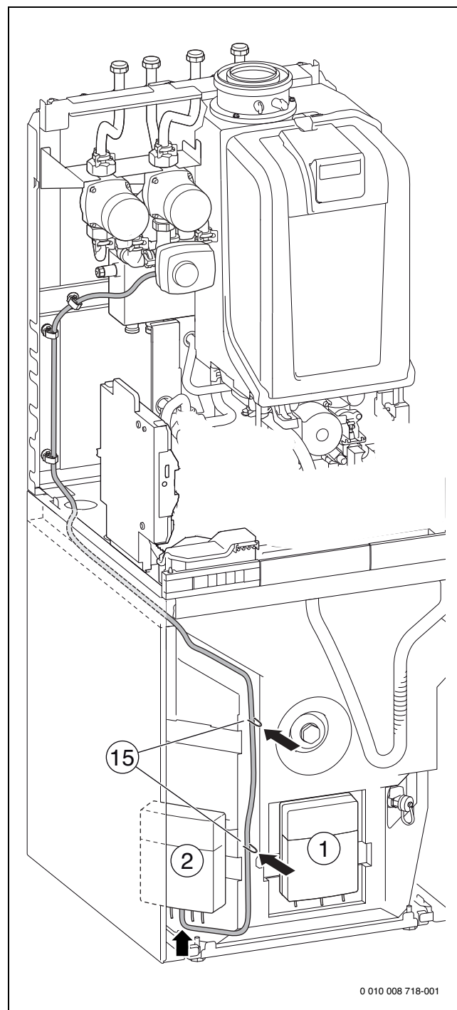
Bild 145 GB.192...iT100...-Geräte: Anschluss Mischermotor
