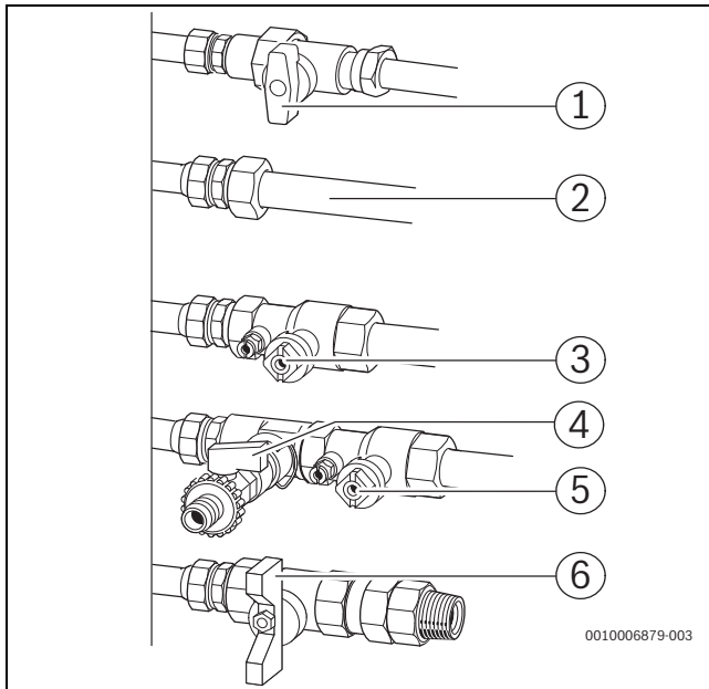
Bild 225 Gas- und wasserseitige Anschlüsse (Beispiel: Anschlusszubehör waagrecht rechts)
