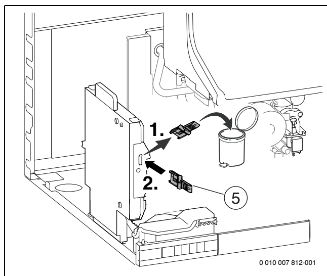
Bild 153 KIM tauschen
