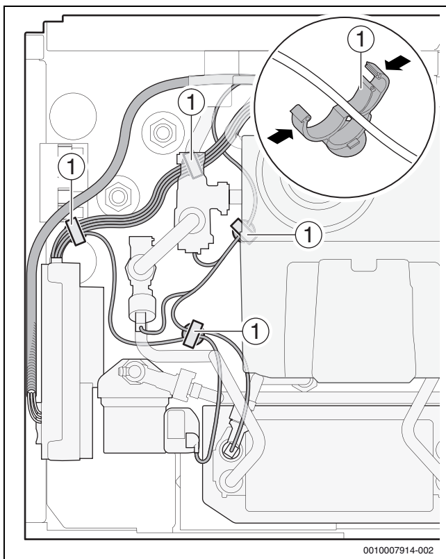
Bild 70 Kabel mit 4 Clips befestigen
