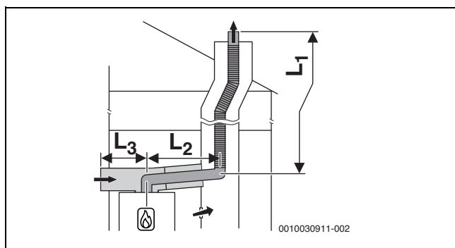
Bild 28 Flexible Abgasführung nach C 53x im Schacht und Luft-Abgas-Führung mit separater Luftzufuhr und konzentrischer Abgasableitung im Aufstellraum
