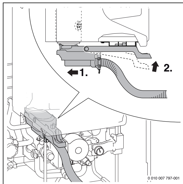
Bild 54 Schmutzfänger montieren
