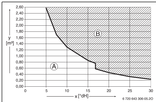
Bild 43 Anforderungen an Füll- und Ergänzungswasser Geräte < 50 kW
