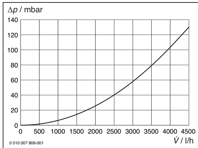
Bild 223 Druckverlust-Diagramm ungemischter Heizkreis (HK1)
