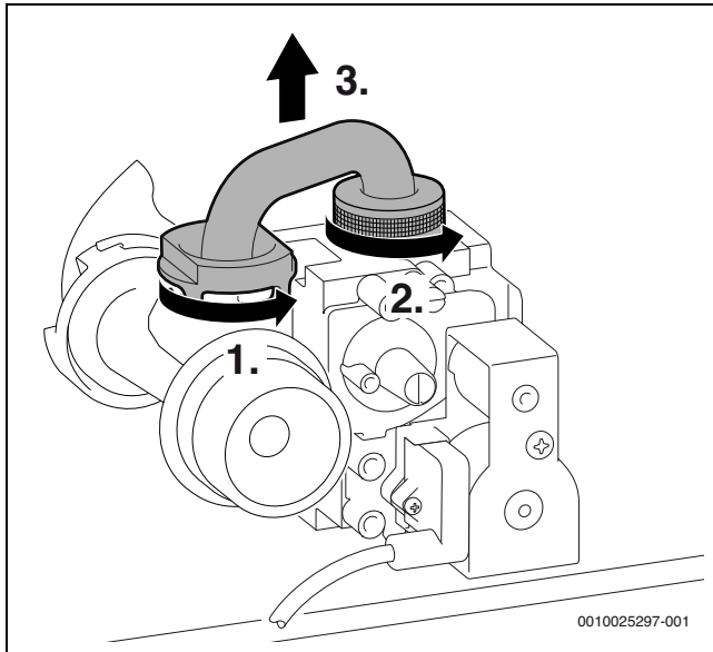
Bild 215 Gasrohr ausbauen
