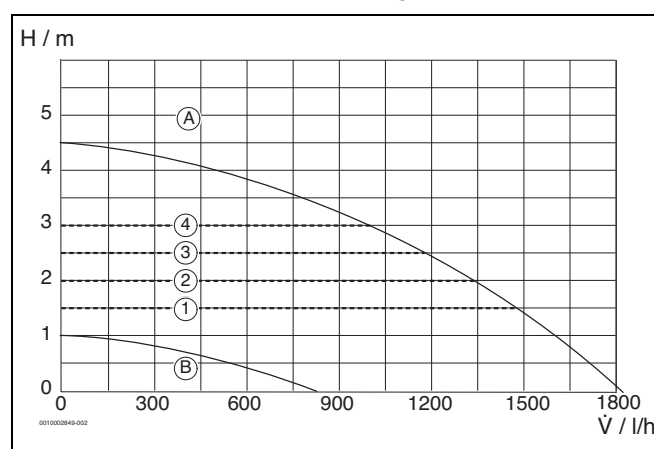
Bild 222 Pumpenkennfelder und Pumpenkennlinien
