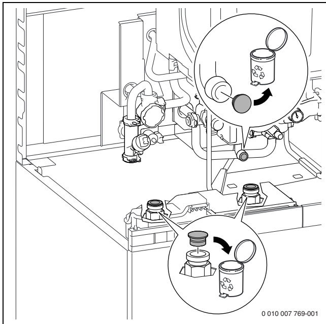
Bild 56 Stopfen am Wärmeblock und am Speichervor- und -Rücklauf entfernen
