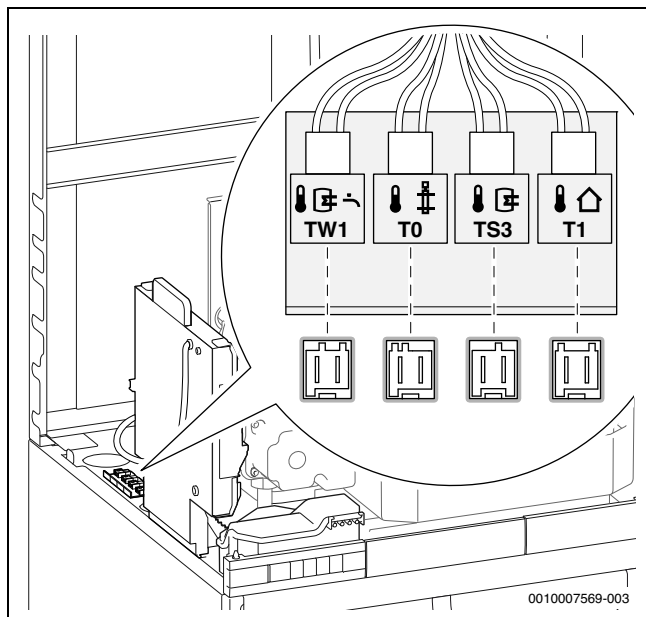
Bild 183 Stecker am Steuergerät
