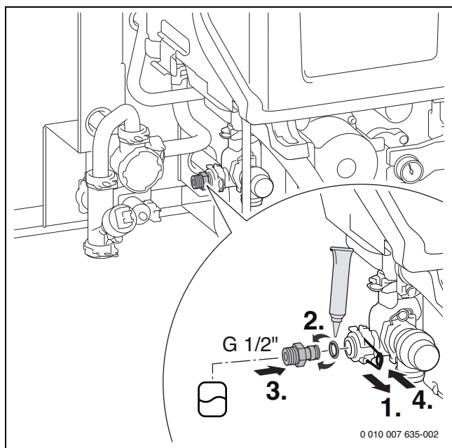
Bild 110 Verbindungsstück für den bauseitigen Anschluss eines externen Ausdehnungsgefäßes montieren
