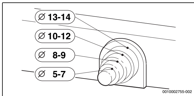
Bild 135 Zugentlastung Kabel Mischermotor anpassen
