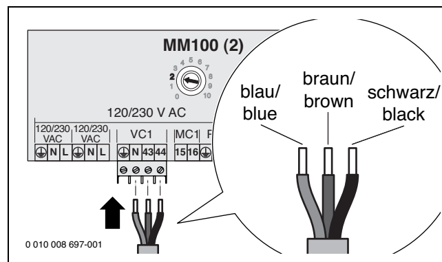
Bild 136 Anschluss Kabel Mischermotor am Modul MM100 [2]
