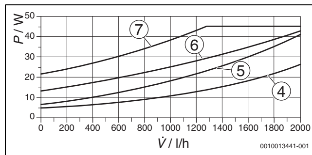
Bild 230 Leistungsaufnahme für Proportionaldruck und Konstantdruck
