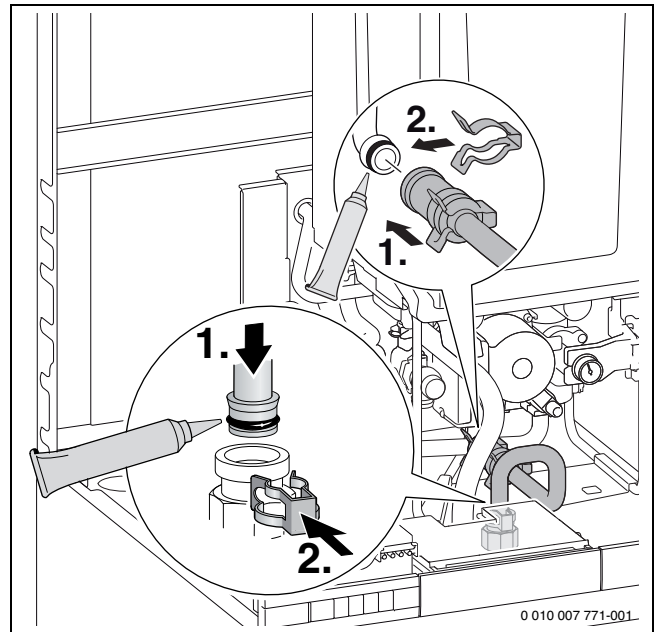
Bild 58 Rohrverbindung zwischen Speicherrücklauf und Wärmeblock erstellen
