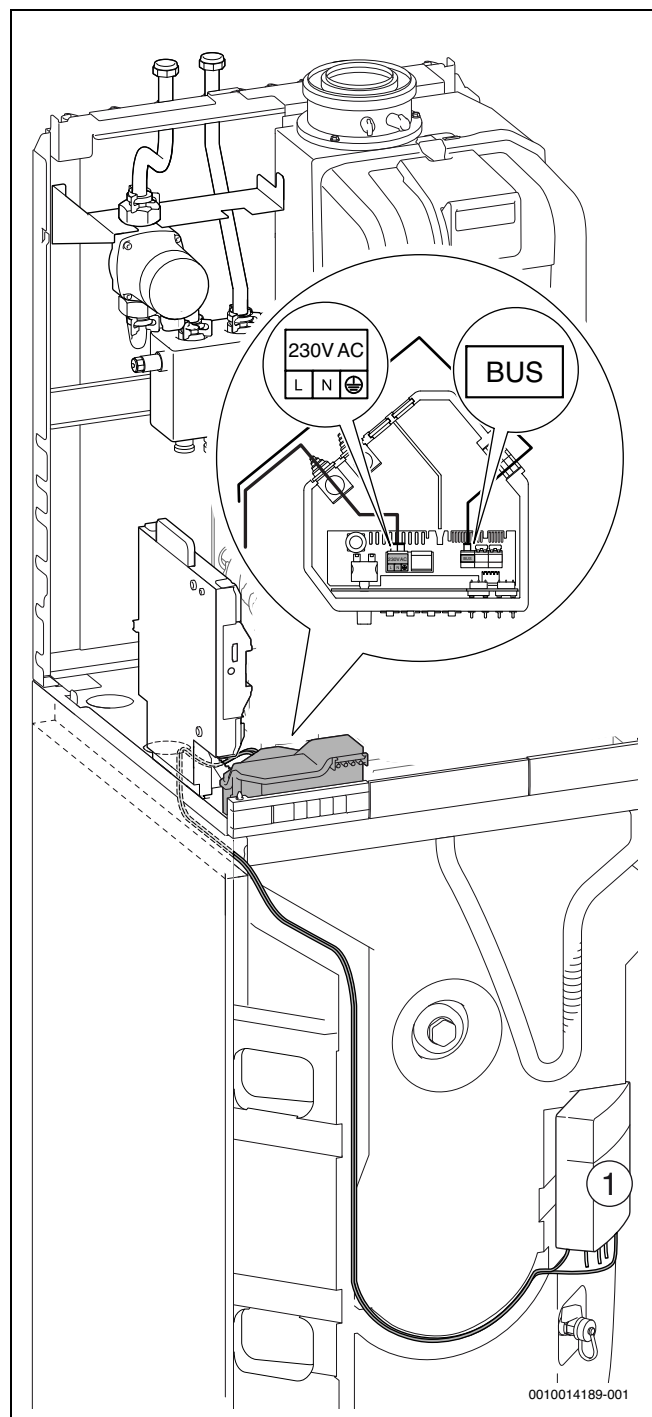
Bild 108 Anschluss Modul MM100
