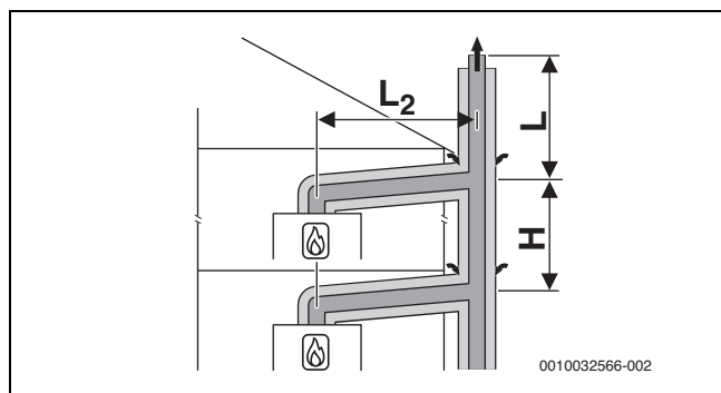
Bild 38 Mehrfachbelegung nach C (13)3x mit konzentrischer Luft-Abgas-Führung an der Außenwand und im Aufstellraum
