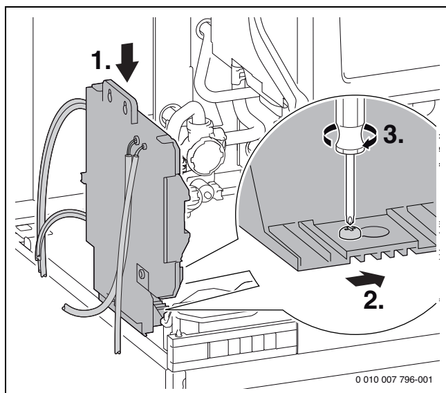
Bild 60 Steuergerät auf dem Speicher befestigen
