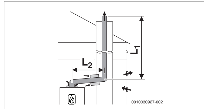
Bild 32 Starre Abgasführung im Schacht nach B 23p /B 53p mit raumluftabhängiger Luftzufuhr am Gerät und konzentrischem Verbindungsstück zwischen Aufstellraum und Schacht
