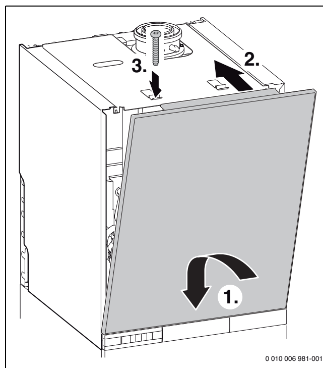
Bild 189 Vordere Verkleidung einhängen und mit Schraube aus Lieferumfang sichern
