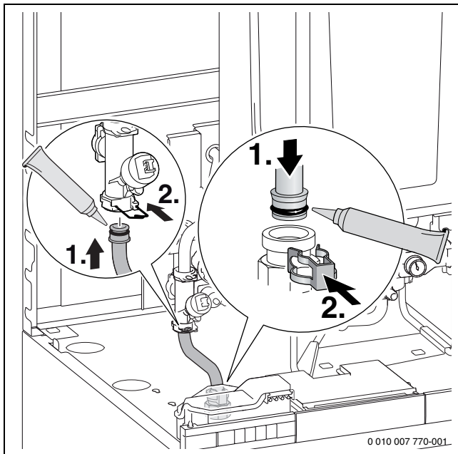
Bild 57 Rohrverbindung zwischen 3-Wege-Ventil und Speichervorlauf erstellen
