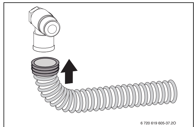
Bild 45 Schlauch am Sicherheitsventil montieren
