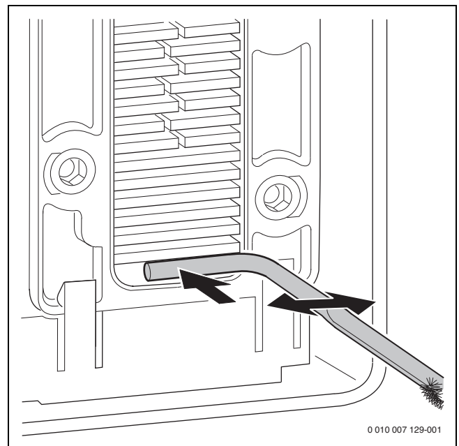
Bild 209 Kondensatwanne reinigen
