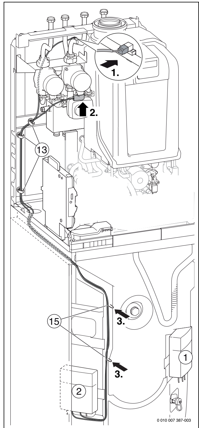
Bild 133 Anschluss Heizungspumpe gemischter Heizkreis und Temperaturfühler
