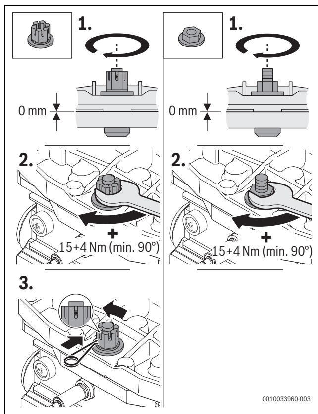
Bild 205 Mutter am Brennerdeckel festziehen
