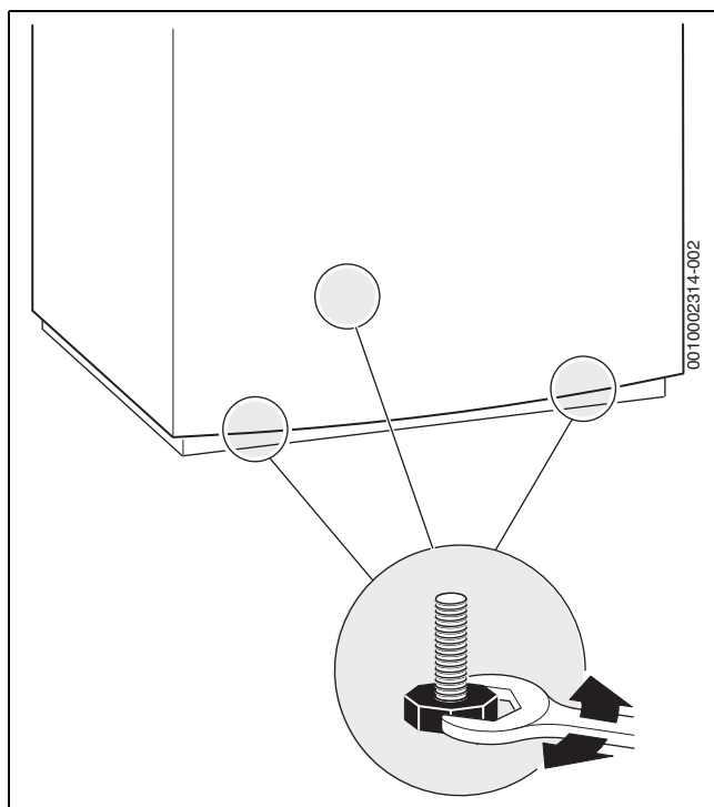
Bild 50 Speicher ausrichten
