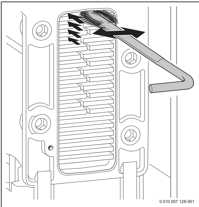
Bild 207 Wärmeblock mit Bürste reinigen
