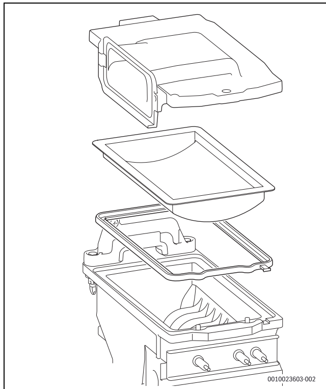
Bild 204 Brenner
