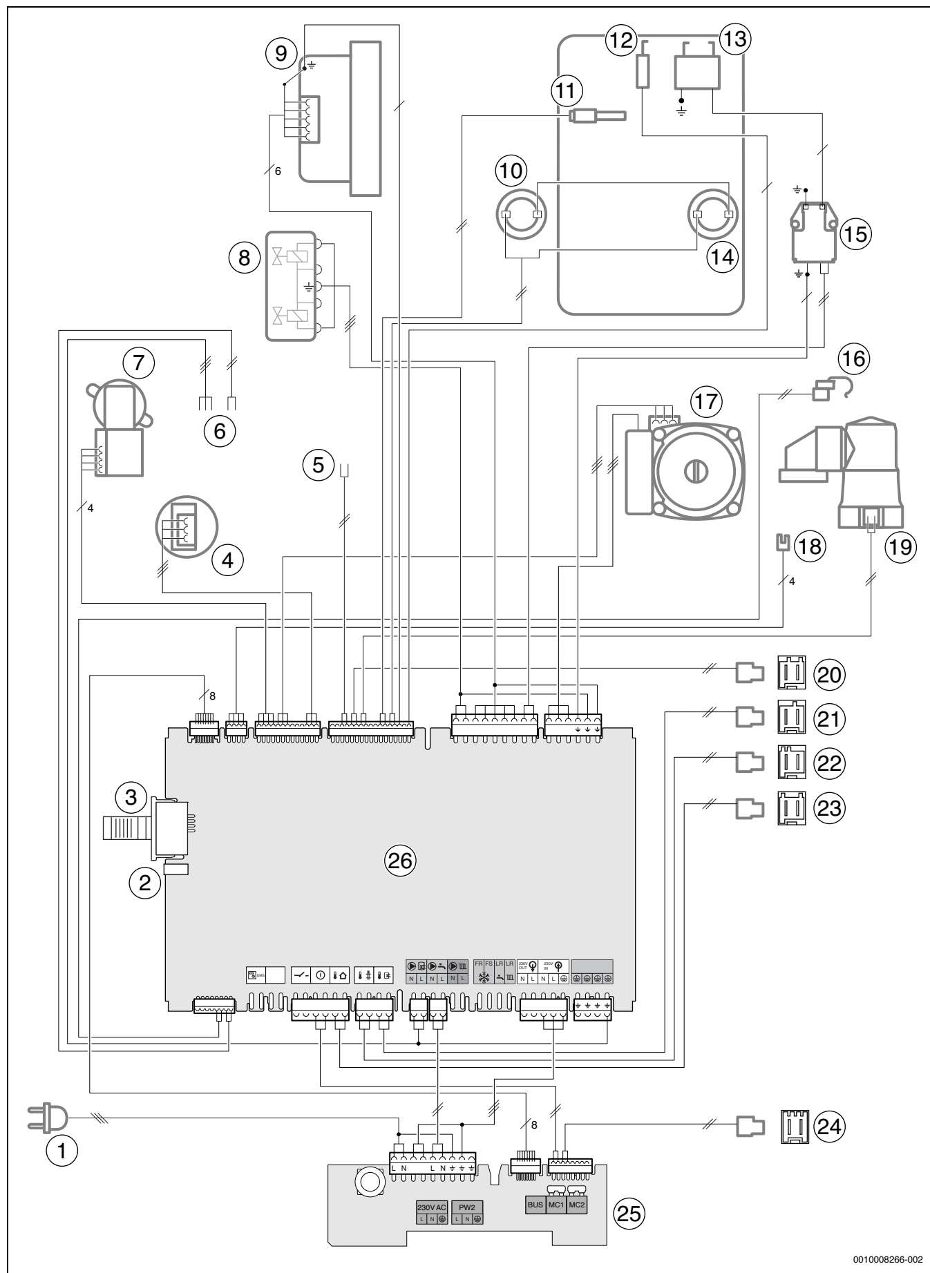
Bild 221 Elektrische Verdrahtung
