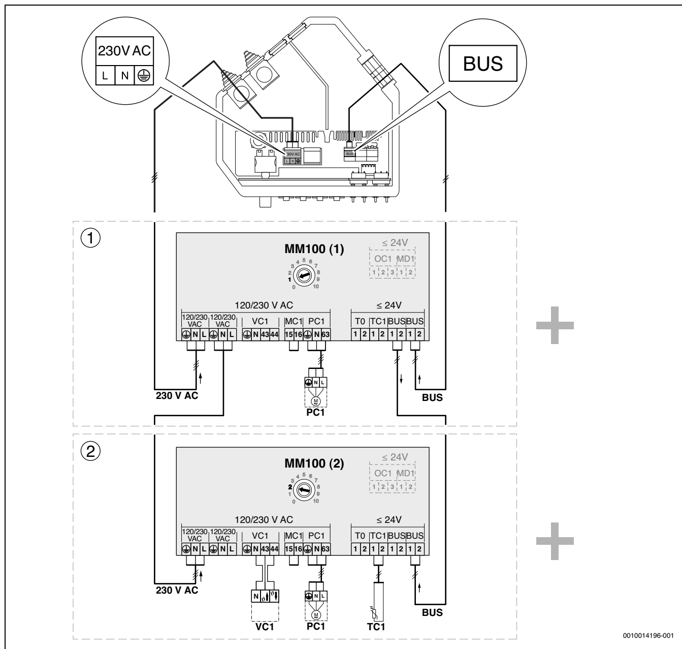
Bild 182 Anschluss der Module MM100, wenn vorhanden
