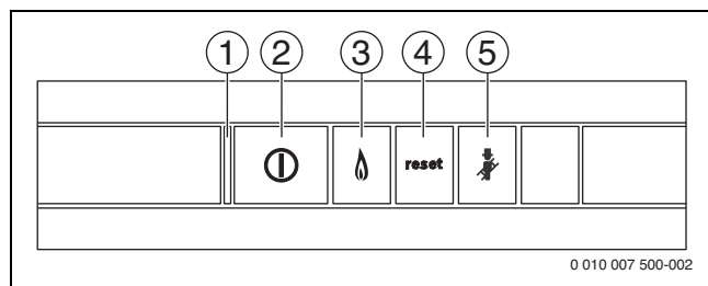
Bild 191 Bedientasten
