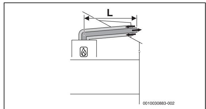
Bild 23 Horizontale konzentrische Luft-Abgas-Führung nach C 13x über das Dach
