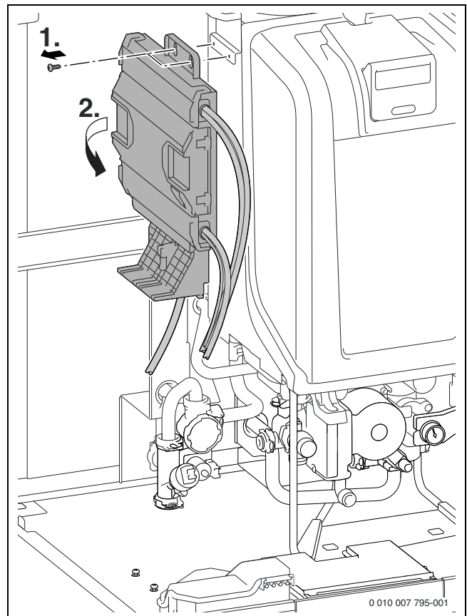
Bild 59 Steuergerät abnehmen
