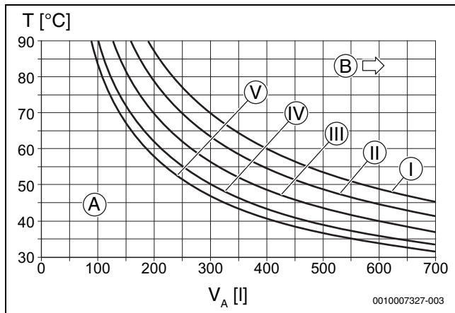
Bild 44 Kennlinien des Ausdehnungsgefäßes 17 I
