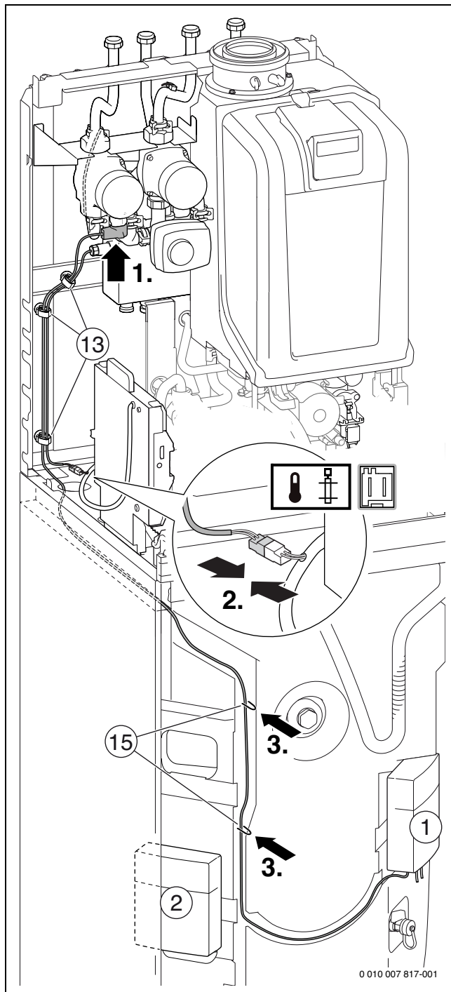
Bild 132 Anschluss Heizungspumpe ungemischter Heizkreis und Hydraulische Weiche
