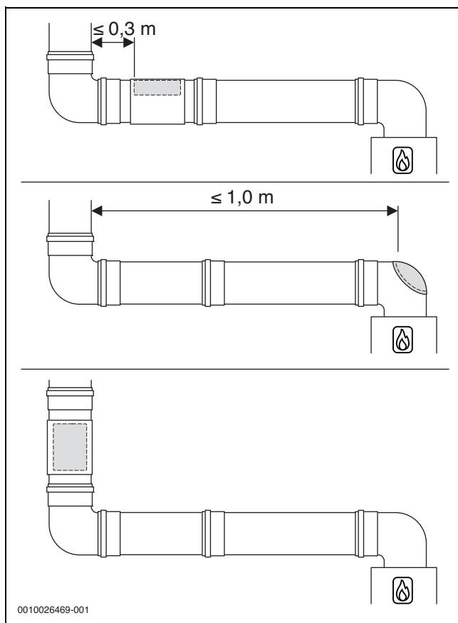
Bild 18 Anordnung der unteren Prüföffnung
