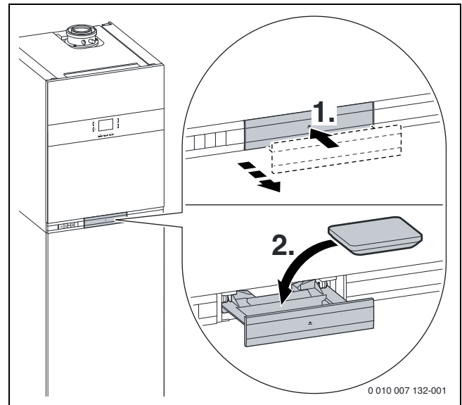
Bild 185 Heizungsregler einstecken
