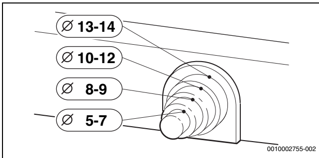
Bild 180 Zugentlastung an Kabeldurchmesser anpassen
