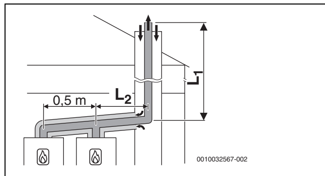
Bild 42 Kaskade mit 2 Geräten:
