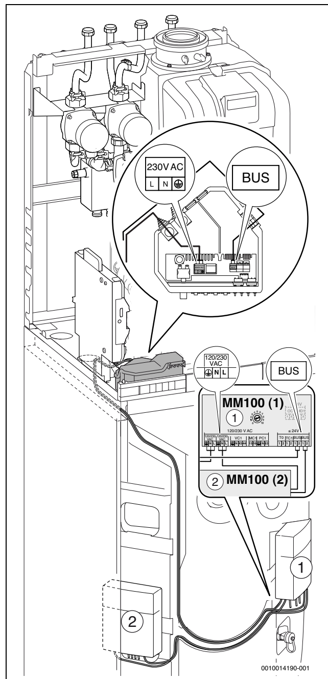
Bild 137 Anschluss MM100 (1) und MM100 (2)
