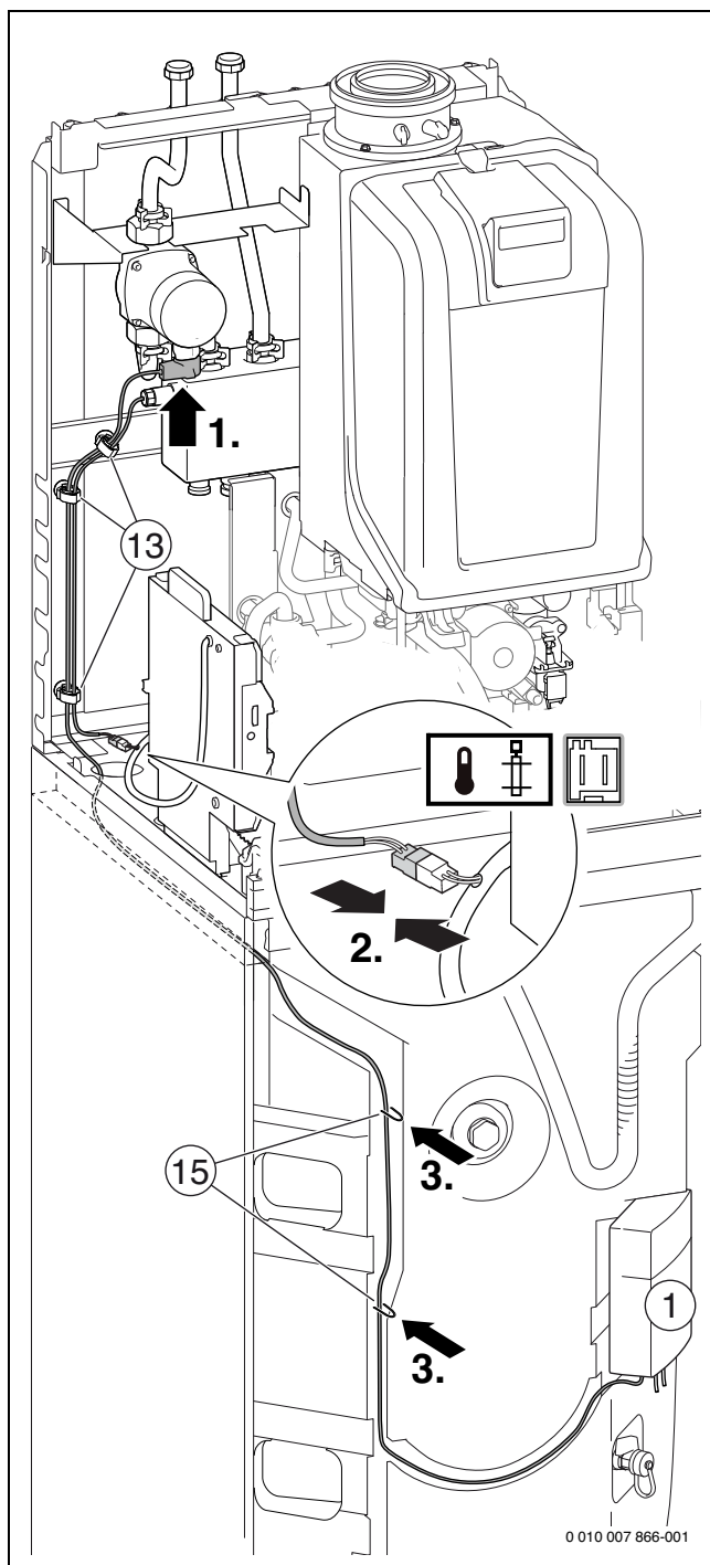
Bild 107 Anschluss Heizungspumpe ungemischter Heizkreis und Hydraulische Weiche
