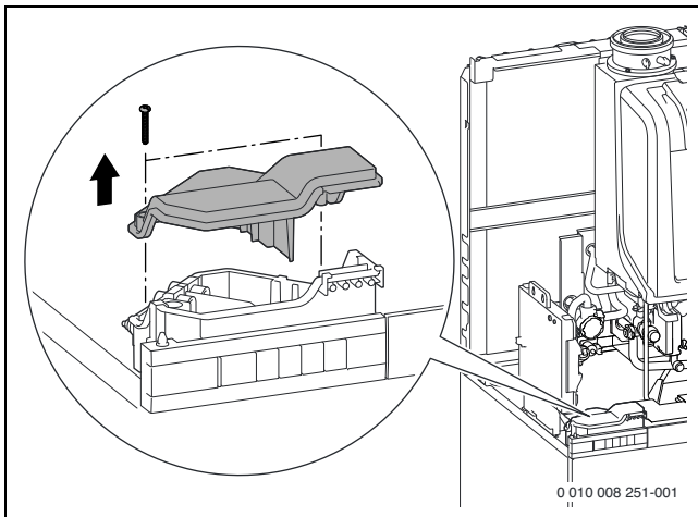
Bild 179 Abdeckung der Anschlussbox entfernen
