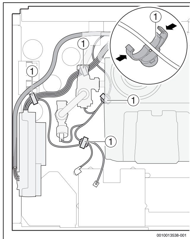
Bild 65 Kabel mit 4 Clips befestigen
