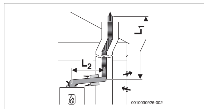
Bild 33 Flexible Abgasführung im Schacht nach B 23p /B 53p mit raumluftabhängiger Luftzufuhr am Gerät und konzentrischem Verbindungsstück zwischen Aufstellraum und Schacht
