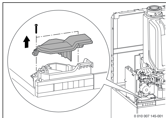
Bild 63 Abdeckung der Anschlussbox entfernen
