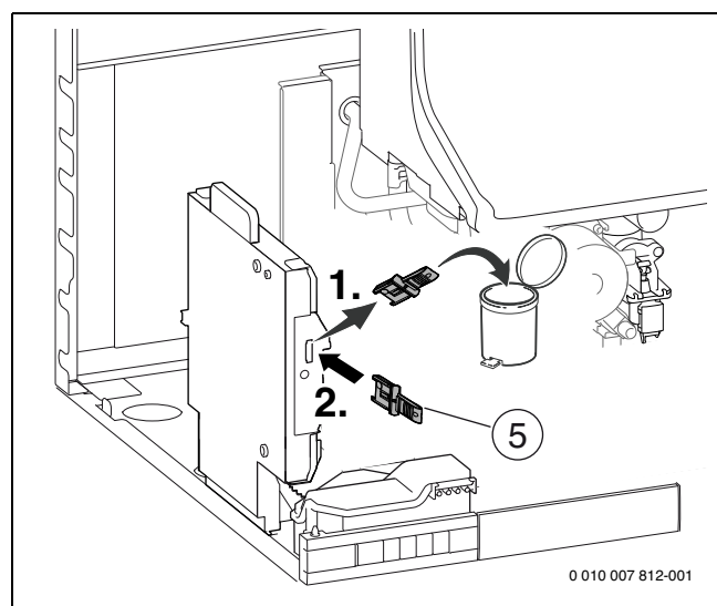
Bild 141 KIM tauschen
