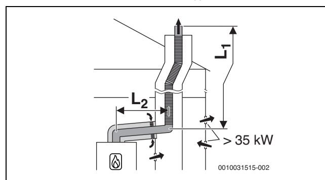
Bild 35 Flexible Abgasführung im Schacht nach B 33 mit raumluftabhängiger Luftzufuhr über die konzentrische Luft-Abgas-Führung im Aufstellraum
