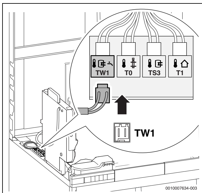
Bild 62 Speichertemperaturfühler anschließen
