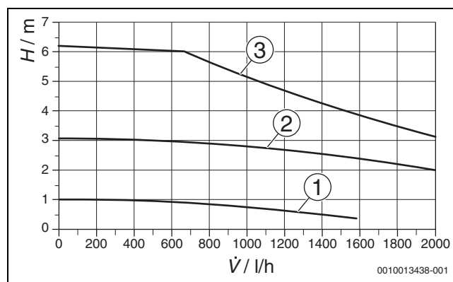
Bild 227 Pumpenkennlinien für die Pumpenstufen I bis III
