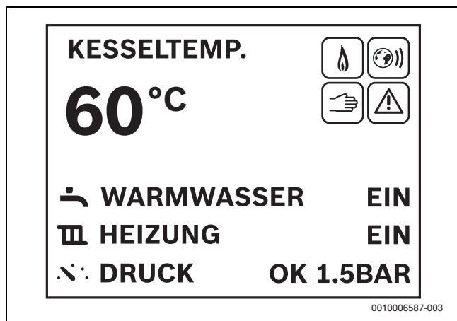
Bild 193 Standardanzeige
