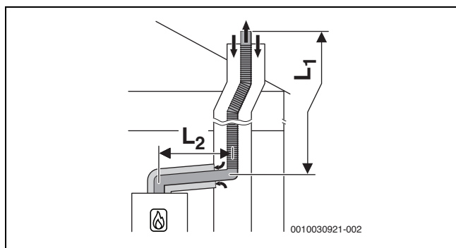
Bild 31 Flexible Abgasführung nach C 93x im Schacht und konzentrische Luft-Abgas-Führung im Aufstellraum
