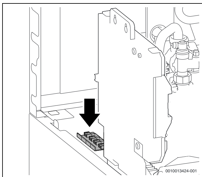
Bild 61 Steckerleiste auf dem Speicher befestigen
