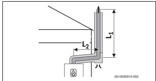
Bild 29 Konzentrische Luft-Abgas-Führung nach C 53x an der Außenwand
