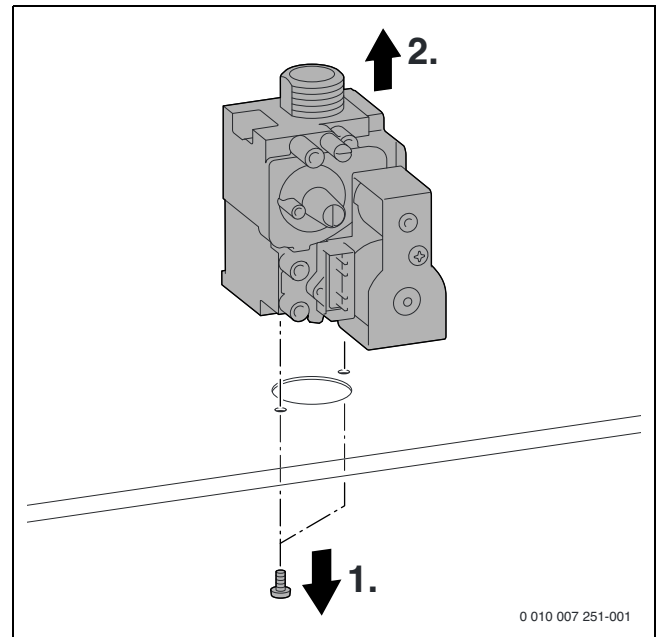
Bild 217 Gasarmatur ausbauen
