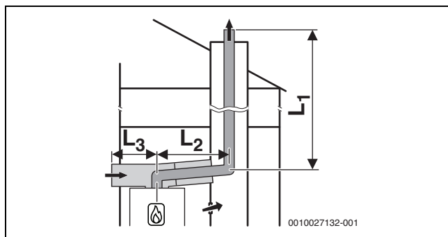
Bild 27 Starre Abgasführung nach C 53x im Schacht und Luft-Abgas-Führung mit separater Luftzufuhr und konzentrischer Abgasableitung im Aufstellraum
