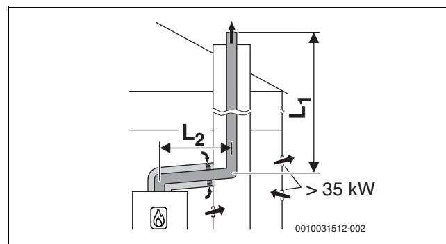
Bild 34 Starre Abgasführung im Schacht nach B 33 mit raumluftabhängiger Luftzufuhr über die konzentrische Luft-Abgas-Führung im Aufstellraum
