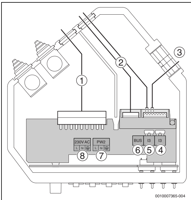
Bild 181 Anschlussbox
