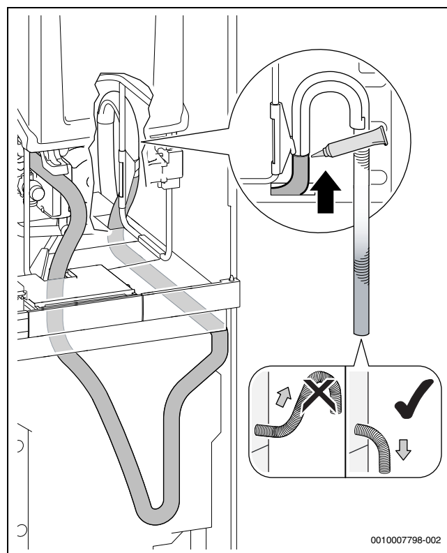
Bild 55 Siphonschlauch am Endstück einstecken
