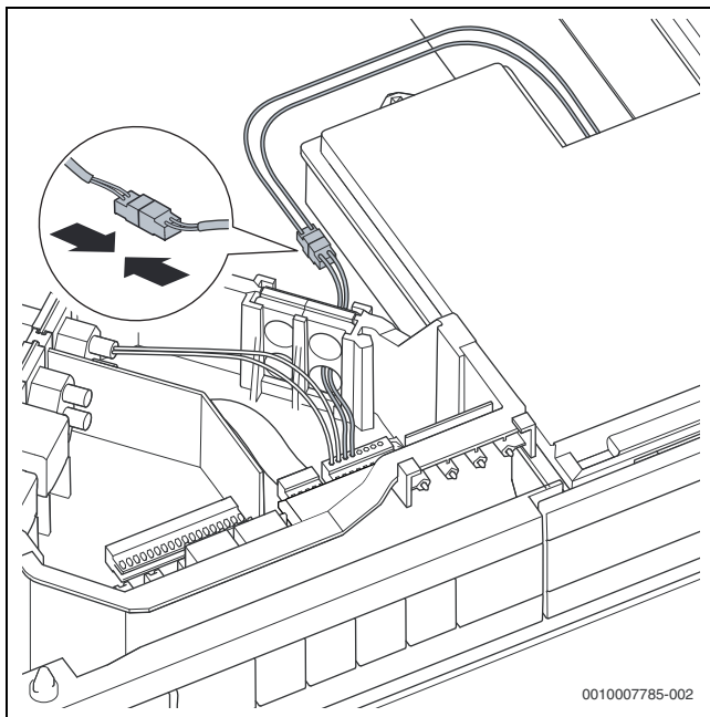
Bild 66 Schublade für den Regler an der Anschlussbox anschließen
