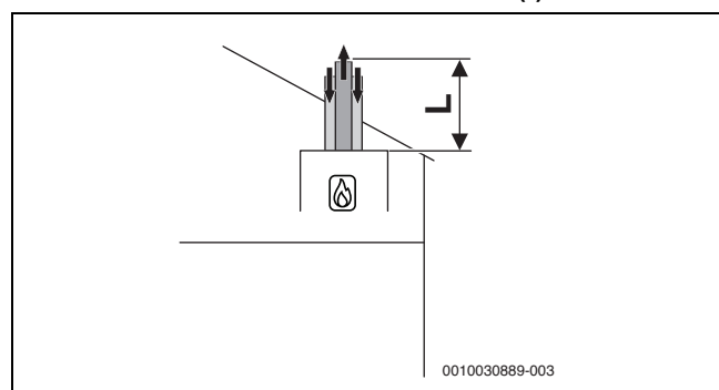
Bild 25 Vertikale konzentrische Luft-Abgas-Führung nach C 33x
