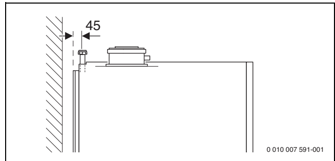
Bild 8 Anschlussmaße des Zubehörs AS-V1/Vertikales Anschluss-Set (Maße in mm)
