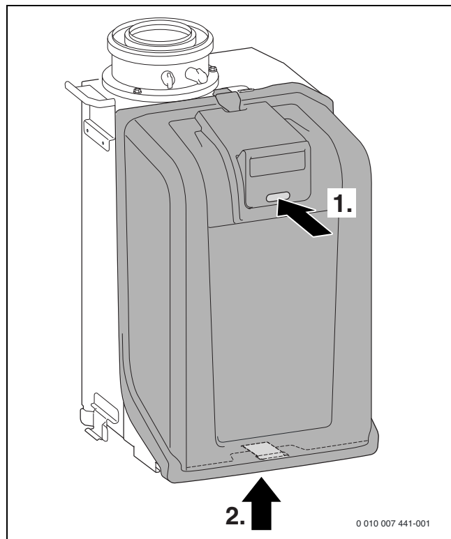
Bild 195 Brennerhaube abnehmen
