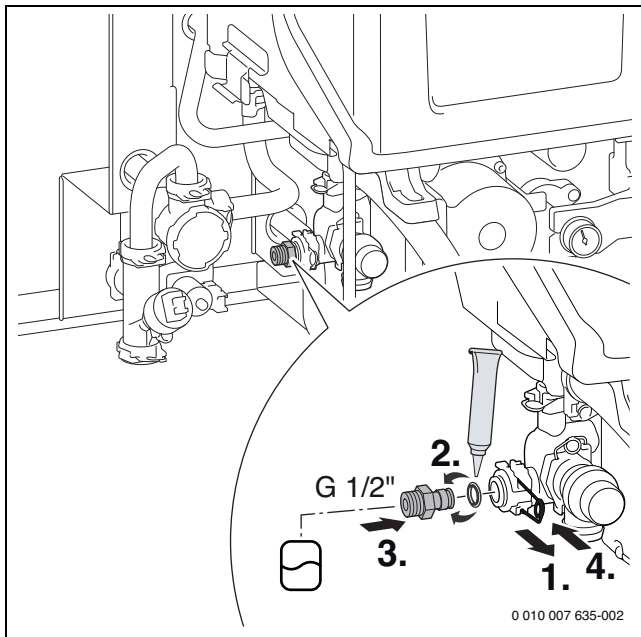
Bild 139 Verbindungsstück für den bauseitigen Anschluss eines externen Ausdehnungsgefäßes montieren
