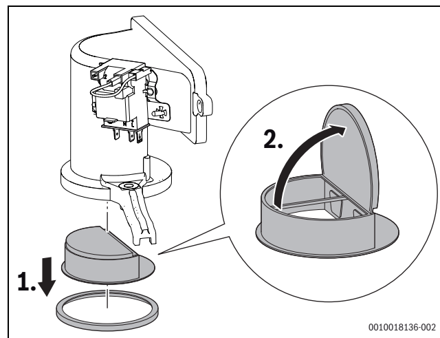
Bild 213 Rückschlagklappe in der Mischeinrichtung
