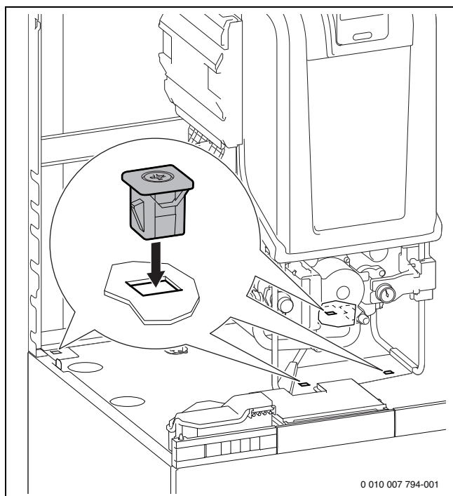
Bild 52 Gerät mit den 4 mitgelieferten Clips auf dem Speicher fixieren
