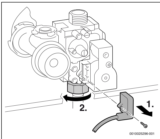
Bild 216 Stecker abziehen und Überwurfmutter lösen
