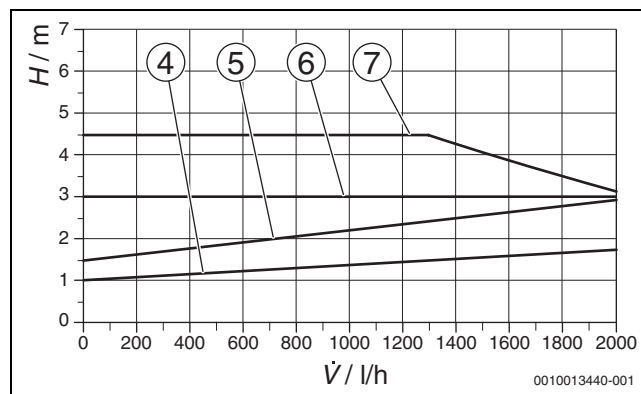
Bild 228 Pumpenkennlinien für Proportionaldruck und Konstantdruck
