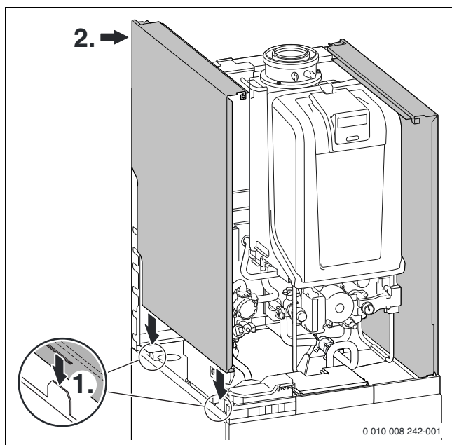
Bild 187 Rechte und linke Verkleidung montieren
