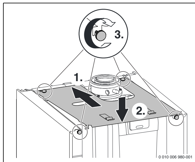
Bild 188 Obere Verkleidung nach hinten schieben und mit den 4 Schrauben vorne und hinten befestigen
