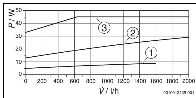
Bild 229 Leistungsaufnahme für die Pumpenstufen I bis III
