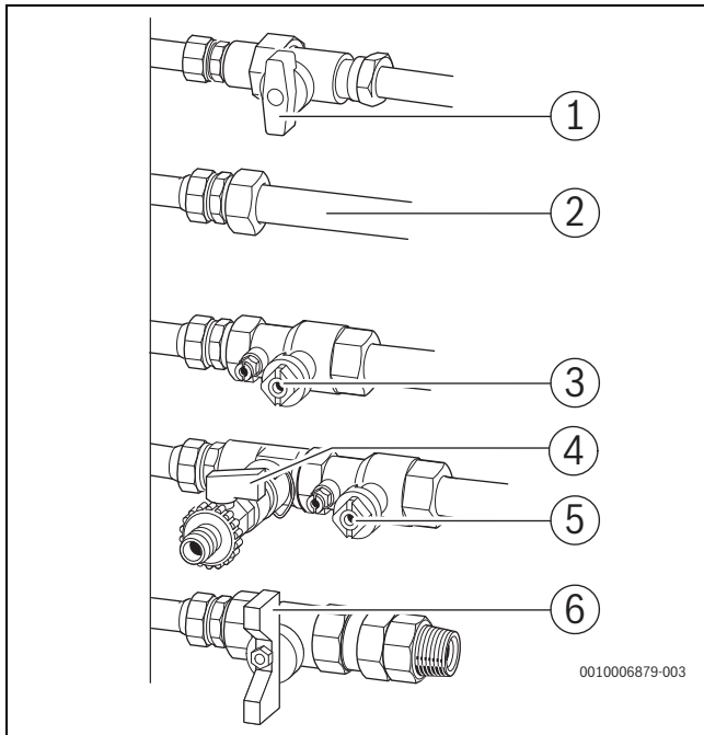
Bild 177 Gas- und wasserseitige Anschlüsse (Beispiel: Anschlusszubehör waagrecht rechts)
