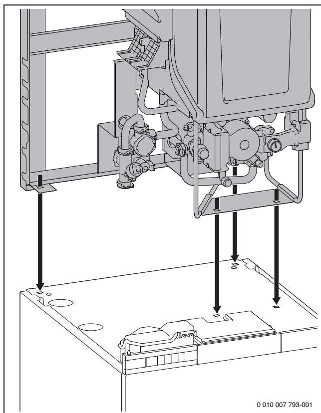
Bild 51 Gerät auf dem Speicher aufsetzen
