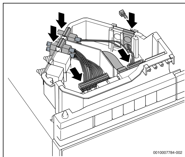
Bild 64 Steuergerät an der Anschlussbox anschließen
