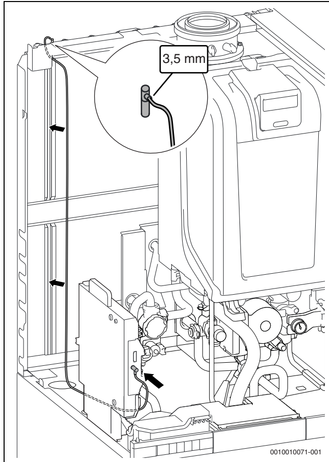
Bild 184 Anschluss und Verlegung des Kabels an Buderus Logamatic web KM100
