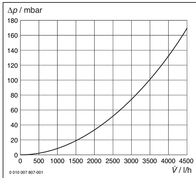
Bild 224 Druckverlust-Diagramm gemischter Heizkreis (HK2)
