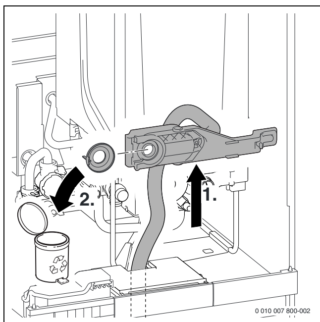
Bild 53 Schmutzfänger aus der Wartungsposition abnehmen und Schutzdeckel abnehmen
