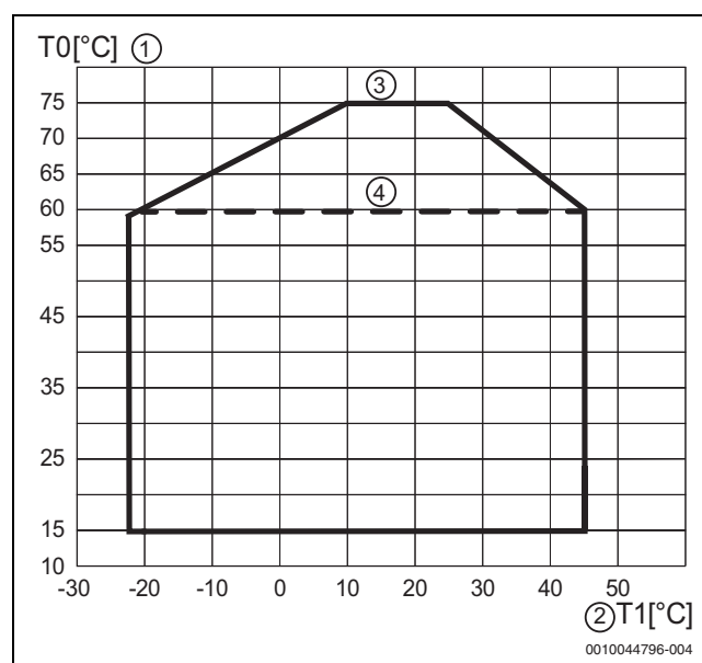
Bild 4 Wärmepumpe im Heizbetrieb ohne Zuheizter
