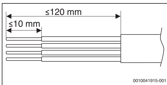
Bild 33 Abisolierung CAN-BUS
