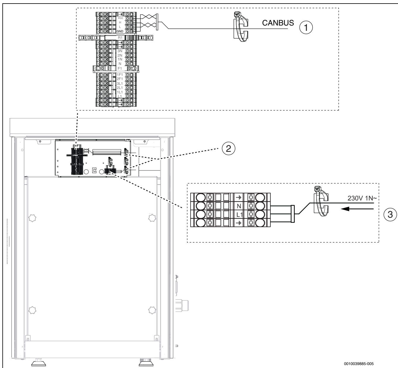
Bild 35 Klemmenkasten
