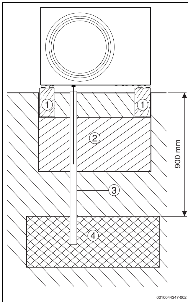
Bild 27 Kondensatableitung in Kiesbett
