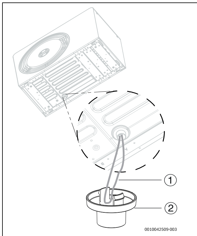
Bild 25 Installation des Ablaufstutzens
