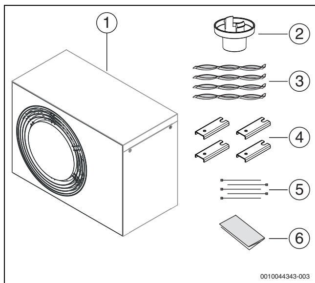
Bild 1 Lieferumfang
