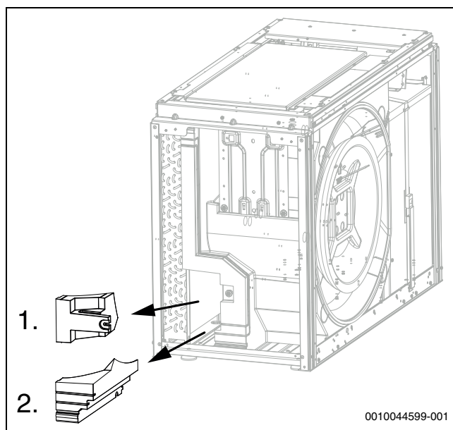
Bild 39 EPP-Segmente
