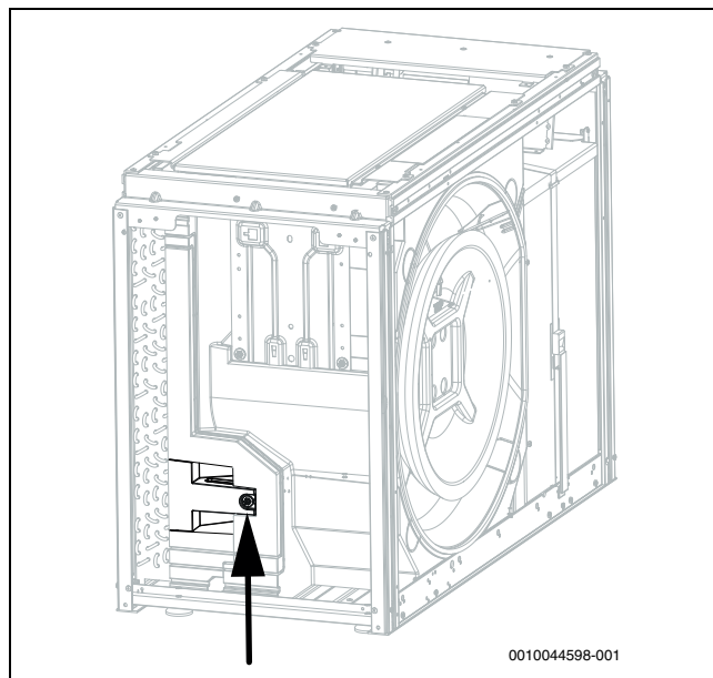
Bild 38 Abschrauben
