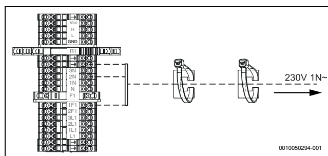
Bild 37 Heizkabelanschluss (Zubehör)
