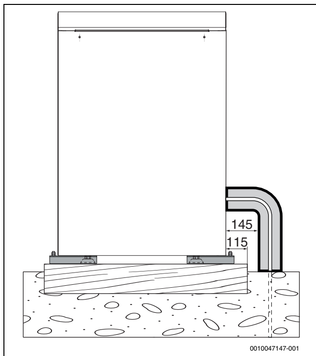
Bild 20 Montageset, Seitenansicht
