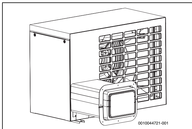
Bild 21 Montageset, Wandmontage
