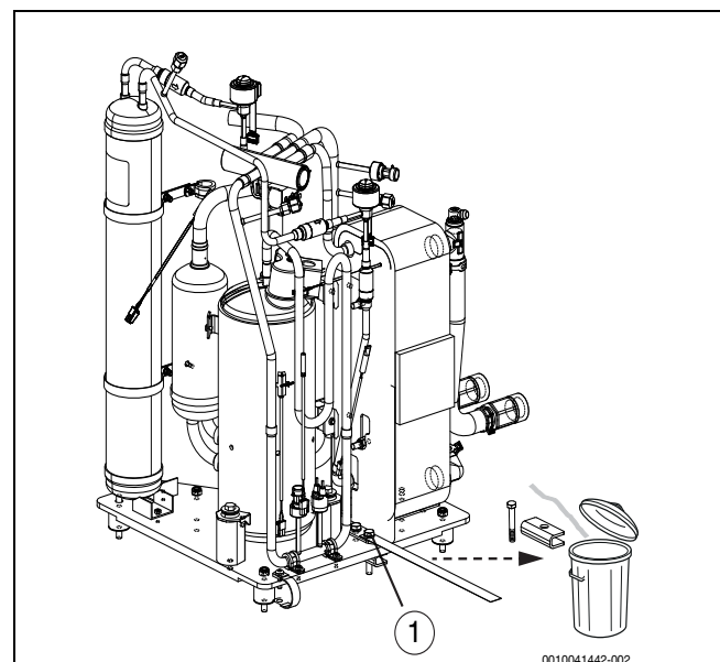
Bild 38 Transportsicherung
