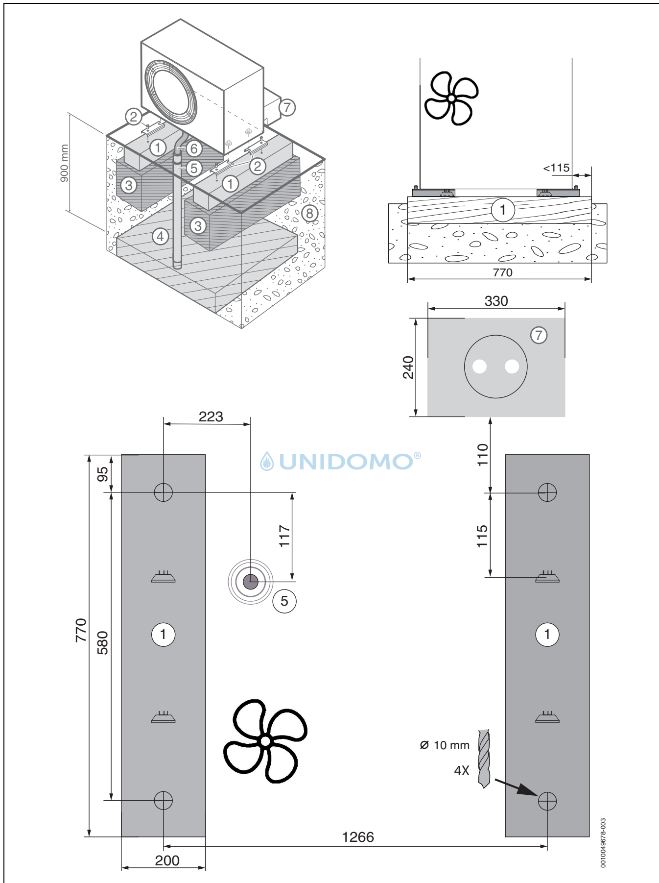
Bild 29 Fundamentplan, Alternative 1
