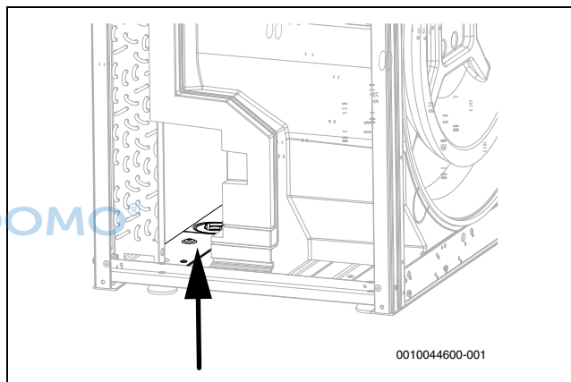
Bild 47 Auffangwanne reinigen
