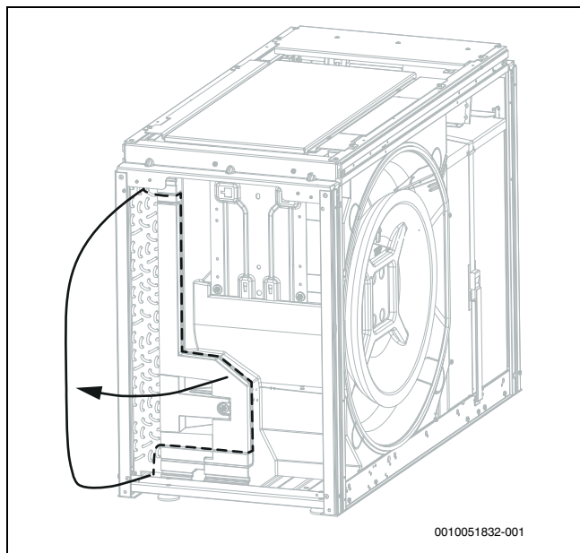
Bild 46 EPP-Segmente
