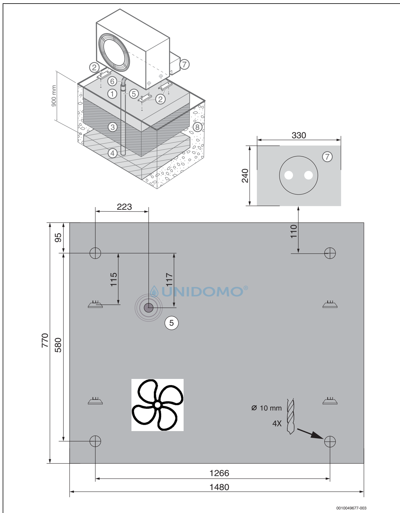
Bild 30 Fundamentplan, Alternative 2
