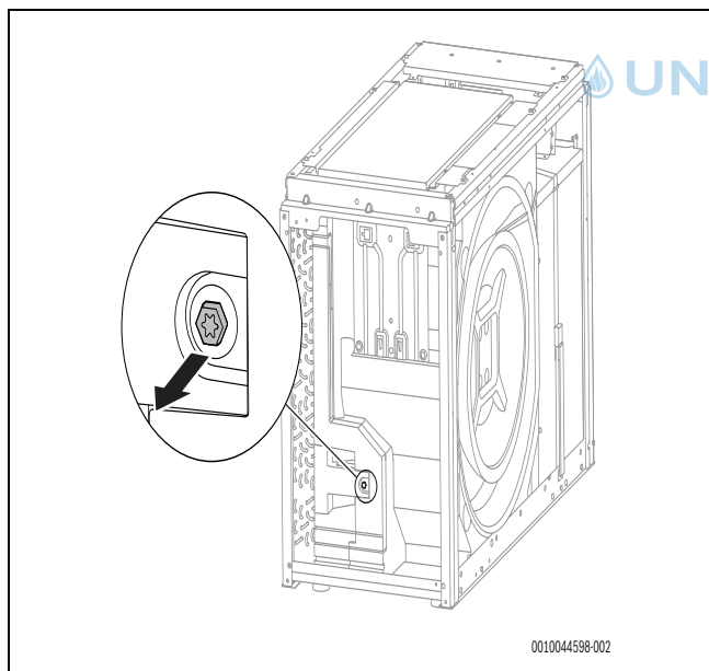
Bild 45 Abschrauben
