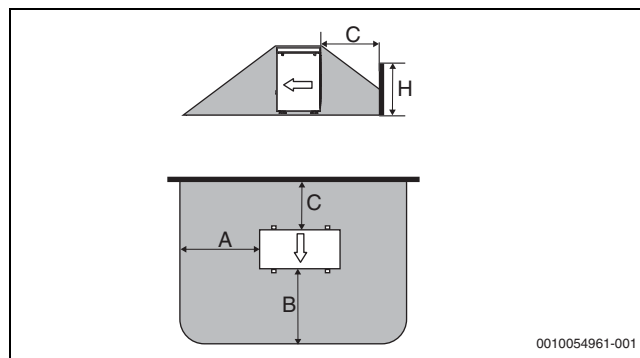
Bild 13 Schutzbereich mit Barriere hinter der freistehenden Wärmepumpe
