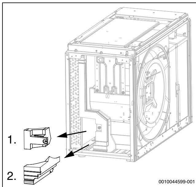
Bild 46 EPP-Segmente
