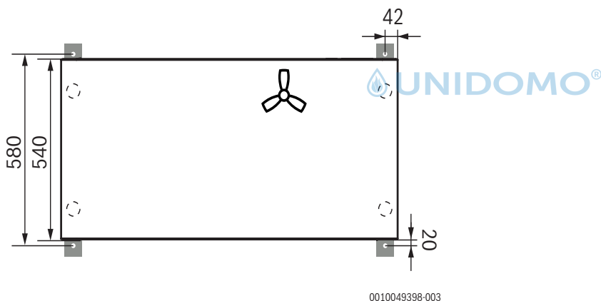
Bild 5 Abmessungen der Wärmepumpe, Oberseite
