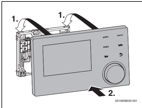
Bild 5 Bedieneinheit einhängen
