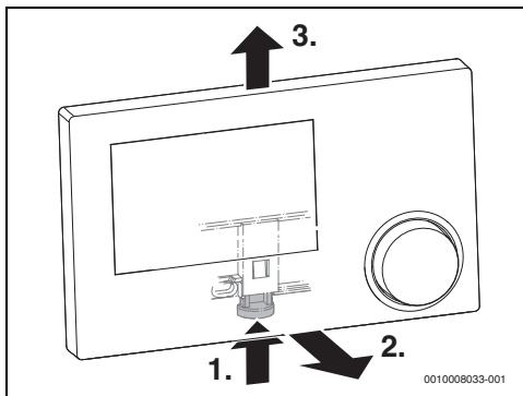
Bild 6 Bedieneinheit abnehmen
