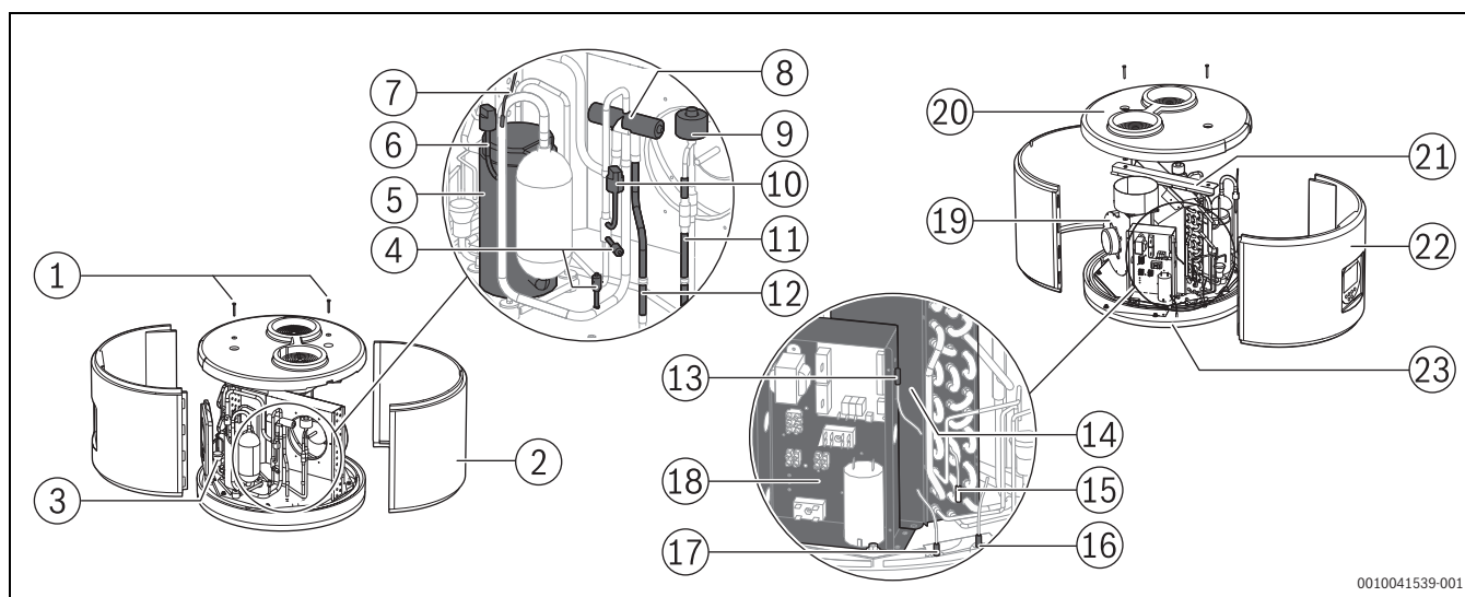
Bild 4 Produktübersicht
