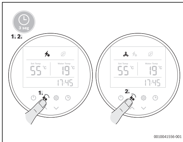
Bild 23 Einstellung Betriebsart "Nur elektrischer Zuheizter"
