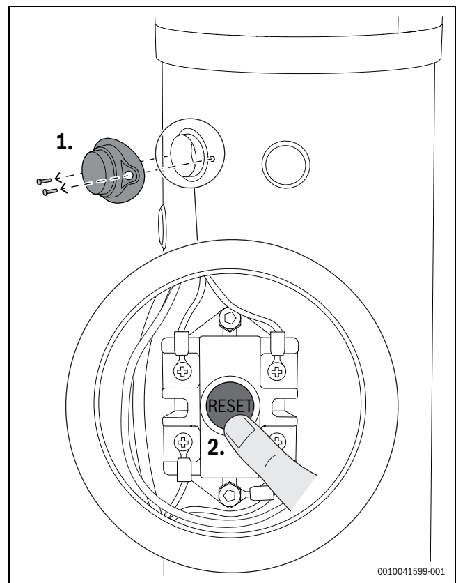
Bild 31 Thermostat-Reset
