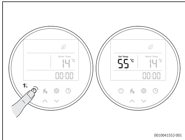
Bild 15 Standby-Funktion
