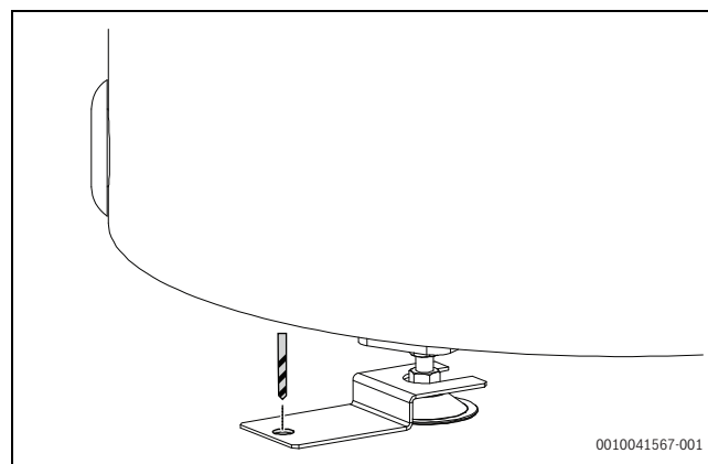
Bild 8 Befestigungswinkel
