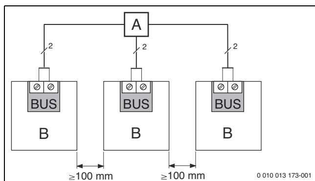
Bild 15 Verteilerdose anschließen
