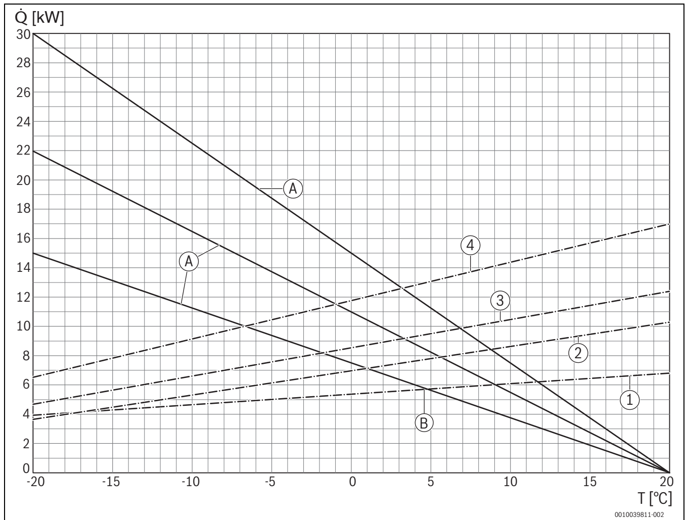
Bild 31 Diagramm zu Tab. 16; Zur Bestimmung der Bivalenzpunkte bei 55 °C Vorlauftemperatur
