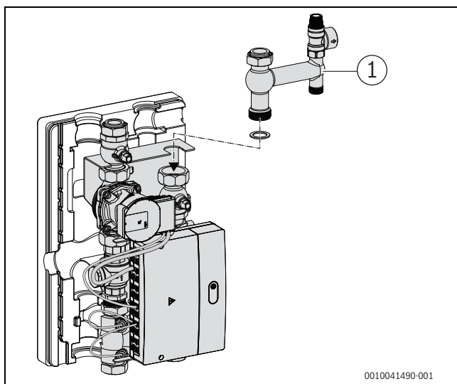
Bild 7 Sicherheitsventil montieren
