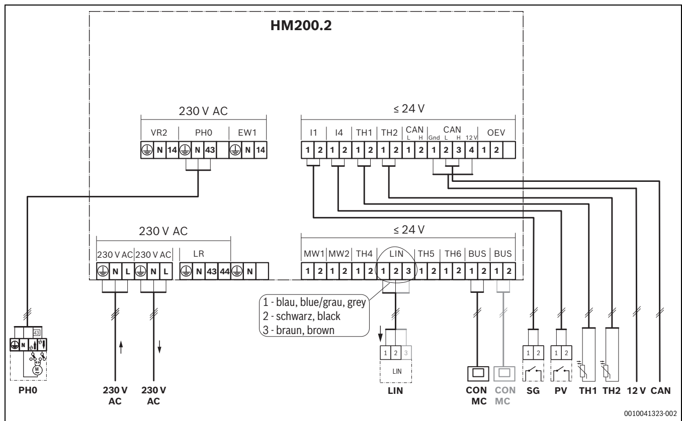
Bild 23 Überblick Anschlussklemmenbelegung
