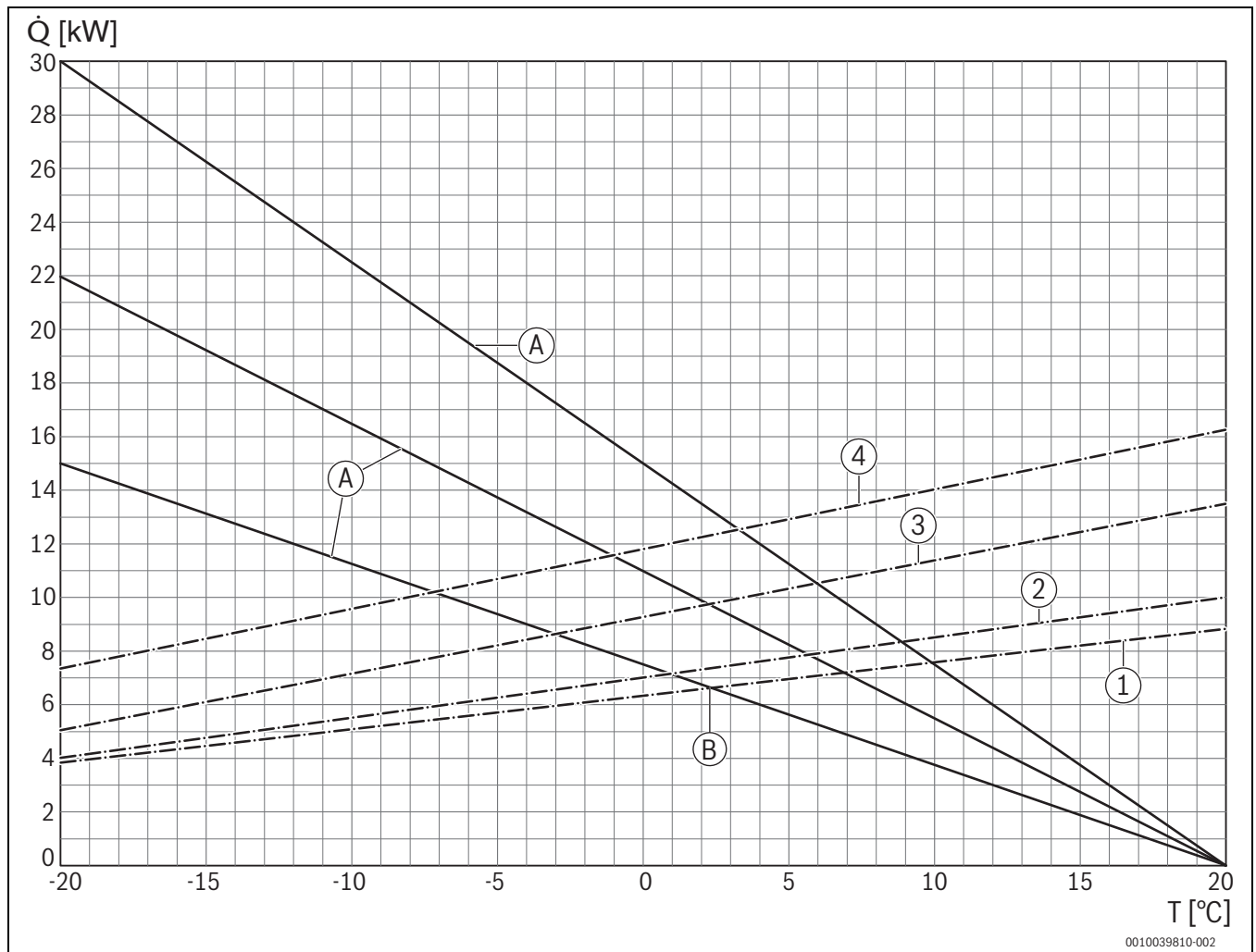
Bild 29 Diagramm zu Tab. 14; Zur Bestimmung der Bivalenzpunkte bei 45 °C Vorlauftemperatur
