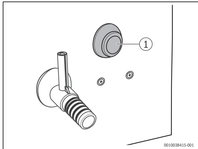
Bild 14 Durchführungstülle montiert
