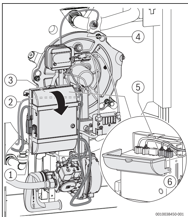
Bild 20 Steckverbinder anschließen
