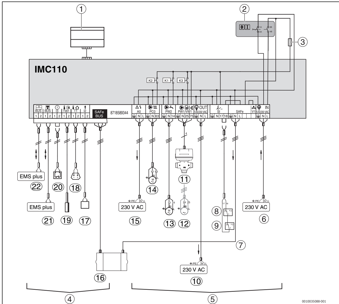
Bild 56 Anschlussplan Regelgerät IMC110
