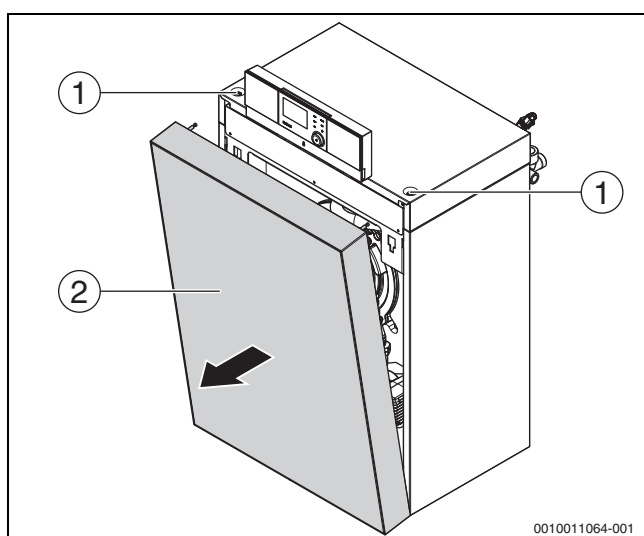
Bild 5 Kesselvorderwand demontieren
