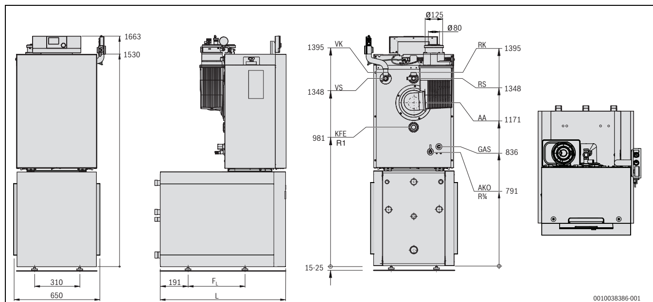
Bild 4 Abmessungen und Anschlüsse Logano plus KB195i Gas mit Logamatic und L135...L200.3 RS (Maße in mm)
