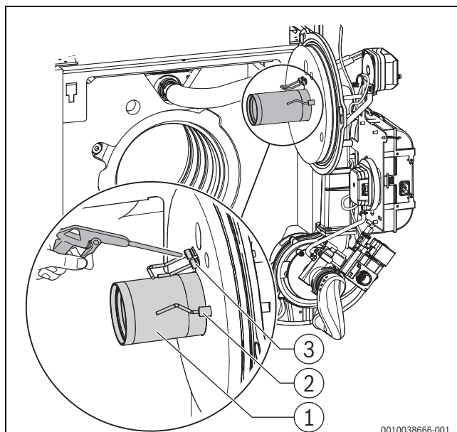
Bild 45 Brennerrohr mit Druckluft ausblasen
