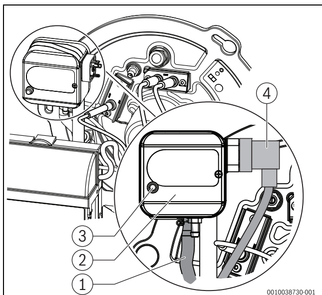
Bild 51 Feuerraum-Druckwächter
