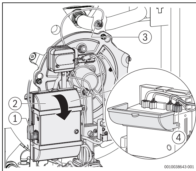
Bild 38 Steckverbinder lösen
