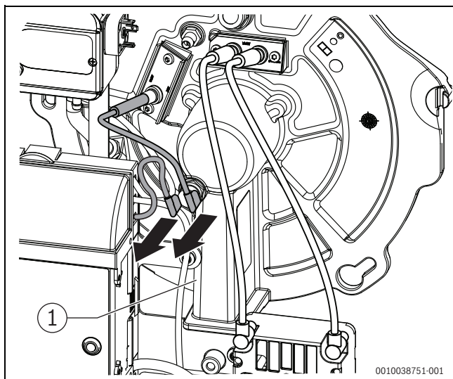
Bild 53 Stecker am Temperaturwächter abziehen
