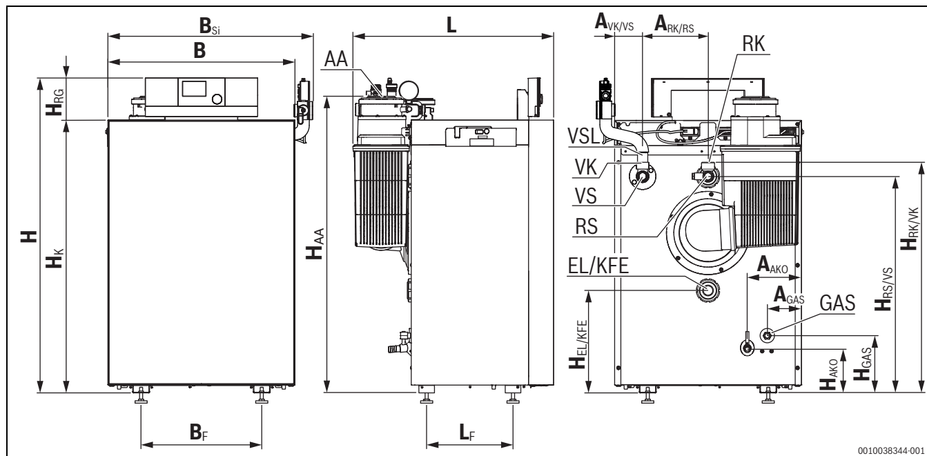
Bild 3 Abmessungen und Anschlüsse für KB195i-22 Gas (Maße in mm)
