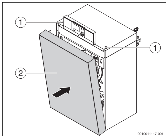
Bild 33 Kesselvorderwand montieren
