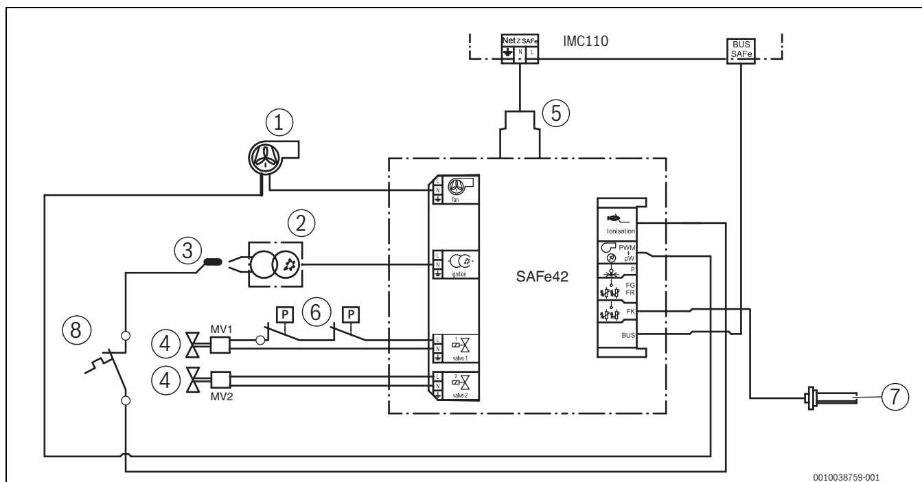
Bild 57 Anschlussplan Feuerungsautomat
