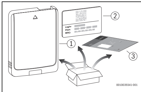
Bild 3 Lieferumfang
