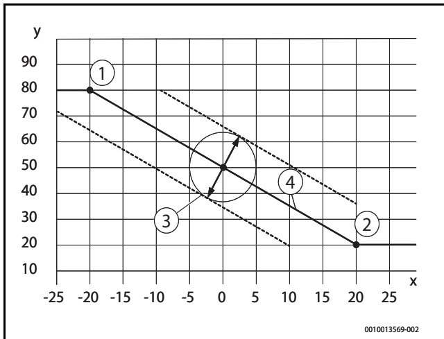
Bild 4 Außentemperaturgeführte Heizkurve
