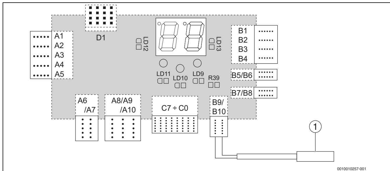
Bild 32 Anschluss eines externen Temperatursensors für die minimale Raumtemperatur oder eines zusätzlichen Raumthermostats
