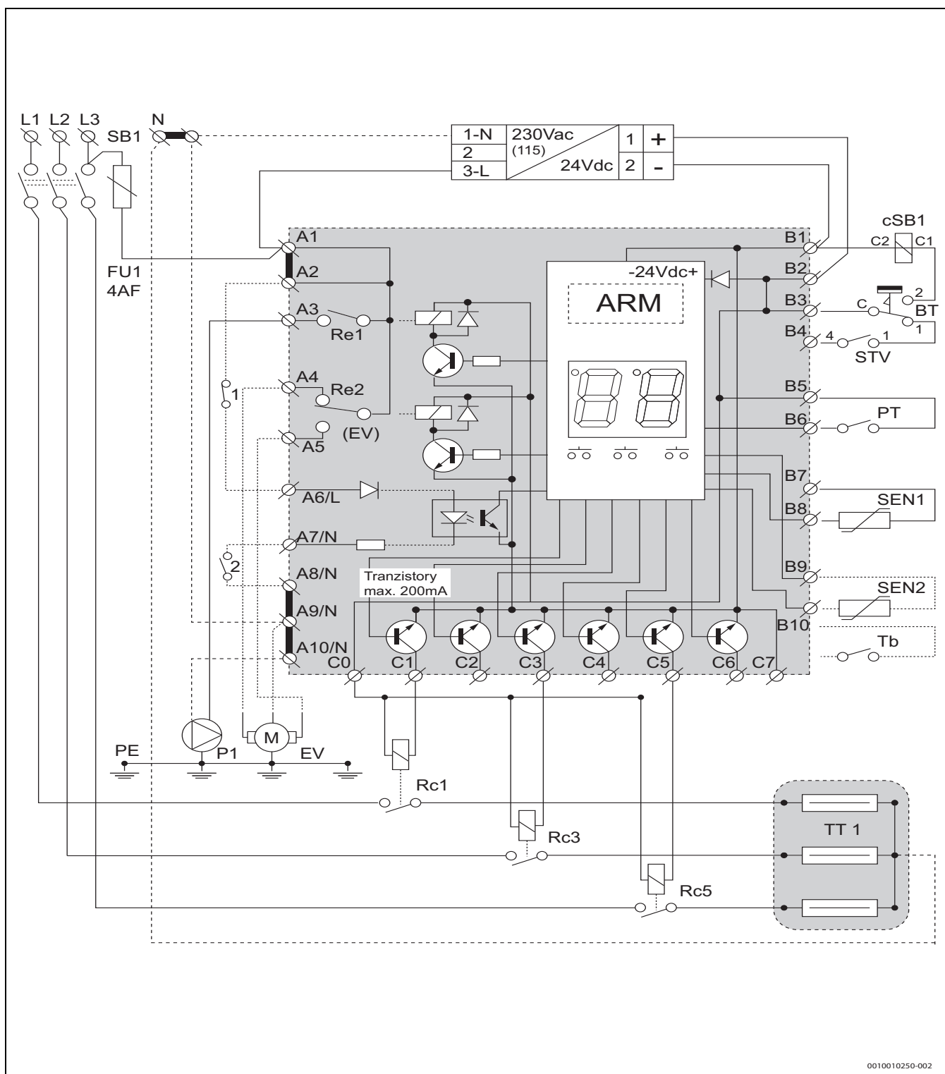
Bild 20 Bedienschema des Heizgeräts Logamax E156 (4-12 kW), 3x 400/230 V AC
