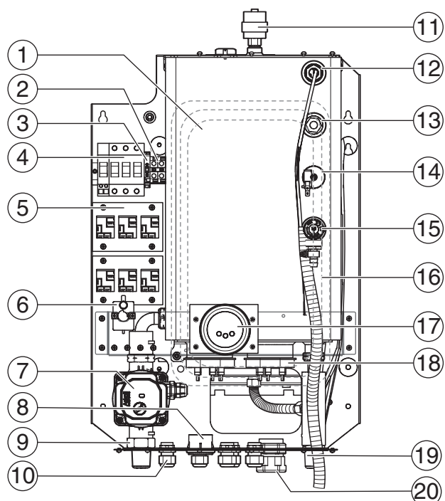
Bild 2 Funktionselemente des Heizgeräts Logamax E156 15-24 kW
