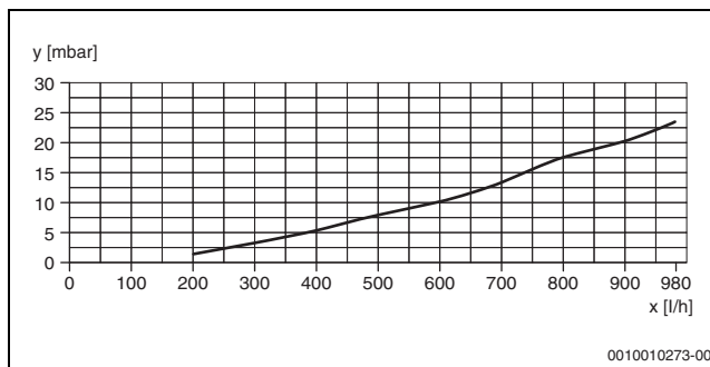
Bild 38 Hydraulischer Widerstand Logamax E156 15...24 kW
