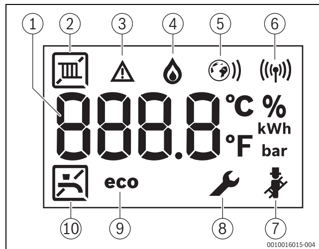
Bild 5 Displayanzeigen
