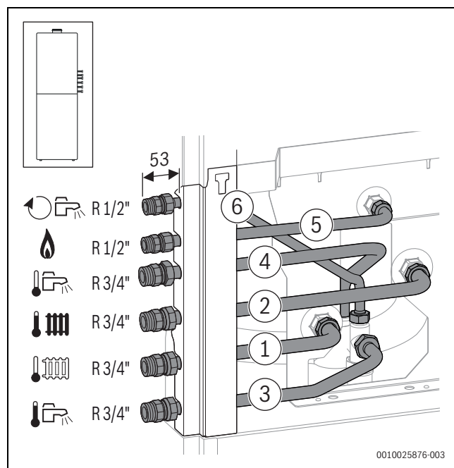
Bild 54 Zubehör CS 10 auf der rechten Seite montiert
