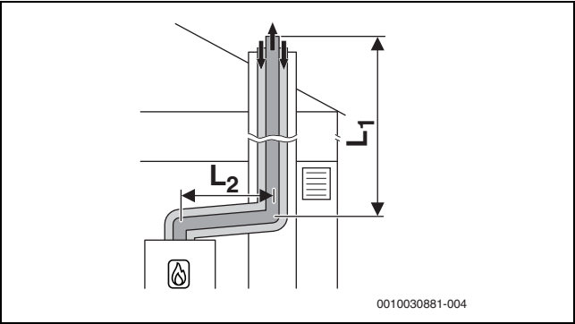
Bild 26 Konzentrische Luft-Abgas-Führung nach C 33x im Schacht
