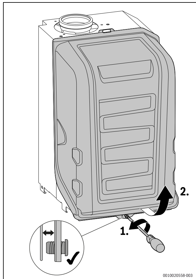
Bild 101 Brennerhaube abnehmen
