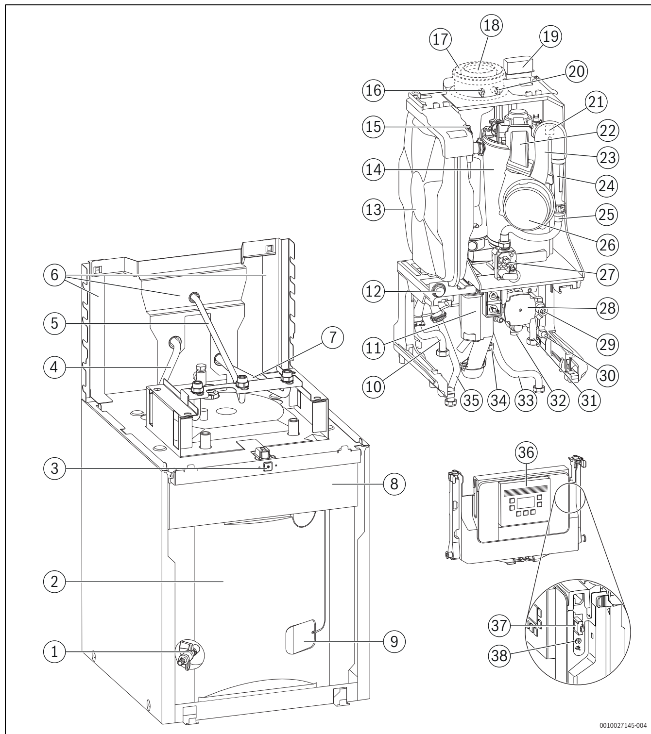
Bild 4 Produktübersicht
