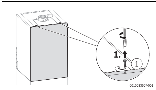
Bild 109 Sicherungsschraube lösen
