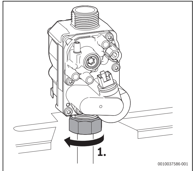
Bild 138 Überwurfmutter lösen
