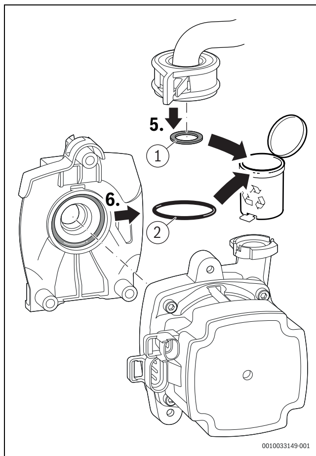
Bild 135 Dichtungen entsorgen
