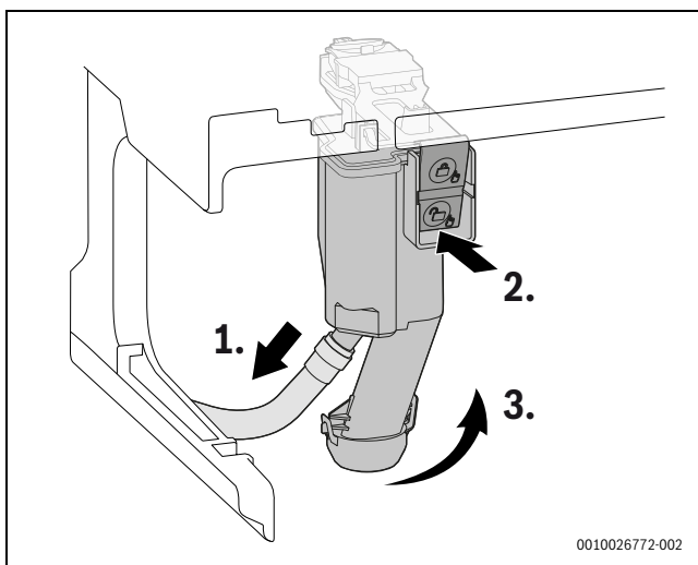
Bild 145 Kondensatsiphon ausbauen
