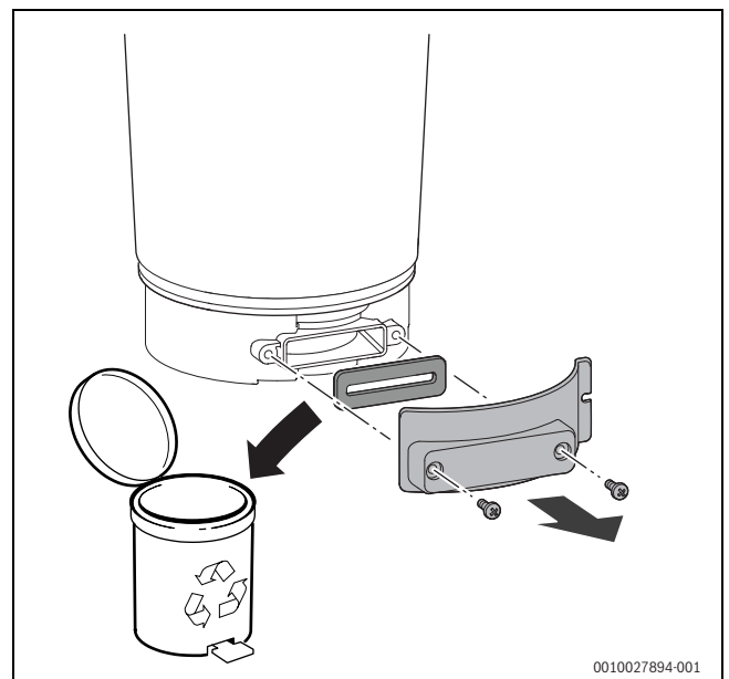
Bild 127 Prüföffnung öffnen
