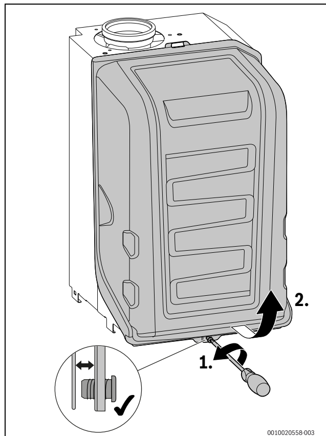
Bild 76 Brennerhaube abnehmen
