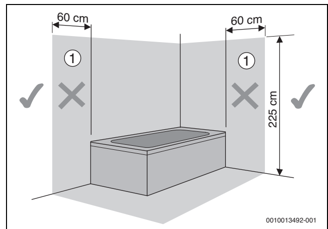
Bild 45 Schutzbereiche
