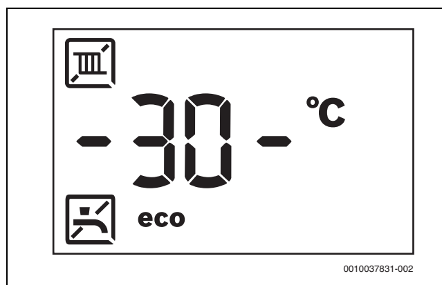
Bild 100 Vorlauftemperatur steht zwischen blinkenden Strichen
