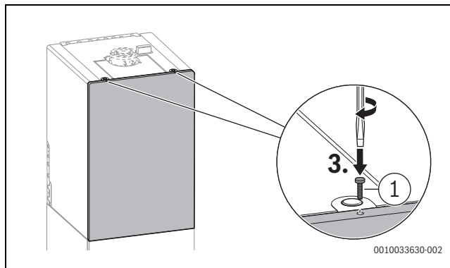
Bild 91 Vorderteil der Geräteverkleidung mit Schraube aus Lieferumfang sichern
