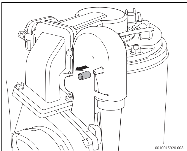
Bild 113 Messstutzen an der Mischeinrichtung
