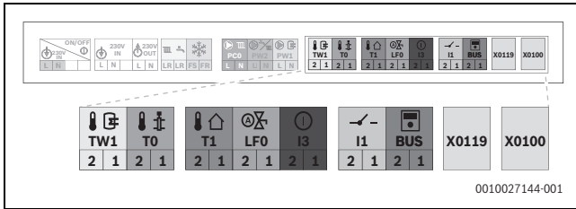
Bild 85 Niederspannungsbereich: Klemmleiste
