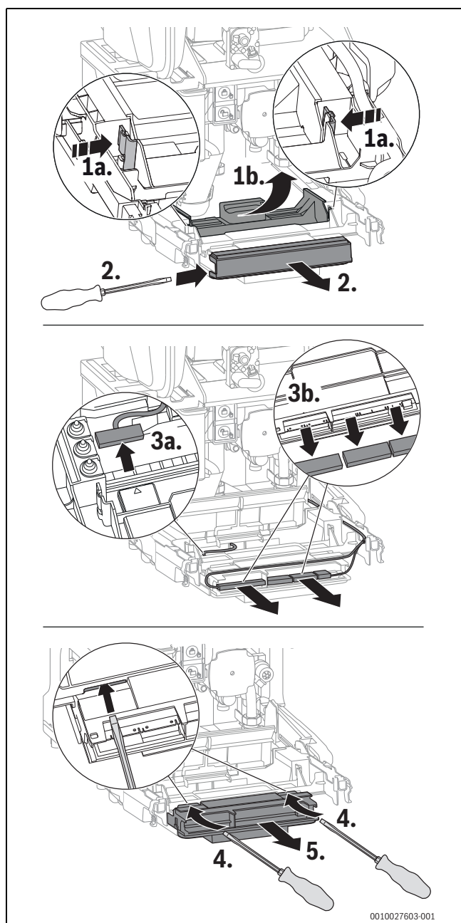
Bild 144 Steuergerät herausnehmen
