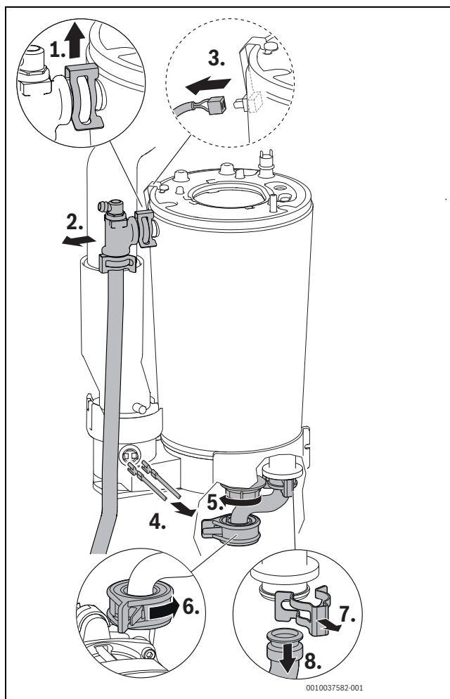
Bild 130 Vorlaufrohr lösen, Kabel abziehen und Rücklaufrohr lösen
