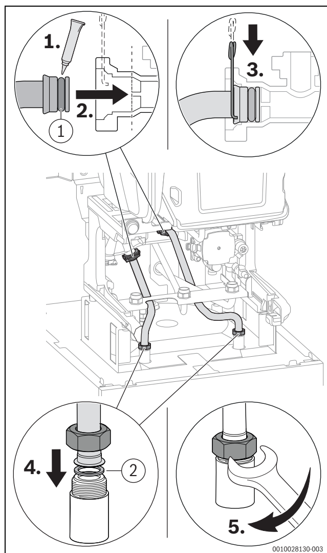
Bild 62 Vorlaufrohr und Rücklaufrohr zum Rohrwendelspeicher anschließen
