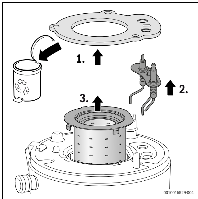
Bild 121 Brenner herausnehmen
