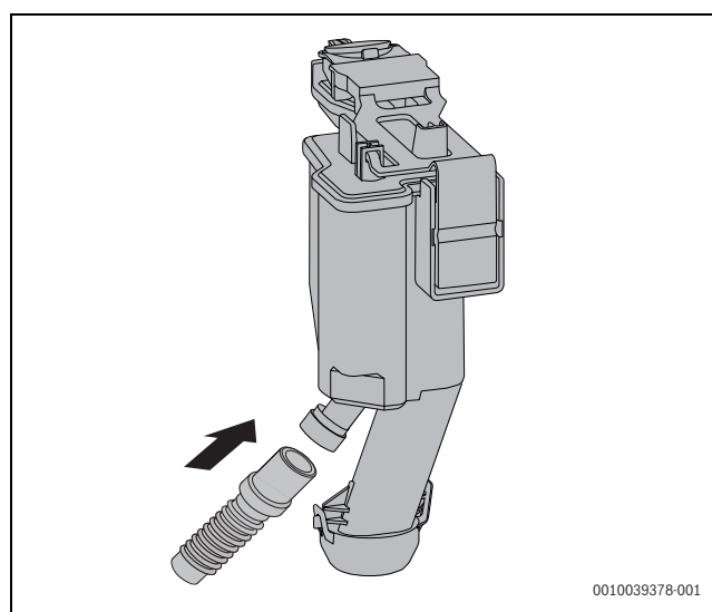
Bild 70 Schlauch am Kondensatsiphon anschließen
