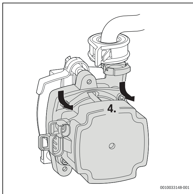
Bild 134 Heizungspumpe abnehmen
