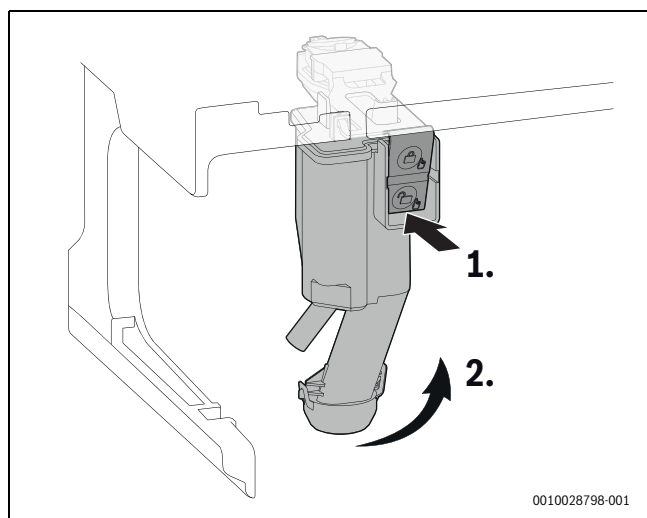
Bild 61 Kondensatsiphon herausnehmen
