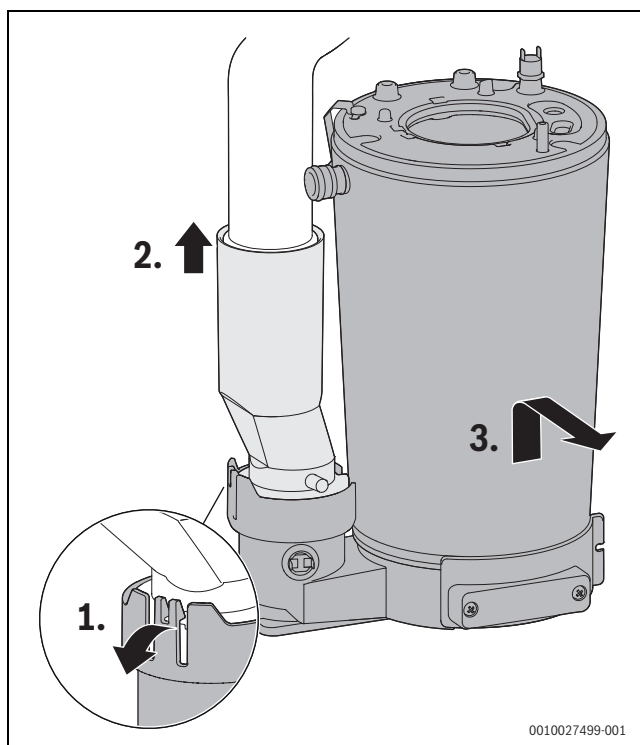
Bild 131 Wärmeblock ausbauen
