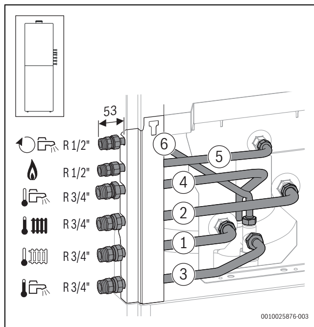
Bild 12 Ansicht von der Rückseite (Maß in mm): Zubehör CS 10 auf der rechten Seite montiert
