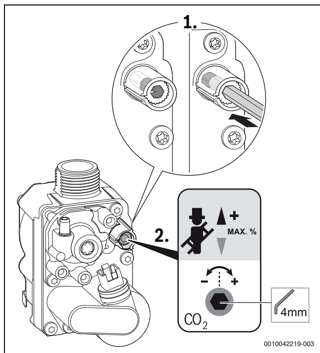
Bild 104 CO 2 /O 2 -Gehalt bei maximaler Nennwärmeleistung einstellen
