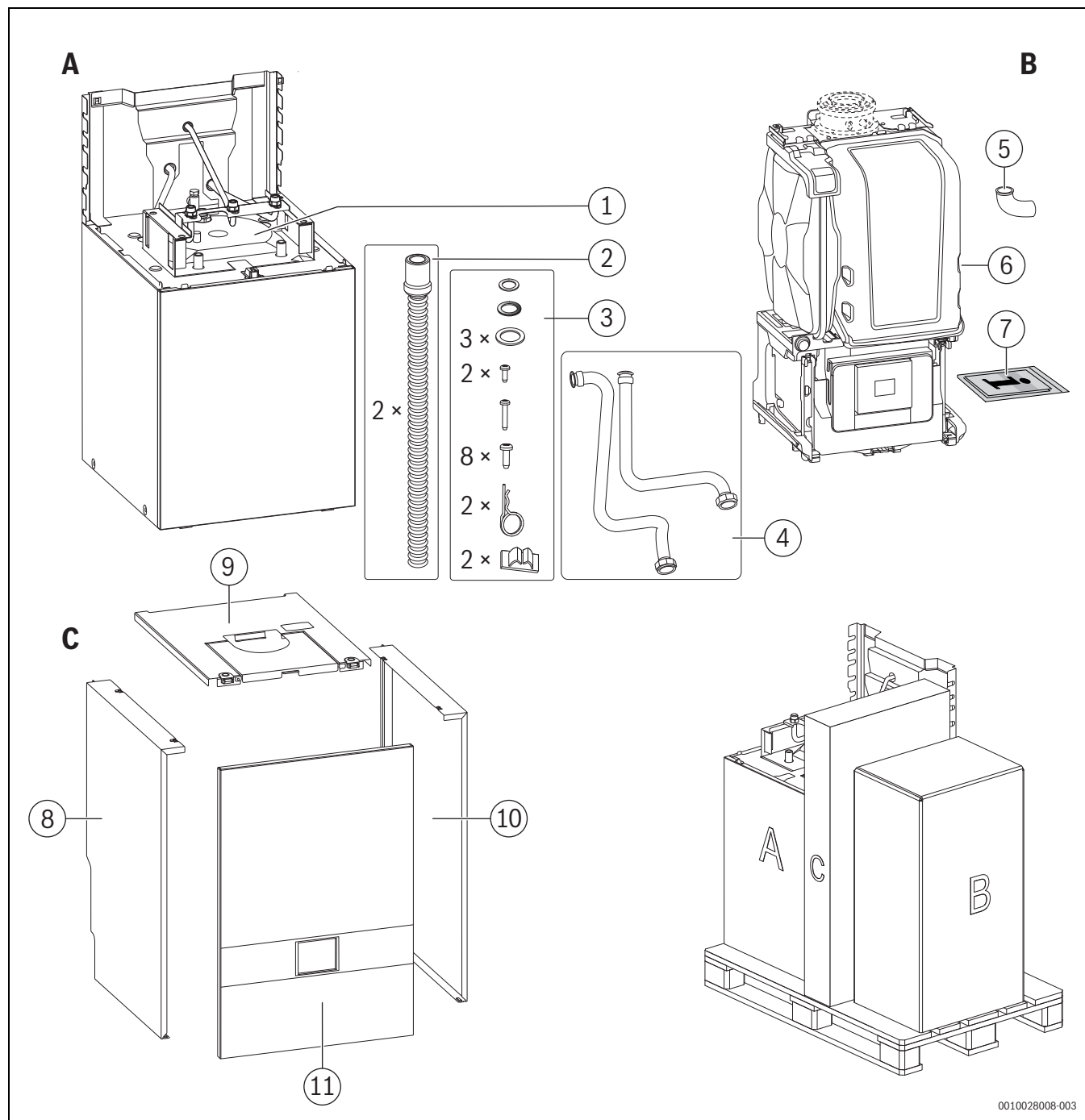
Bild 3 Lieferumfang
