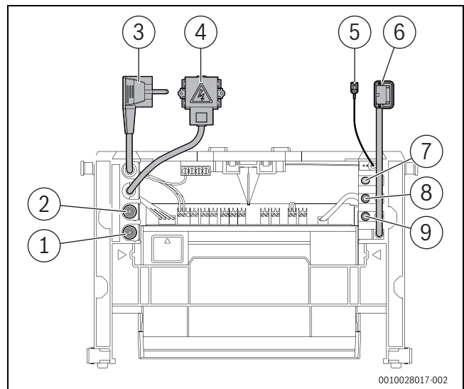
Bild 82 Lieferzustand des Steuergeräts mit angeschlossenen Komponenten
