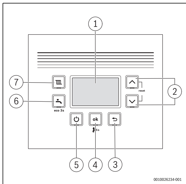
Bild 4 Bedienfeldübersicht
