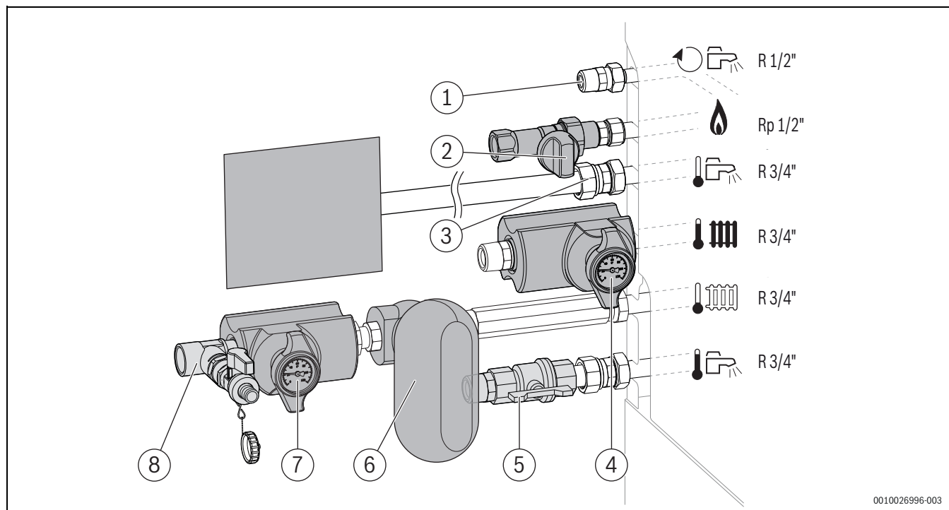
Bild 4 Beispiel: Gas- und wasserseitiger Anschluss mit dem Anschluss-Set Hähne (Zubehör CS 28-1) auf der linken Seite
