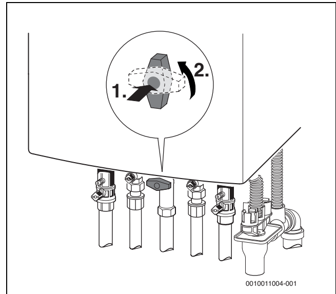
Bild 5 Gashahn öffnen
