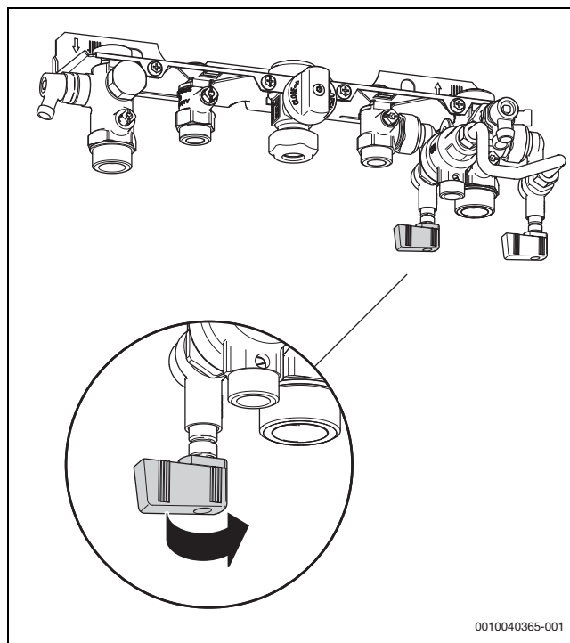
Bild 6 Füllinrichtung öffnen
