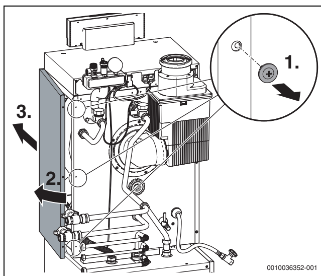
Bild 31 Seitenverkleidung demontieren
