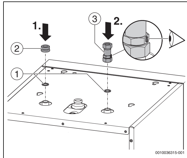
Bild 10 Verrohrung Verbindung Kessel und Speicher vorbereiten
