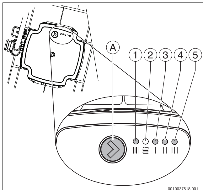
Bild 27 Einstellung der Pumpe
