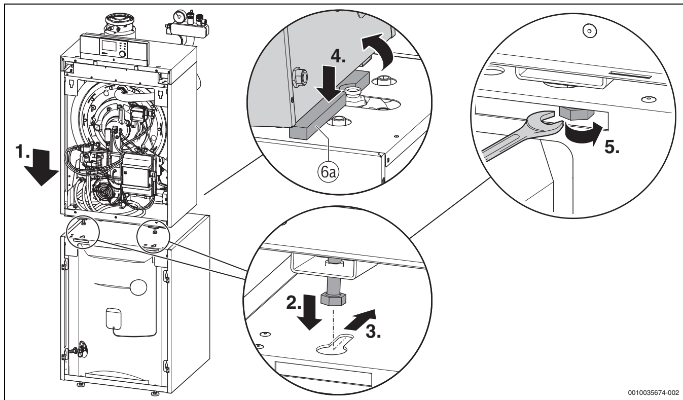
Bild 13 Kessel auf Speicher stellen
