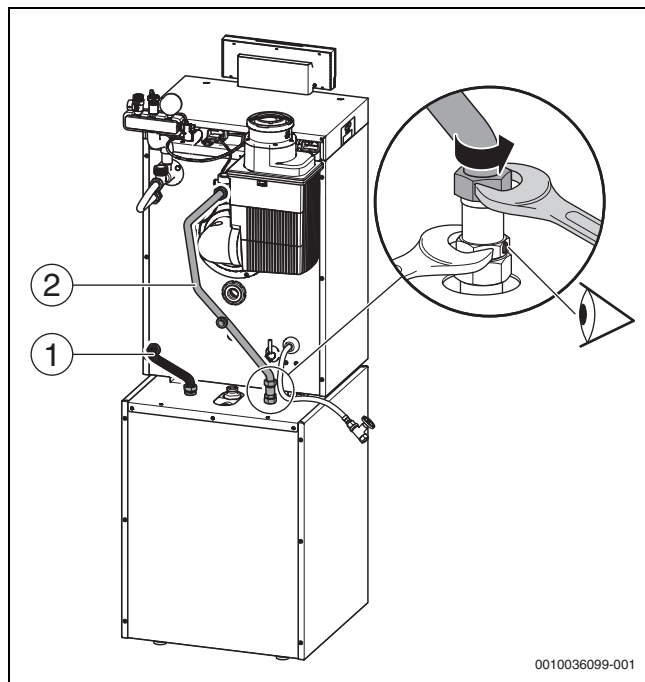
Bild 17 Rohre Verbindung Kessel und Speicher montieren
