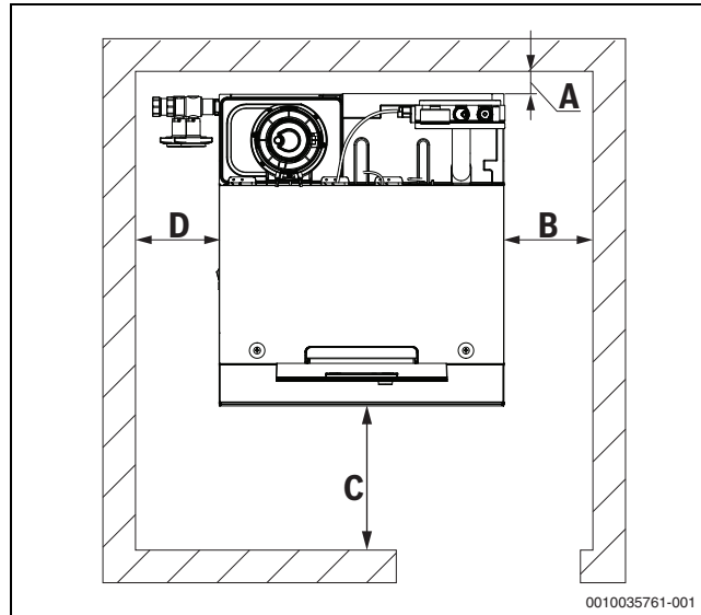
Bild 6 Wandabstände im Aufstellraum
