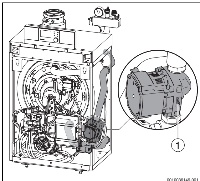
Bild 28 Pumpe
