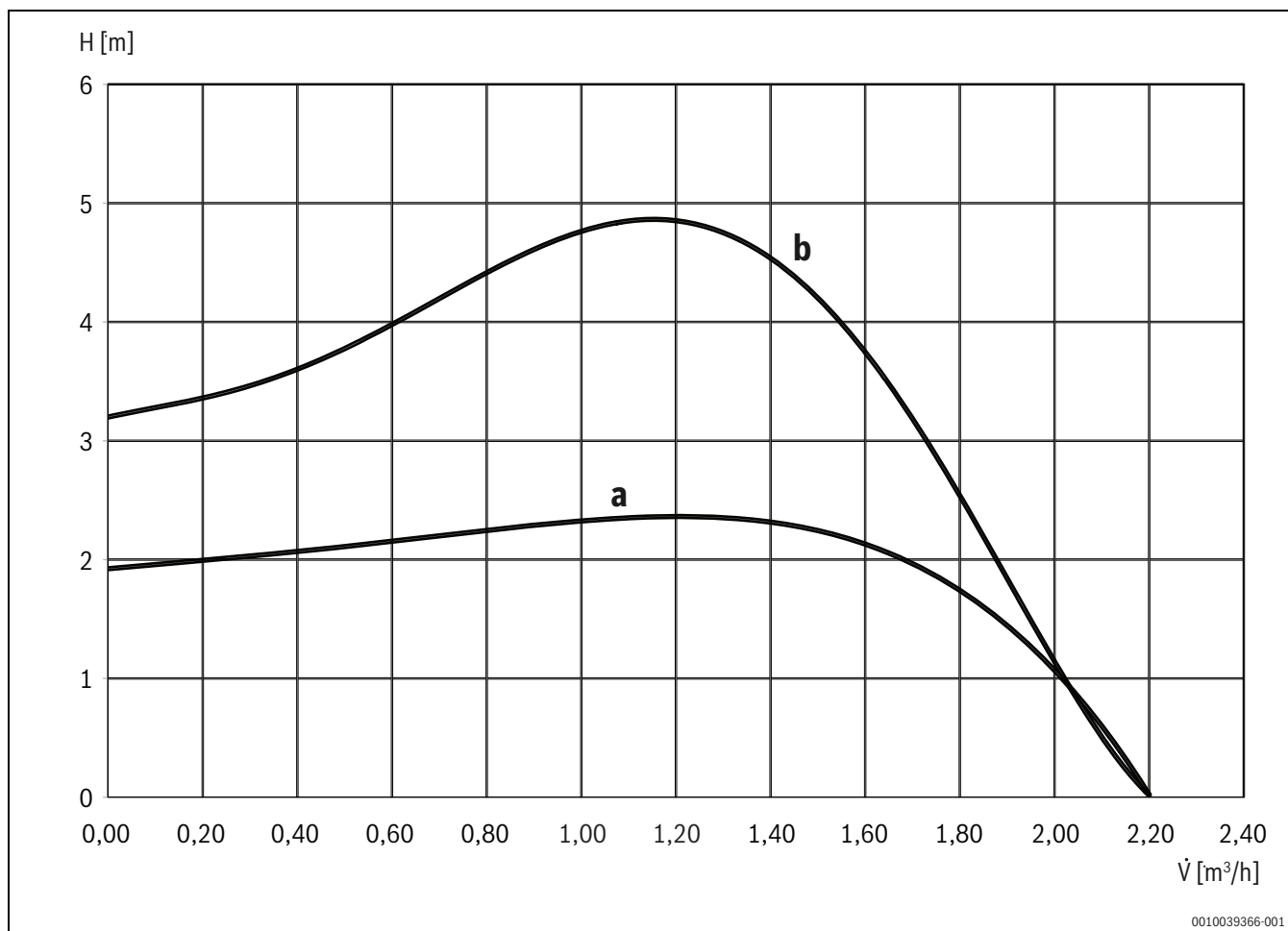
Bild 26 Restförderhöhe KB195iT-19 S120 BZ/ KB195iT-25 S120 BZ mit integrierter Hocheffizienzpumpe Grundfos UPM3 AUTO 15-70 130
