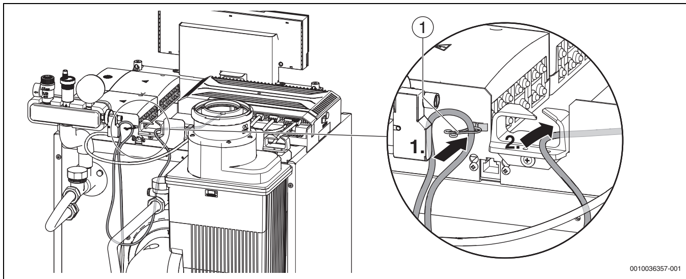
Bild 16 Fühlerkabel befestigen und einstecken (Kessel)
