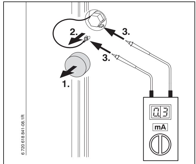
Bild 34 Schutzanode prüfen
