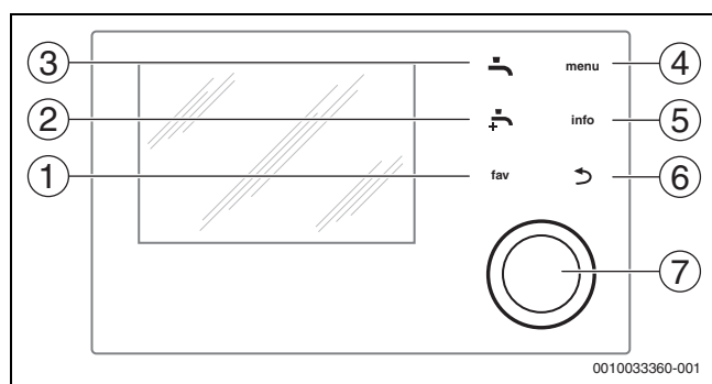
Bild 3 Bedienelemente
