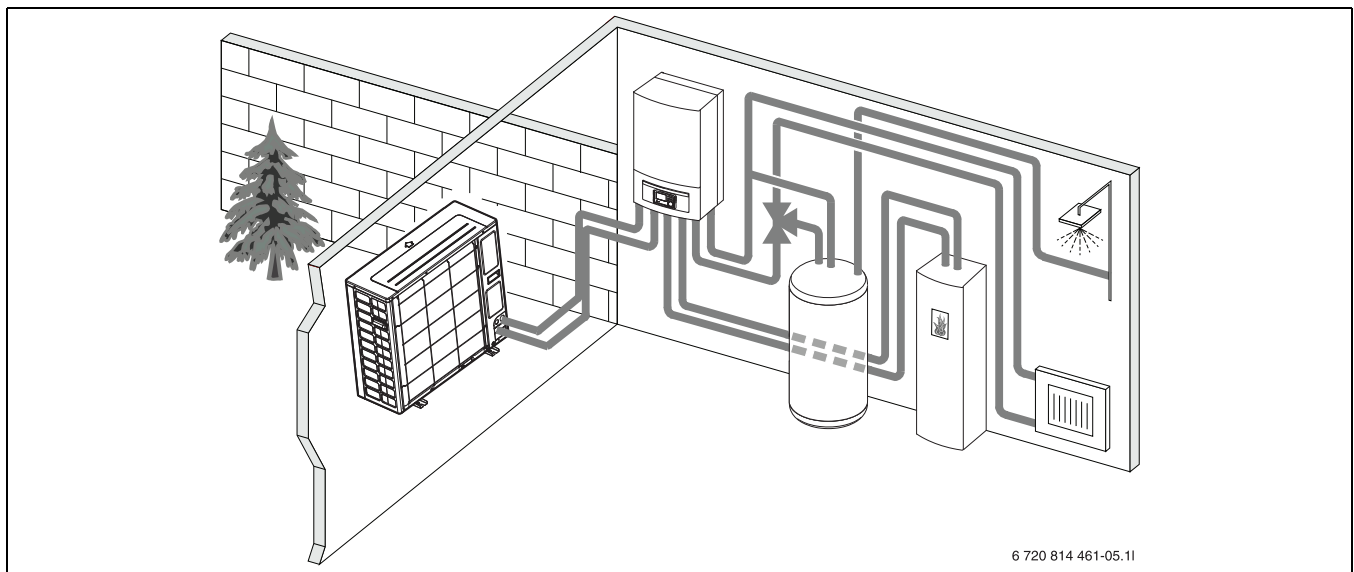
Bild 2 Wärmepumpe Außeneinheit, Inneneinheit IDUS B ohne elektrischen Zuheizer, externer Warmwasserspeicher und externer Zuheizer
