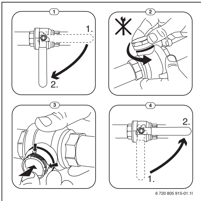
Bild 6 Siebreinigung
