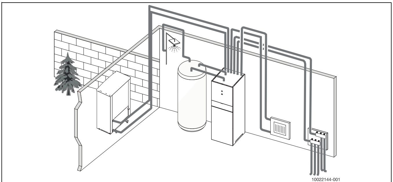
Bild 3 Wärmepumpe WLW196.2i..IR/AR, Inneneinheit IDU iTP mit integriertem Pufferspeicher und elektrischem Zuheizer, externer Warmwasserspeicher
