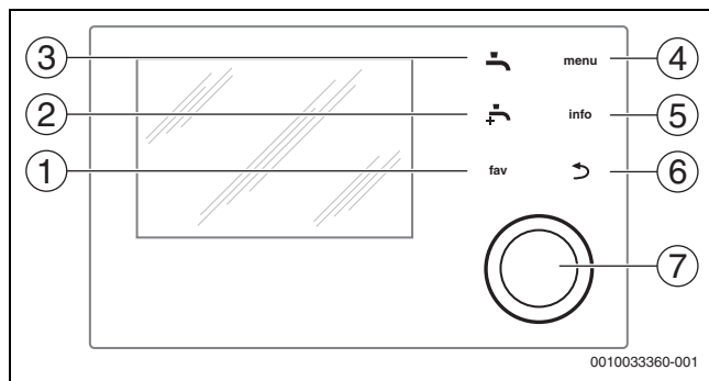
Bild 4 Bedienelemente
