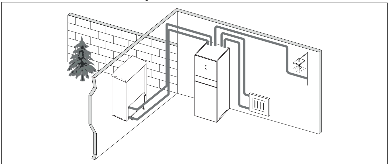
Bild 3 Wärmepumpe WLW196i.2 AR/IR, Inneneinheit IDU-..iT / IDU-..iTS mit integriertem Warmwasserspeicher und elektrischem Zuheizer
