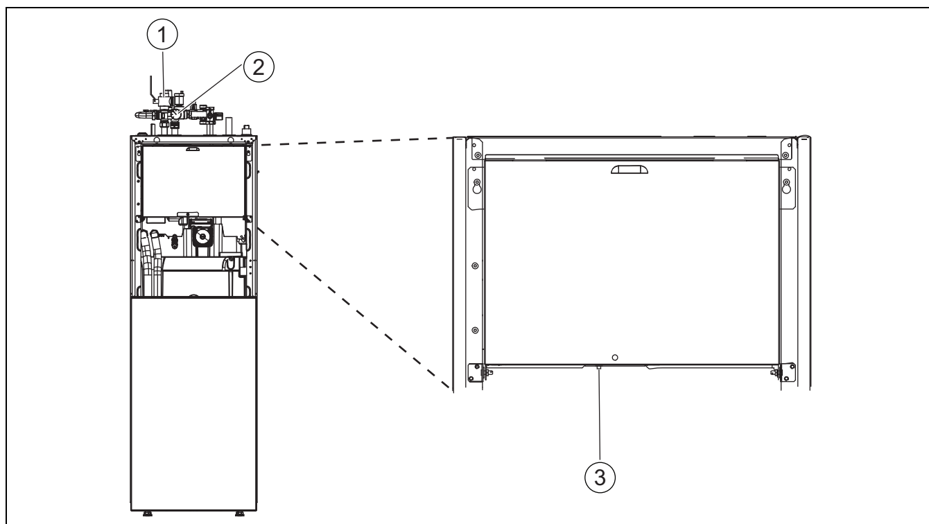
Bild 6 IDU-..iT / IDU-..iTS
