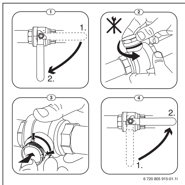
Bild 7 Siebreinigung
