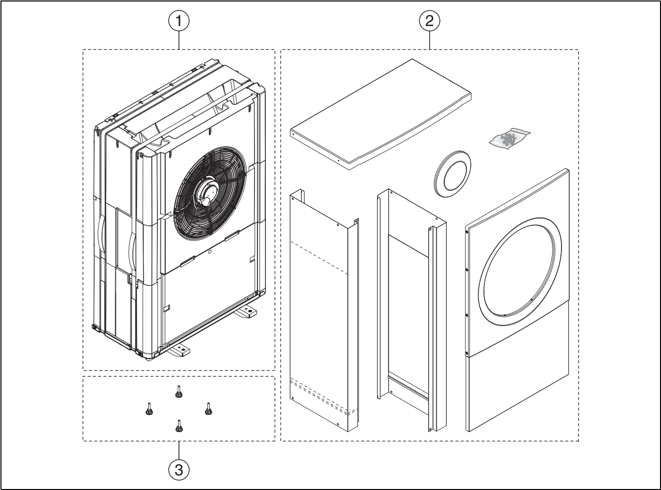
Bild 2 Lieferumfang
