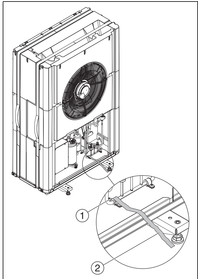
Bild 13 Transportsicherung
