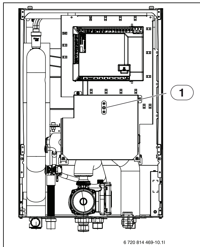
Bild 6 Inneneinheit IDUS E
