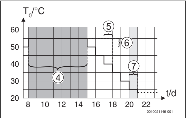
Bild 7 Ablauf der Estrich trocknung mit den Grundeinstellungen in der Abkühlphase
