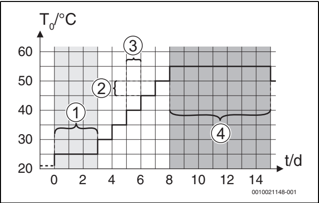
Bild 6 Ablauf der Estrich trocknung mit den Grundeinstellungen in der Aufheizphase
