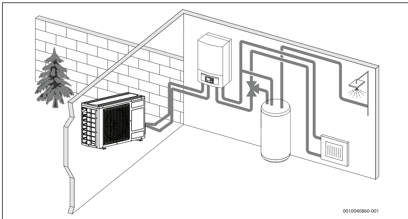
Bild 2 Wärmepumpe als Außeneinheit, Inneneinheit WLW166i E mit integriertem Warmwasserspeicher und elektrischem Zuheizgerät
