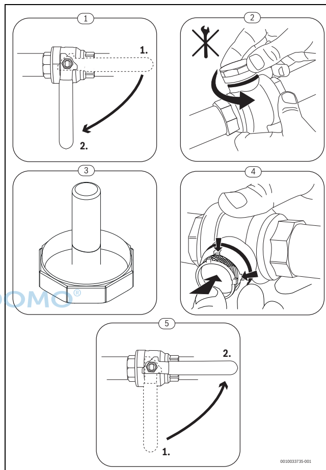
Bild 6 Siebreinigung
