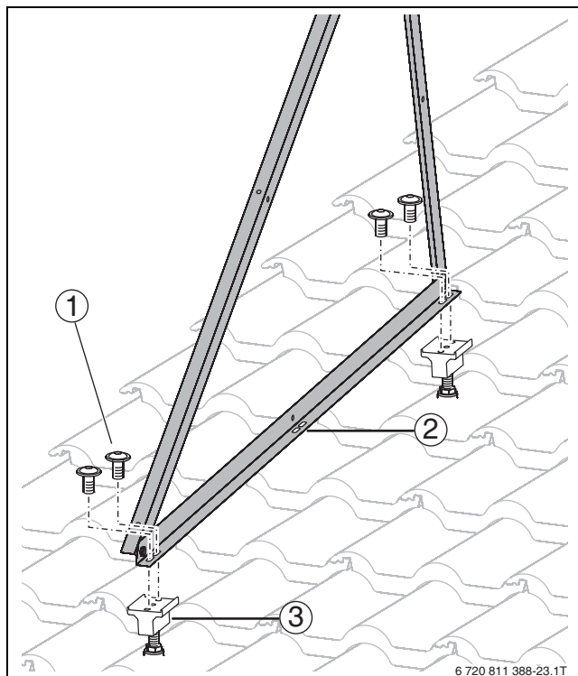
Bild 178 Aufständerung für Flachkollektoren in Verbindung mit Stockschrauben
