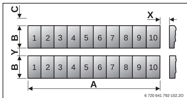
Bild 152 Flächenbedarf für Kollektorfelder mit mehreren Reihen bei Aufdachmontage (Erklärung im Text)
