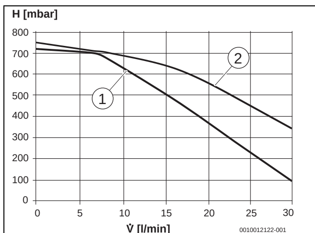
Bild 53 Restförderhöhe Primärkreispumpe
