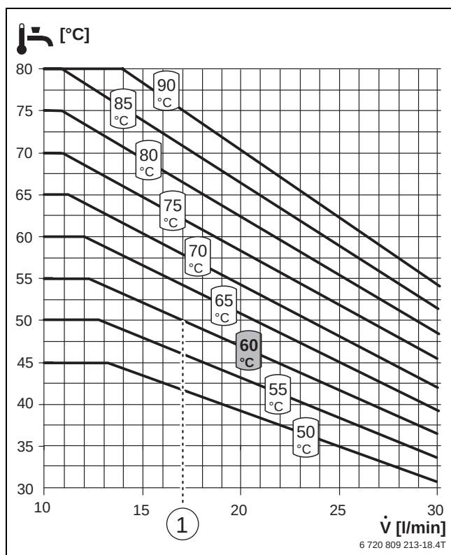
Bild 124 Temperaturverhalten Frischwasserstation
