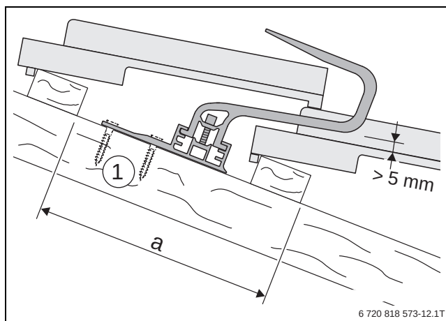
Bild 162 Dachanbindung mit Sparrenanker
