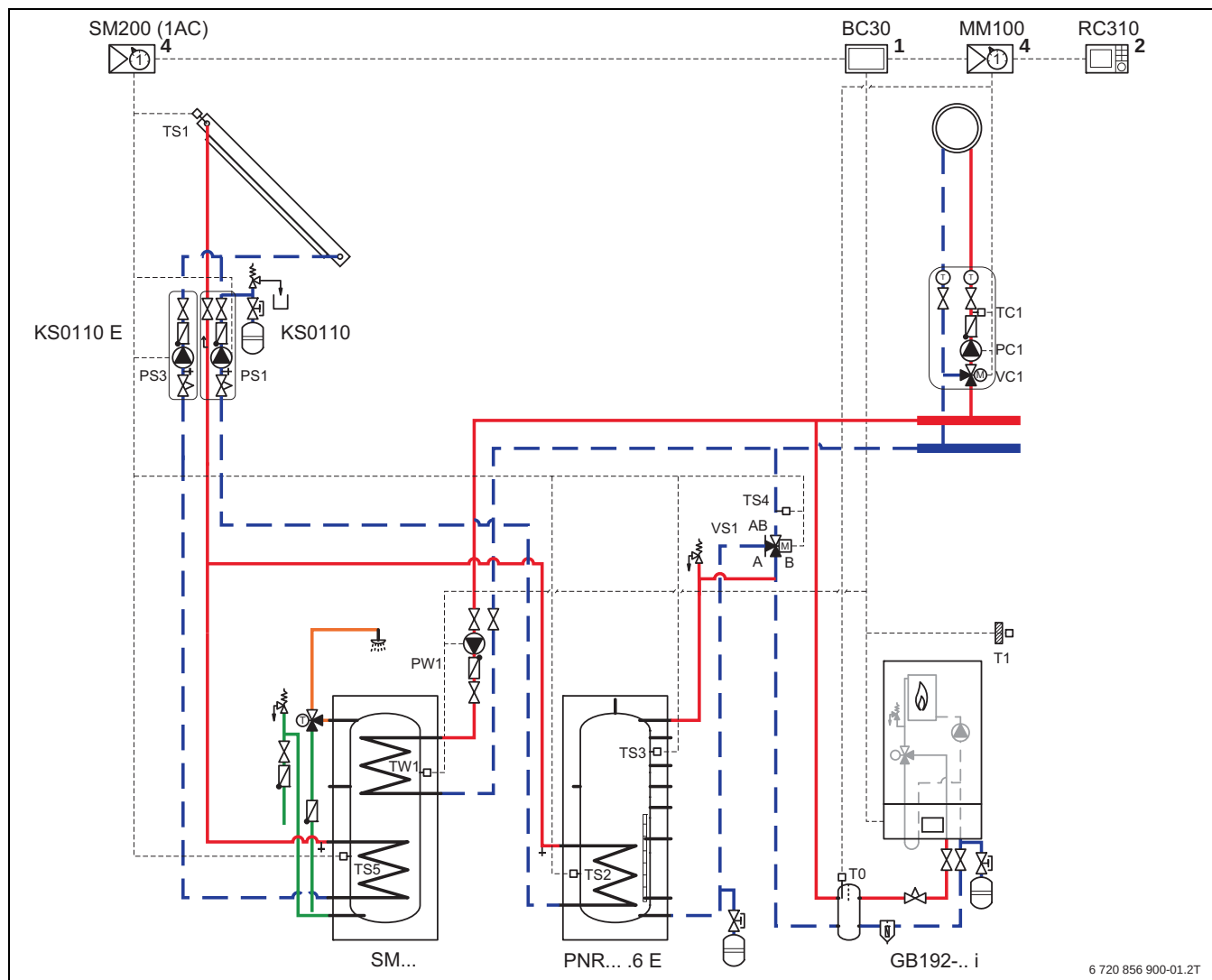
Bild 89 Solaranlage mit Flachkollektoren und 2 Solarpumpen für 2 Verbraucher
