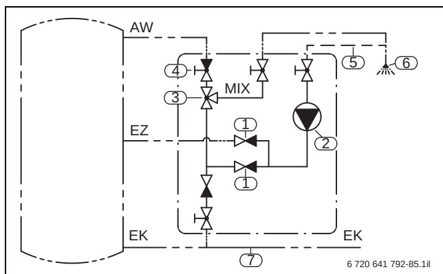
Bild 72 Installationsschema Warmwasser-Mischergruppe
