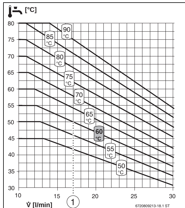
Bild 56 Temperaturverhalten FS/2
