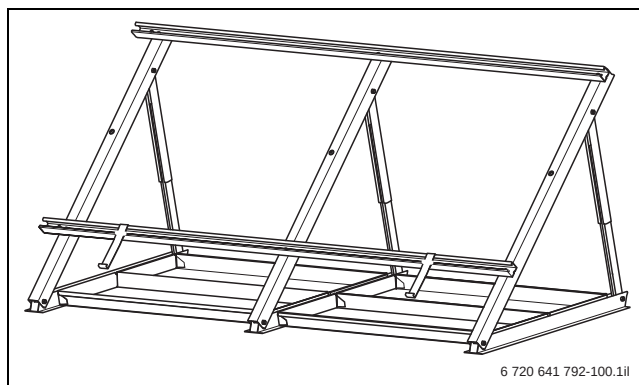
Bild 185 Flachdachmontage für einen waagerechten Logasol SKN4.0 oder SKT1.0 mit Beschwerungswannen
