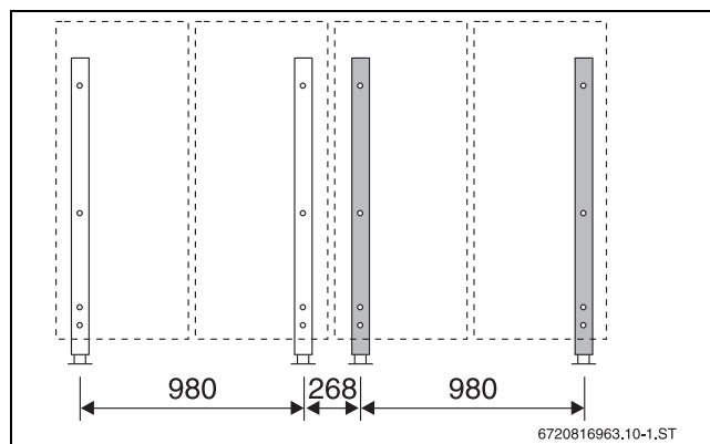
Bild 228 Grundausführung für 2 Kollektoren und Erweiterung für 2 Kollektoren, Maße in mm
