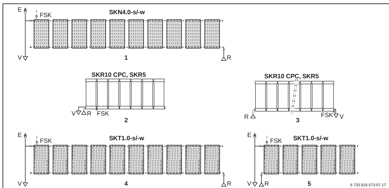
Bild 128 Anschluss einer Kollektorreihe
