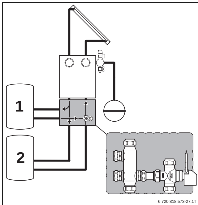
Bild 84 Anlagenschema mit Umschaltmodul SBU
