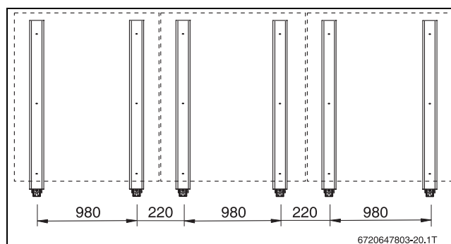
Bild 188 Abstände der Kollektorstützen bei 3 senkrechten Kollektoren bei erhöhten Lasten (Angaben in mm)
