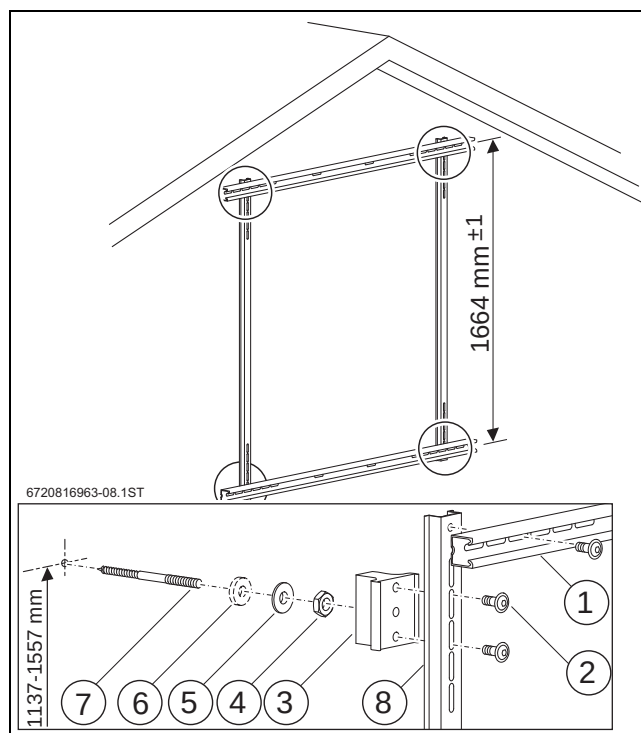
Bild 240 Aufdach-Schienen-Set mit dem Stockschrauben-Set an der Fassade montieren
