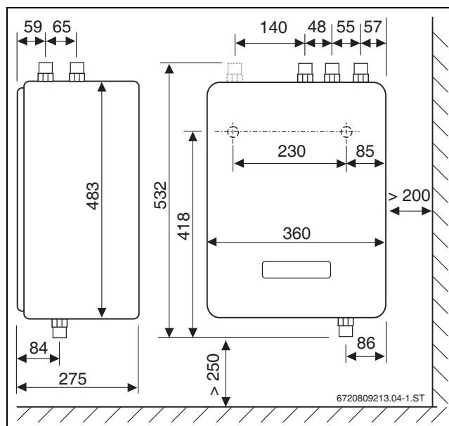
Bild 52 Abmessungen (Maße in mm)
