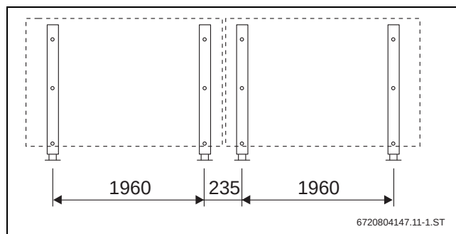
Bild 196 Abstände der Kollektorstützen bei Grundausführung für 2 waagerechte Kollektoren SKT1.0-w, Maße in mm
