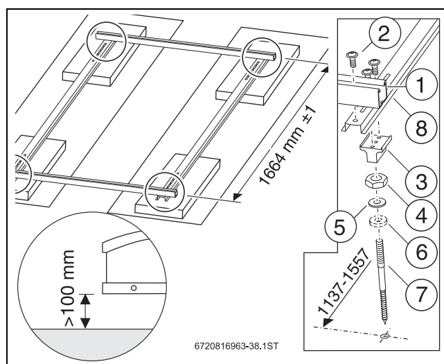
Bild 236 Profilschienen mit Stockschräben montieren
