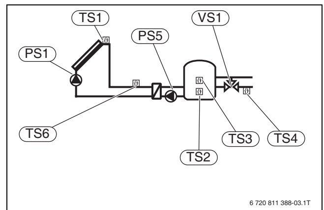
Bild 99 Hydraulikschema 1AE des Solar-Funktionsmoduls SM200 für die Speicherbeladung über einen externen Wärmetauscher
