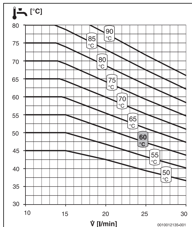
Bild 57 Temperaturverhalten FS20/2
