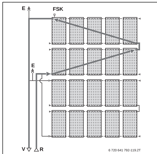
Bild 137 Kombination aus Reihen- und Parallelschaltung in einem Kollektorfeld mit Logasol SKN4.0
