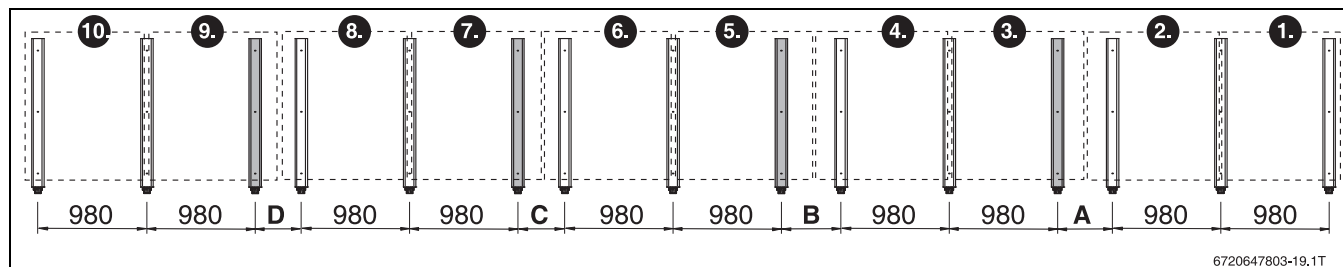
Bild 187 Grundauführung: Abstände der Kollektorstützen bei Verwendung von Beschwerungswannen für 10 senkrechte Kollektoren (Angaben in mm), Zusatzstützen in grau
