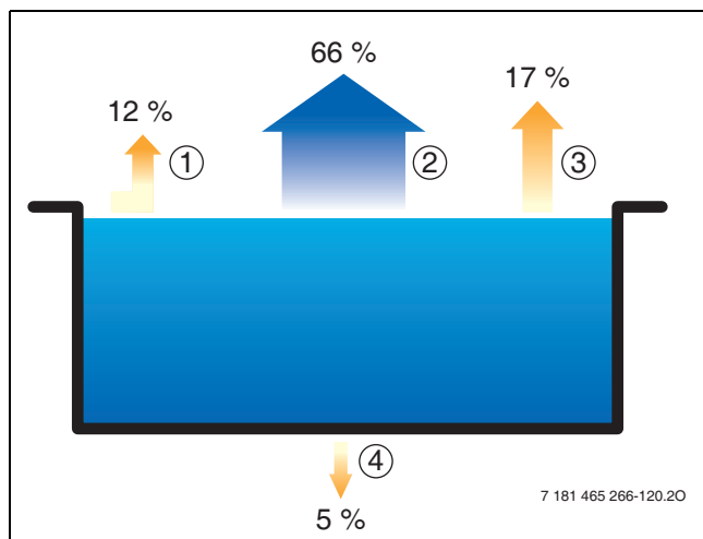
Bild 127 Wärmeverluste Schwimmbaden
