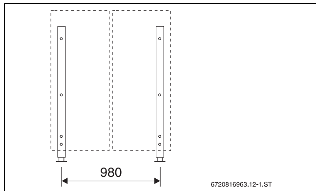
Bild 226 Grundausführung für 2 Kollektoren, Maße in mm
