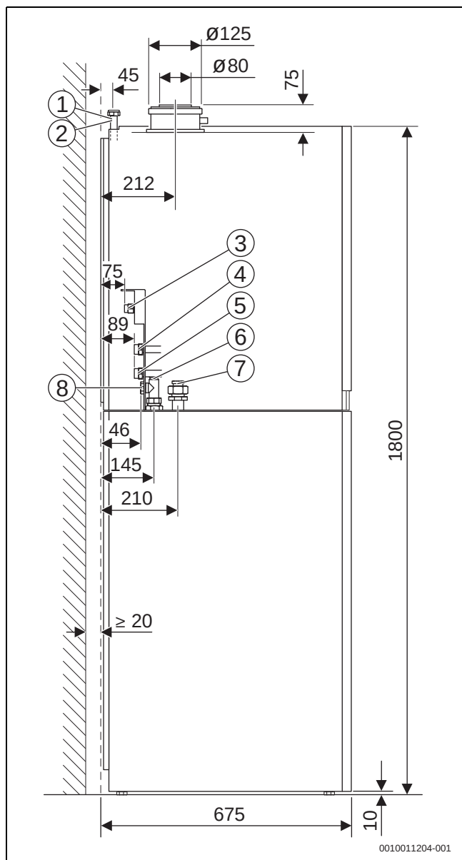
Bild 22 Abmessungen und Anschlüsse für GB192iT ohne Zubehör (Maße in mm)
