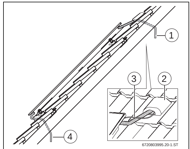
Bild 172 Anschlussrohr durch das Dach führen
