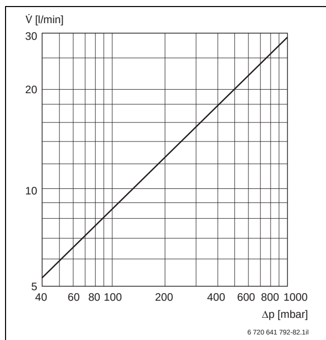
Bild 68 Druckverlust thermostatischer Warmwassermischer R \frac{3}{4} bei 80 °C Warmwassertemperatur, 60 °C Mischwassertemperatur und 10 °C Kaltwassertemperatur
