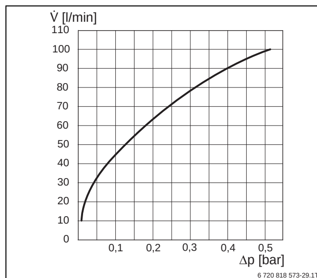
Bild 88 Druckverlust VS-SU und HZG-Set
