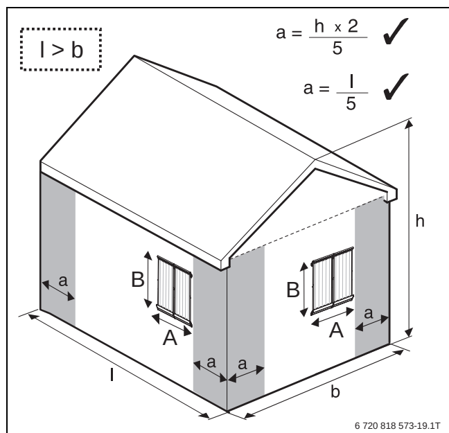
Bild 238 Einzuhaltende Abstandsmaße zum Gebäude- und Gebäuderand (a); der kleinere Wert kann genutzt werden
