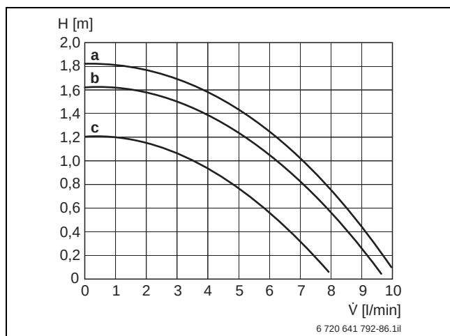
Bild 73 Restförderhöhe Zirkulationspumpe
