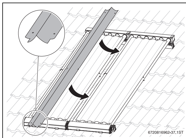
Bild 13 Zwischenspiegel einlegen
