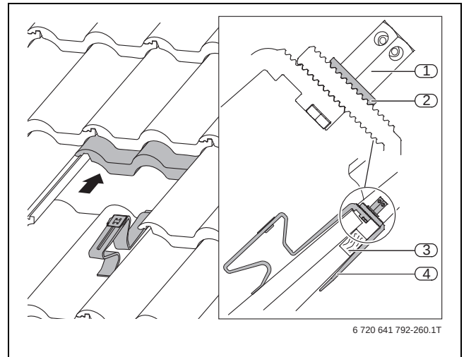
Bild 158 Eingängter Dachhaken
