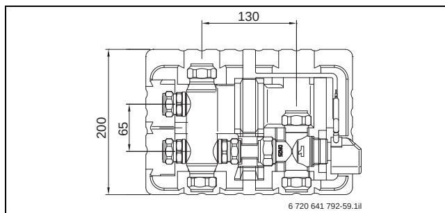
Bild 85 Abmessungen SBU (Maße in mm)
