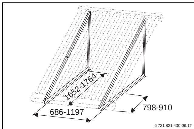
Bild 218 Abstände für die Befestigungspunkte der Dreieckstützen für die Aufständerung (Maße in mm)
