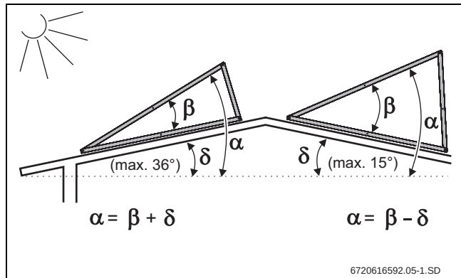
Bild 177 Anstellwinkel bei geneigten Dächern
