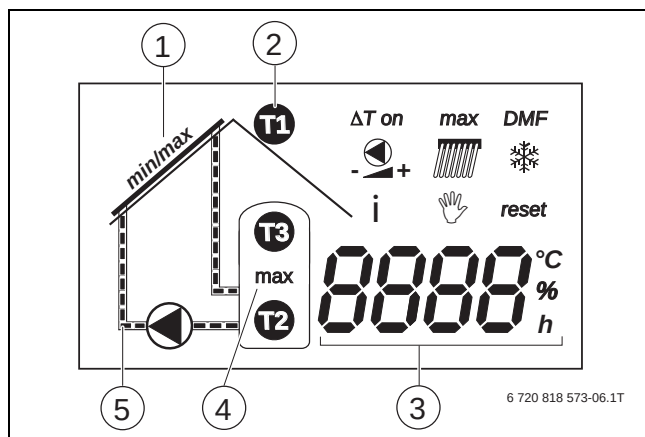
Bild 76 LCD-Segmentdisplay Logamatic SC20/2
