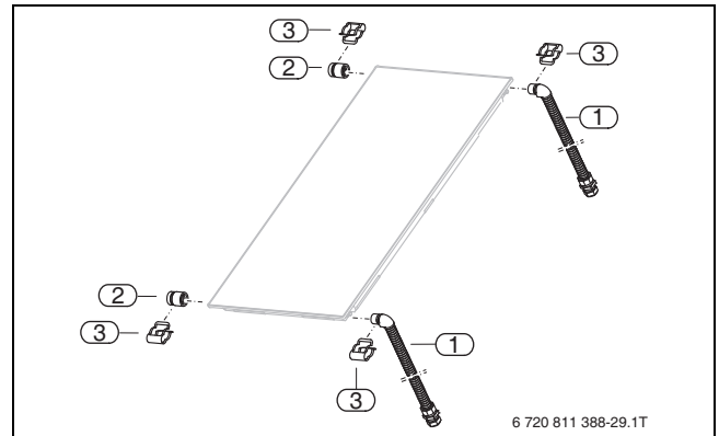
Bild 171 Anschluss-Set Logasol SKT1.0 Aufdach/Indach
