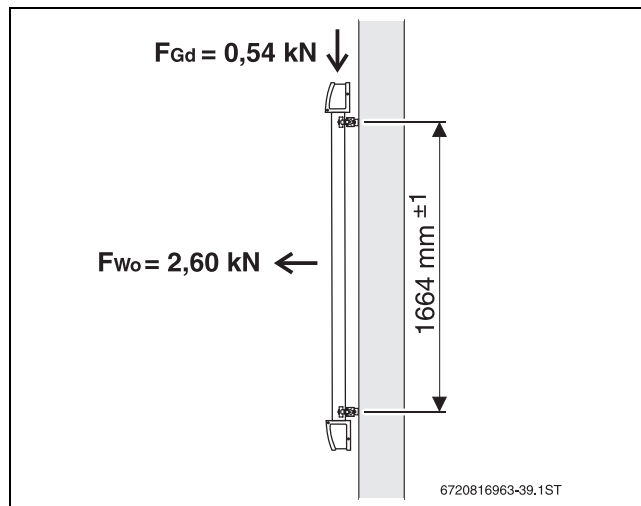
Bild 239 Logasol SKR bauseits an der Fassade montieren
