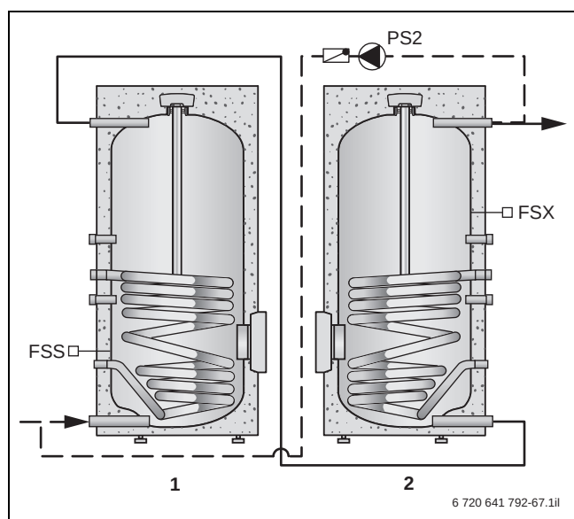
Bild 96 Umladung bei Speicherreihenschaltung
