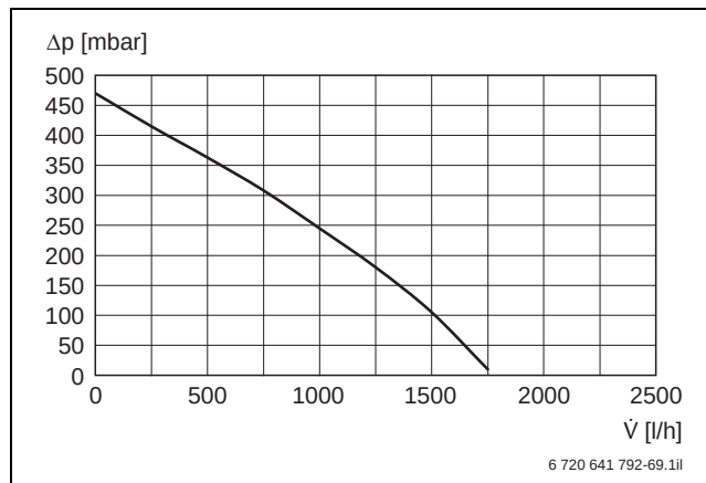
Bild 98 Restförderhöhe SBL
