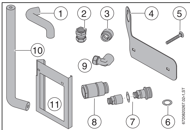
Bild 59 Lieferumfang Speichermontage-Set
