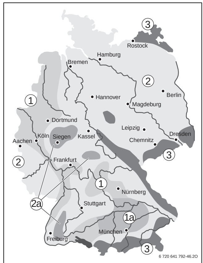
Bild 150 Schneelastzonenkarte nach DIN EN 1991-1-3/NA
