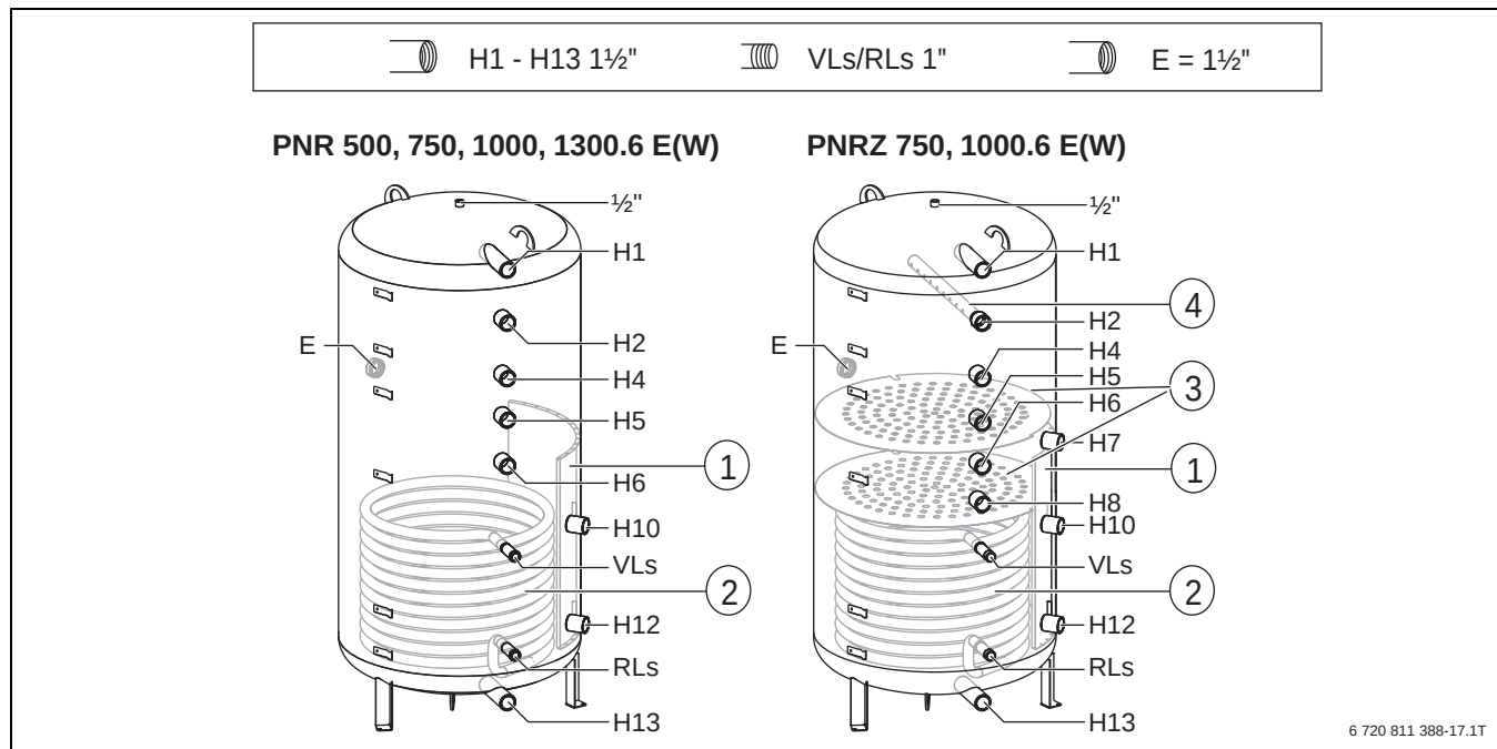
Bild 31 Aufbau und Anschlüsse PNR(Z)....6 E
