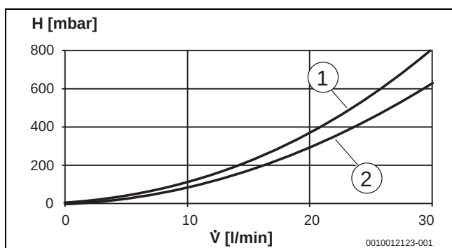
Bild 54 Druckverlust Sekundärseite
