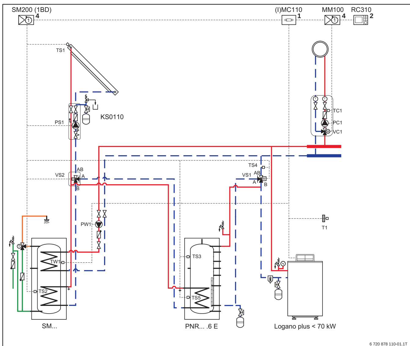
Bild 82 Solaranlage mit Flachkollektoren und Umschaltventil für 2 Verbraucher; Abkürzungsverzeichnis → Tabelle 44, Seite 78
