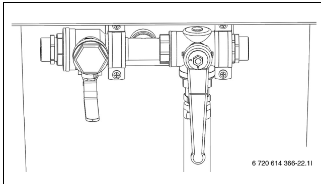
Bild 26 Befüllstation in Mischposition
