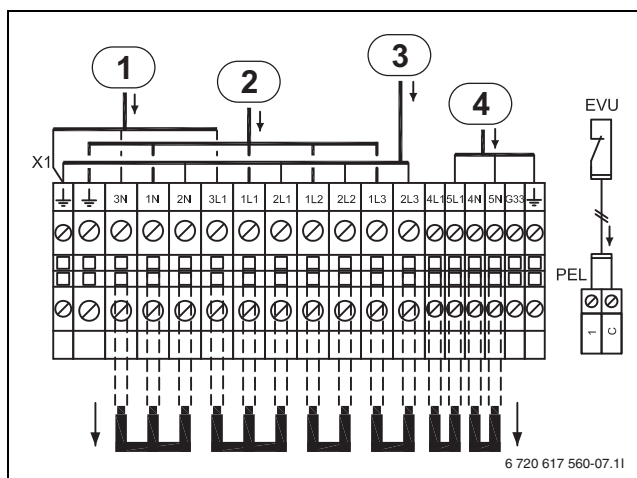
Bild 42 Alternative C, WPS 6-1 - 10-1 und WPS 6K-1 - 10K-1
