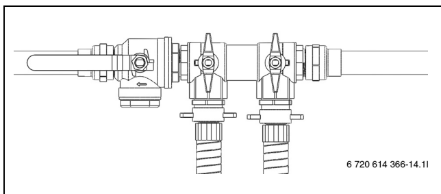
Bild 22 Befüllereinrichtung WPS 6-1...10-1, WPS 6K-1...10 K-1
