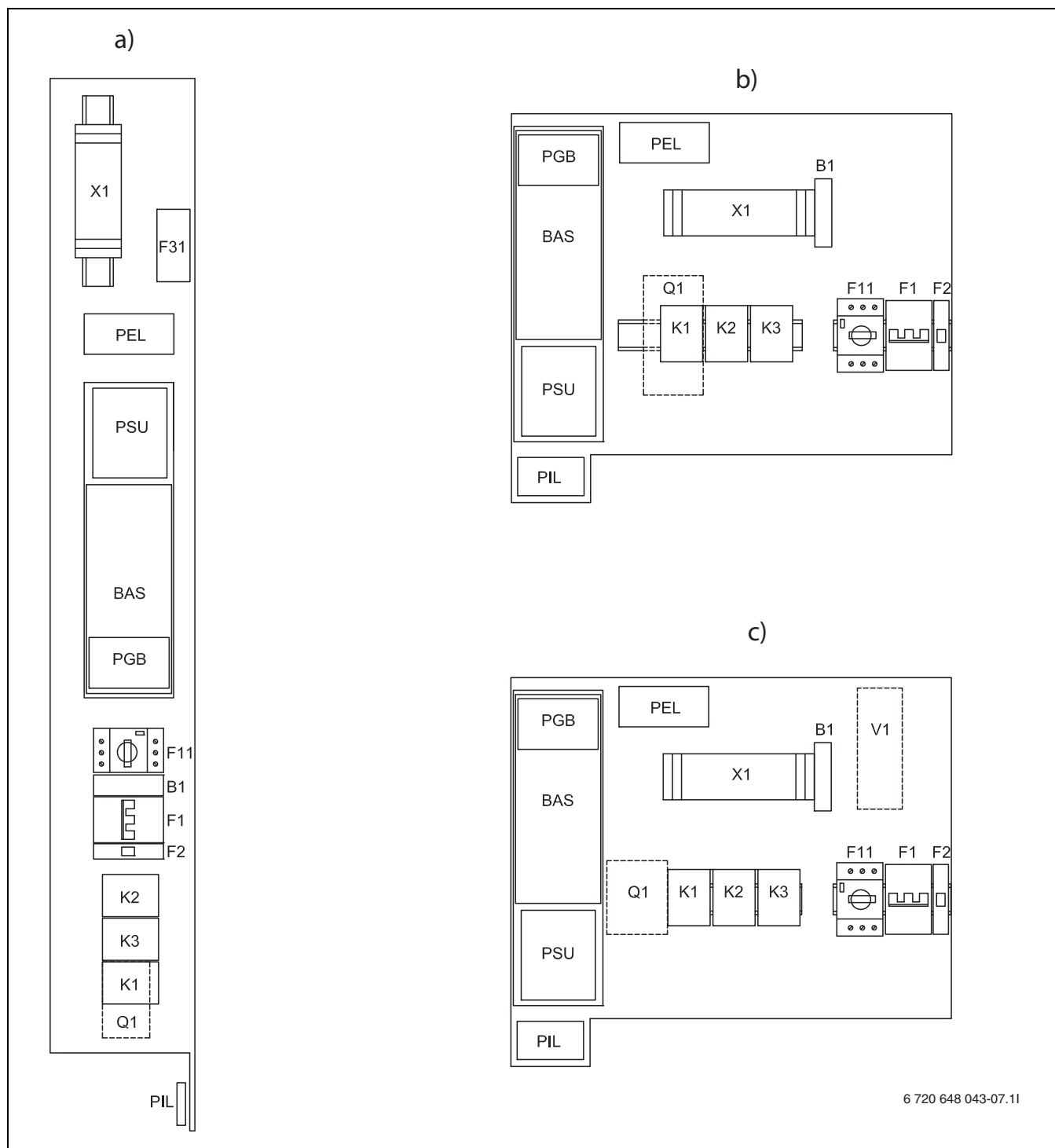
Bild 34 Übersicht Leiterplatte
