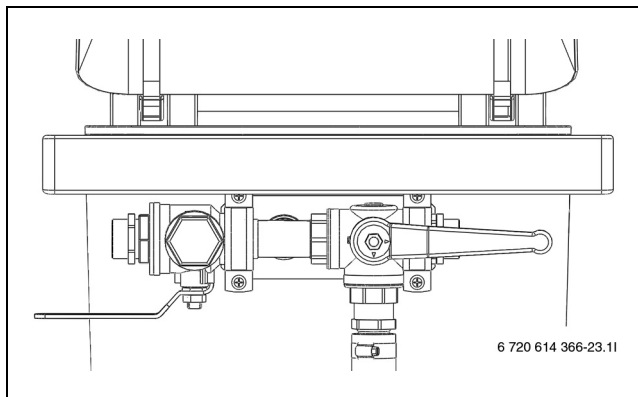
Bild 27 Befüllstation in Befüllposition
