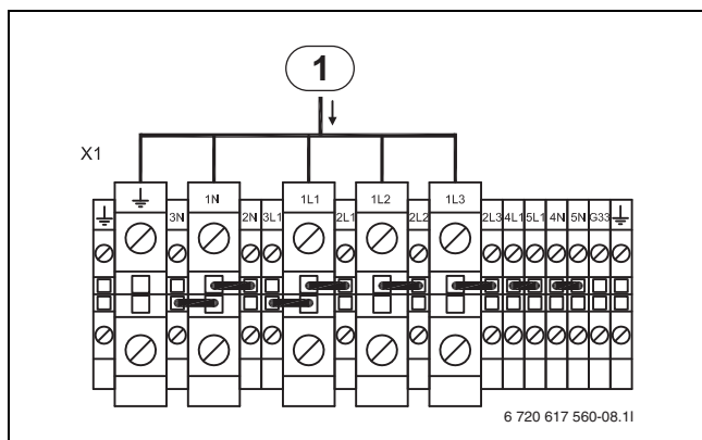
Bild 43 Standardausführung, WPS 13-1 - 17-1
