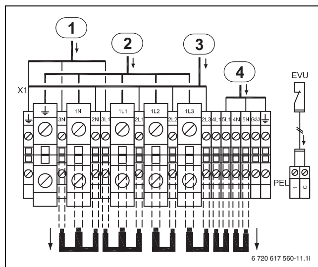
Bild 46 Alternative C, WPS 13-1 - 17-1
