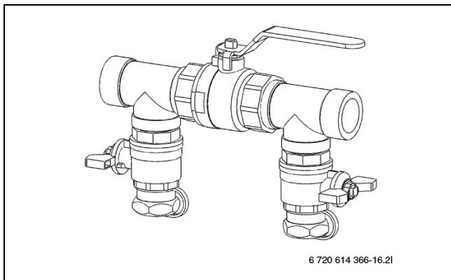
Bild 23 Befüllereinrichtung WPS 13-1...17-1
