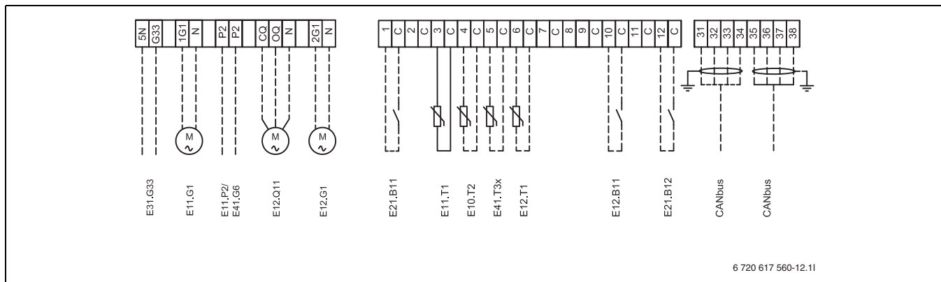
Bild 47 Externe Anschlüsse
