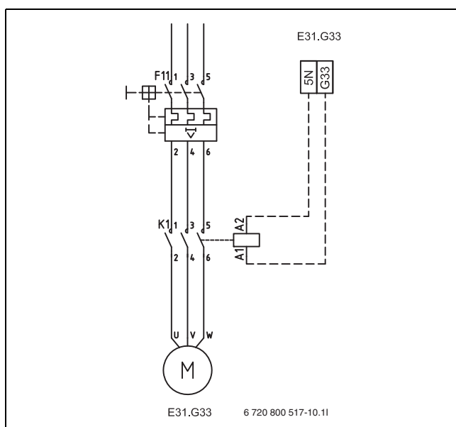
Bild 48 Anschluss Grundwasserpumpe
