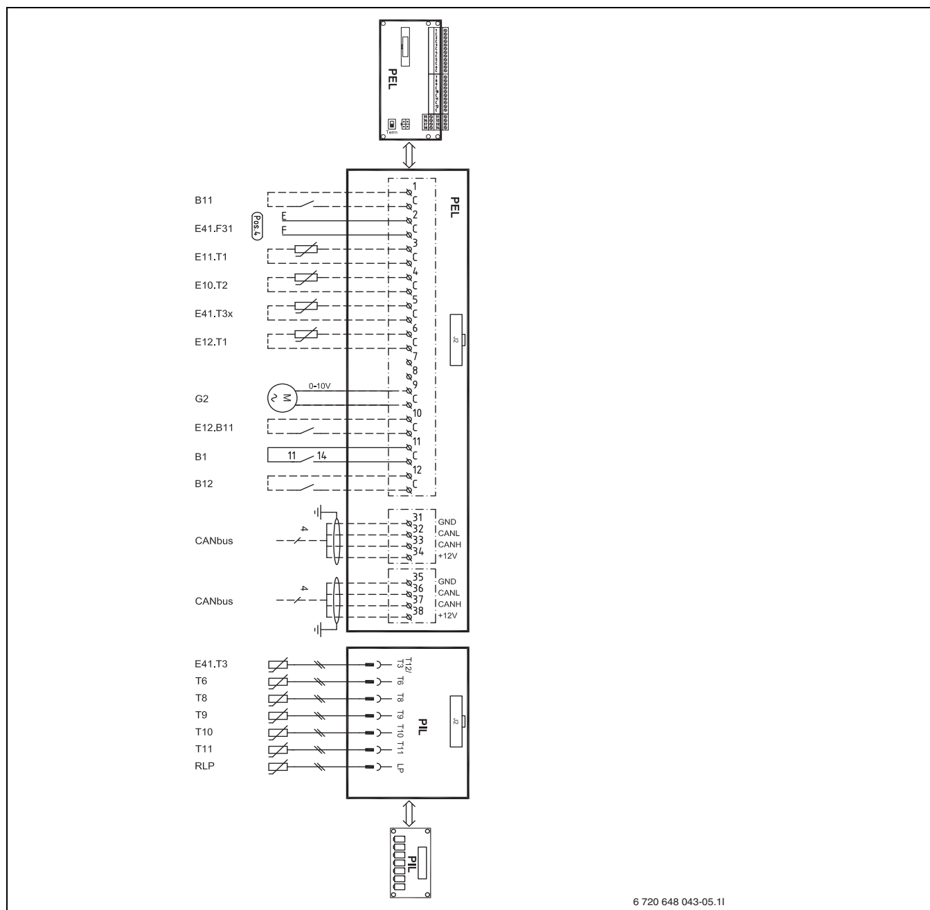
Bild 51 Kompletter Anschlussschaltplan (Niederspannung)
