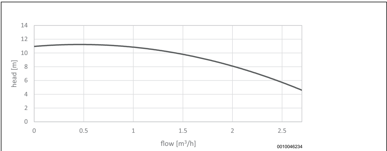
Wärmeträgerpumpe, Erdwärmepumpe 17 kW
