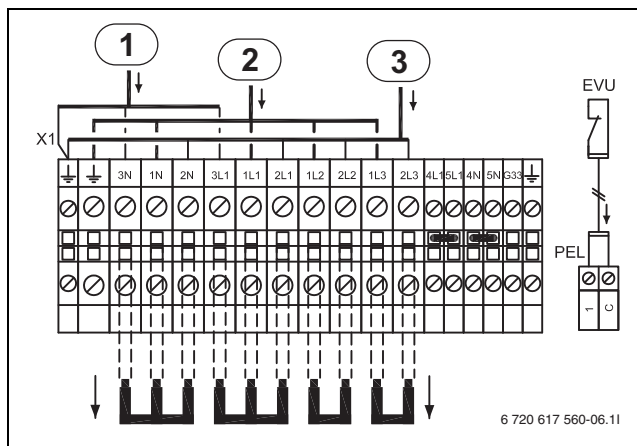
Bild 41 Alternative B, WPS 6-1 - 10-1 und WPS 6K-1 - 10K-1
