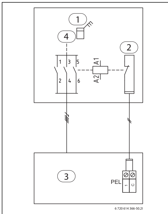
Bild 37 Sperrzeit aktiv
