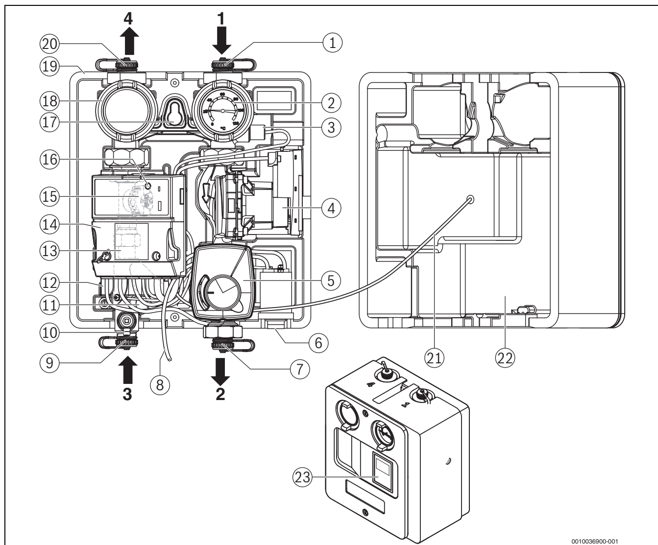
Bild 3 Komponenten Bypassentsalzungsmodul
