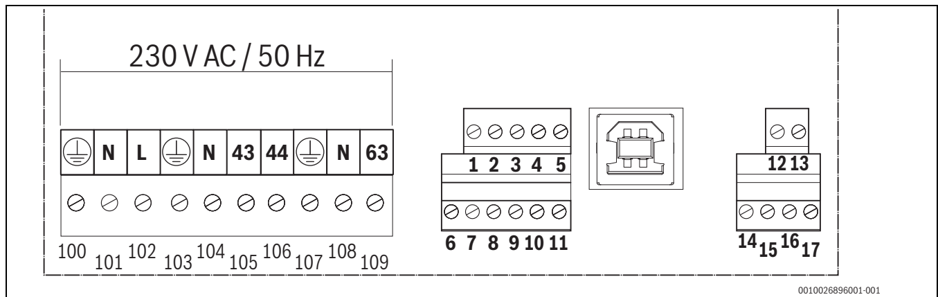
Bild 32 Anschlussplan
