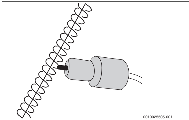
Bild 19 Elektroden reinigen
