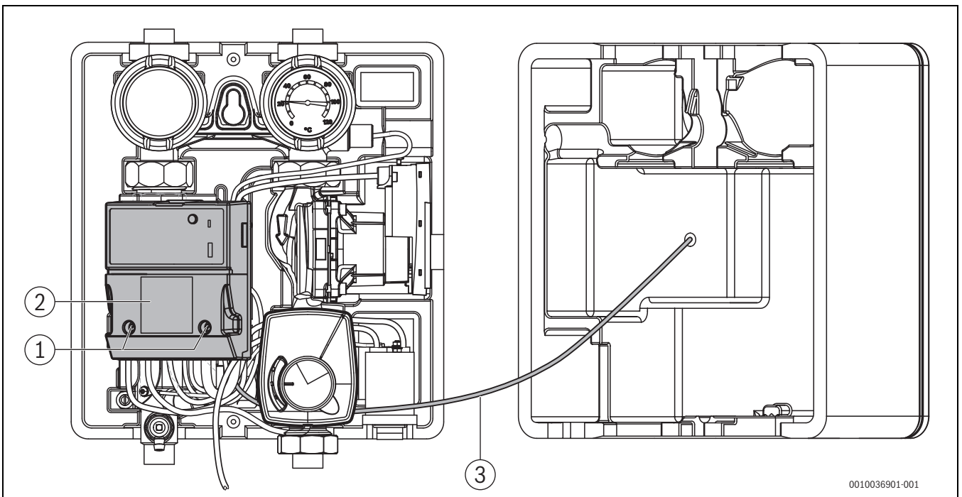
Bild 21 Elektronik-Modul öffnen
