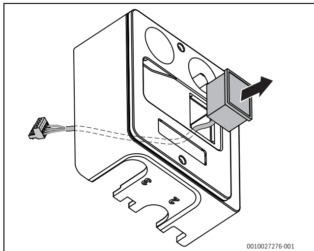
Bild 24 Bedieneinheit entnehmen
