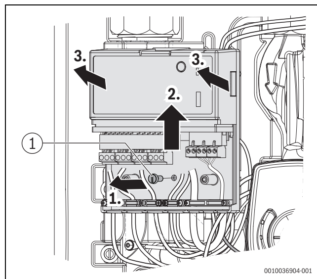
Bild 28 Elektronik-Modul abnehmen
