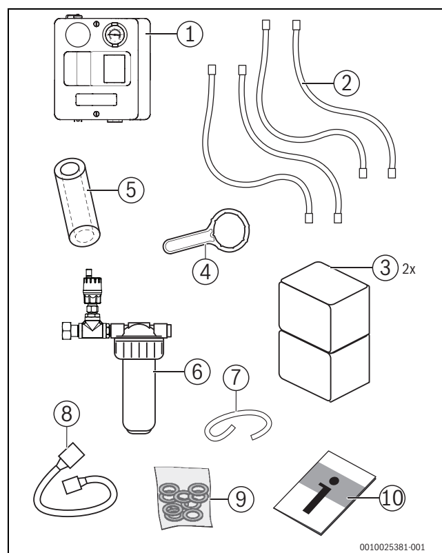
Bild 2 Lieferumfang mobiles Bypassentsalzungsmodul
