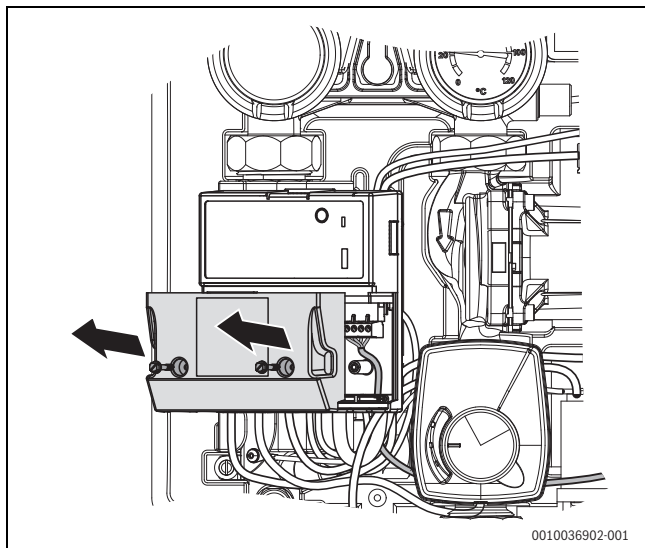
Bild 22 Abdeckung abnehmen
