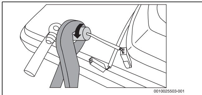
Bild 17 Leitfähigkeitssonde lösen
