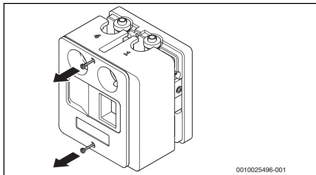
Bild 25 Isolierteil abnehmen
