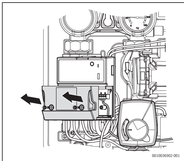
Bild 27 Abdeckung abnehmen
