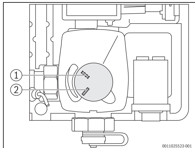
Bild 4 2-Wege-Ventil geschlossen/geöffnet
