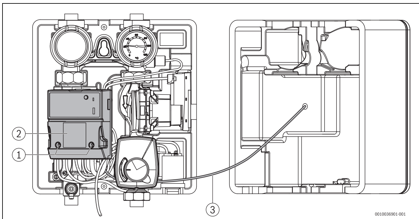
Bild 26 Elektronik-Modul öffnen
