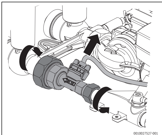
Bild 30 Volumenstromfühler ausbauen
