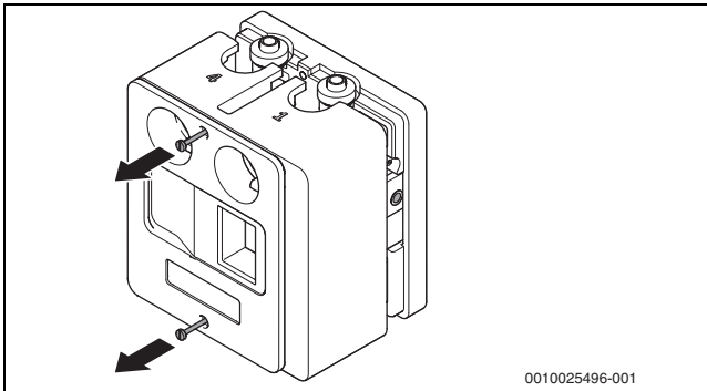
Bild 20 Isolierteil abnehmen
