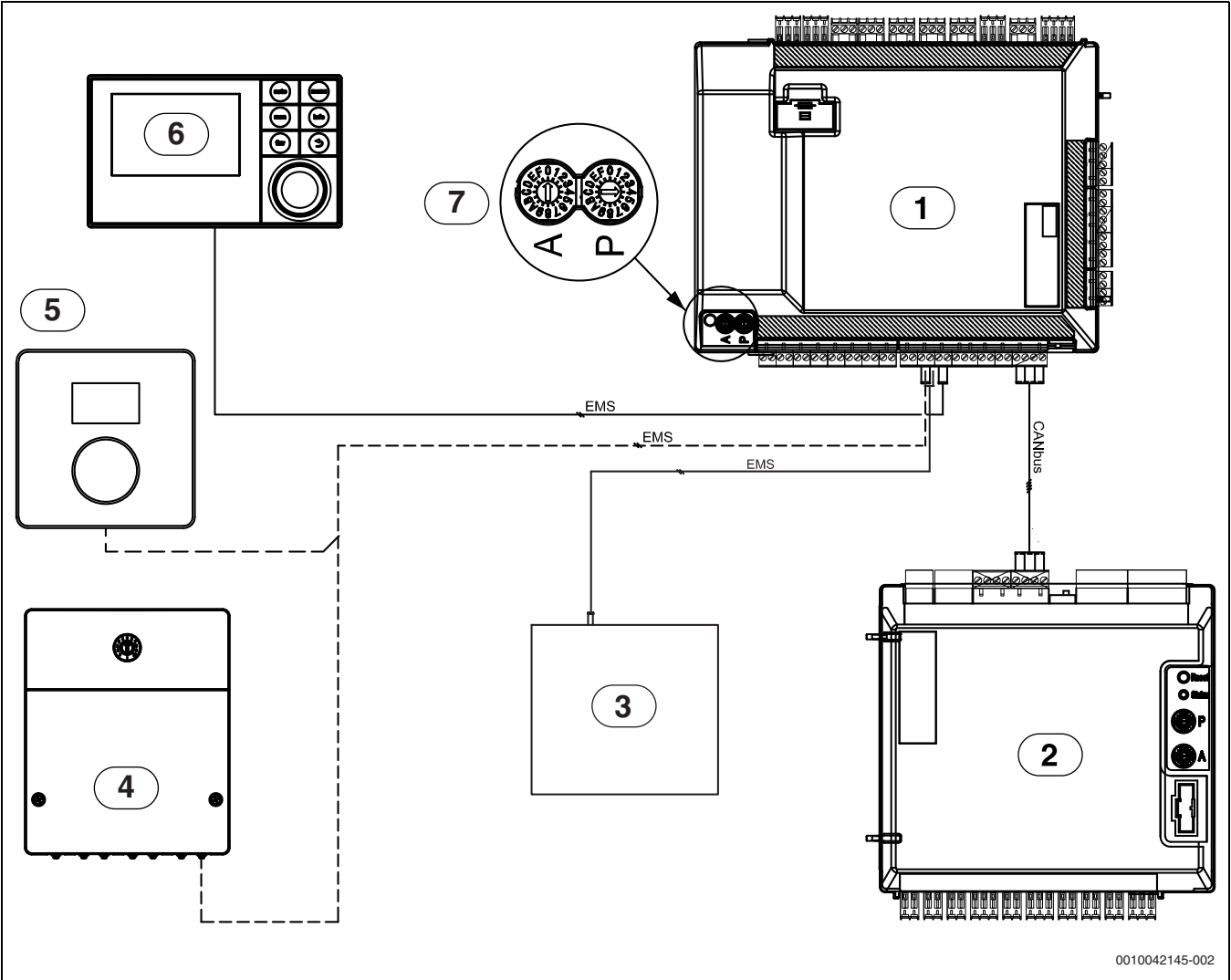
Bild 55 Schaltplan/Inneneinheit
