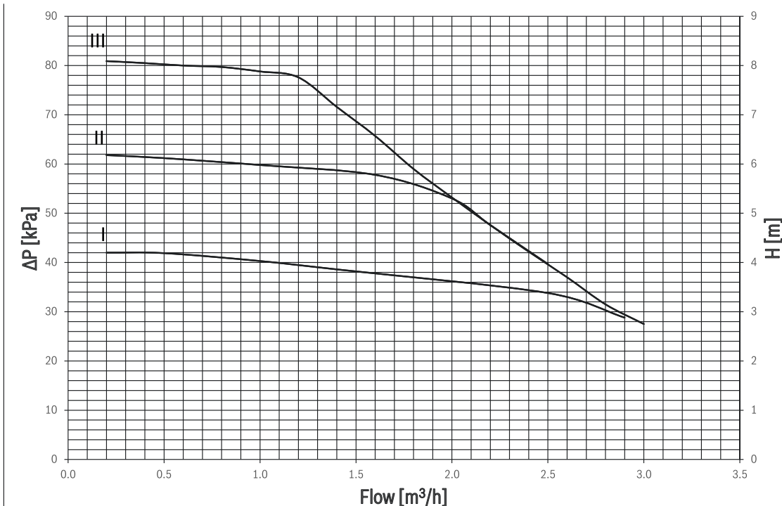
Bild 44 Restförderhöhe Heizkreispumpe für den Anschluss an den ungemischten Heizkreis für PC1 im Betrieb mit konstantem Druck
