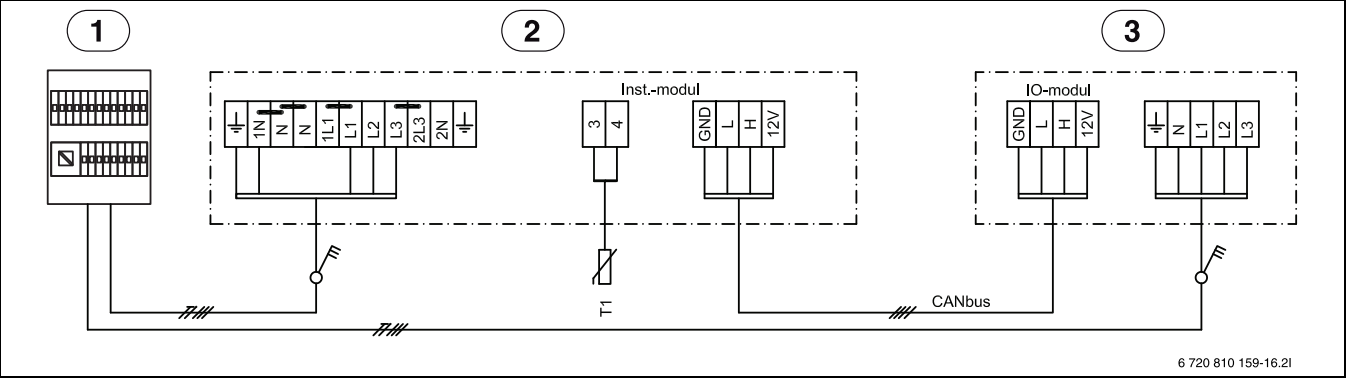
Bild 50 Schaltplan 3 N~
