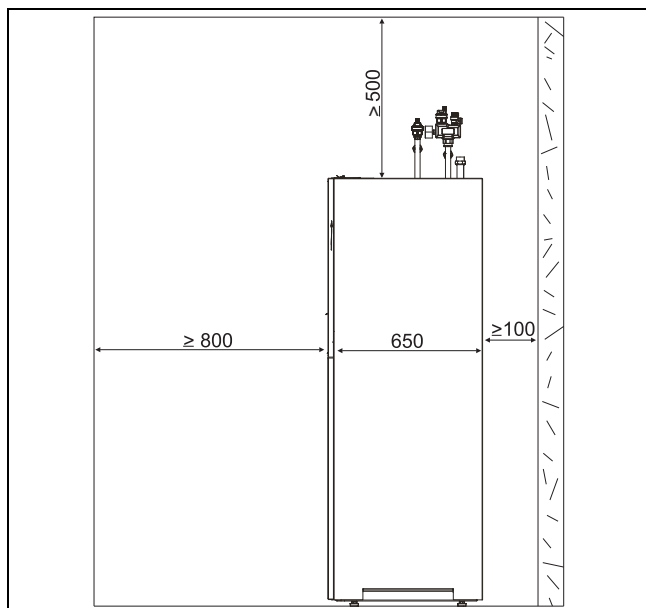
Bild 3 Mindestabstand Inneneinheit
