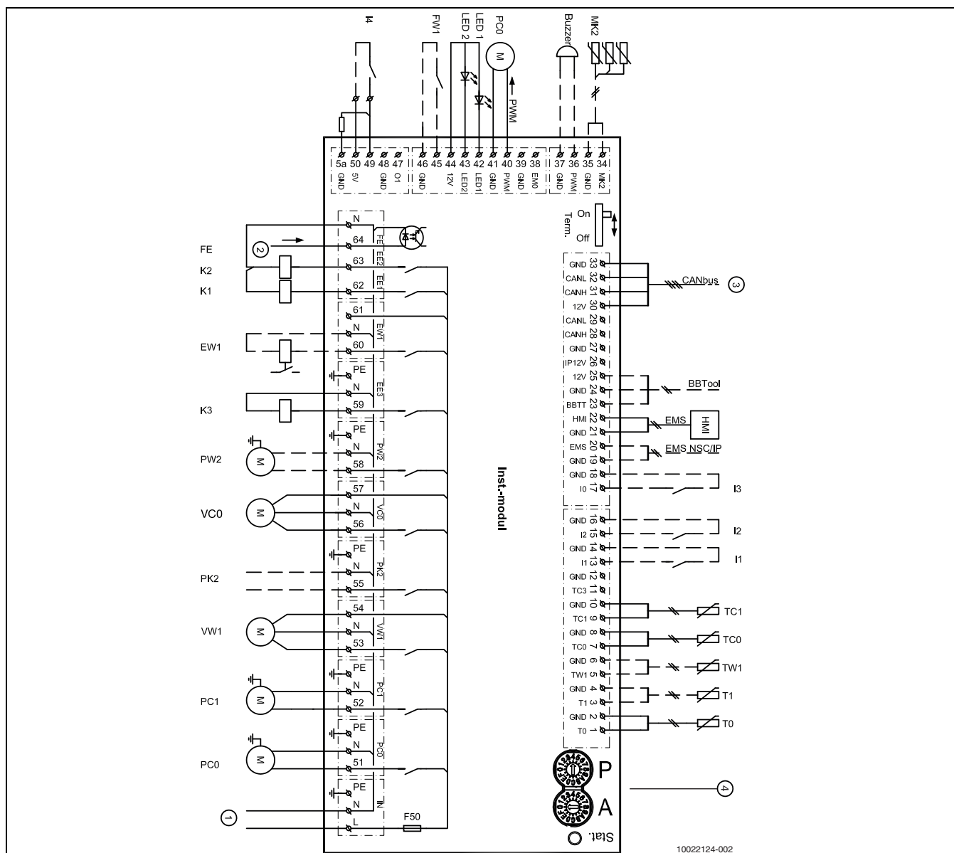
Bild 54 Schaltplan Installationsmodul
