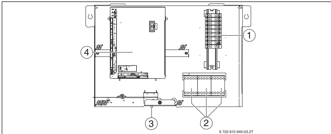
Bild 23 Klemmenkastenordnung
