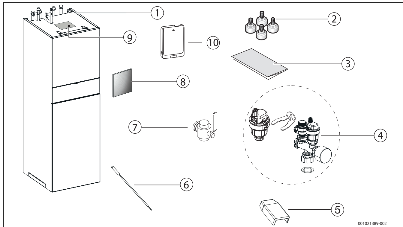
Bild 1 Lieferumfang
