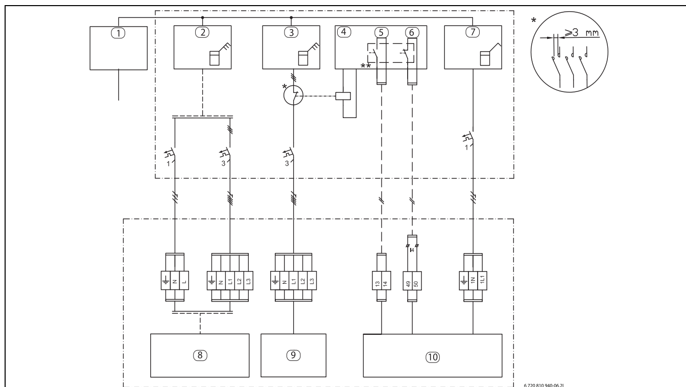
Bild 38 EVU-Typ 2
