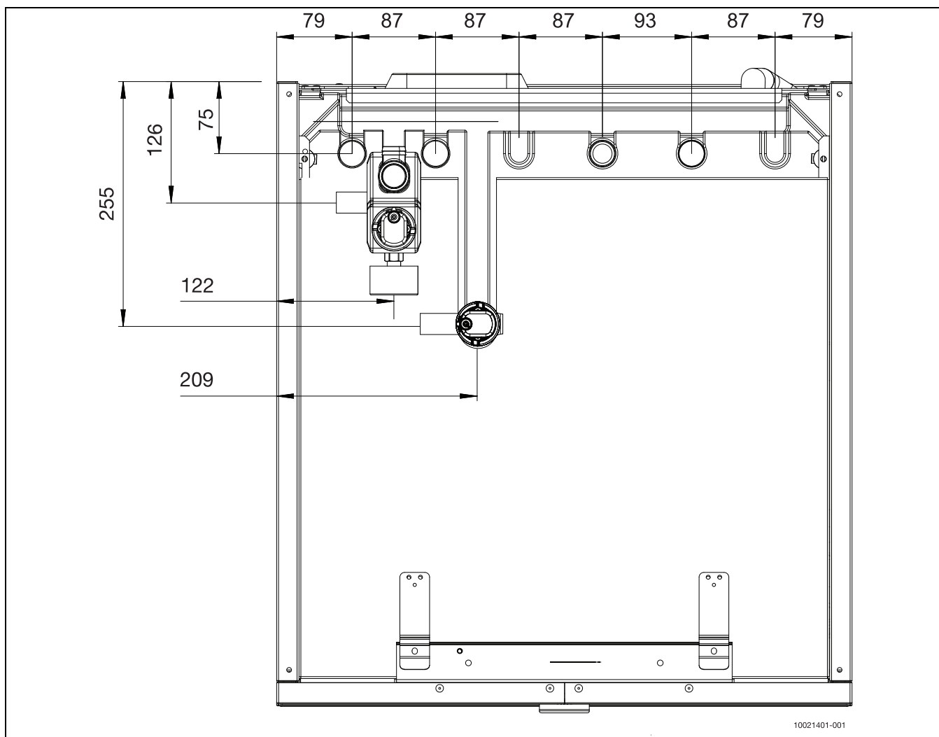
Bild 5 Abmessungen – Draufsicht
