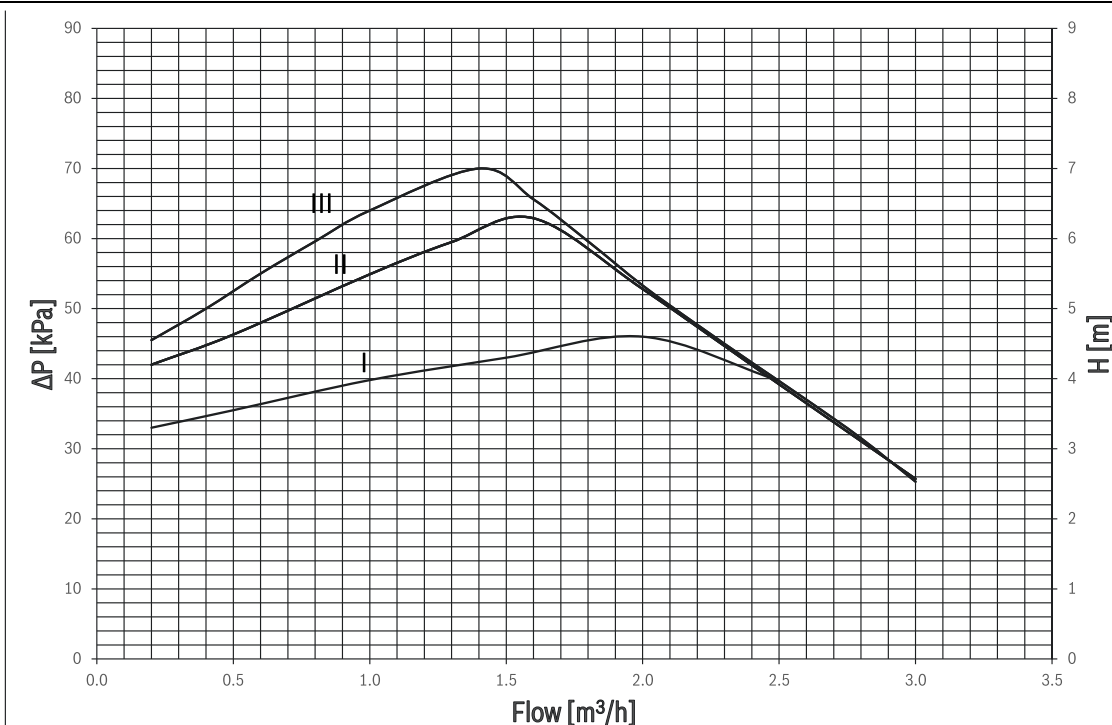
Bild 43 Restförderhöhe Heizkreispumpe für den Anschluss an den ungemischten Heizkreis für PC1 im Betrieb mit proportionalem Druck
