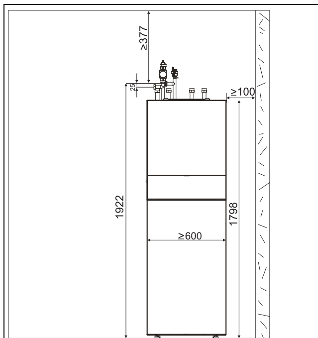
Bild 4 Abmessungen der Inneneinheit (mm)
