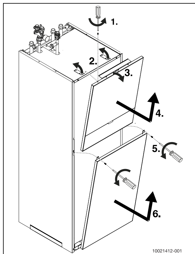
Bild 10 Abdeckungen entfernen
