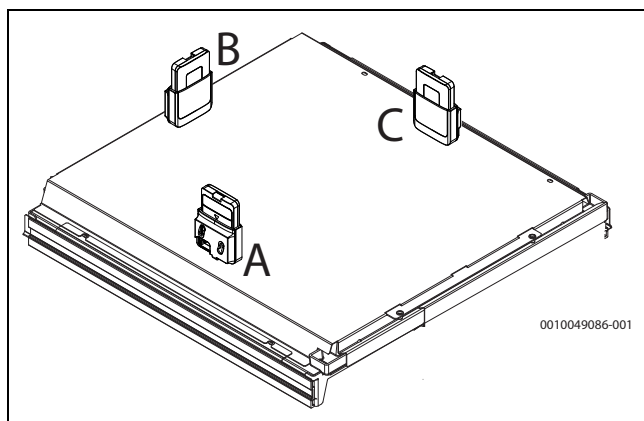
Bild 20 Befestigung des Halters an der oberen Abdeckung der Inneneinheit. Neben dem Halter zeigt die Abbildung auch das im Halter sitzende Funkmodul
