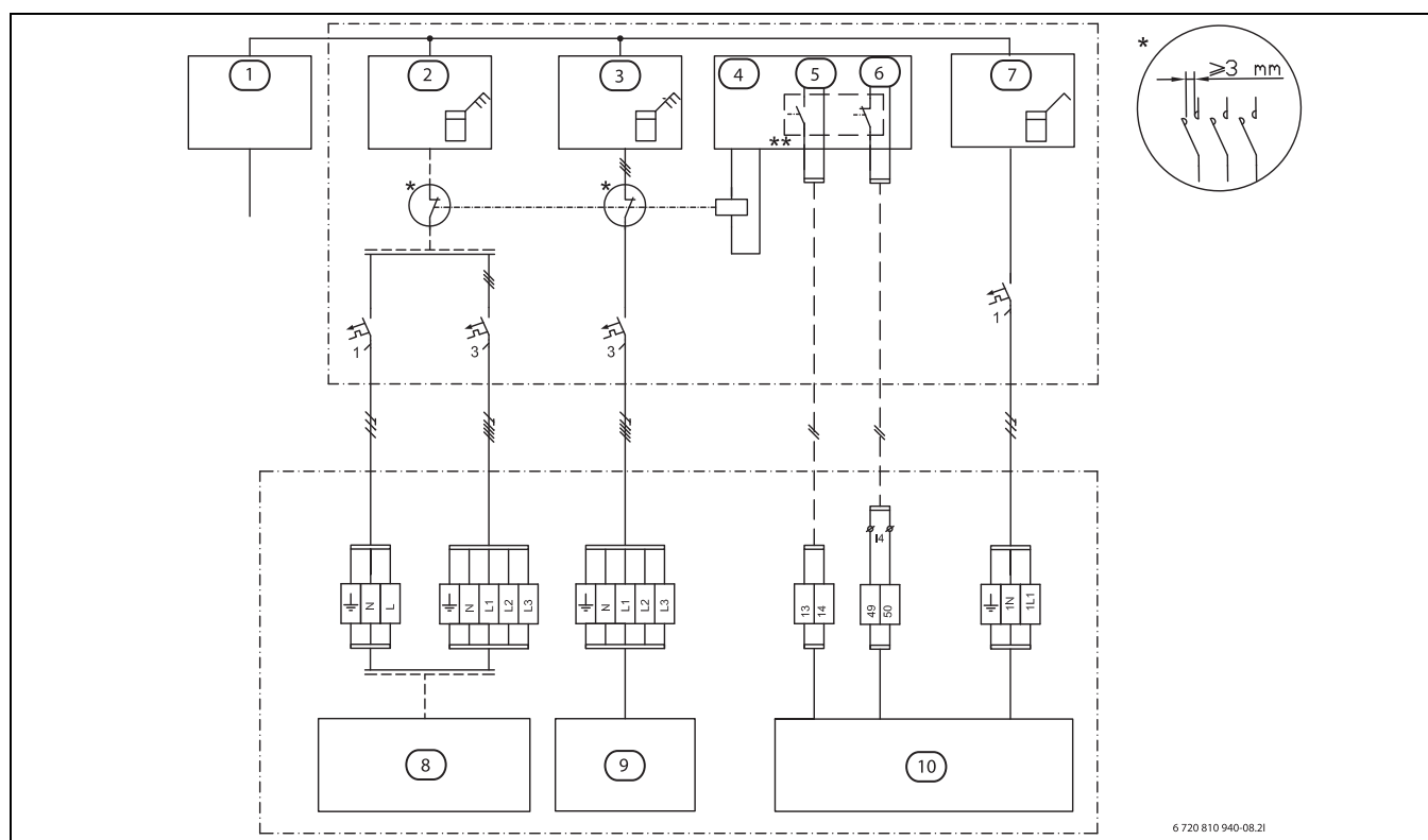
Bild 36 EVU-Typ 1
