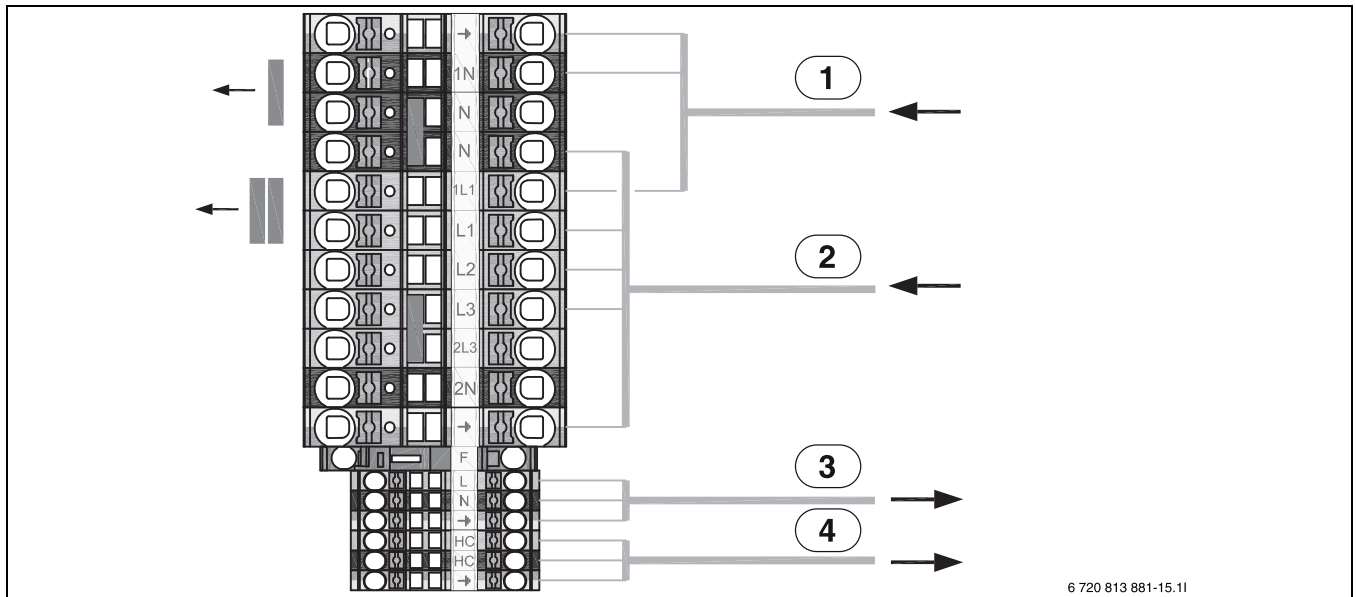
Bild 33 Klemmenbelegung im Schaltkasten
