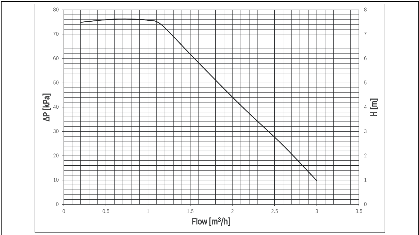
Bild 41 Restförderhöhe Primärpumpe
