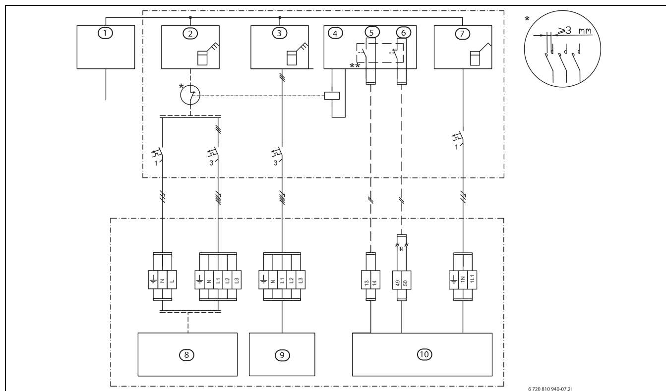
Bild 37 EVU-Typ 2
