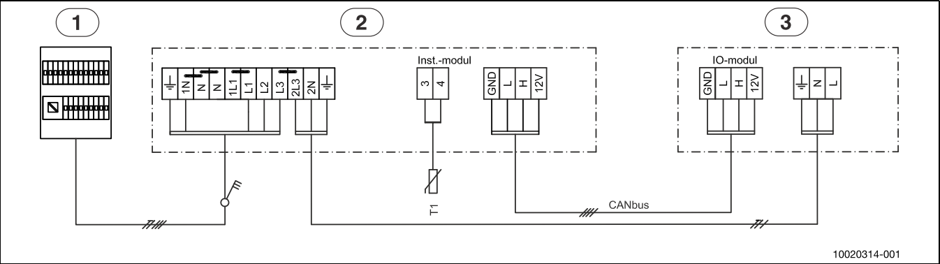
Bild 49 Schaltplan 3 N~
