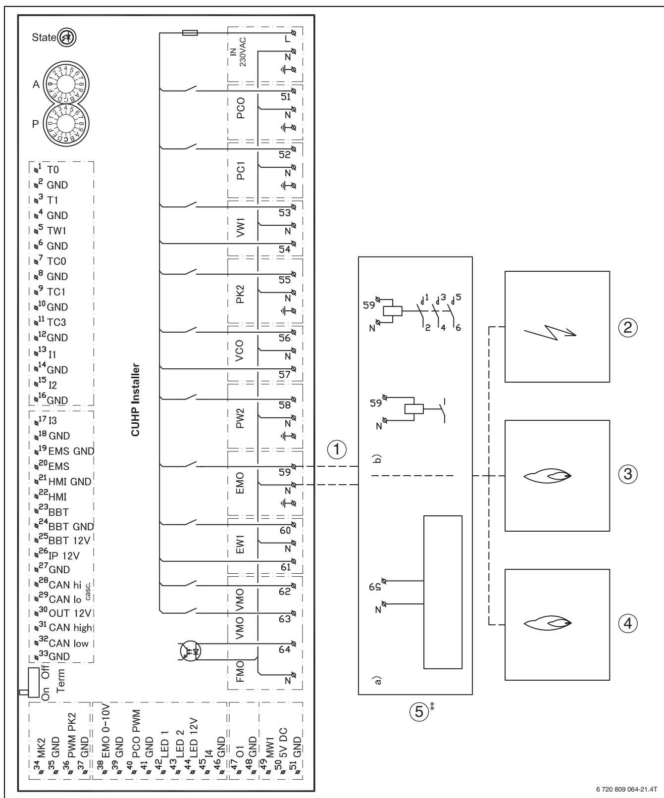
Bild 34 Schaltplan für Installationsmodul, Start/Stop mit externem Zuheiz
