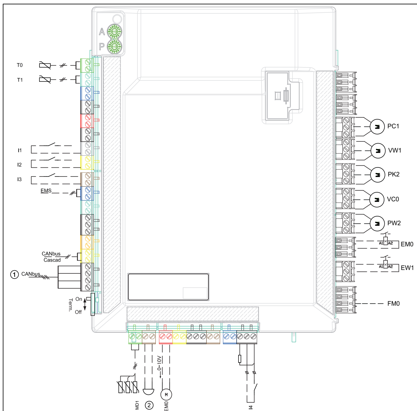
Bild 13 Anschlüsse Installationsmodul
