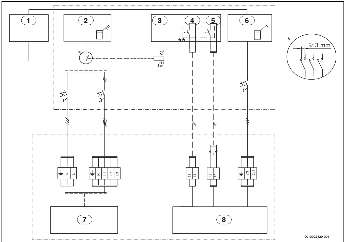
Bild 38 EVU Typ 2
