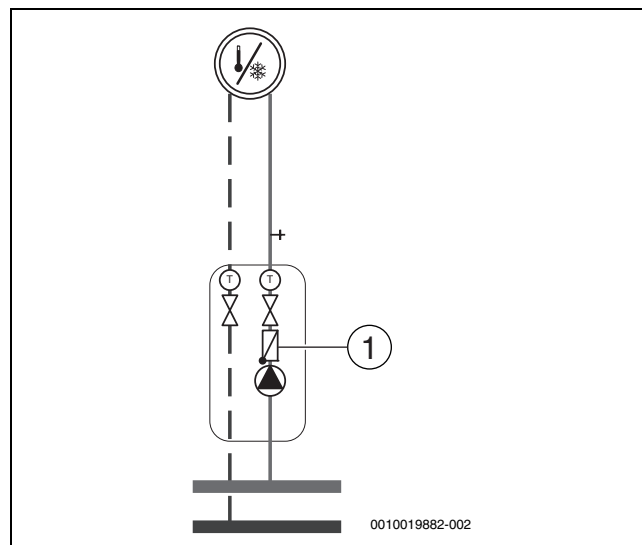
Bild 28 Heizkreis
