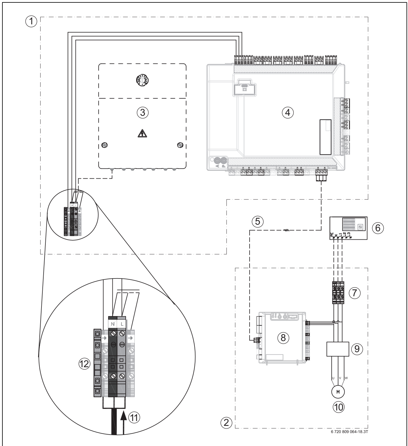
Bild 31 Einphasige Wärmepumpe und Inneneinheit mit externem Zuheizter
