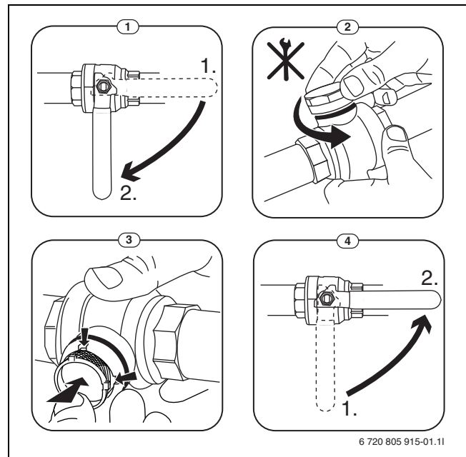
Bild 21 Siebreinigung
