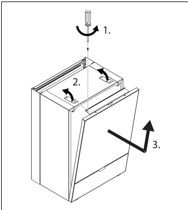
Bild 6 Frontplatte abnehmen
