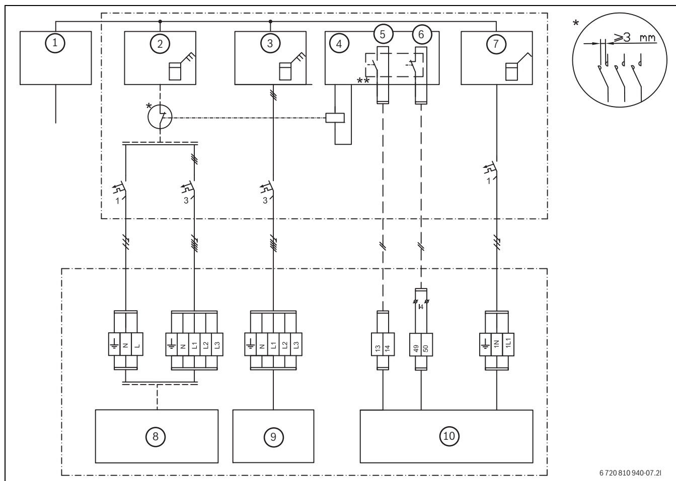
Bild 41 EVU Typ 2
