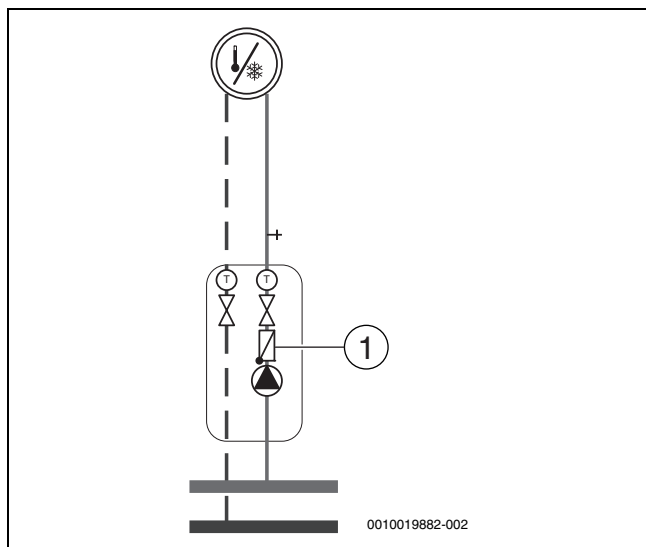
Bild 31 Heizkreis
