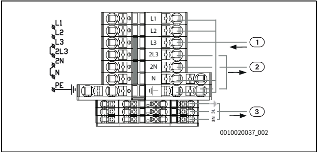
Bild 12 Elektrischer Standardanschluss bei integriertem elektrischen Zuheizer
