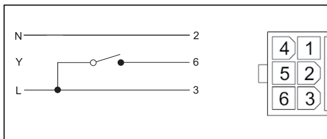
Bild 27 Molex-Stecker
