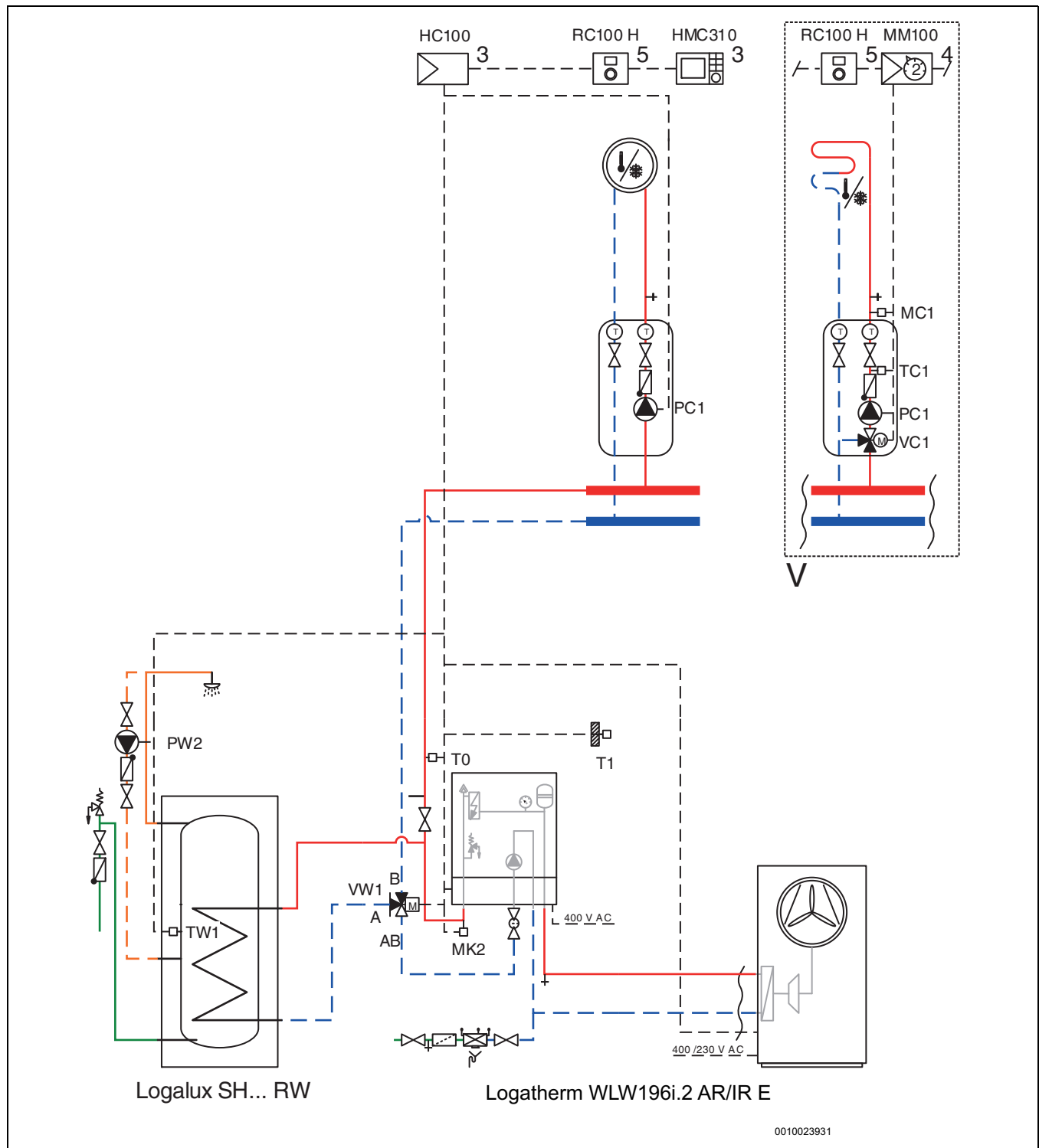
Bild 32 Elektrischer Zuheizter mit Warmwasserbereiter
