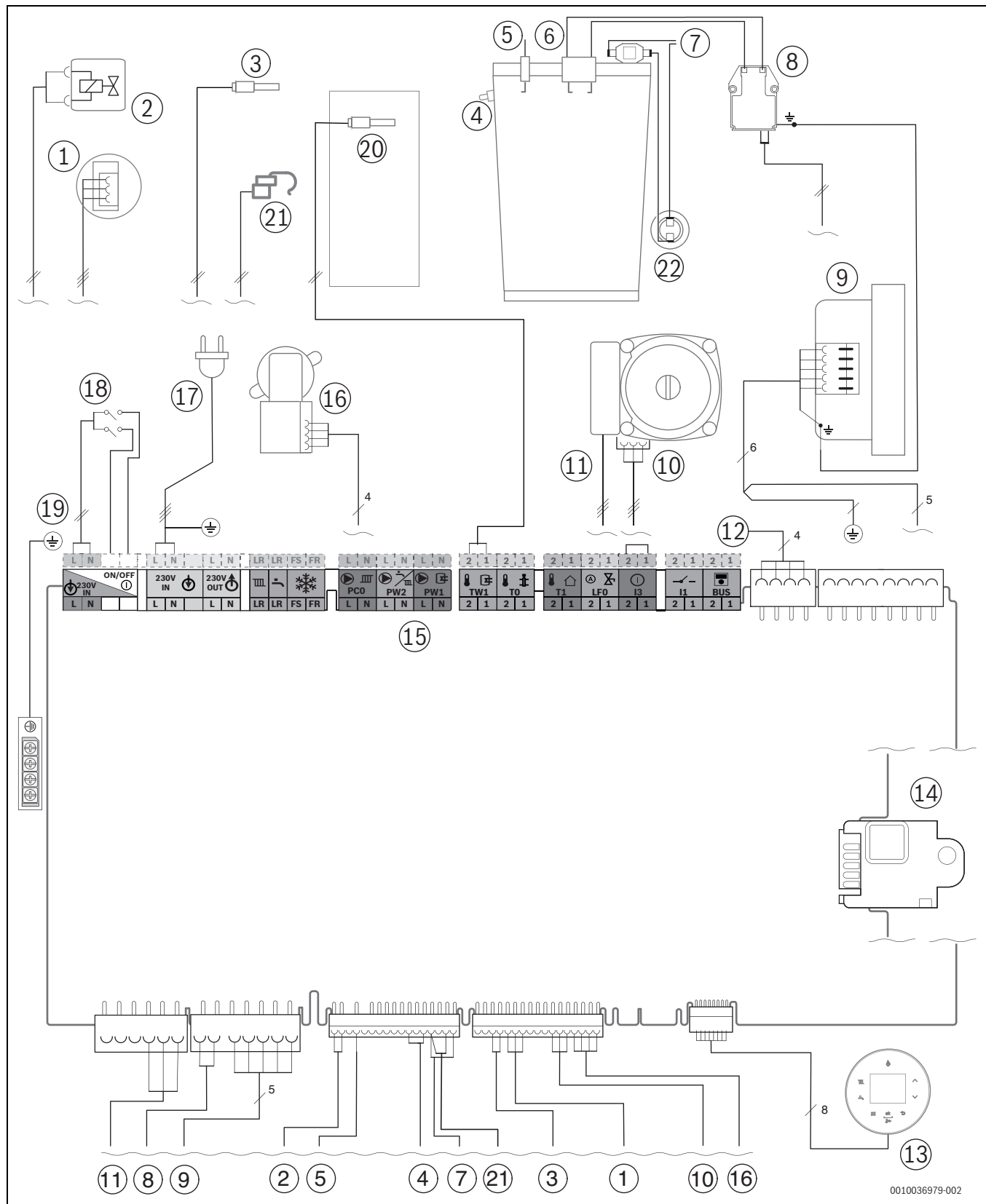
Bild 92 Elektrische Verdrahtung
