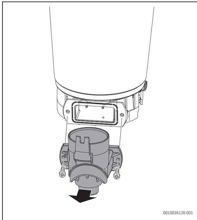
Bild 68 Prüföffnung öffnen
