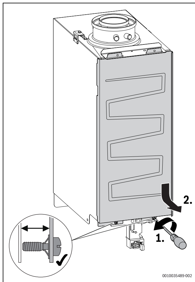
Bild 51 Brennerhaube abnehmen
