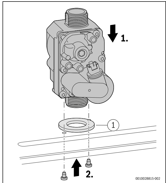
Bild 82 Gasarmatur einbauen
