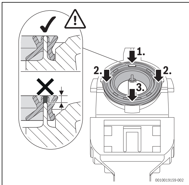
Bild 74 Dichtung andrücken
