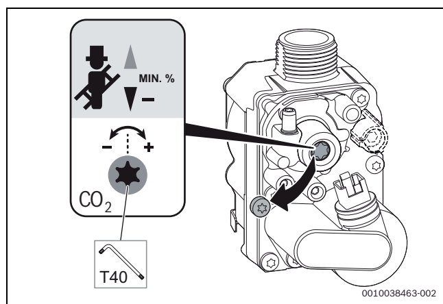
Bild 55 CO 2 /O 2 -Gehalt bei minimaler Nennwärmeleistung einstellen
