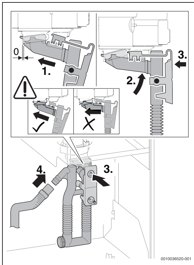
Bild 75 Kondensatsiphon einsetzen
