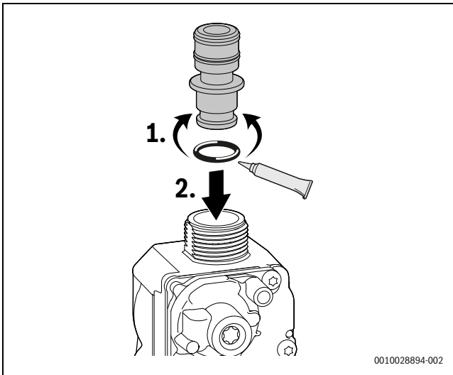
Bild 84 Gassdrossel einsetzen
