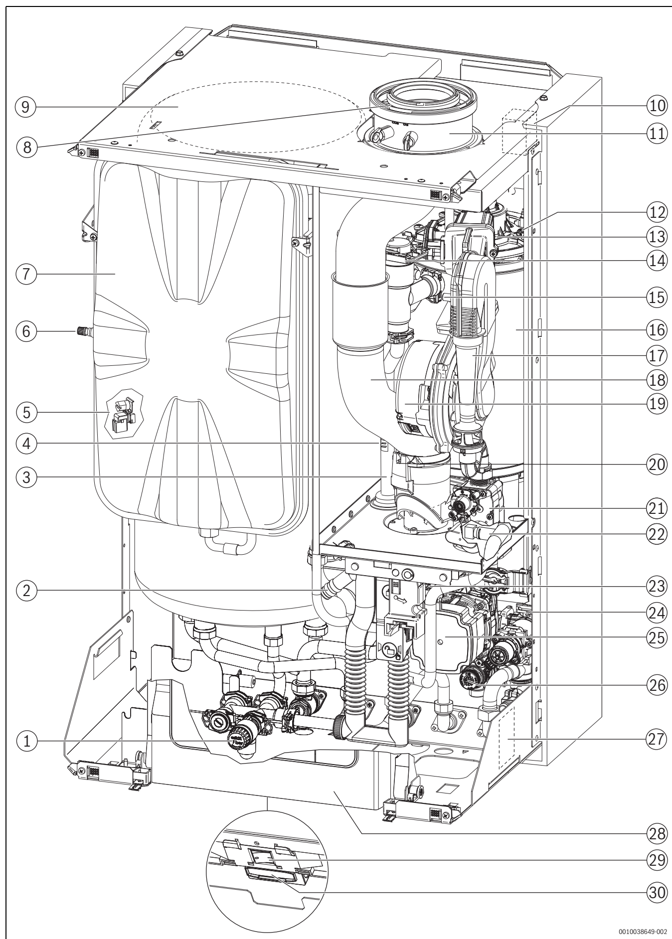
Bild 4 Produktübersicht
