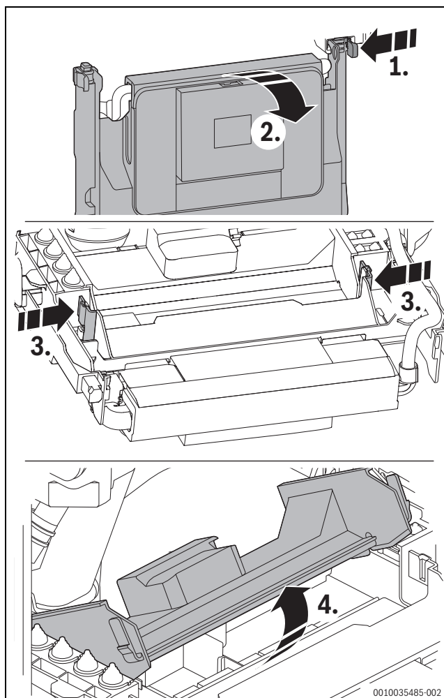
Bild 44 Steuergerät öffnen
