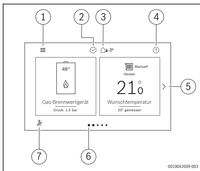
Bild 48 Systembedieneinheit
