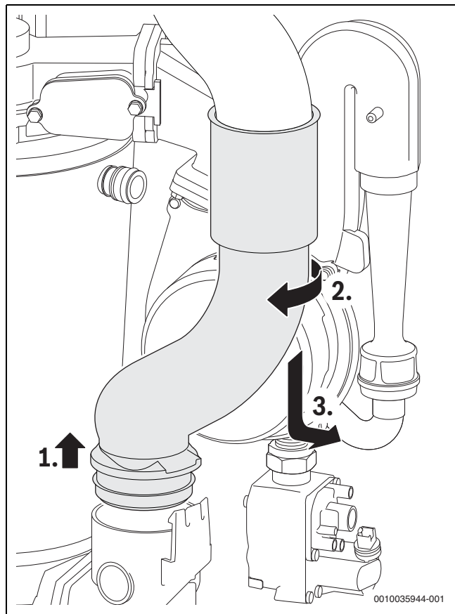
Bild 58 Abgasrohr ausbauen
