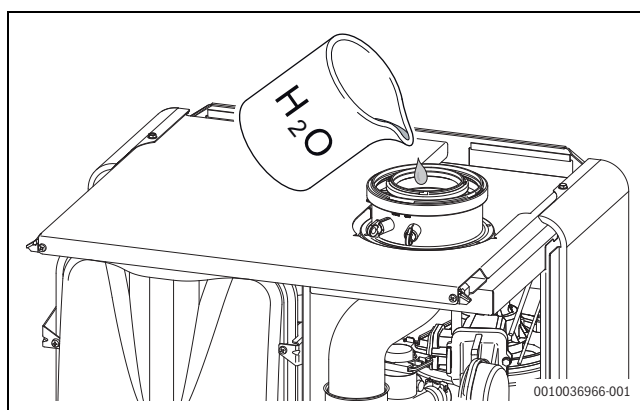
Bild 40 Kondensatsiphon mit Wasser füllen
