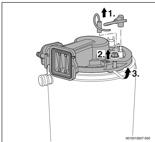
Bild 60 Brennerdeckel lösen
