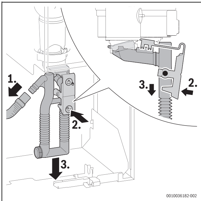
Bild 70 Kondensatsiphon ausbauen
