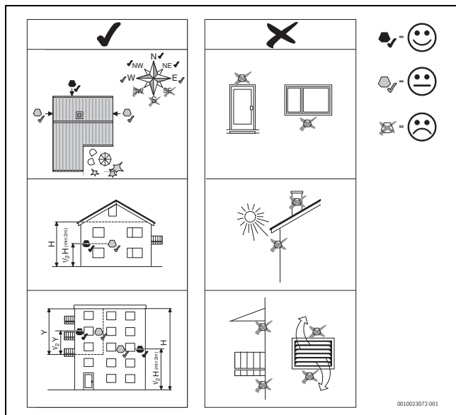
Bild 42 Installationsort Außentemperaturfühler
